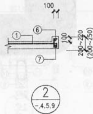
图名 平衡板式阳台C1型平面及详图
