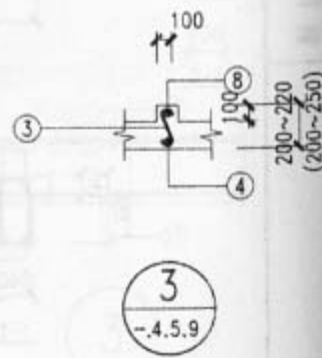
图名 平衡板式阳台C1型平面及详图
