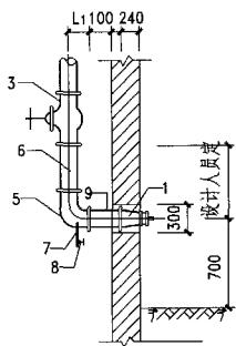
丙型平面图
