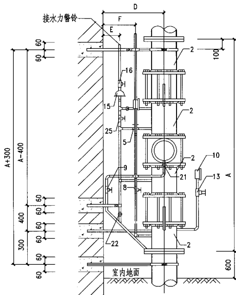
侧视图
