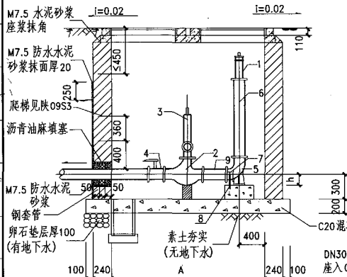
1-1 剖面图
