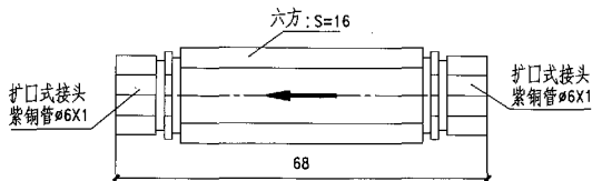
图 9 气路单向阀
