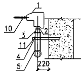
1-1剖面
