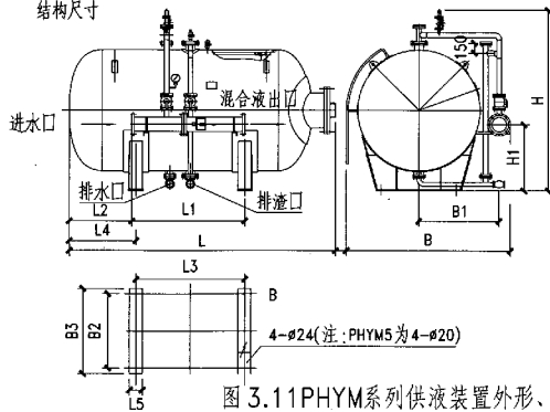
结构尺寸
