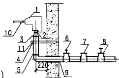
1-1剖面
