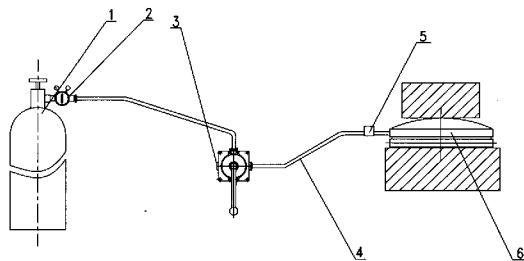
1 高压气瓶 2 氮气减压阀 3 操作控制阀 4 联接管 5 快速接头 6 起重气垫
