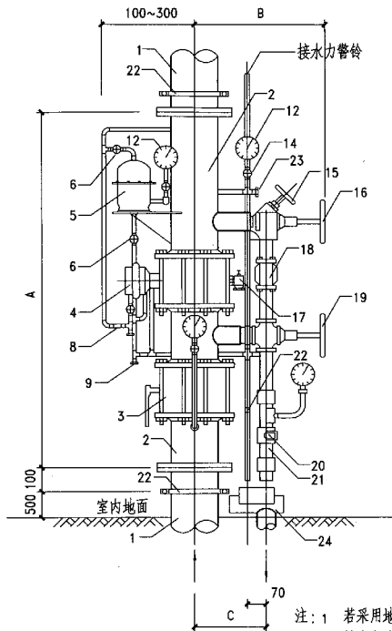
正视图
