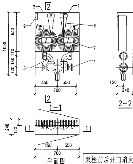
单栓前后开门灭火栓箱(甲型)
