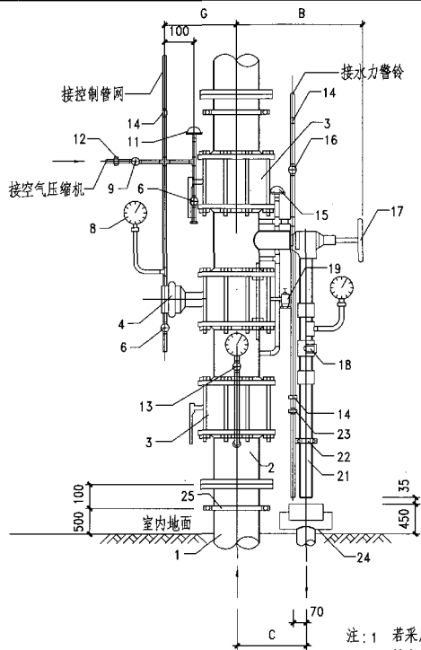
正视图
