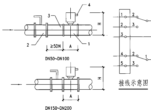
1 水流指示器 2 信号阀门 3 短管 4 接线柱
