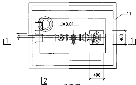
平面图
