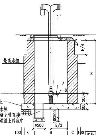
2-2 剖面图
