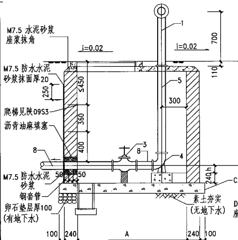
1-1 剖面图
