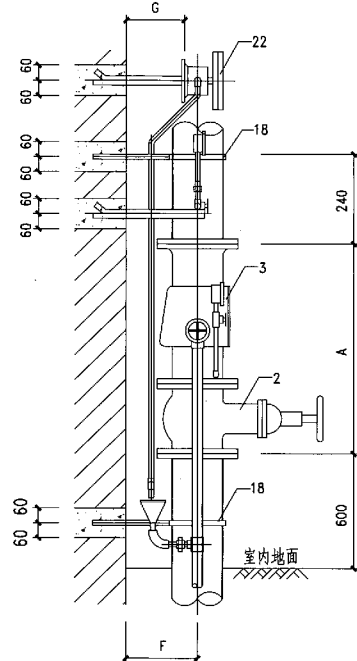
侧视图
