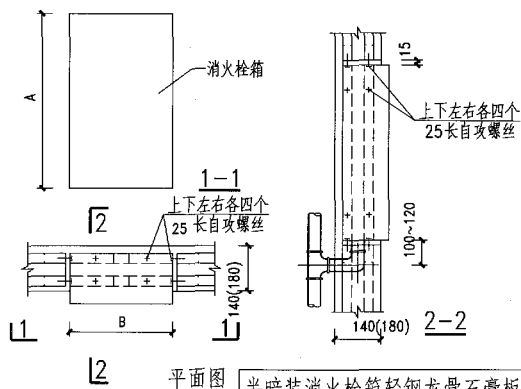
半暗装消防栓箱轻钢龙骨石膏板上安装固定图
