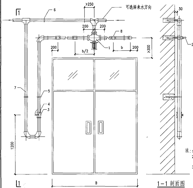
正视图
