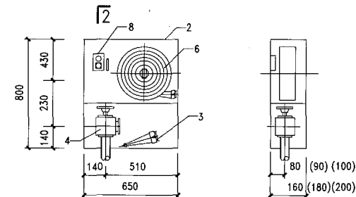
1-1 剖面图
