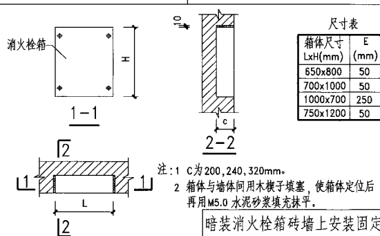
图名 室内消防栓箱安装固定图
