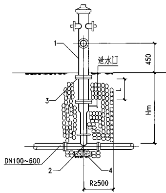
1-1 剖面图
