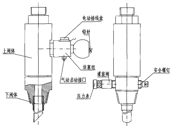
图7 瓶头阀
