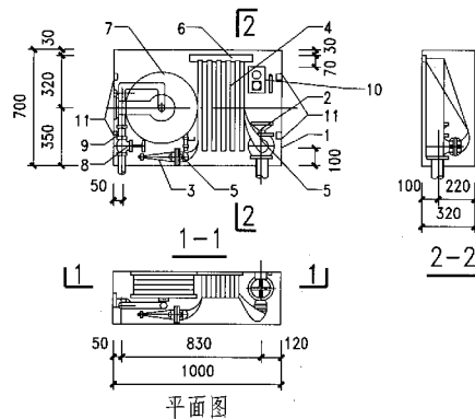
乙型室内消火栓,消防软管卷盘组合型安装图
