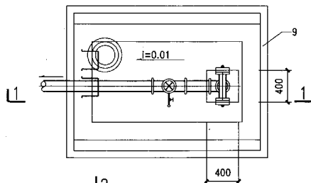
平面图
