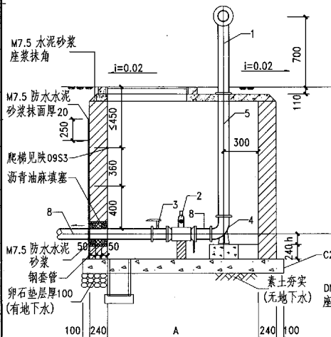
1-1 剖面图
