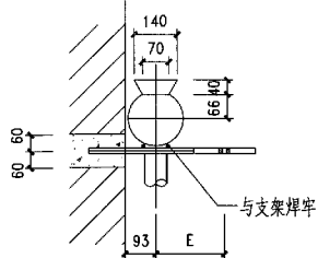
侧视图
