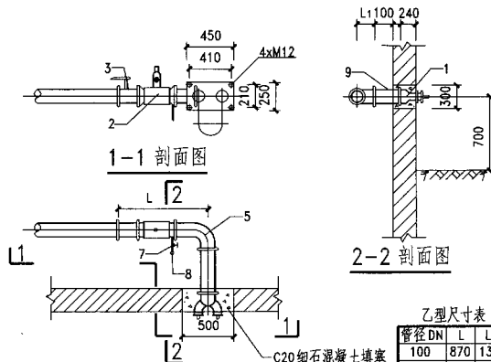
乙型平面图
