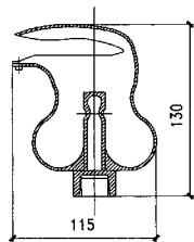
图 3 槽边型(3型) 二氧化碳喷头
