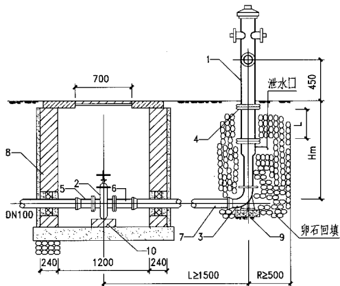
1-1 剖面图
