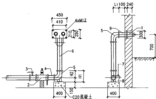
1-1 剖面图
