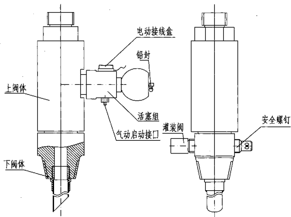
图7 瓶头阀
