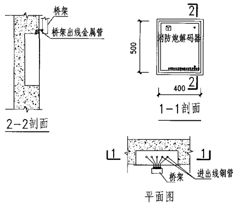
乙型固定消防炮解码器暗装
