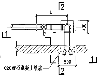
甲型平面图
