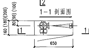
平面图
