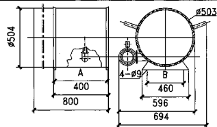
图3.3.7PFS3 型高倍泡沫发生器外形及安装尺寸
