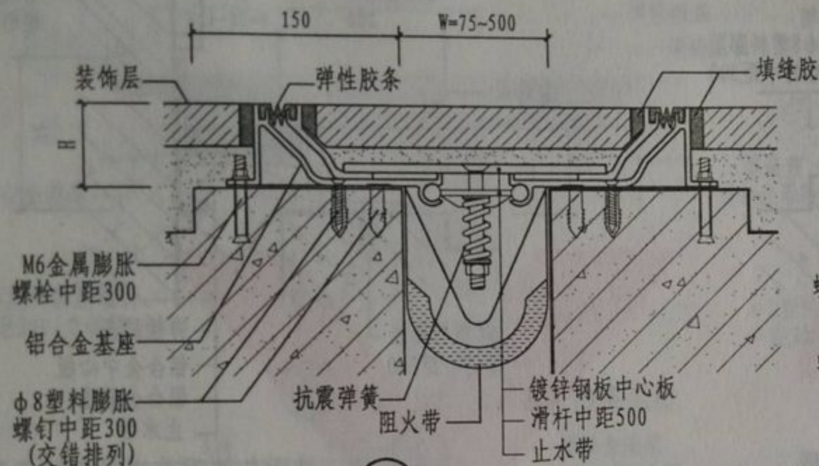
① 楼、地面双列防震型
