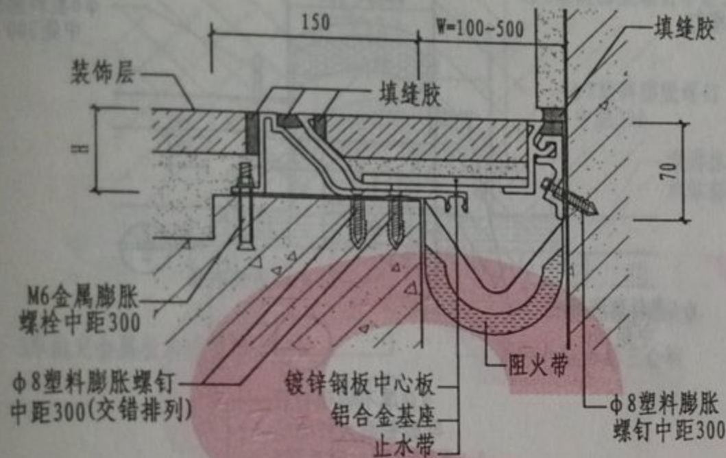
① 楼、地面与墙面胶条防震型
