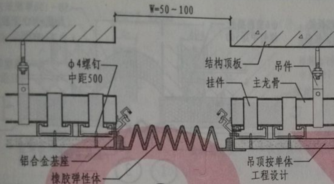
① 吊顶橡胶防震 I 型
