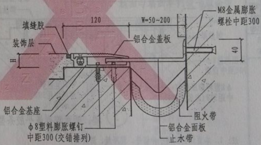
④ 楼、地面与墙面金属卡锁承重型
