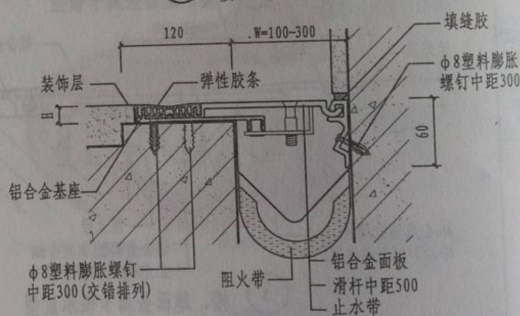
④ 楼、地面与墙面双列嵌平胶条型
