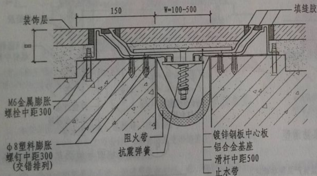
③ 楼、地面胶条防震型
