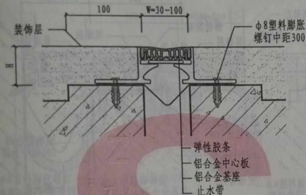
① 楼、地面单列嵌平胶条型
