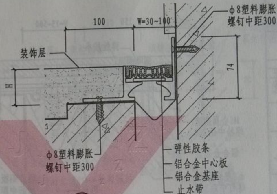
② 楼、地面与墙面单列嵌平胶条型
