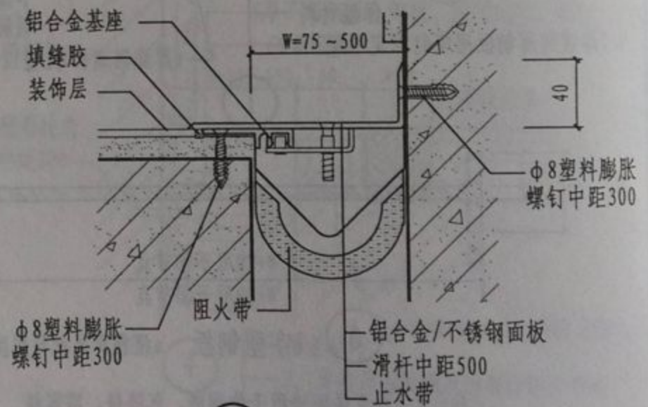
④ 楼、地面与墙面金属盖板型 (后装)
