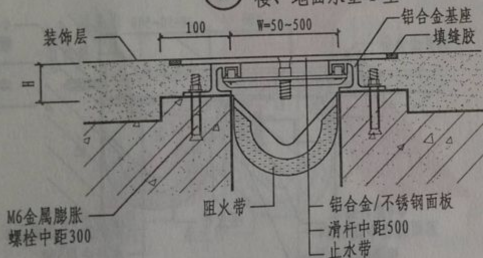
③ 楼、地面承重 II 型
