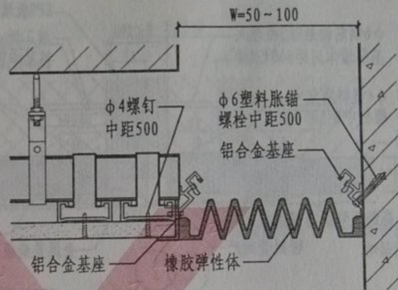
② 吊顶与内墙橡胶防震 I 型
