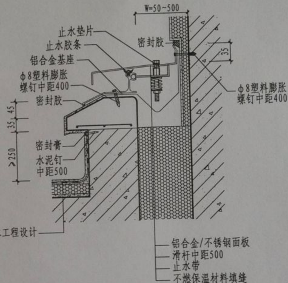
② 屋面与墙面金属盖板防震型
