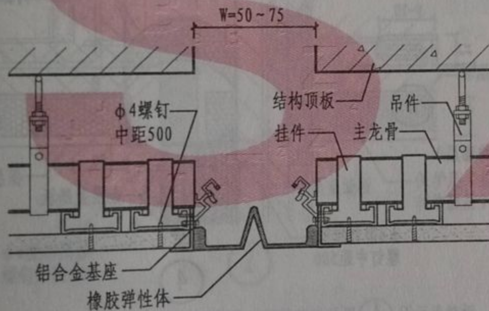
③ 吊顶橡胶防震 II 型
