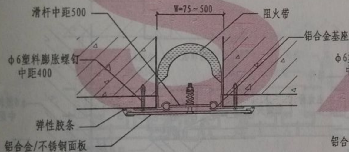
③ 内墙、顶棚金属盖板防震型
