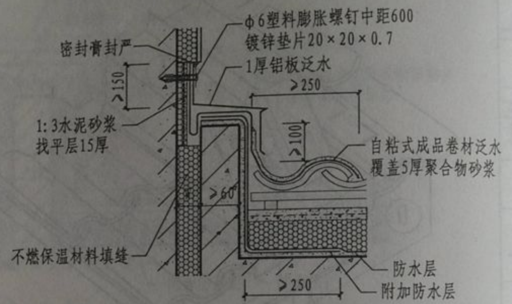
3 高低跨变形缝
