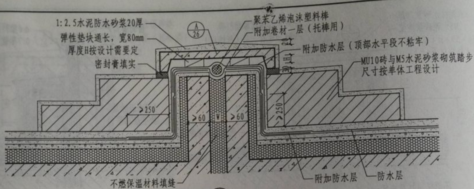
① 屋面消防疏散通道变形缝
