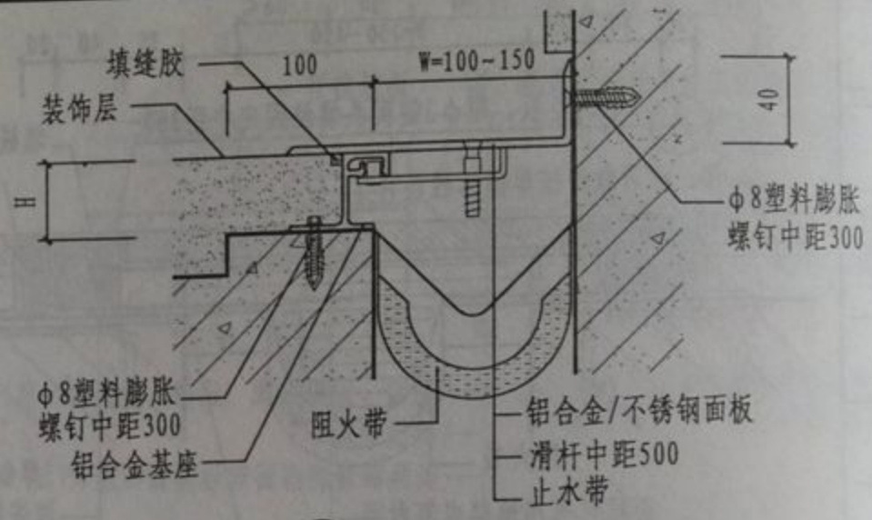
② 楼、地面与墙面金属盖板型
