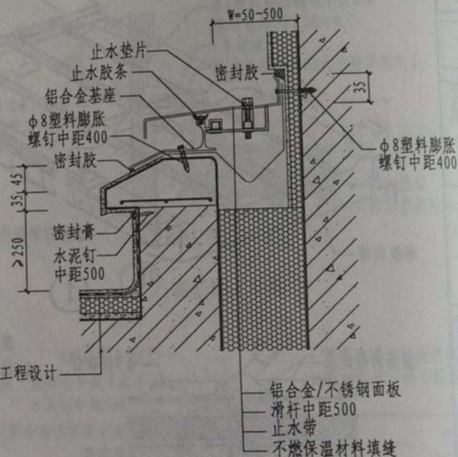
② 屋面与墙面金属盖板型
