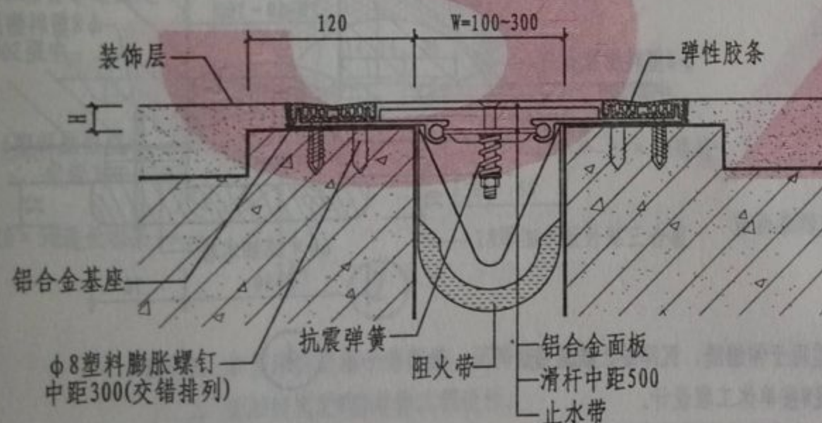
③ 楼、地面双列胶条防震型
