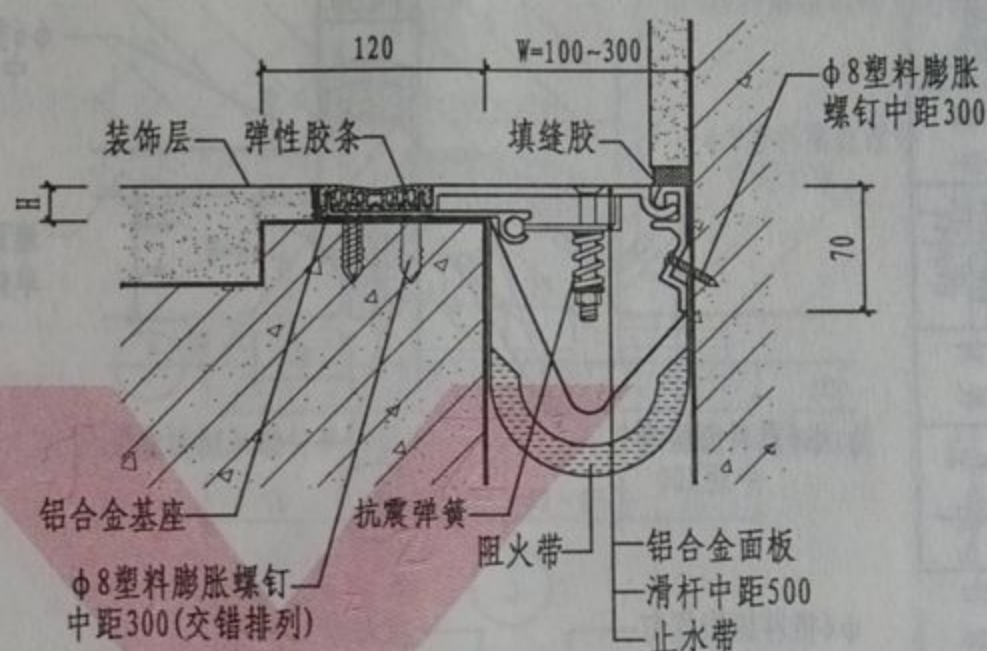
② 楼、地面与墙面双列胶条防震型
