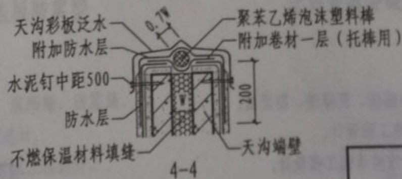
坡屋面变形缝(五)
