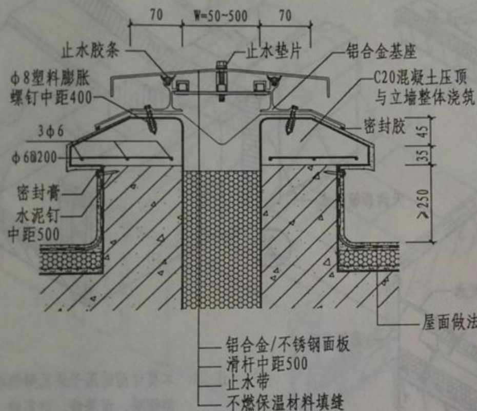
① 屋面金属盖板型
