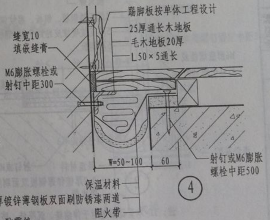
楼、地面变形缝(二)
