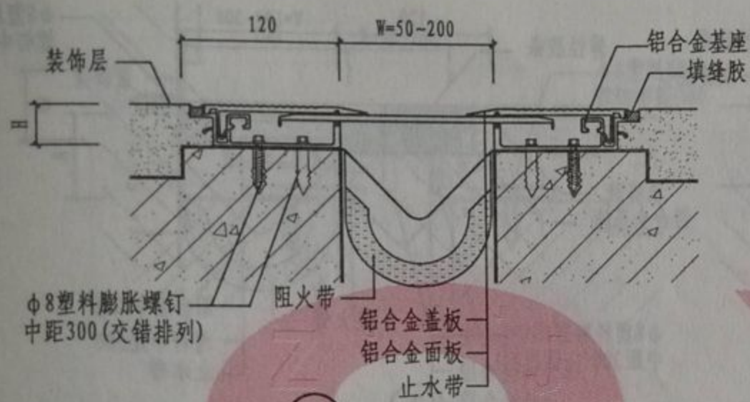
① 楼、地面金属卡锁型
