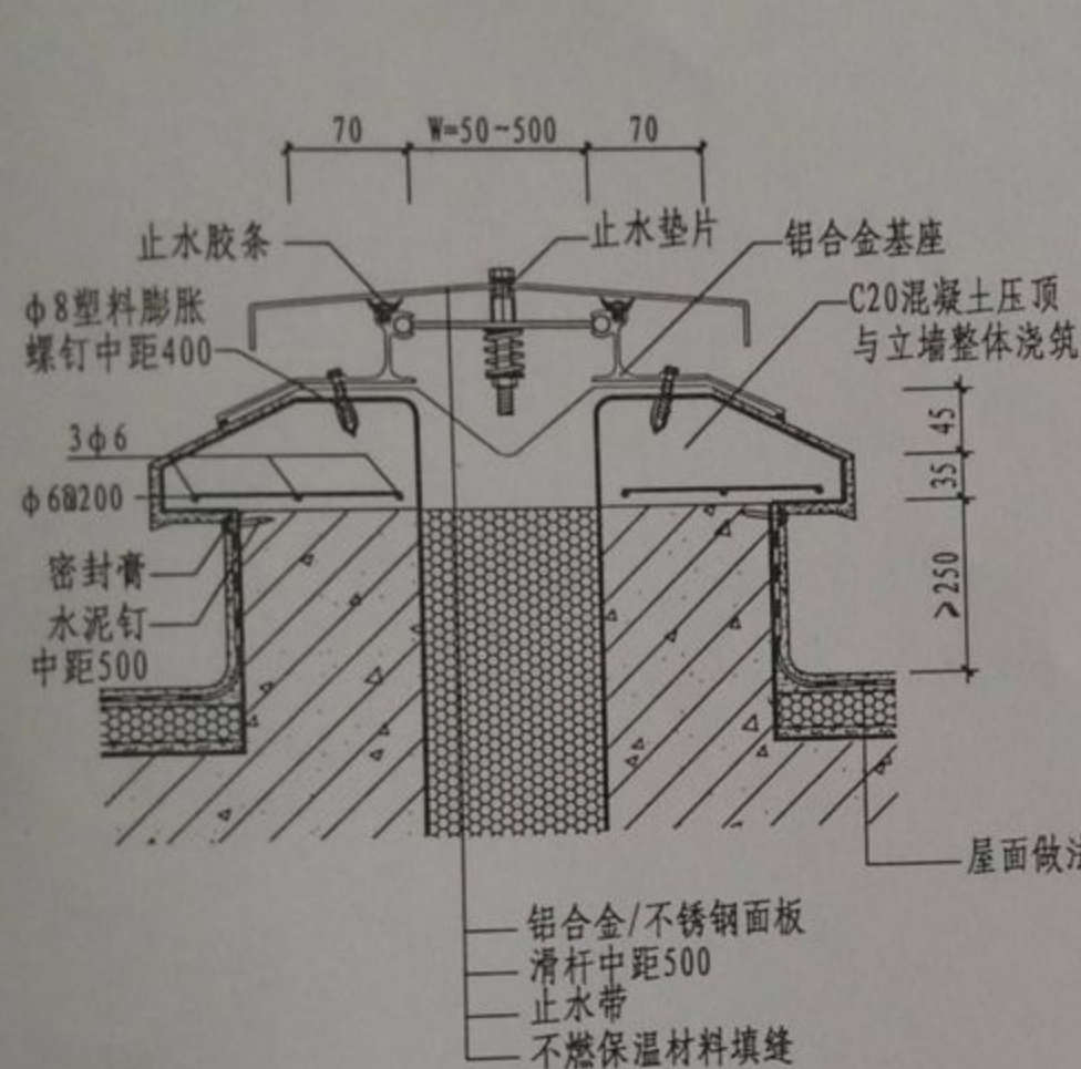
① 屋面金属盖板防震型
