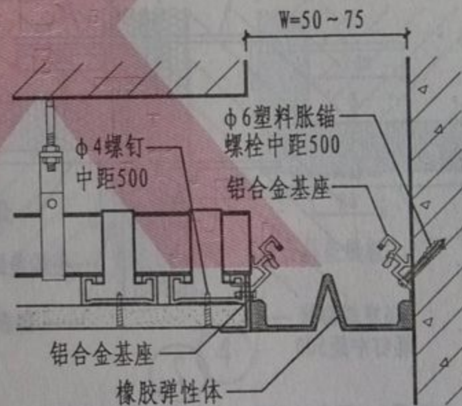
④ 吊顶与内墙橡胶防震 II 型
