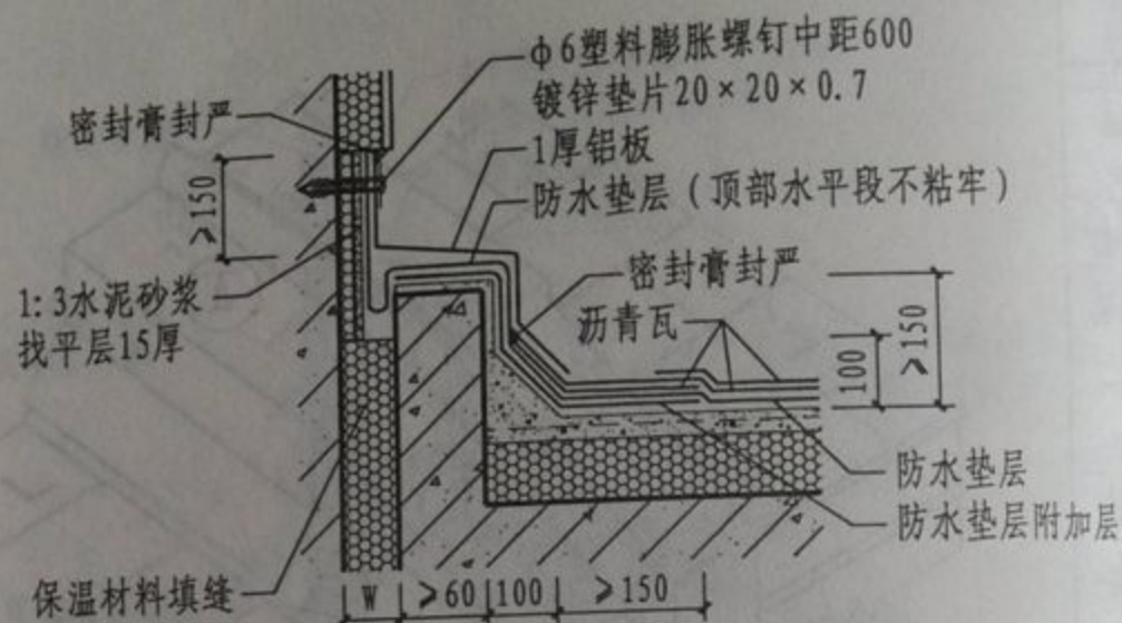
② 高低跨变形缝
