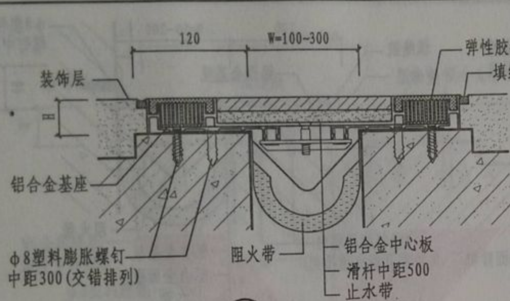
① 楼、地面双列嵌平胶条深型
