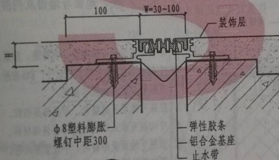
③ 楼、地面单列嵌平胶条防滑型
