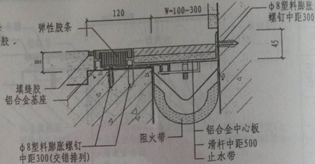
② 楼、地面与墙面双列嵌平胶条深型
