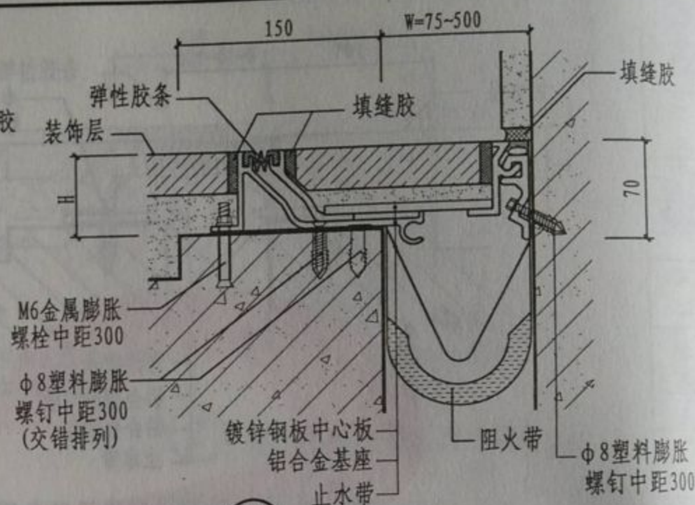
② 楼、地面与墙面双列防震型
