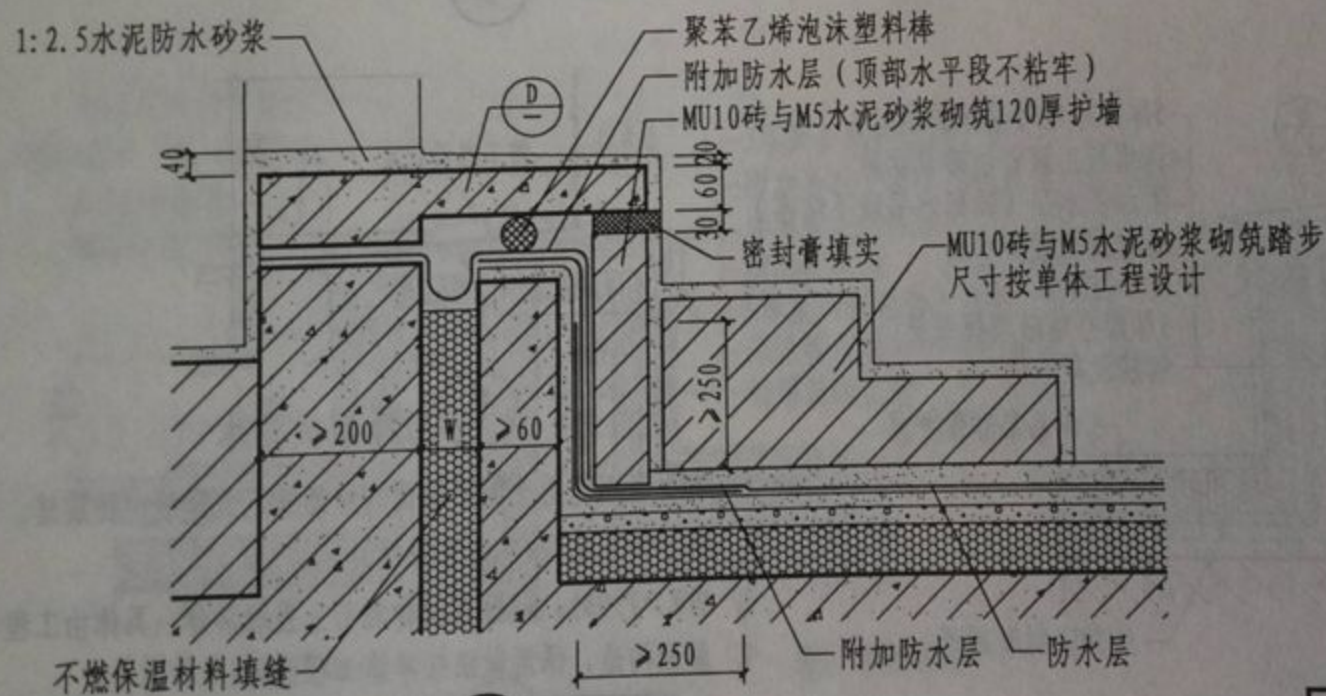
② 屋面出入口变形缝
