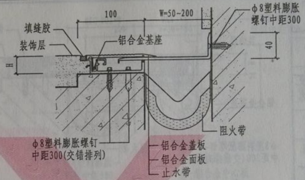
② 楼、地面与墙面金属卡锁型
