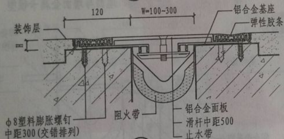
③ 楼、地面双列嵌平胶条型
