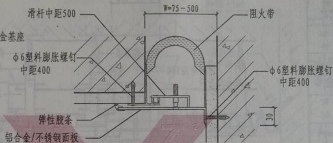
② 内墙、顶棚与内墙金属盖板型
