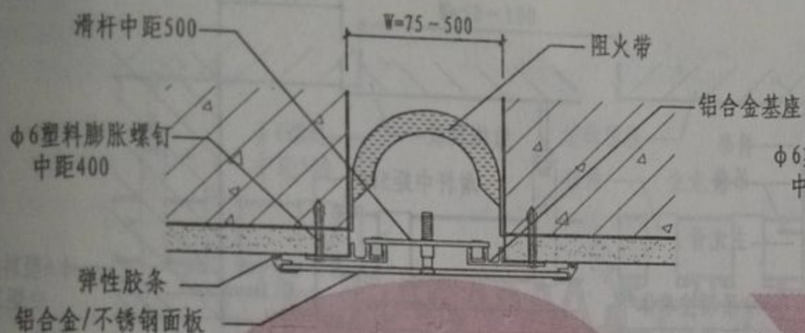
① 内墙、顶棚金属盖板型
