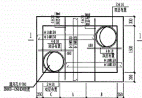
顶板配筋图
