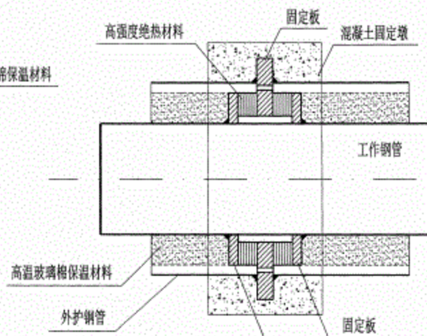
直埋蒸汽管道内外固定支座
