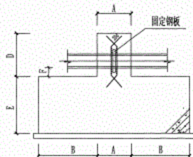
固定墩抗挤压详图
