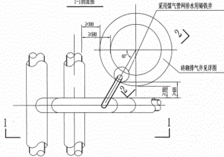
直埋管道分支跨越管安装平面图
