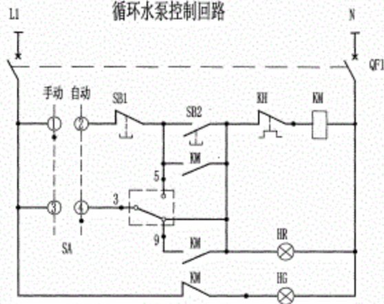
电动机直接起动控制原理图
