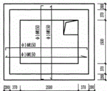
底板配筋图
