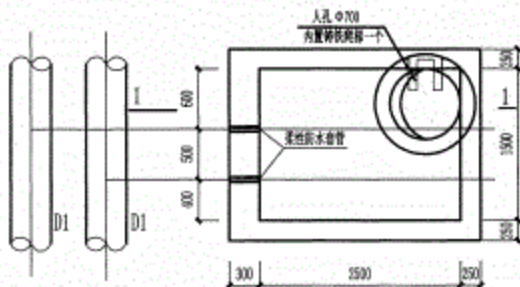
平面图
