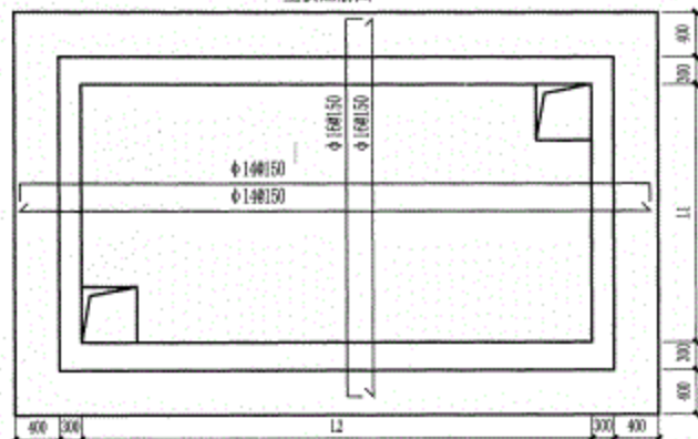
底板配筋图
