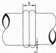
图5.1.2 接头对正性示意
