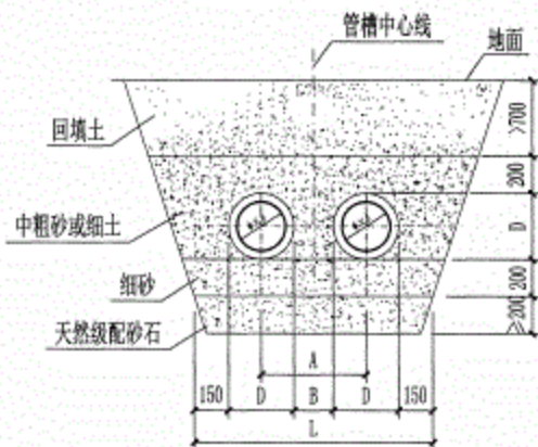
适用于有地下水的直埋管道
