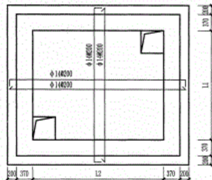
底板配筋图
