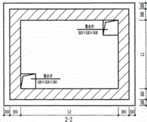
DN50~DN400现浇盖板 热水管道阀门检查井砖结构 (一)
