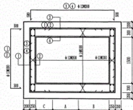
侧板配筋图
