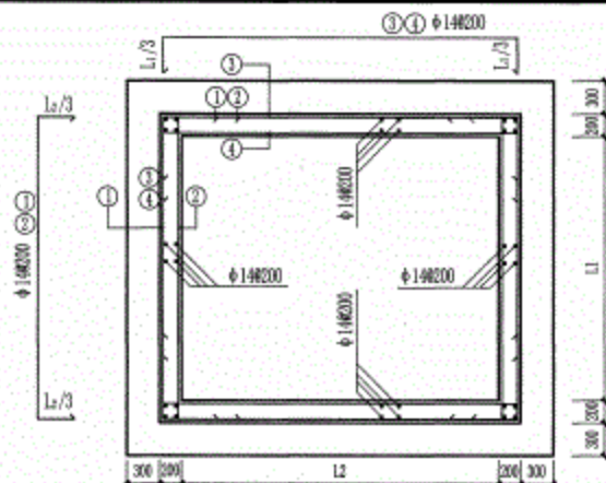
壁板配筋图
