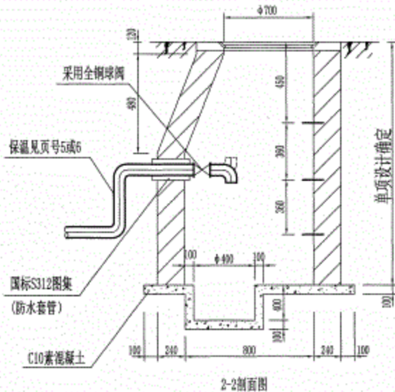
2-2剖面图
