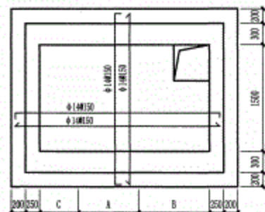
底板配筋图
