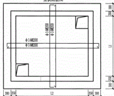
底板配筋图
