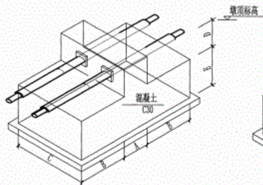
固定墩模板图
