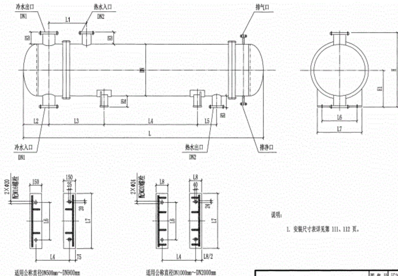
波节管水-水换热器样图
