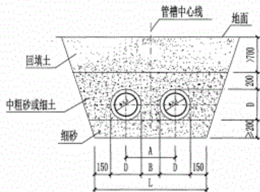
适用于无地下水的直埋管道
