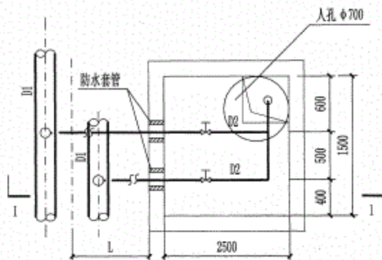
平面图
