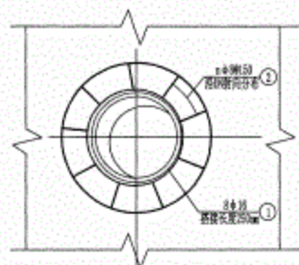
套管加固平面图
