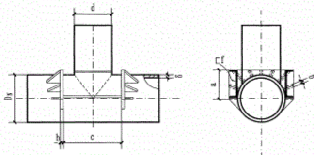
III型加固方案
