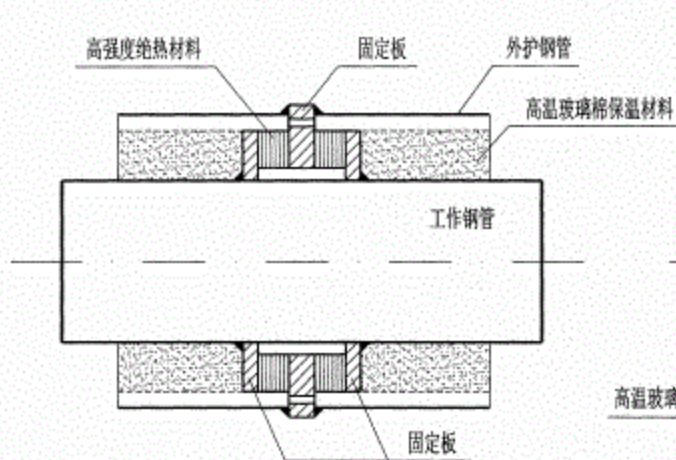
直埋蒸汽管道内固定支座
