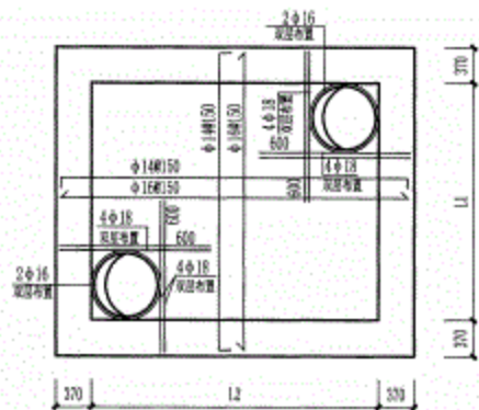
顶板配筋图
