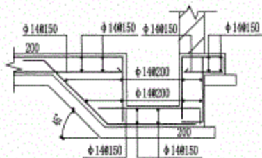
集水井配筋图
