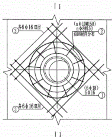
防水套管加固图
