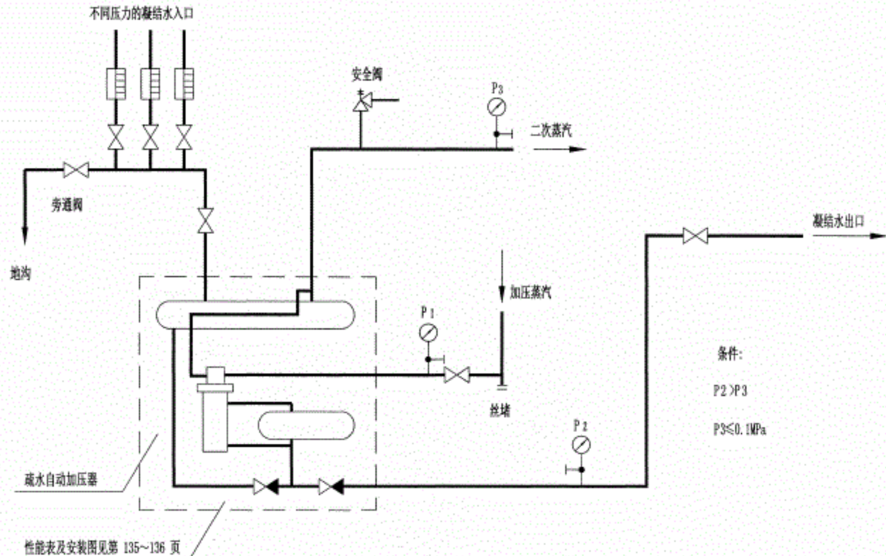
疏水加压器回收二次蒸汽系统
