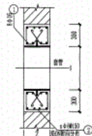
套管加固剖面图
