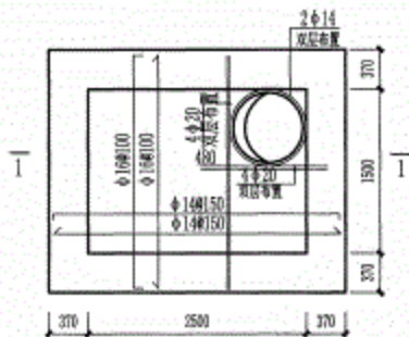
顶板配筋图
