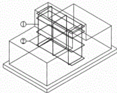
固定墩配筋图
