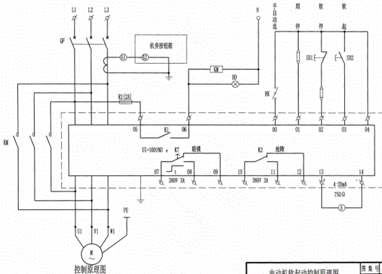
电动机软启动控制原理图
