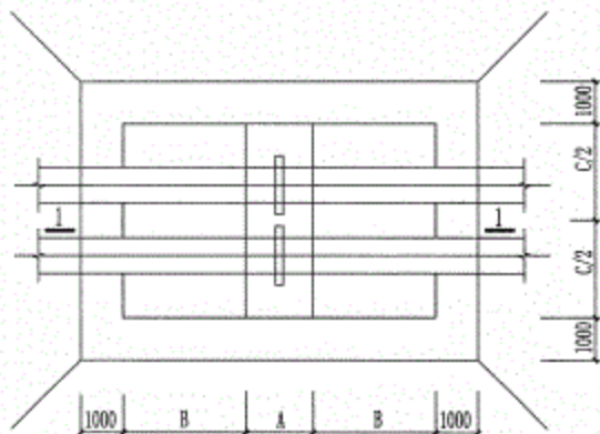
固定墩回填砂子平面图
