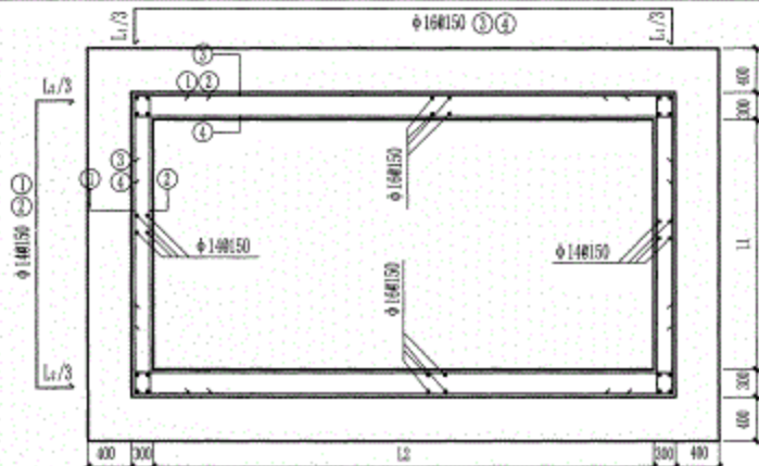
墙板配筋图
