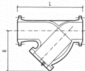
法兰连接Y型过滤器
