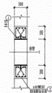
套管加固剖面图
