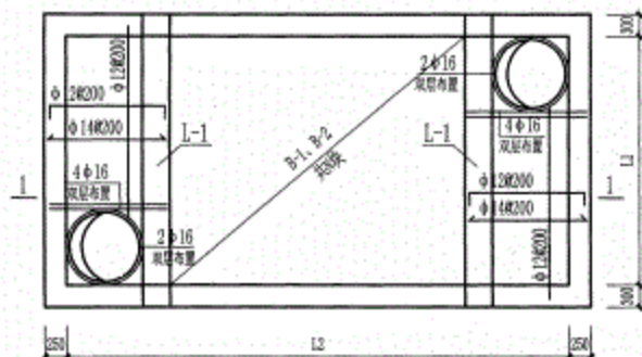
顶板配筋图
