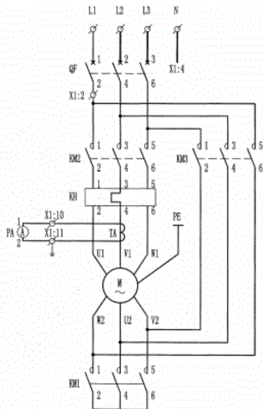
交流电动机Y-△起动控制装置 电路图
