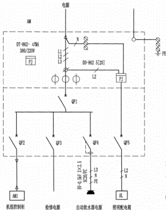
AM箱系统图
