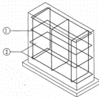
固定墩配筋图
