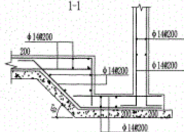
集水井配筋图
