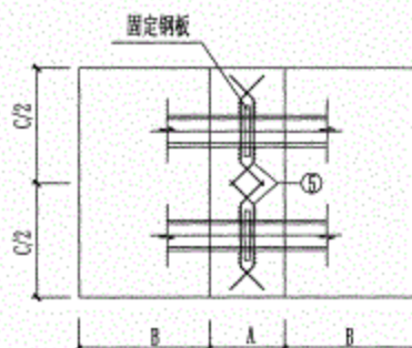
固定墩抗挤压详图
