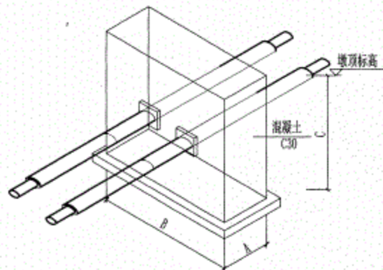
固定墩模板图
