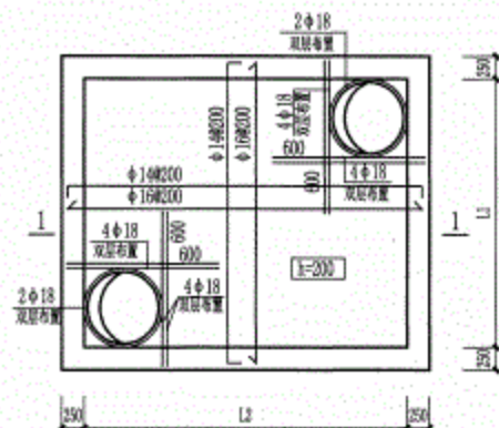
顶板配筋图
