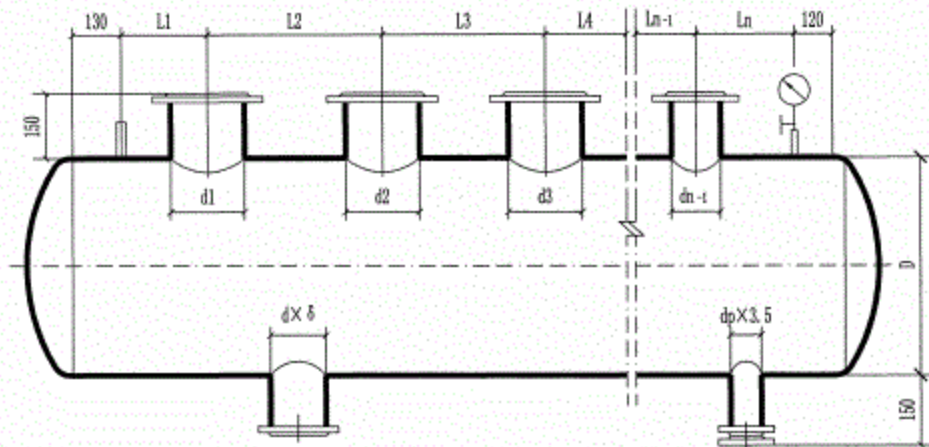
集、分水器安装示意图
