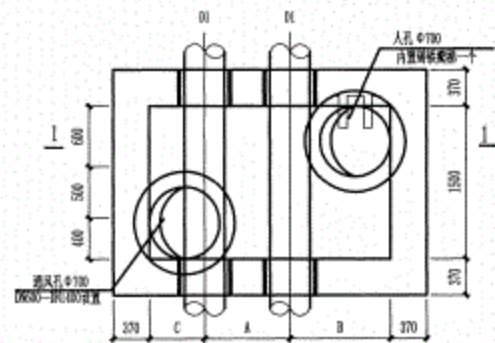
平面图
