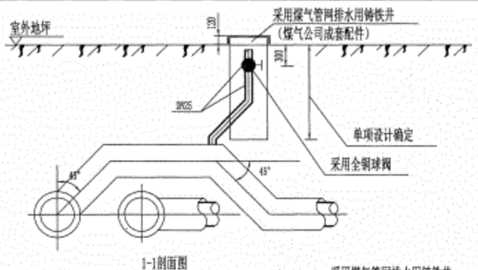
1-1剖面图
