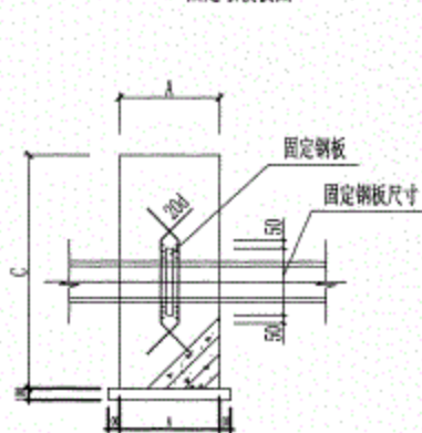
固定墩抗挤压筋详图
