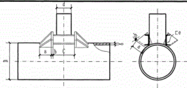
II型加固方案
