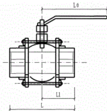
内螺纹连接球阀
