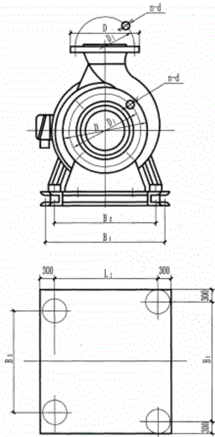
基础平面图
