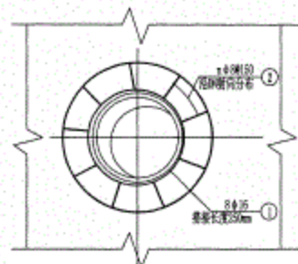
套管加固平面图
