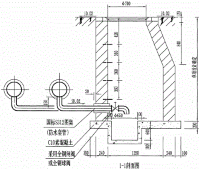
I-I剖面图
