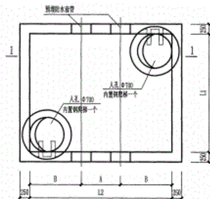
平面图
