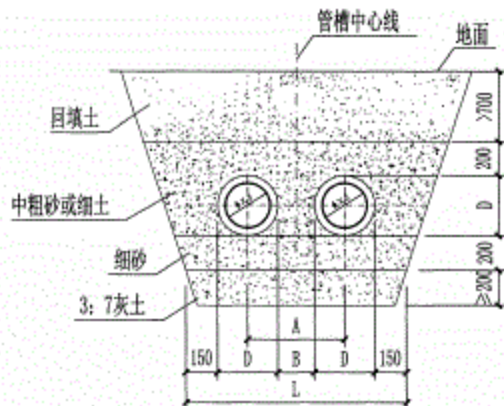
适用于湿陷性黄土的直埋管道
