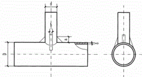
I型加固方案
