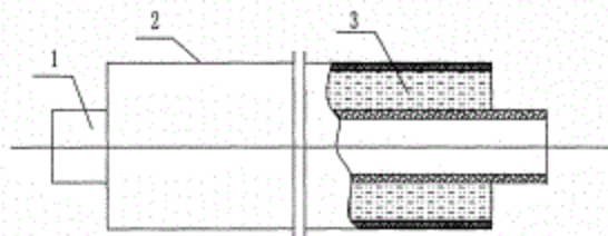
1——工作管(塑料管) 2——外护管(PE管) 3——保温层(聚氨酯)
