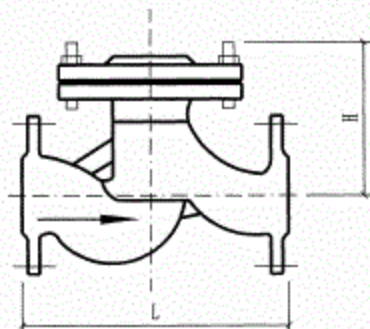
升降式止回阀
