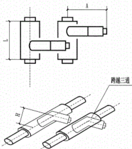
三通节点示意图
