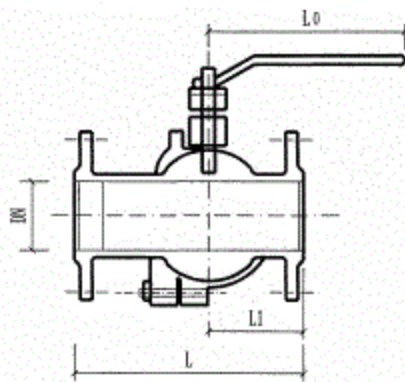
法兰连接球阀
