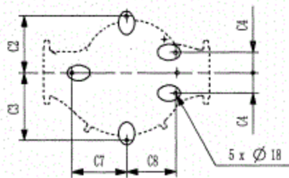
立式离心泵安装图 (二)
