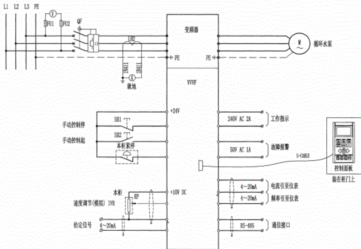
电动机变频启动控制原理图
