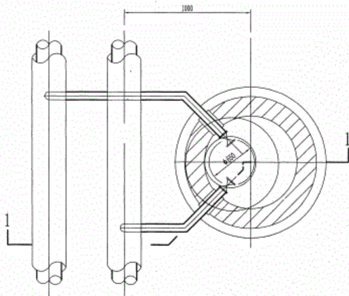
平面图
