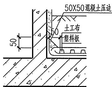
④ 边沿收口
