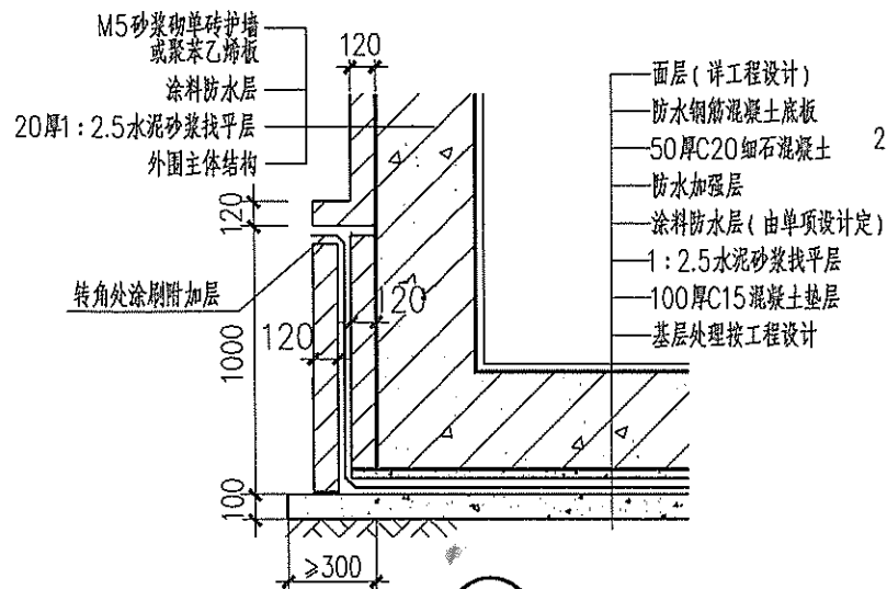
③ 接槎构造
