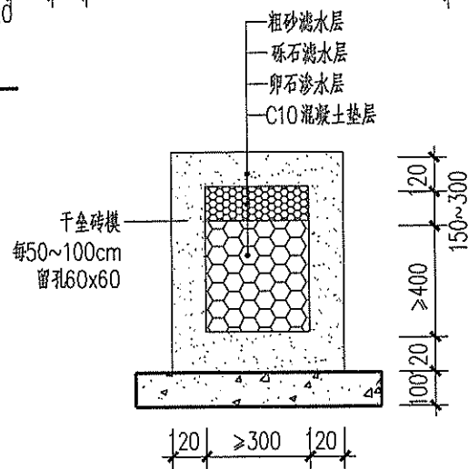
③ 无渗水管管型盲沟
