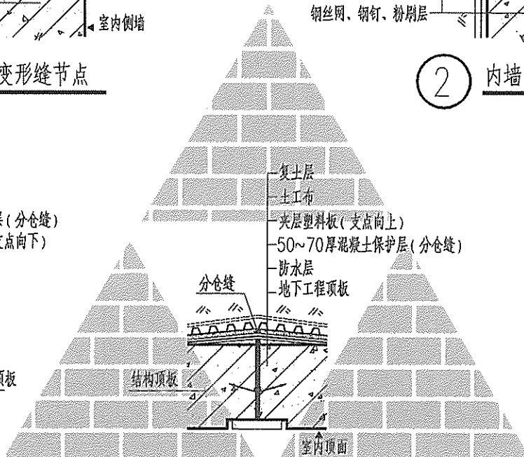
④ 顶板面层变形缝节点二
