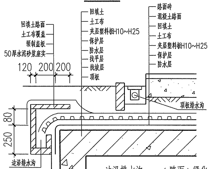
边沿排水沟, (路面+绿化)的排水路径
