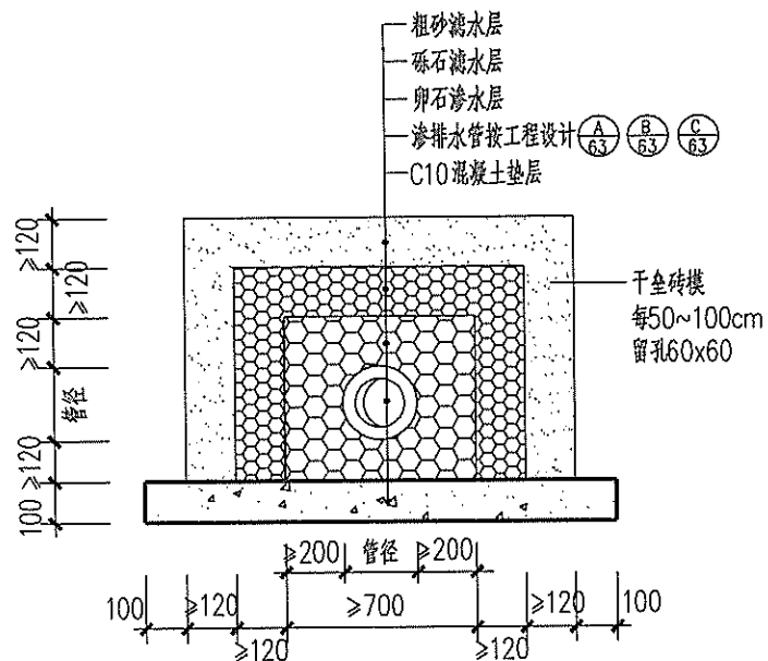
① 有渗水管型盲沟
