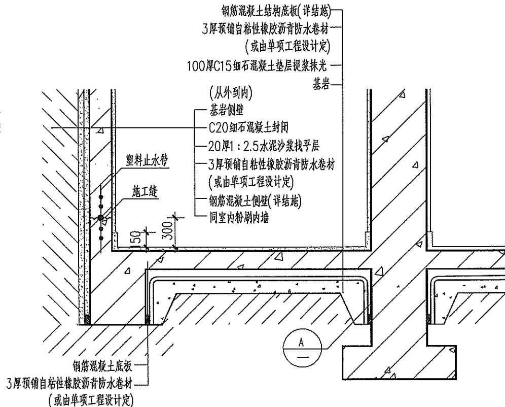
③ 侧墙与底板连接处防水大样
