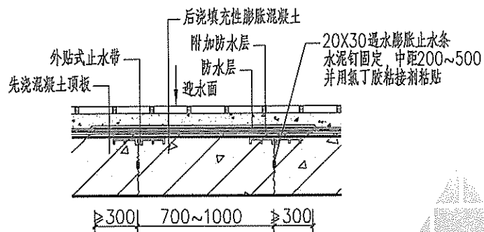
① 顶板后浇带防水构造(一)
