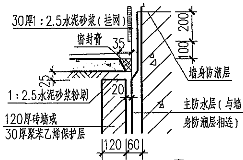
① 卷材封口
