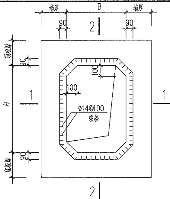
① 平面图
