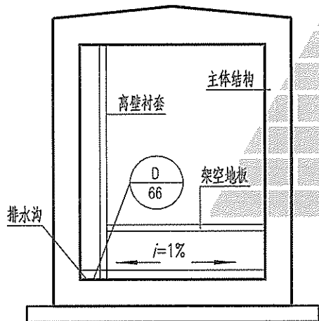
④ 综合排水
