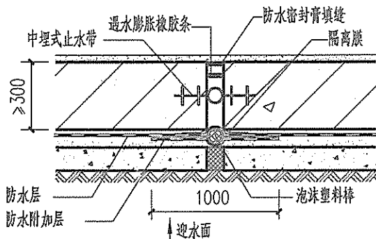
中埋式止水带变形缝<一>
