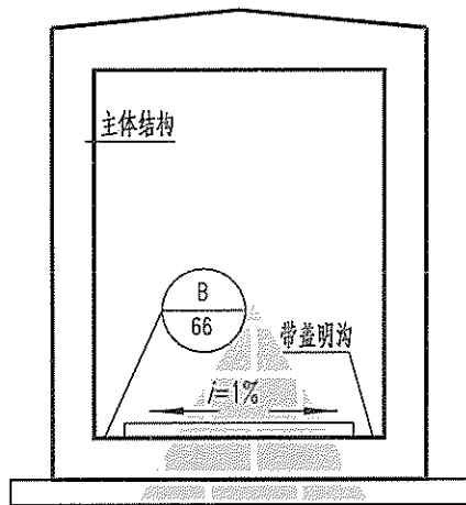
② 带盖明沟排水
