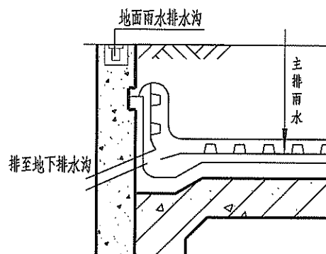
⑥ 边沿围护排水
