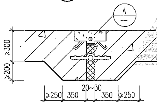
② 中埋式与可卸式止水带并用 一级防水
