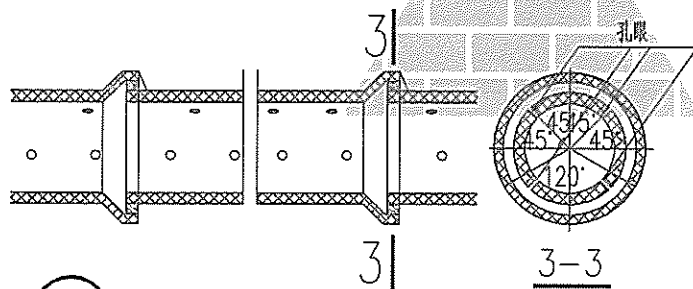
(C) 承插式一般管材渗水管
