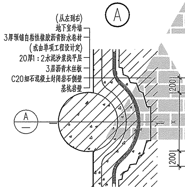
② 柱与侧墙连接防水大样 由具体设计定
