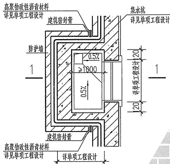
采光窗井平面 窗井与主体结构连接
