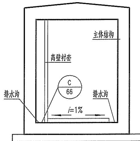
③ 夹层墙排水
