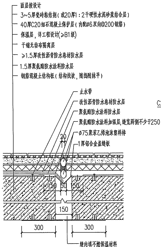
① 地下室顶板变形缝防水大样
