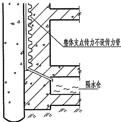
② 外墙构造与隔水仓
