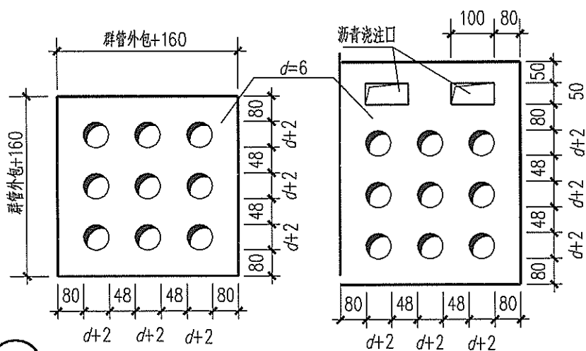
⑧ 背水面封口钢板
