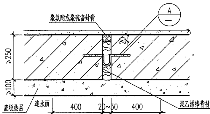
2 立墙、底板<二> 二~四级防水
