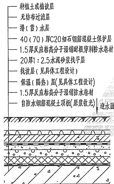
4 种植屋面/顶板防水构造
