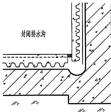
⑥ 封闭排水沟
