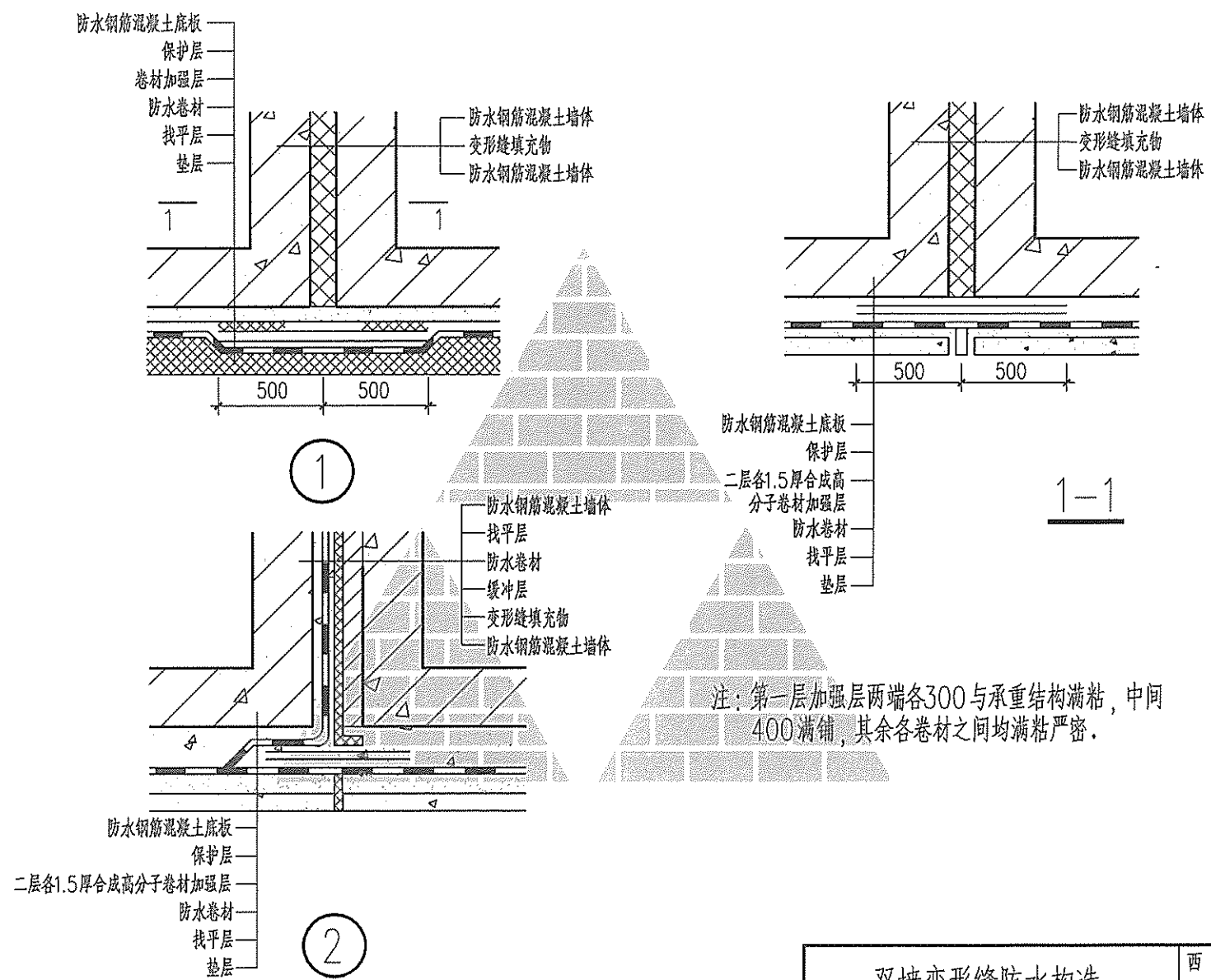
双墙变形缝防水构造
