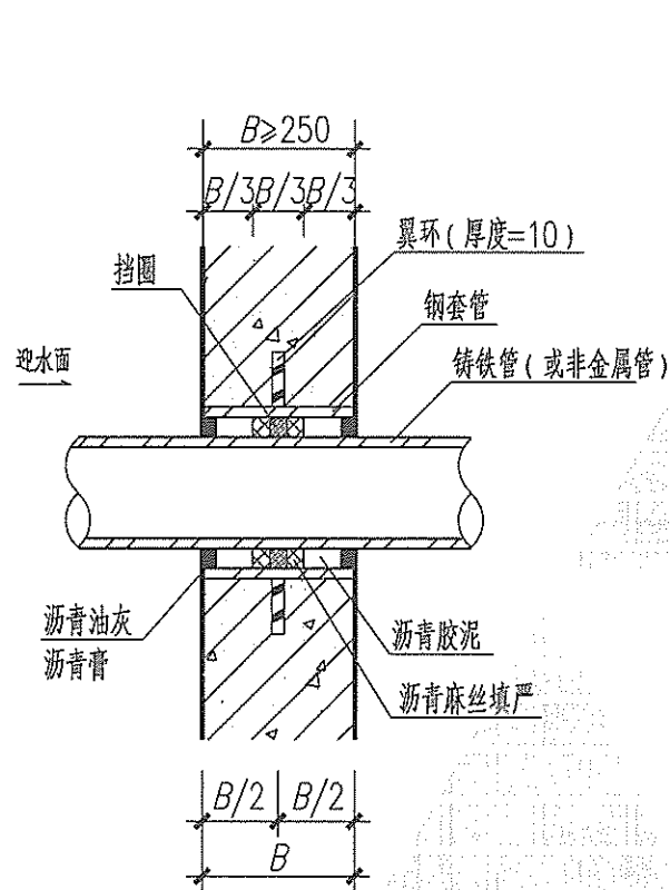
① 预埋钢套管穿墙防水构造
