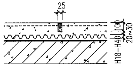
③ 底板分仓缝
