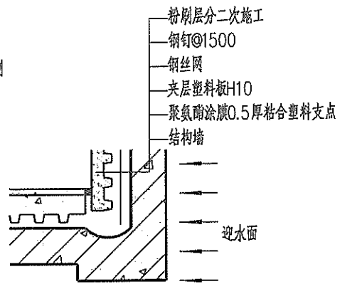
③ 内墙面防排组合构造
