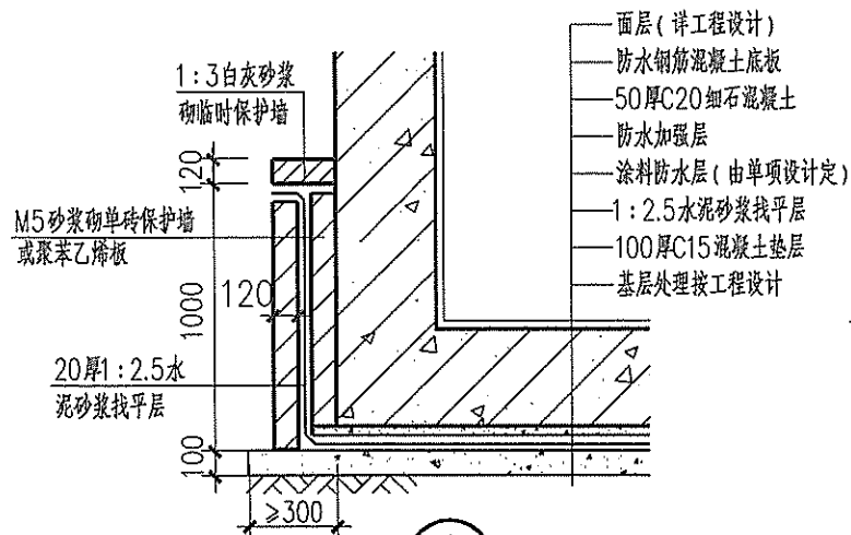
① 甩槎构造
