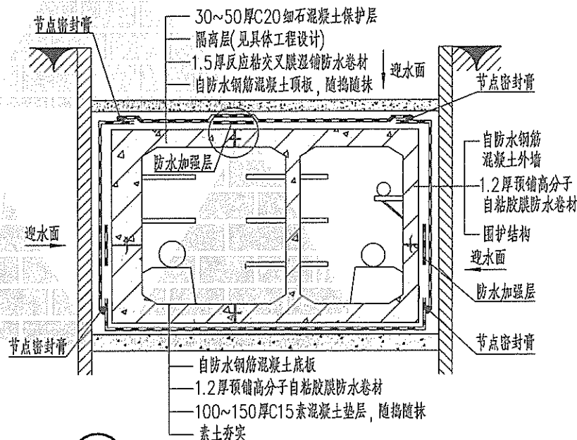
5 明挖法地下管廊防水构造(外防内贴法)
