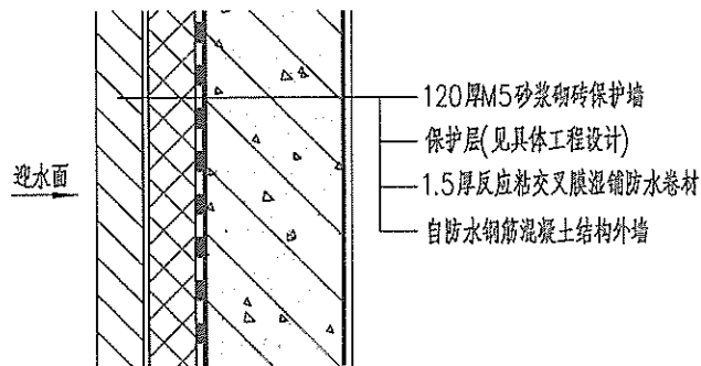
2 地下室外墙防水构造
