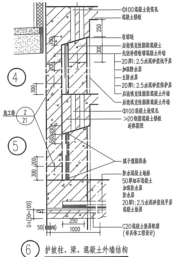
挡土桩、护坡桩、地下连续墙围护结构防水构造(二)
