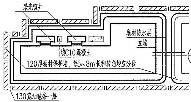
① 双墙防水卷材平面示意
