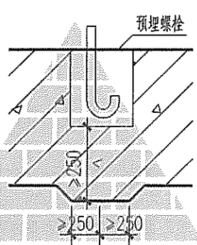
⑥ 预埋螺栓
