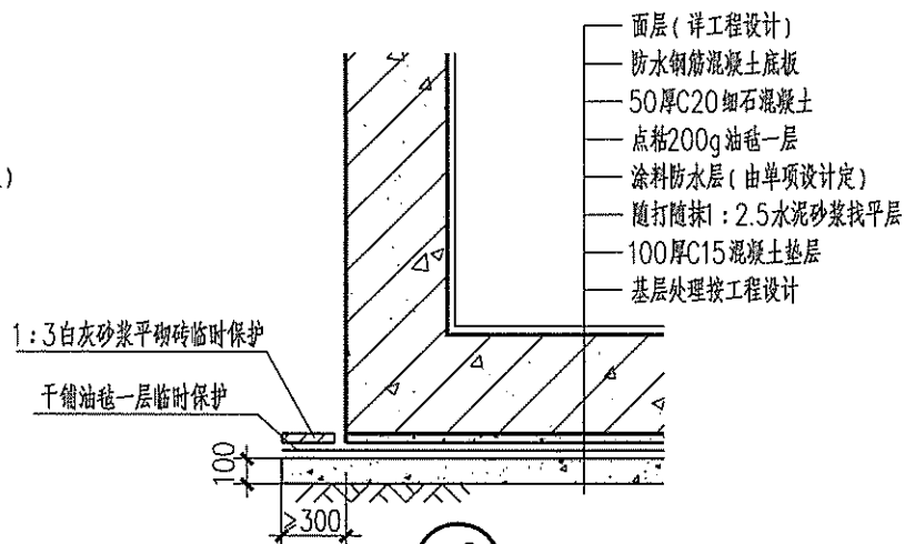
② 甩槎构造
