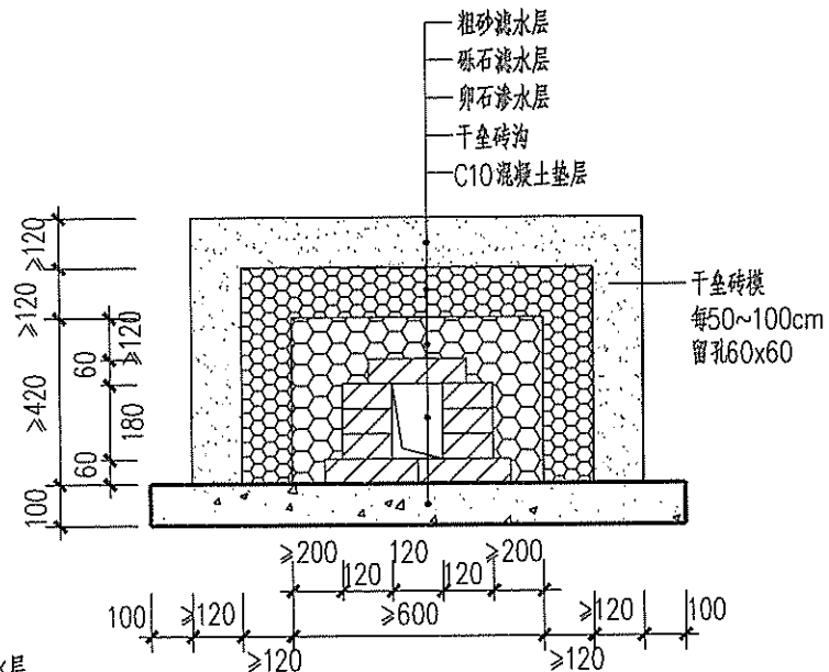
② 干垒砖盲沟
