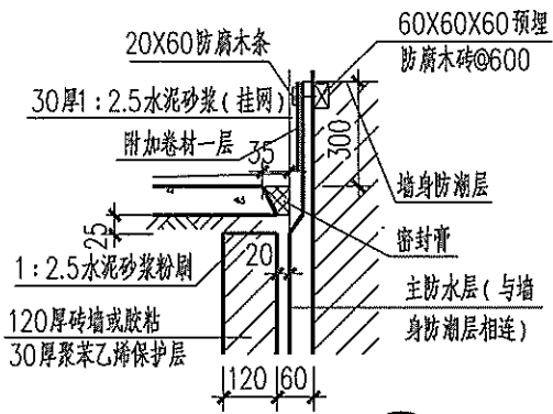
② 卷材封口
