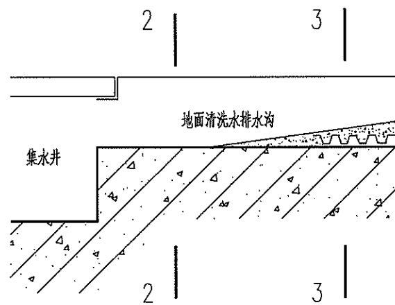
② 排水沟1-1剖面图
