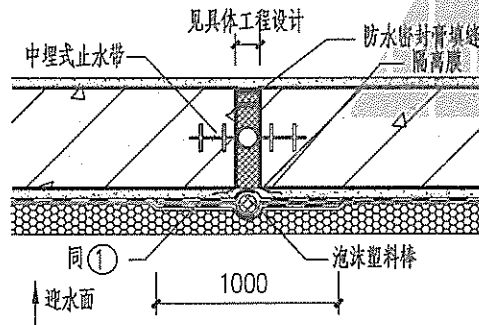
中埋式止水带变形缝<三>
