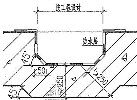
② 底板坑槽做法
