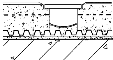
④ 排水沟3-3剖面图
