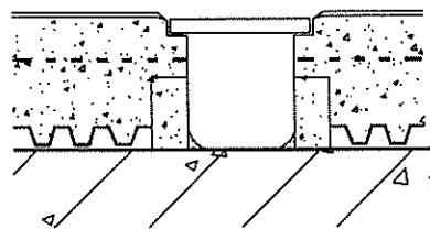
③ 排水沟2-2剖面图
