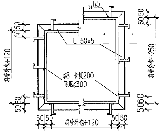
④背水面预埋件
