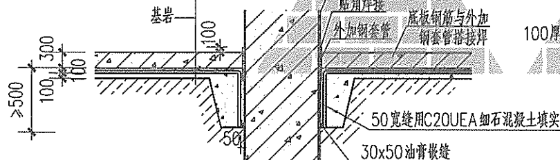
2 钢管混凝土柱与底板连接防水大样
