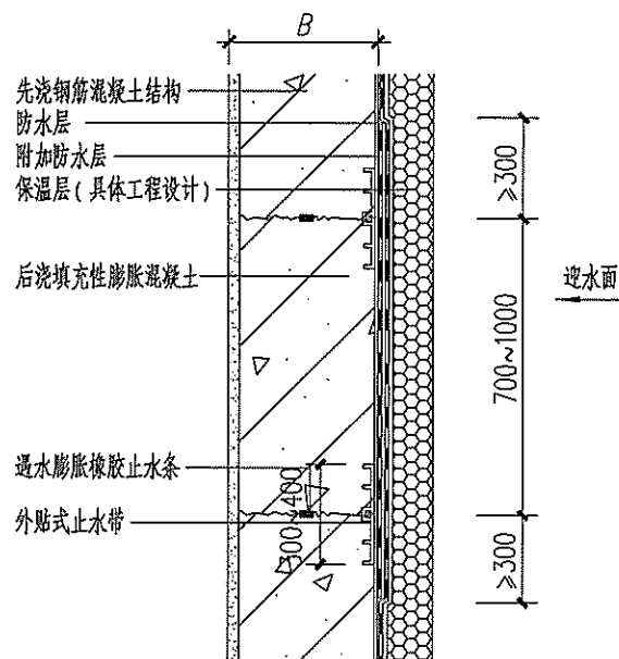
1 外墙后浇带防水构造
