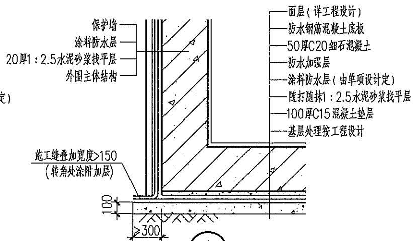
④ 接槎构造
