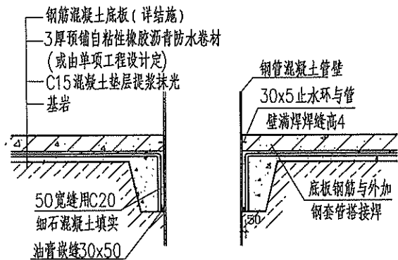
① 钢管混凝土柱与底板连接防水大样
