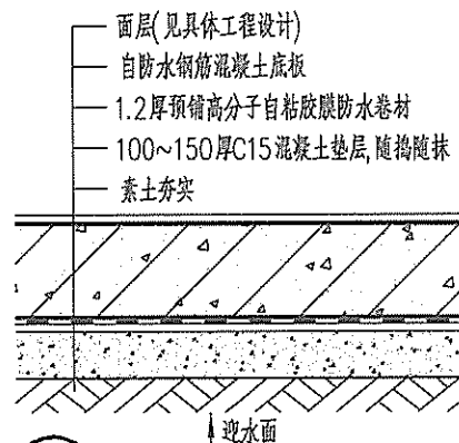
1 地下室底板防水构造
