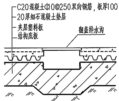
⑦ 封闭排水沟
