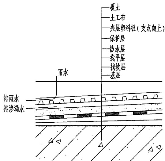
基本构造
