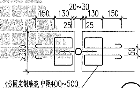
止水带详图
