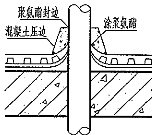
⑤ 穿顶板管道节点
