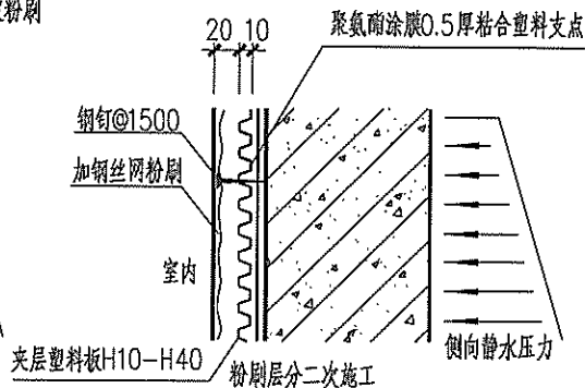
② 侧墙内防水
