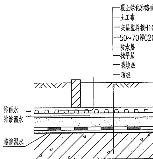
① 顶板防排组合构造
