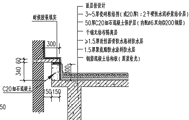
② 地下室顶板与建筑墙体变形缝大样
