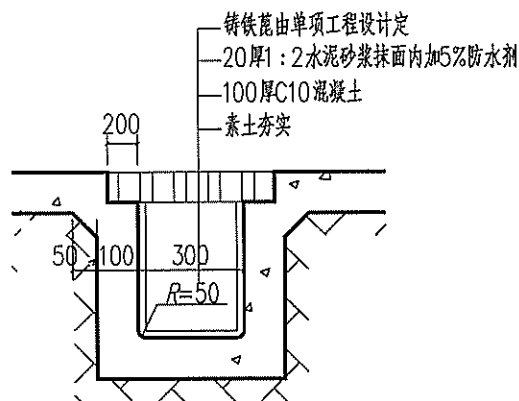
② 排水沟防水大样
