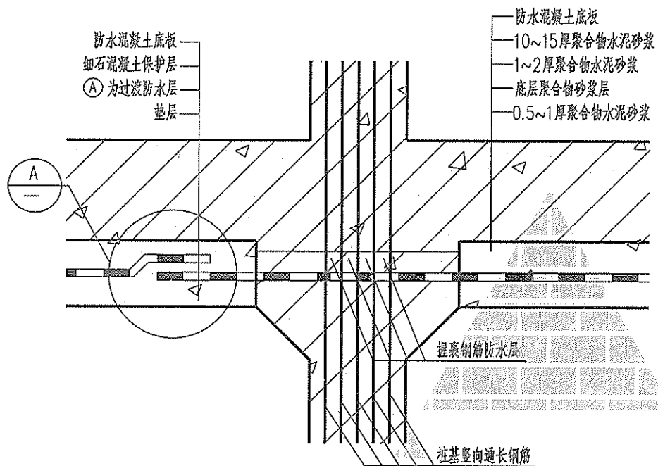
桩基防水构造示意图
