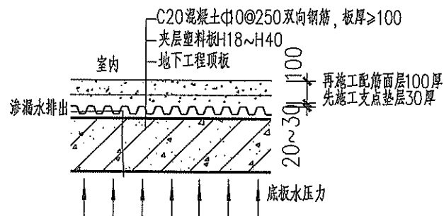
③ 内防水
