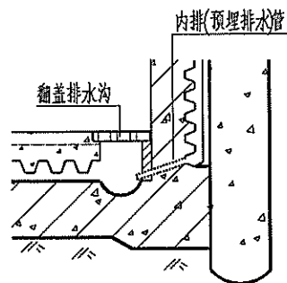
① 底板与外墙排水转角
