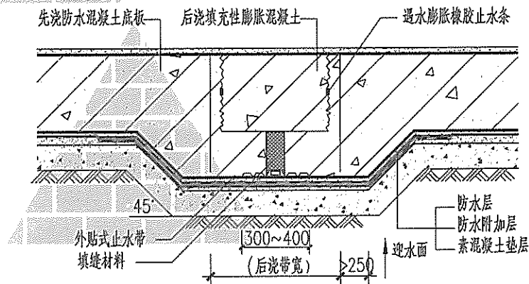
④ 底板后浇带防水构造
