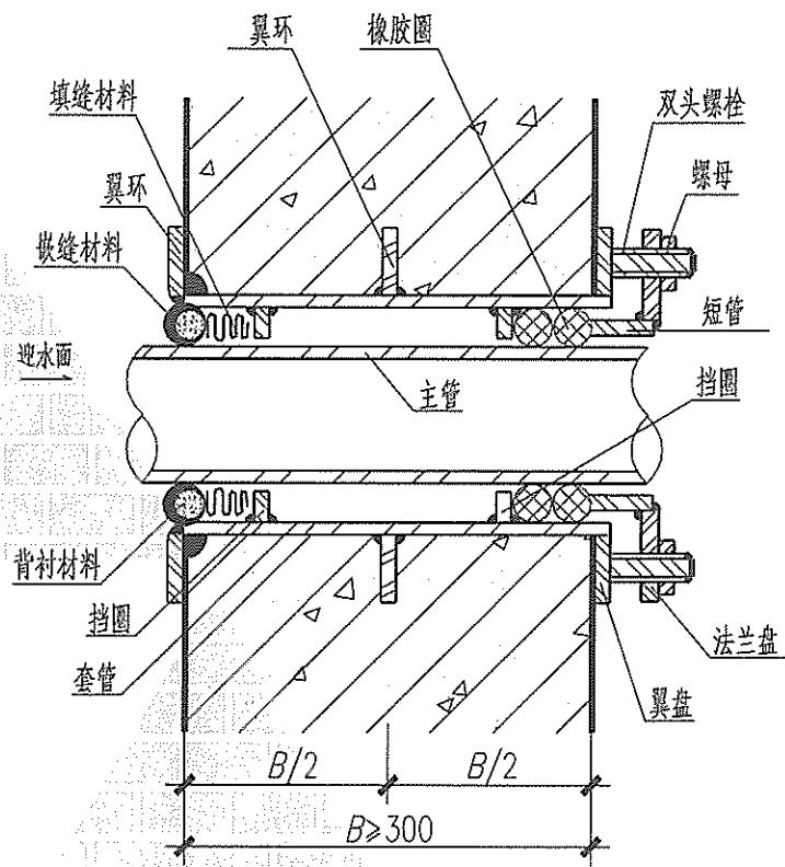
② 套管式穿墙管防水构造
