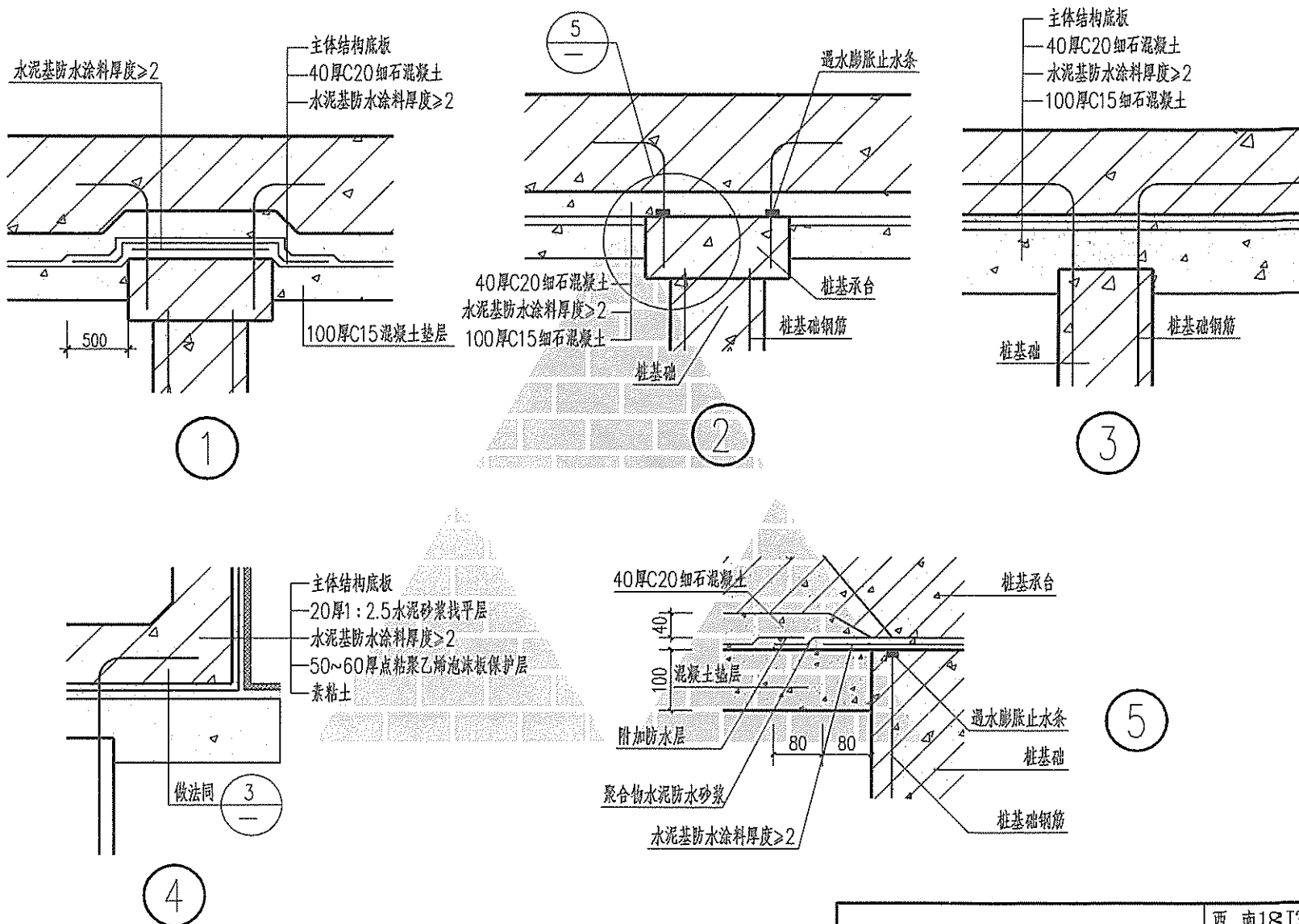
桩基防水构造(二)
