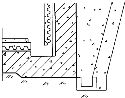
⑤ 底板与内墙排水转角
