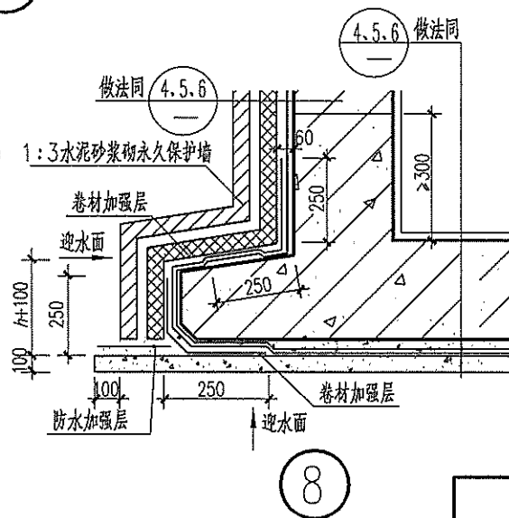
卷材防水层转角构造
