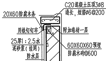
⑥ 采光井外墙压顶(二)
