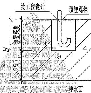
⑤ 预埋螺栓
