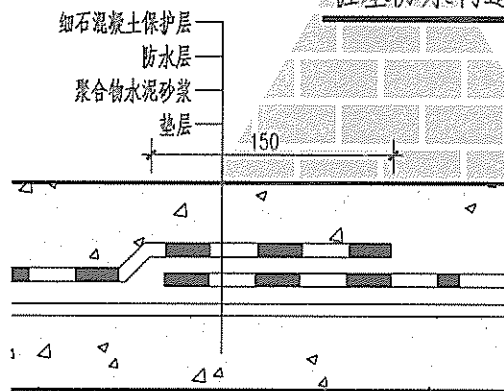
桩基防水构造示意图
