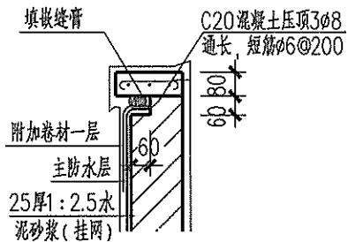
⑤ 采光井外墙压顶(一)
