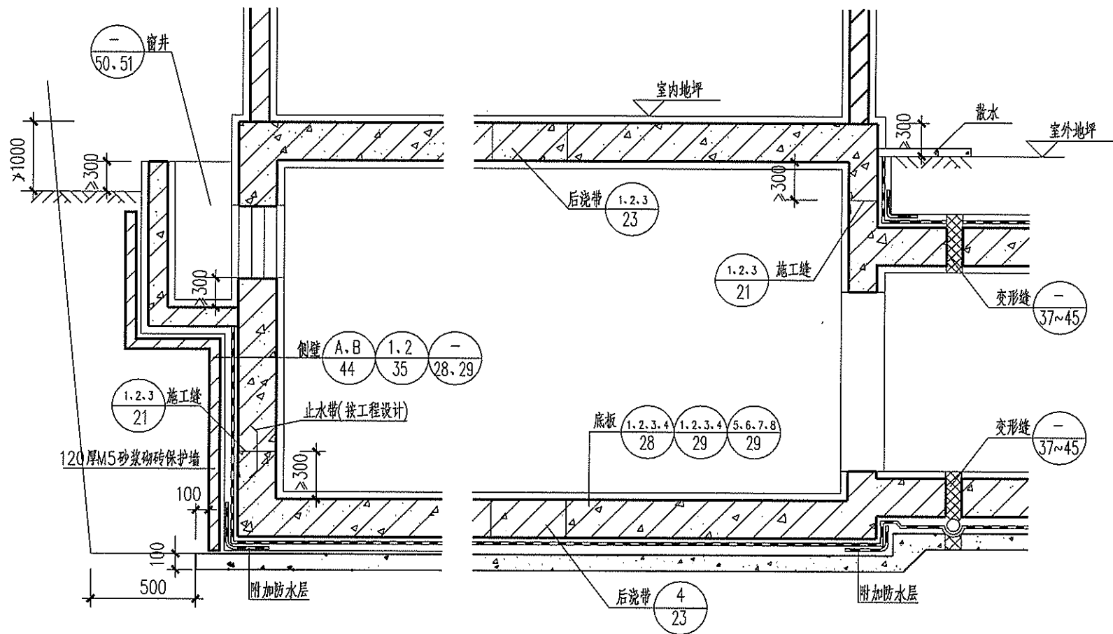
地下工程防水索引图(二)
