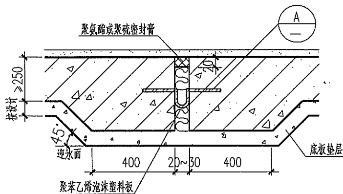
1 立墙、底板<一> 二~四级防水
