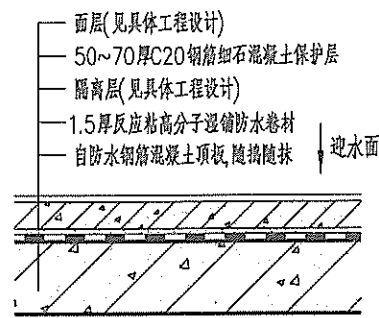
3 地下室顶板防水构造
