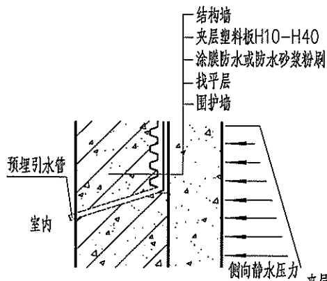
① 侧墙外防水
