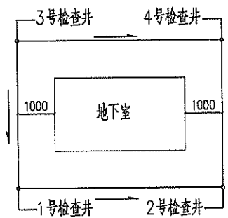
盲沟平面布置示意图
