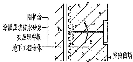
① 外墙变形缝节点
