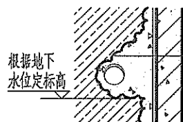
1 地下室侧墙外排水构造节点
