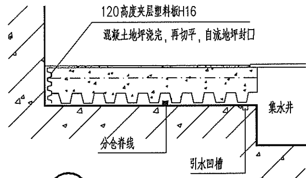
⑤ 整体剖面图
