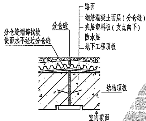
③ 顶板面层变形缝节点一
