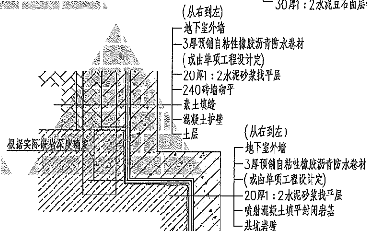
③ 地下室侧墙外防水构造节点
