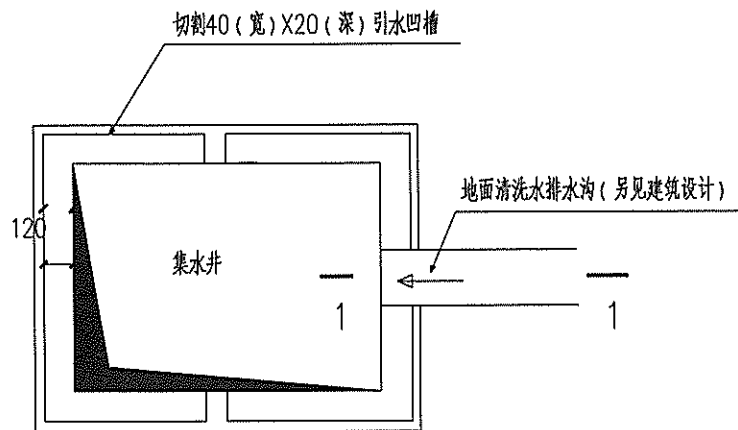
① 集水井平面水源分流图
