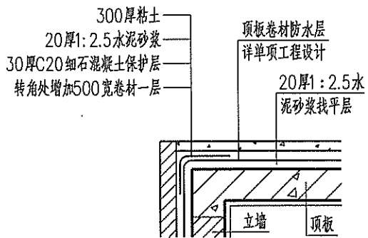
4 顶板卷材防水做法
