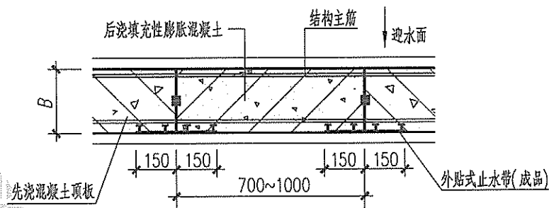
② 顶板后浇带防水构造(二)
