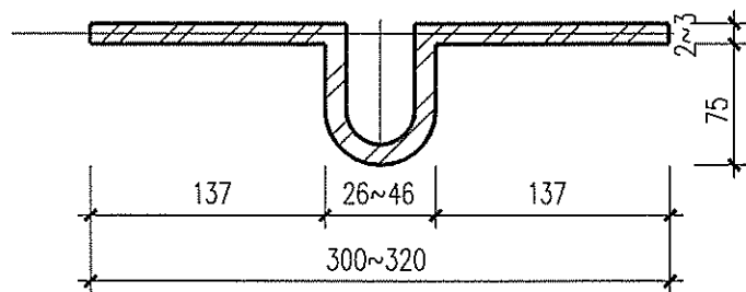
A 金属止水带
