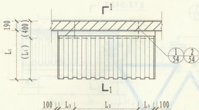
平面图
