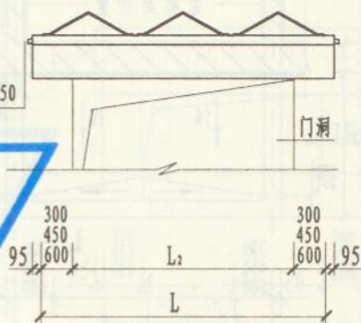
立面图
