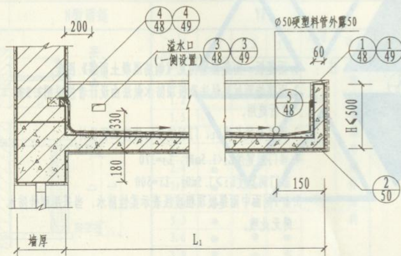
1-1剖面图
