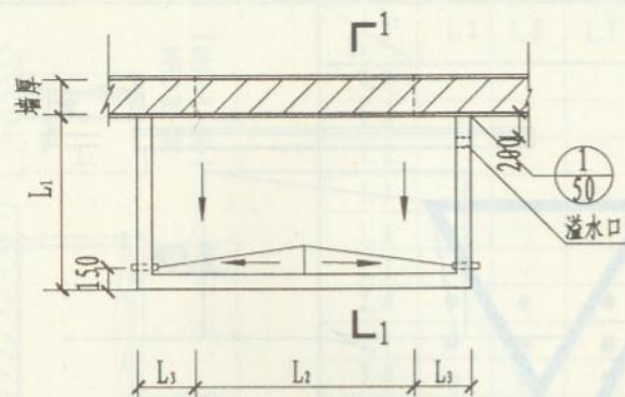
平面图
