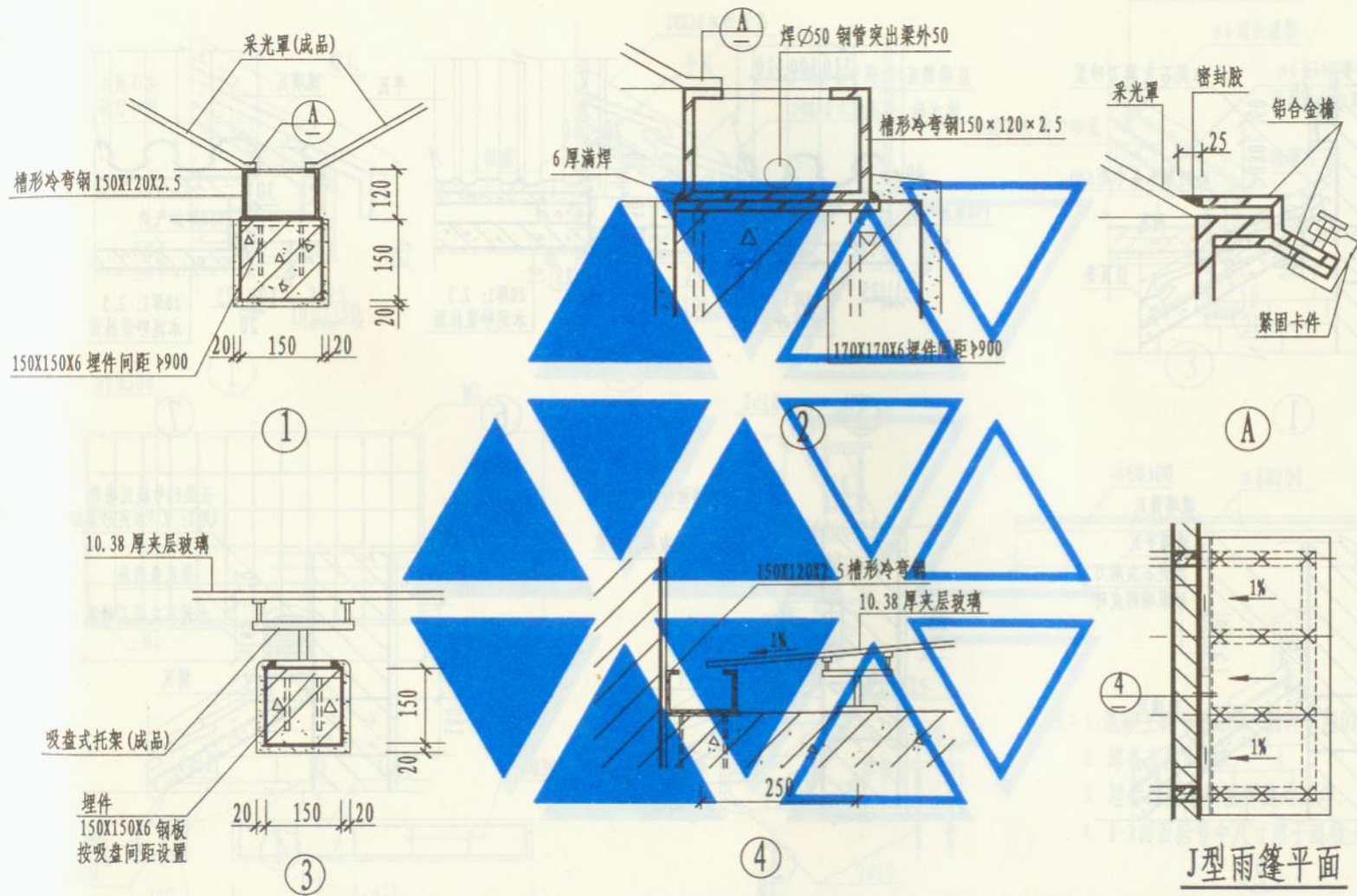
雨篷建筑详图(四)
