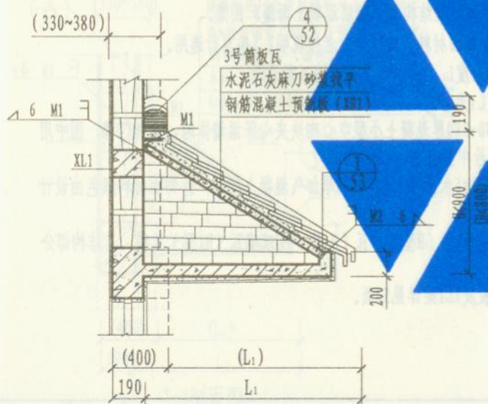
1-1剖面图
