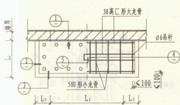
吊顶平面(I)
