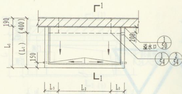
平面图
