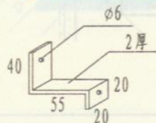
扁钢卡件
