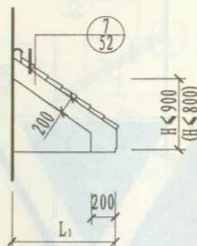
侧立面图
