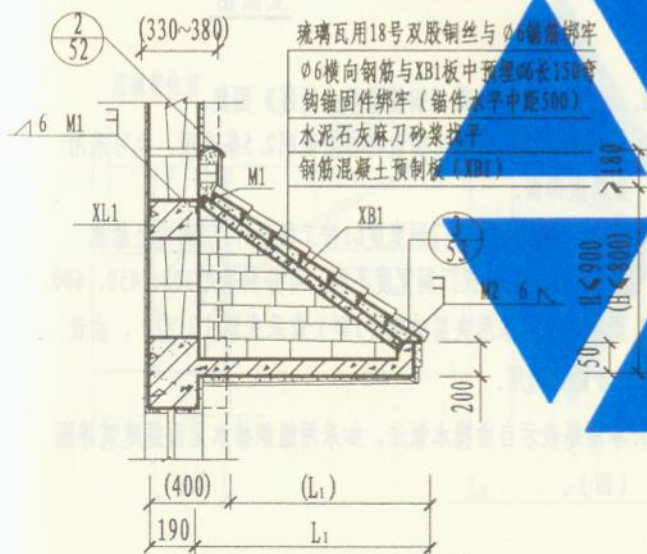
1-1剖面图
