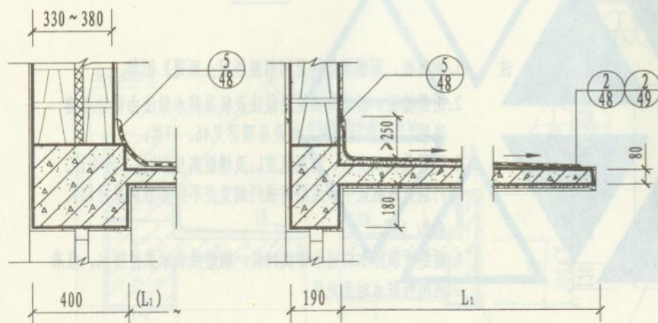
1-1剖面图
