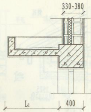
1-1剖面图
