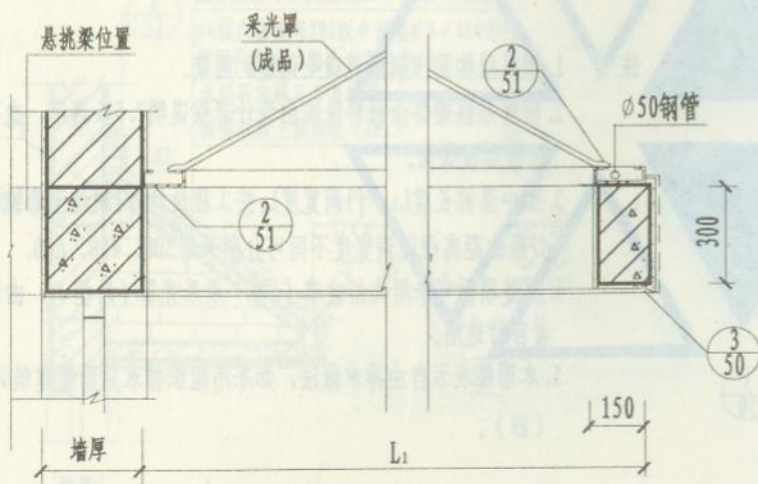
1-1剖面图
