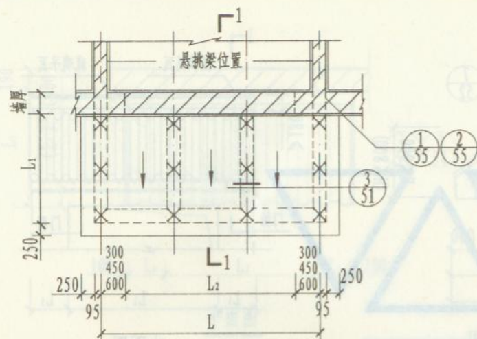
平面图
