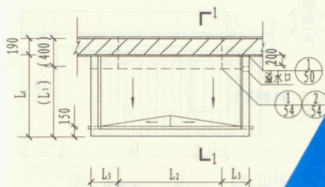
平面图
