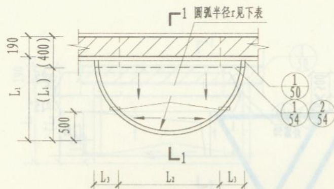
平面图
