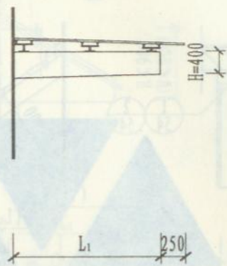
侧立面图
