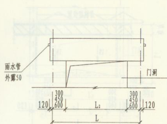
立面图
