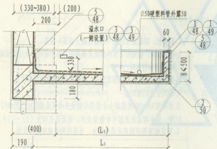
1-1剖面图
