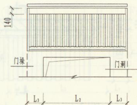
立面图
