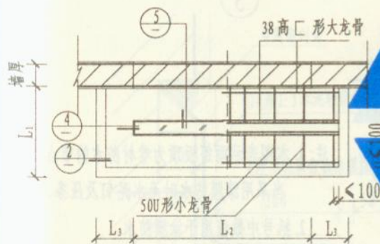
吊顶平面(II)
