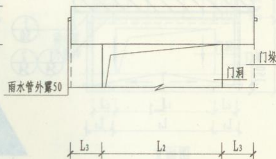
立面图
