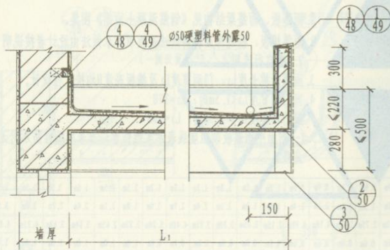
1-1剖面图
