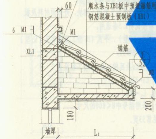
1-1剖面图
