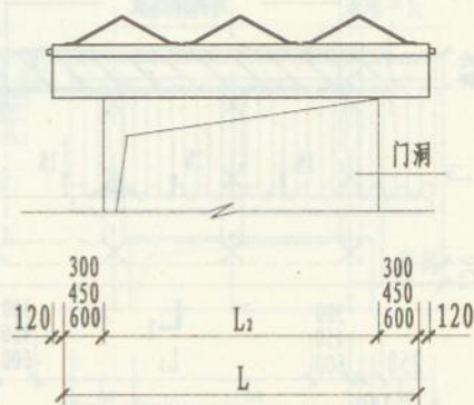
立面图
