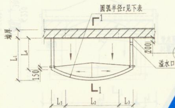
平面图
