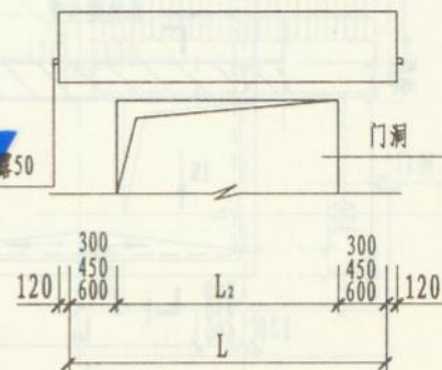
立面图
