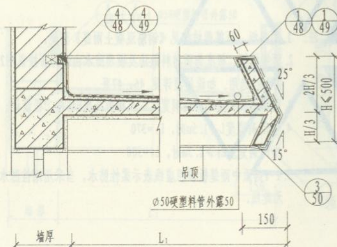
1-1剖面图
