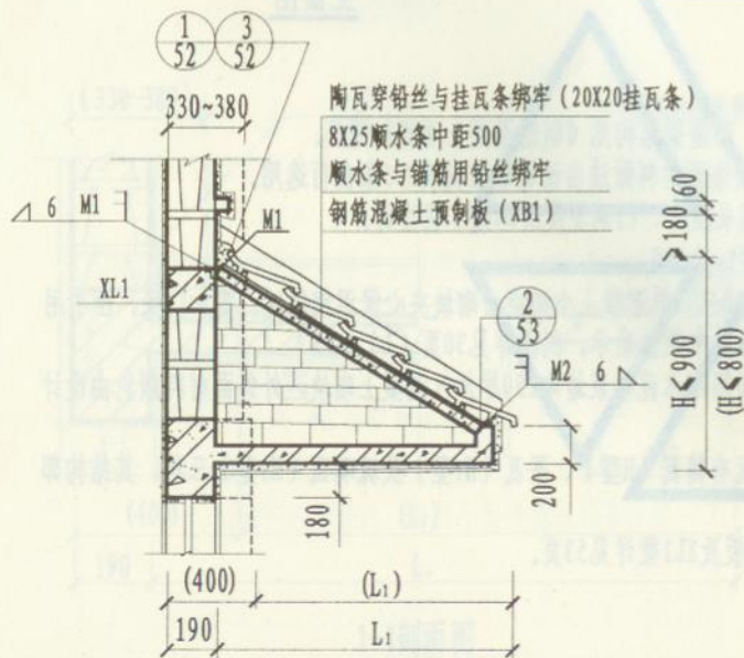
1-1剖面图
