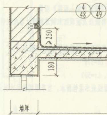
1-1剖面图
