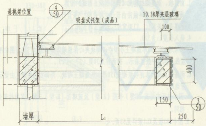
1-1剖面图
