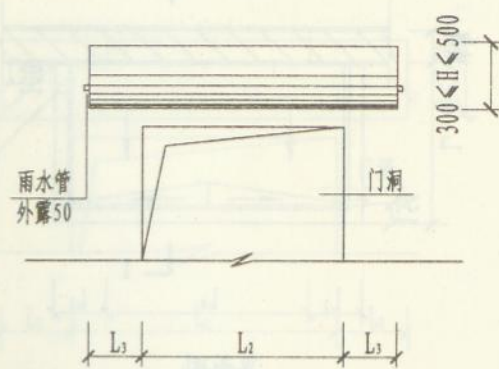
立面图
