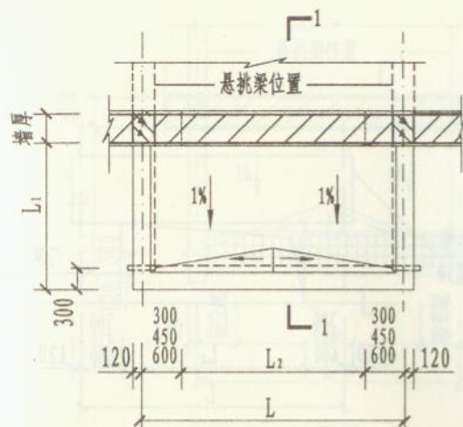
平面图
