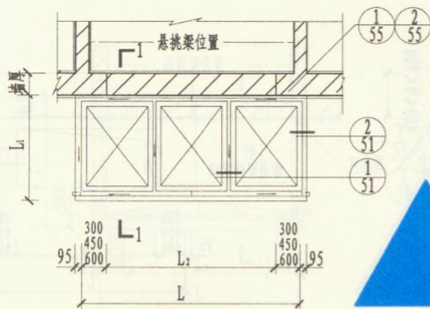
平面图
