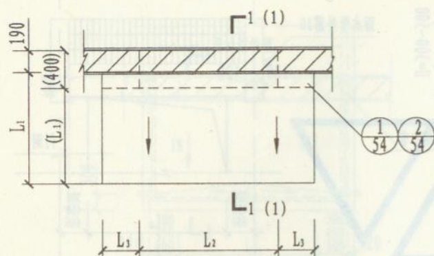
平面图
