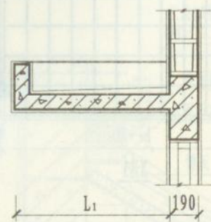
2-2剖面图
