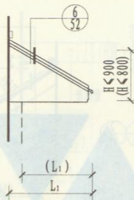
侧立面图
