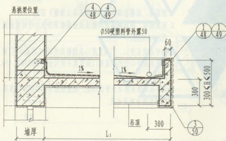
1-1剖面图
