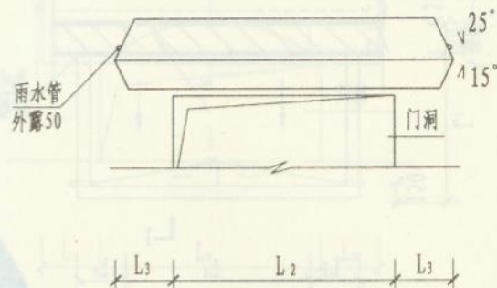
立面图
