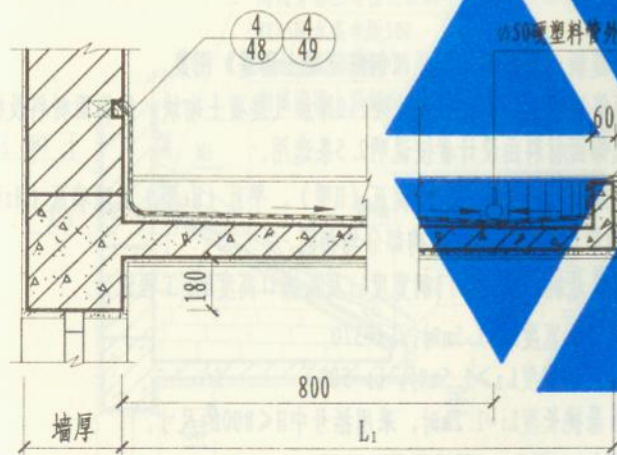
1-1剖面图
