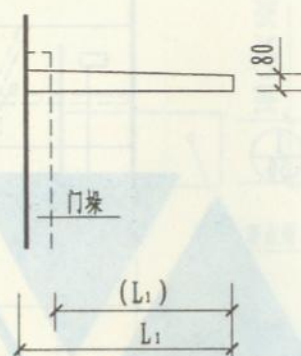
侧立面图
