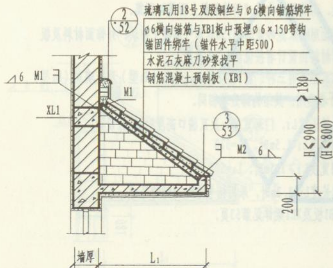
1-1剖面图
