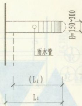
侧立面图
