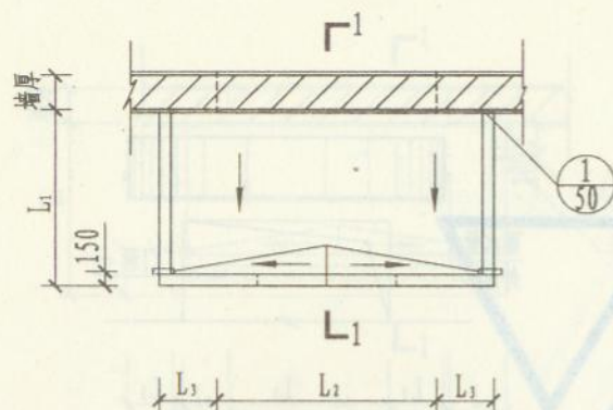
平面图
