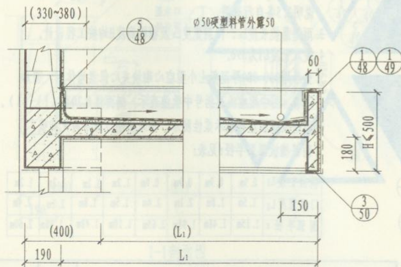
1-1剖面图
