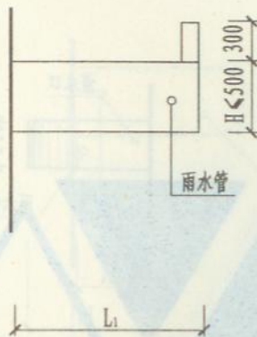
侧立面图
