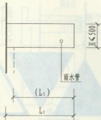
侧立面图
