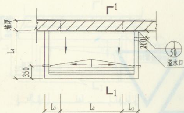
平面图
