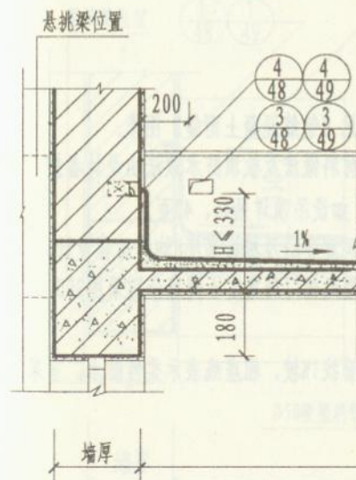
1-1剖面图
