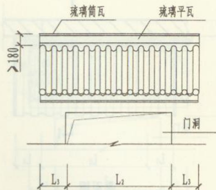
立面图
