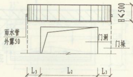
立面图
