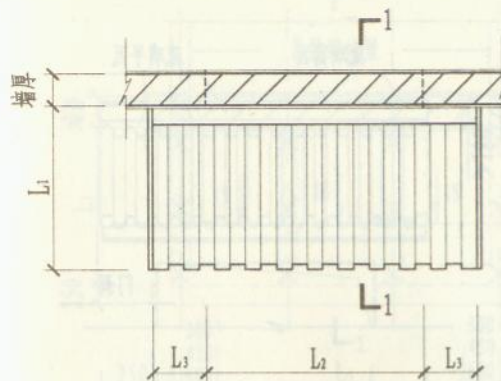
平面图
