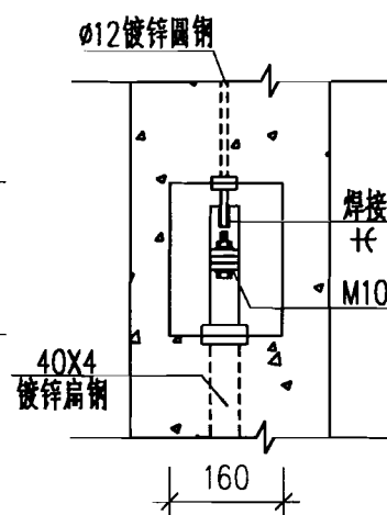
I-I 剖面图
