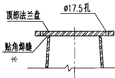
① 顶部法兰盘与钢管杆焊接大样
