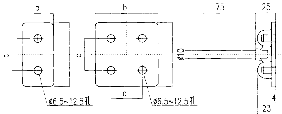
接地端子板外形图
