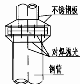
节点处外包不锈钢板大样图
