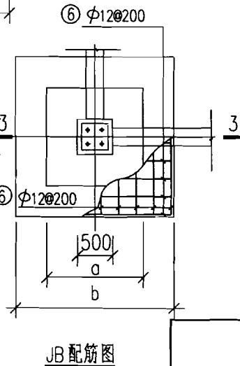
独立基础JB平面及大样图
