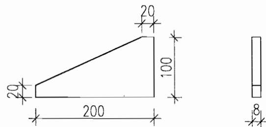
2号零件
