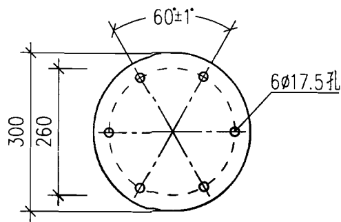
顶部法兰盘
