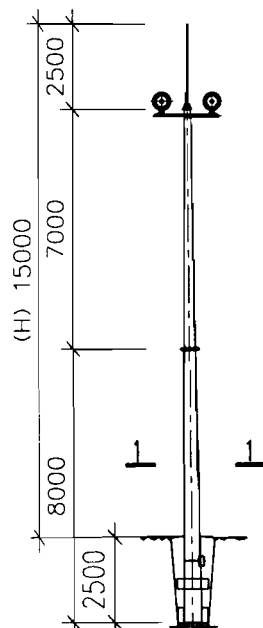
15m 针塔
