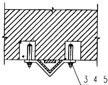
引下线保护(I)
