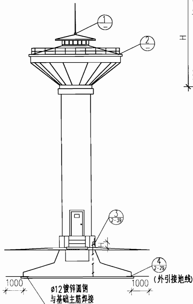
水塔避雷做法
