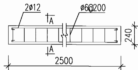
梁钢筋图
