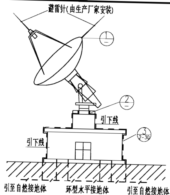
卫星地面站防雷接地示意图
