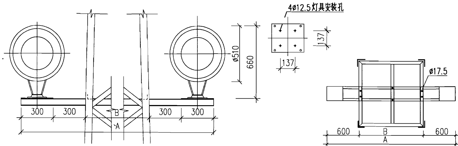
DLTG3型投光灯安装示意
