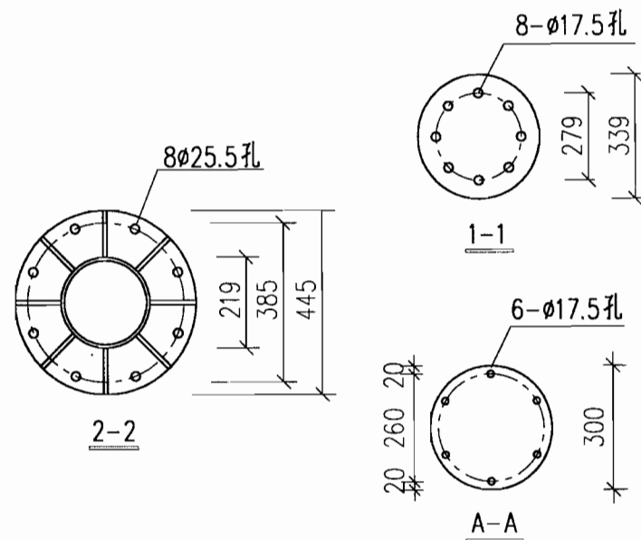
节点处外包不锈钢板大样图
