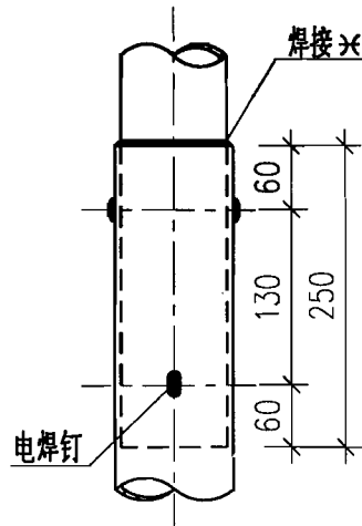
节点 IV
