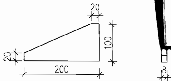
2号零件
