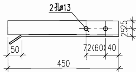
2号零件
