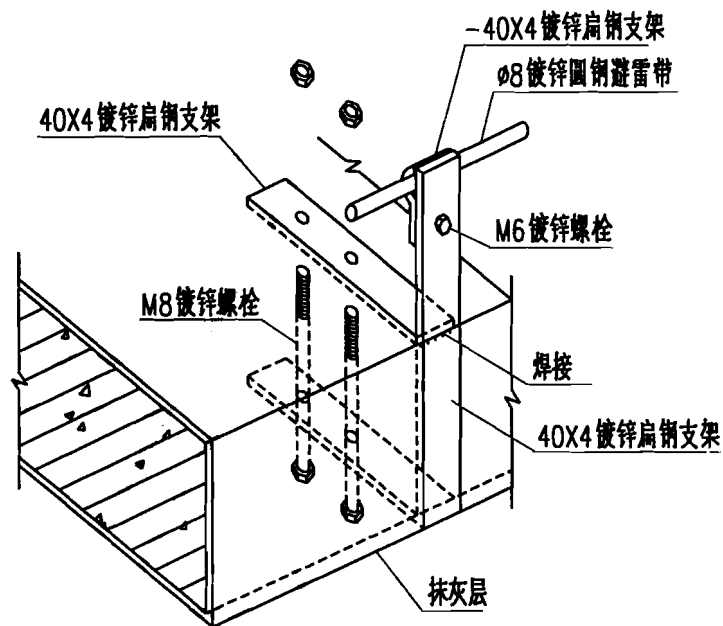
支架透视图
