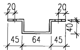
2号零件(II)
