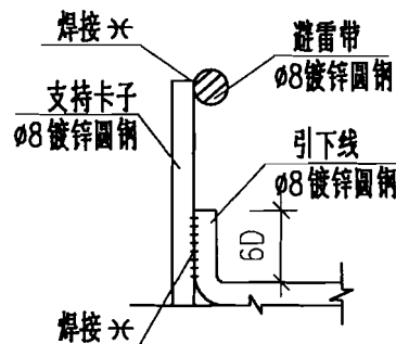
圆钢引下线连接
