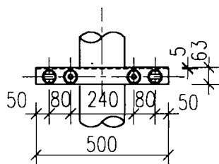
1-1 剖面
