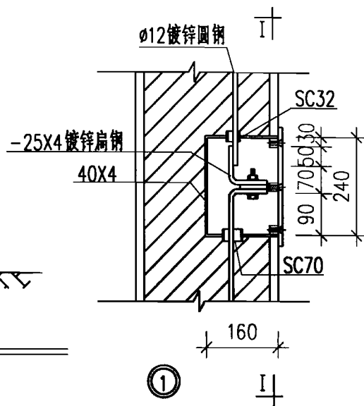
暗装断接卡子做法(一)
