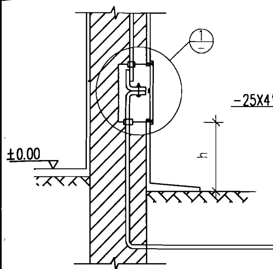
暗装断接卡子做法(一)
