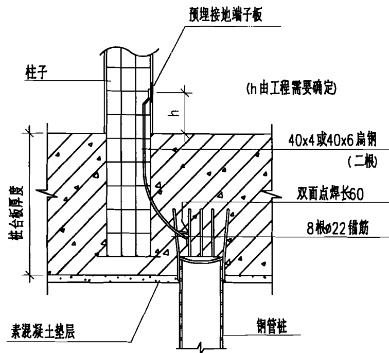
柱内扁钢与钢管桩锚筋焊接剖面图
