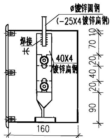
II-II 剖面图
