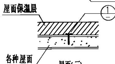
屋面(三) (暗装)
