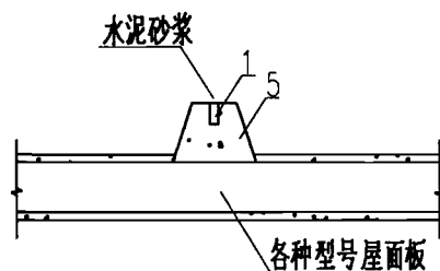
屋面(一) (明装)
