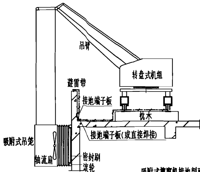
吸附式擦窗机接地剖面图
