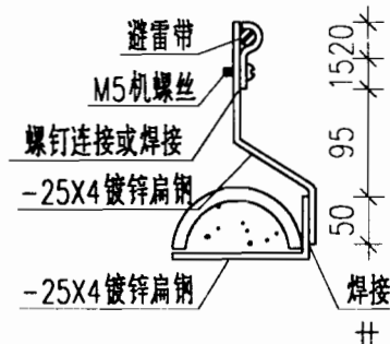
② 脊瓦上的防雷做法(二)
