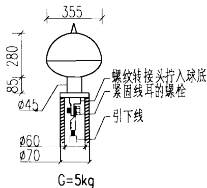
S3000针外形尺寸图
