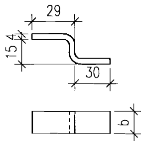
(9) S形卡子
