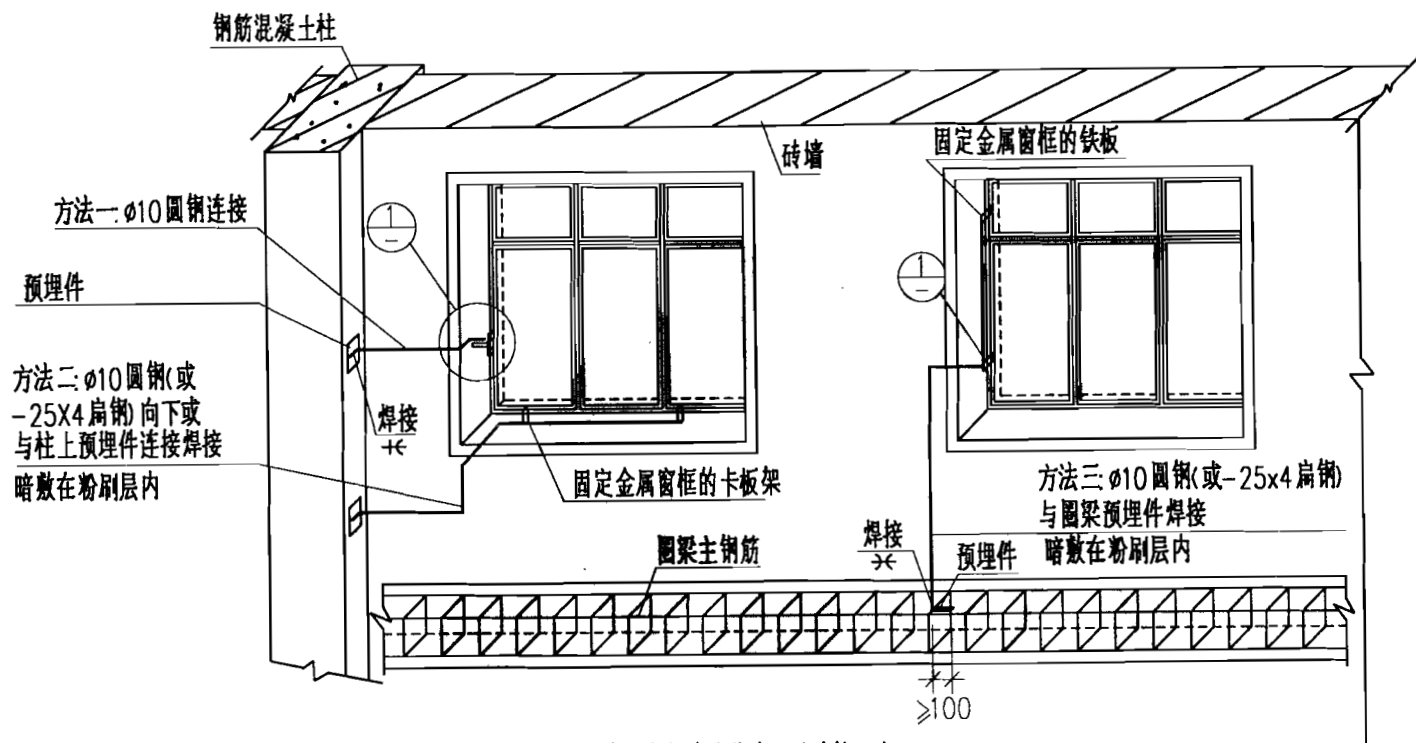
金属窗与建筑物金属体连接示意
