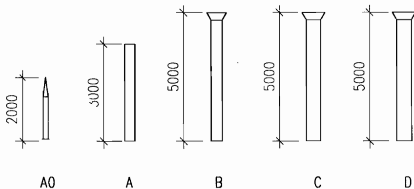
不锈钢针杆分段图
