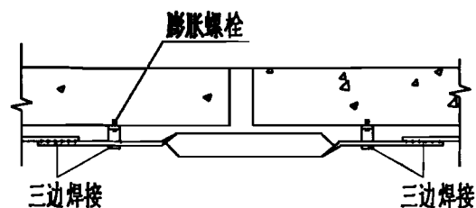
I-I剖面图
