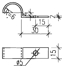
圓鋼卡子
