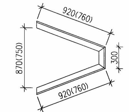
2号零件
