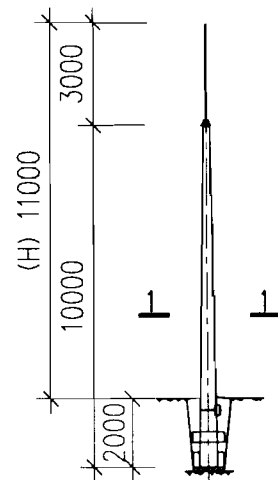
11m 针塔
