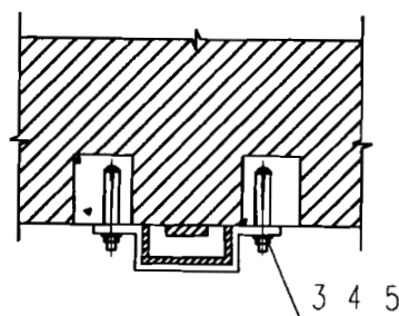
引下线保护(II)
