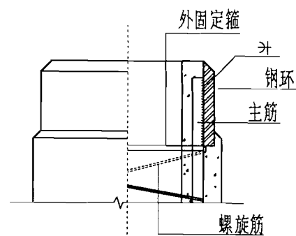
电杆顶部纵向钢筋 与钢环连接大样
