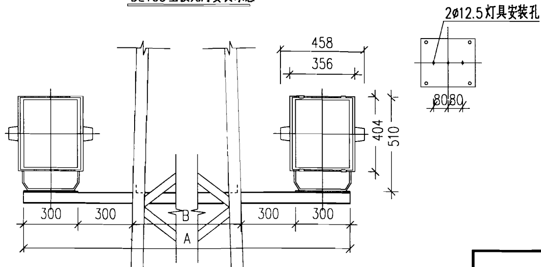
DLTG4型投光灯安装示意
