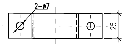
管卡 1
