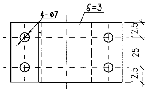
管卡 1
