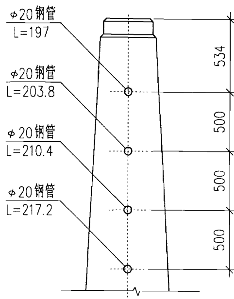
预埋钢管大样图
