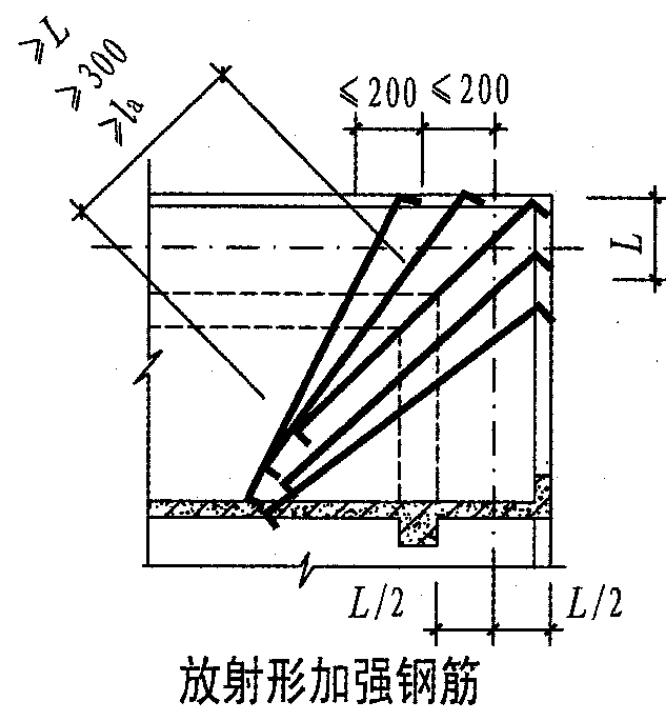
悬臂板在阳角和阴角的附加加强钢筋构造
