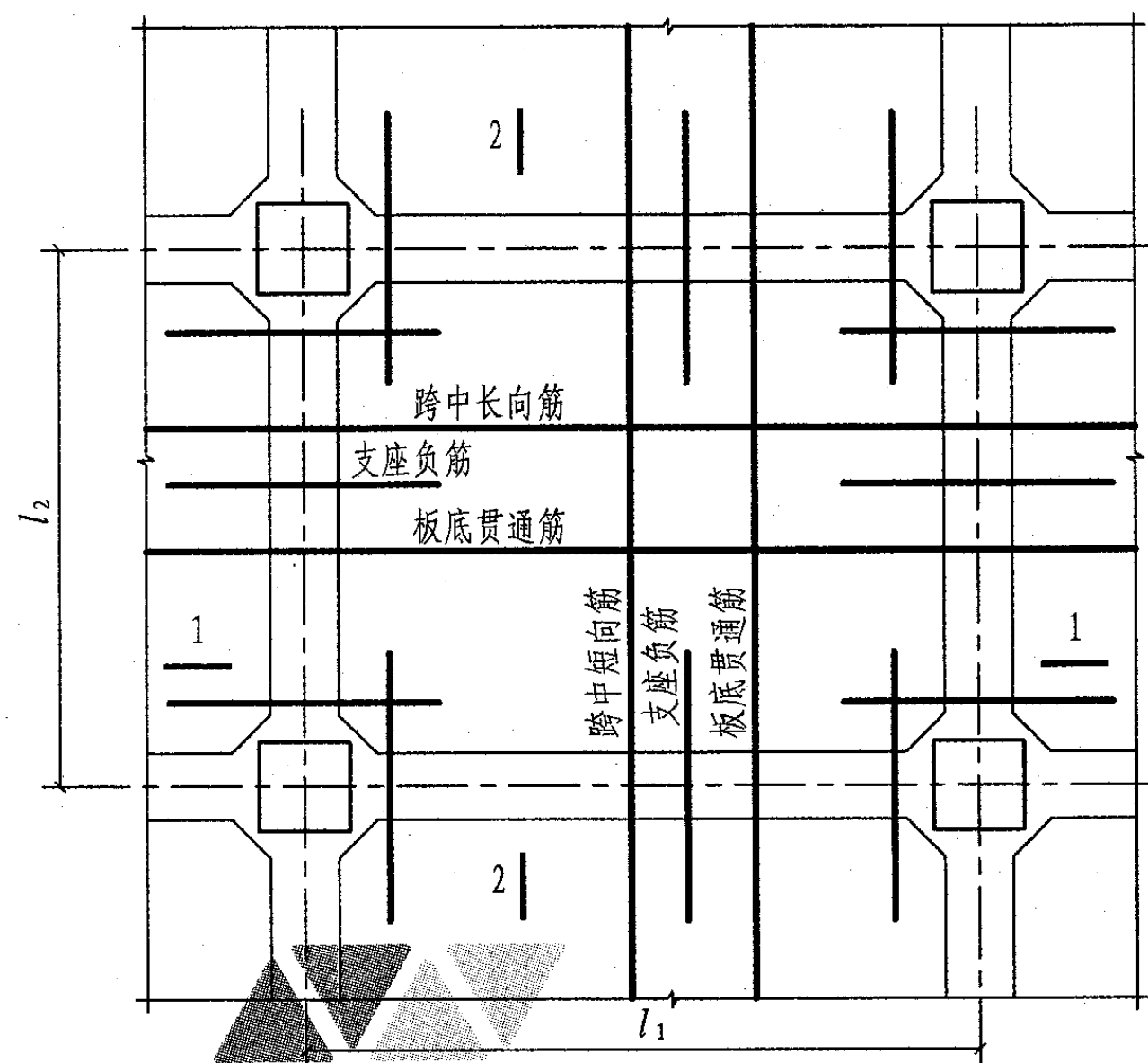
底平梁板式筏形基础配筋构造
