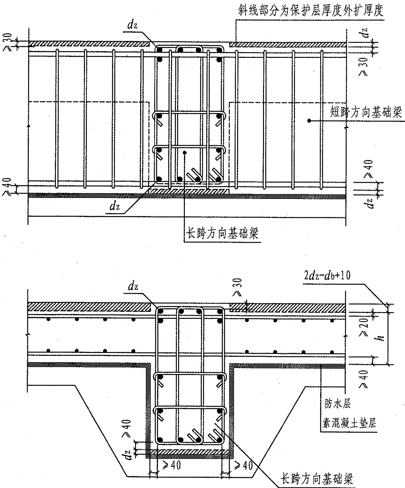
顶平筏形基础钢筋位置关系 (一)
