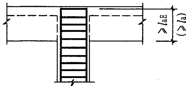
中部小墙肢纵筋直锚做法
