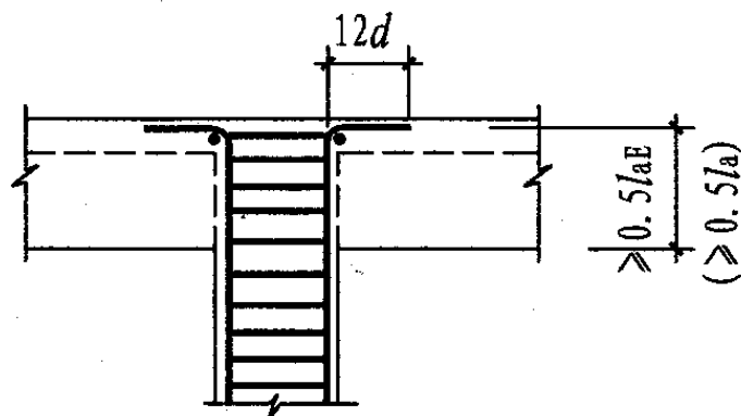
中部小墙肢纵筋弯锚做法
