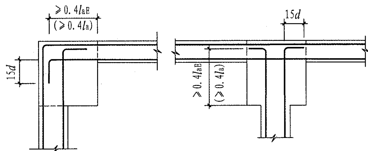
剪力墙一侧与边框柱平 剪力墙水平分布钢筋在边框柱中锚固
