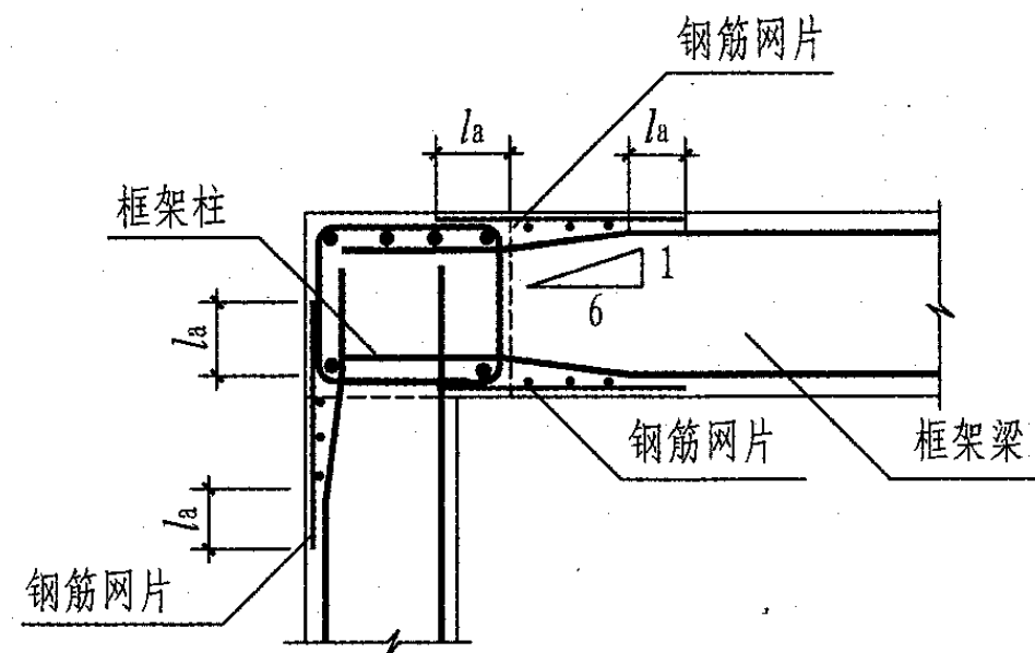
框架柱与框架梁宽度相同
