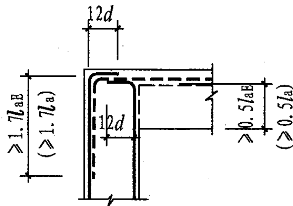
边角小墙肢在框架柱中连接做法
