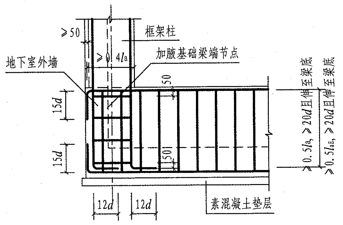
梁板式基础梁端部纵筋与柱纵筋锚固构造（一）
