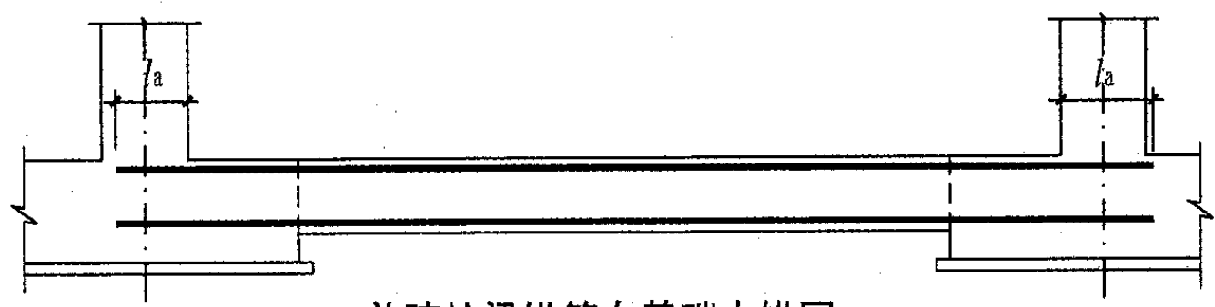
单跨拉梁纵筋在基础内锚固
