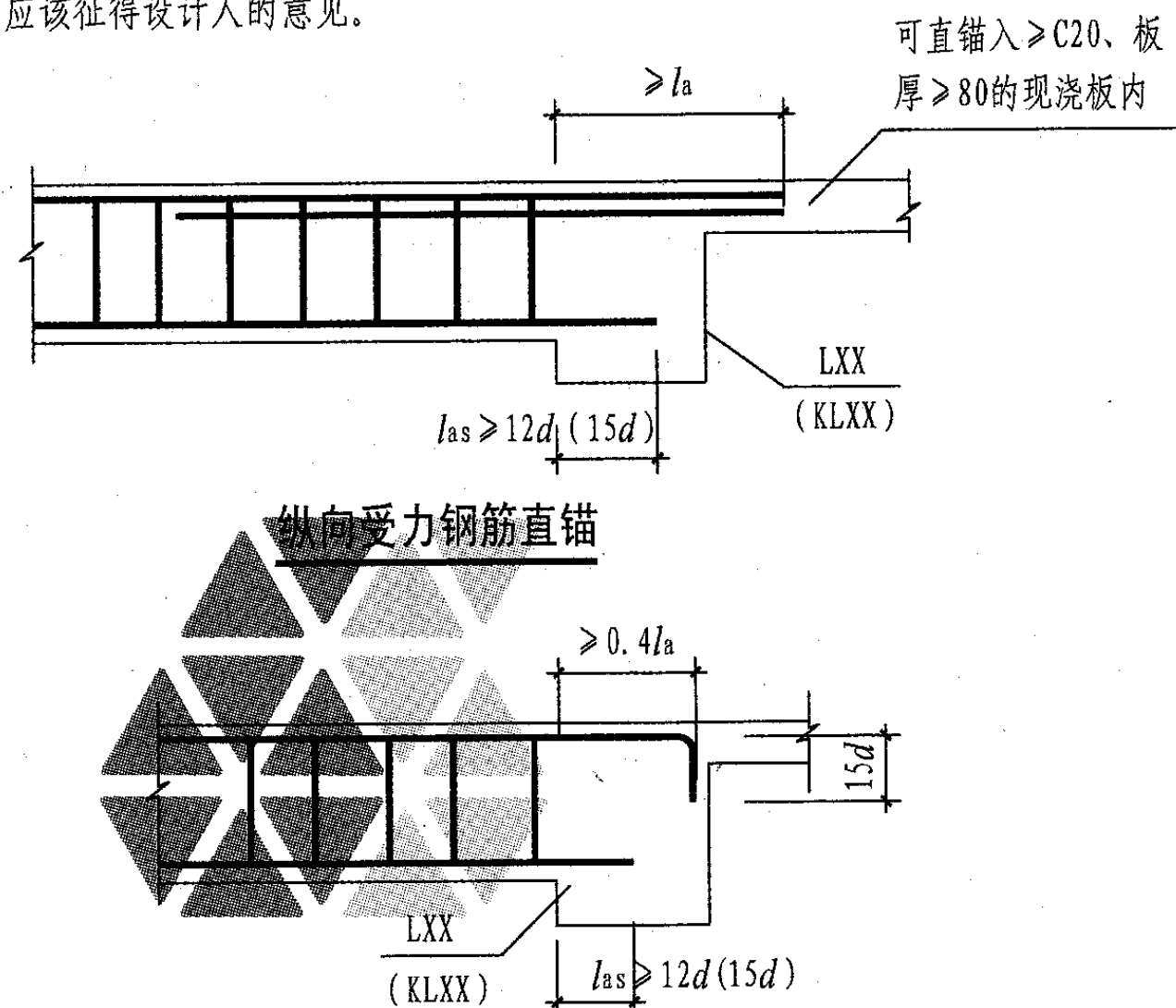
上部纵向钢筋锚固
