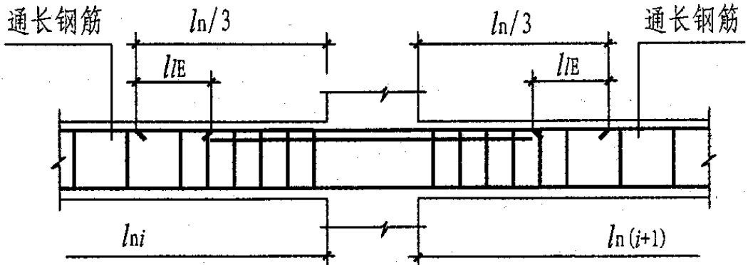
上部通长纵向钢筋搭接
