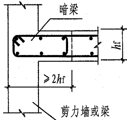
楼板边缘部位边梁
