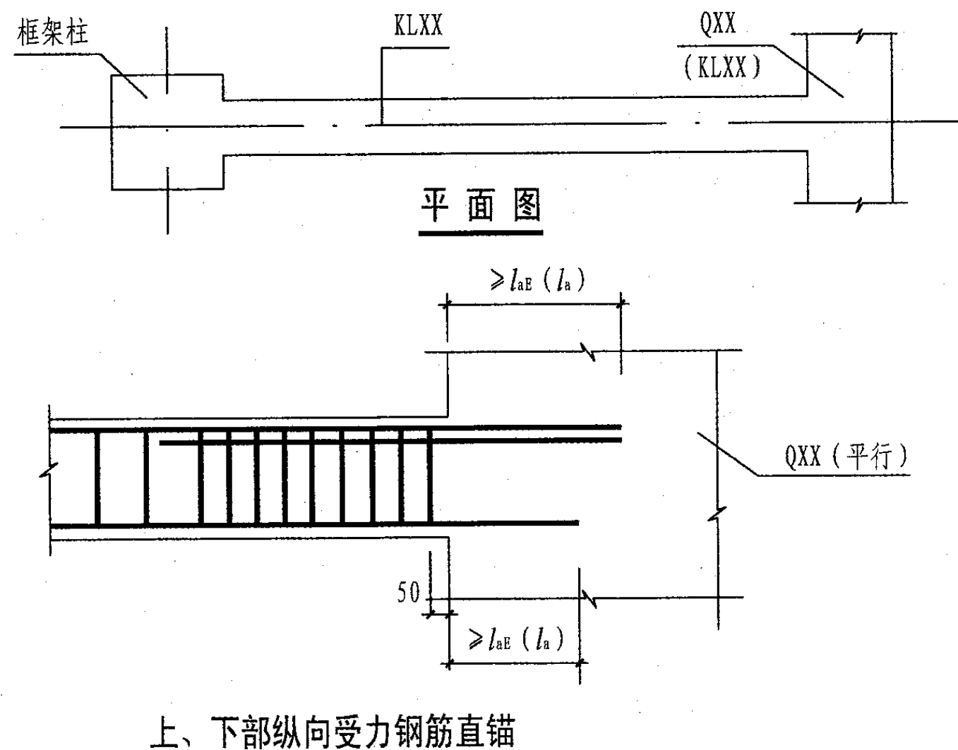
梁有一端支座为非框架柱时的配筋构造
