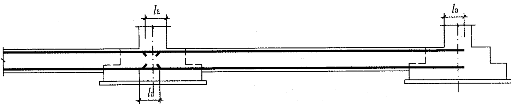
连续拉梁纵筋在基础内锚固
