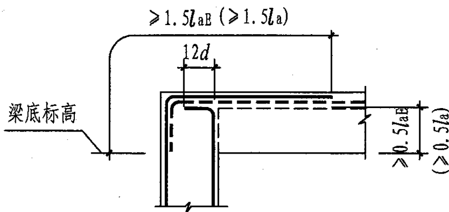
边角小墙肢在框架梁中连接做法
