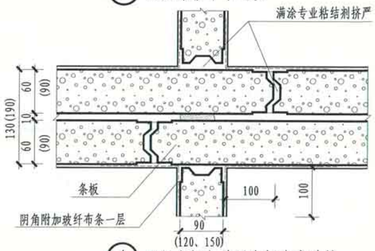
② 双层条板十字连接
