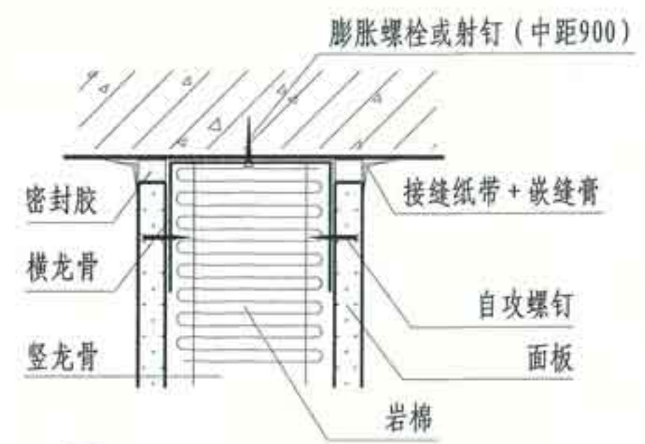
③ 单层板、有隔音、无密封胶条
