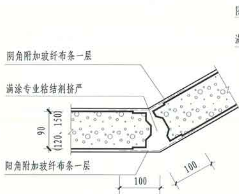
④ 条板任意角连接
