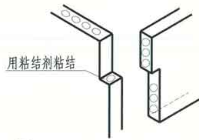
④ 转角轻隔墙与门上板搭接
