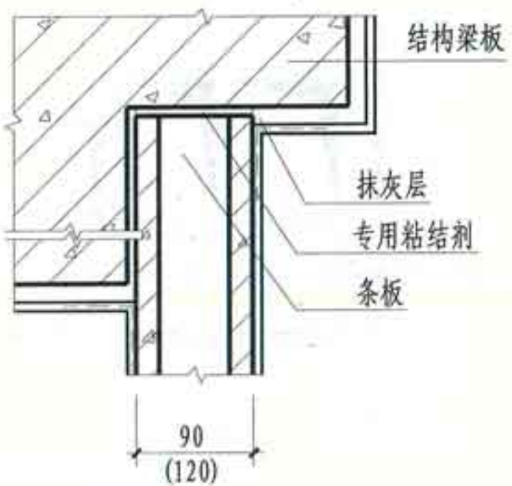
④ 条板与梁侧连接
