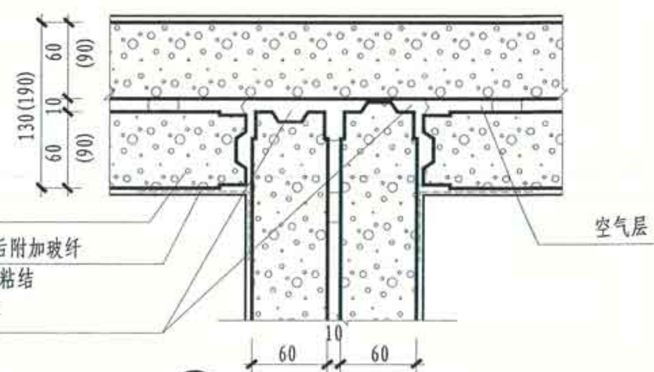
⑤ 双层条板丁字连接
