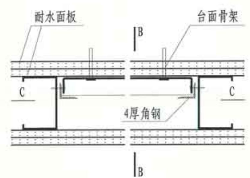
② 台面支架平面
