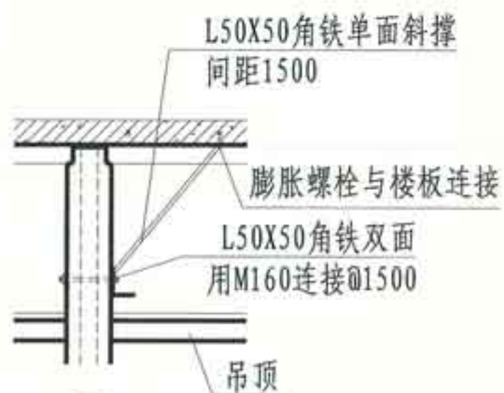
⑤ 与顶部结构层连接
