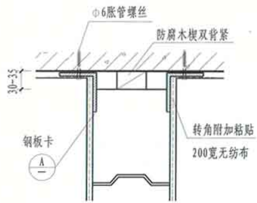
② 砌块隔墙与混凝土顶板连接
