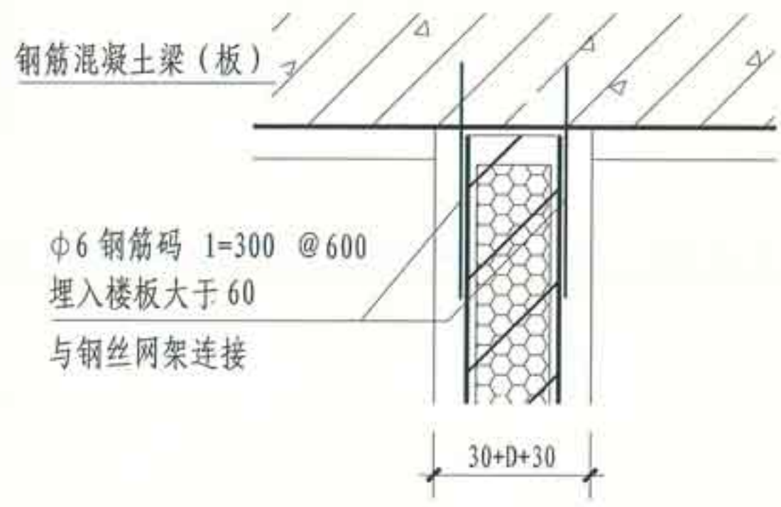
③ 板墙与楼板连接构造
