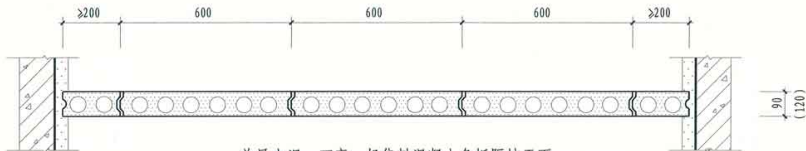
单层水泥、石膏、轻集料混凝土条板隔墙平面
