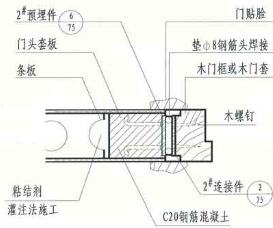
② 条板与门头套板、木门框连接
