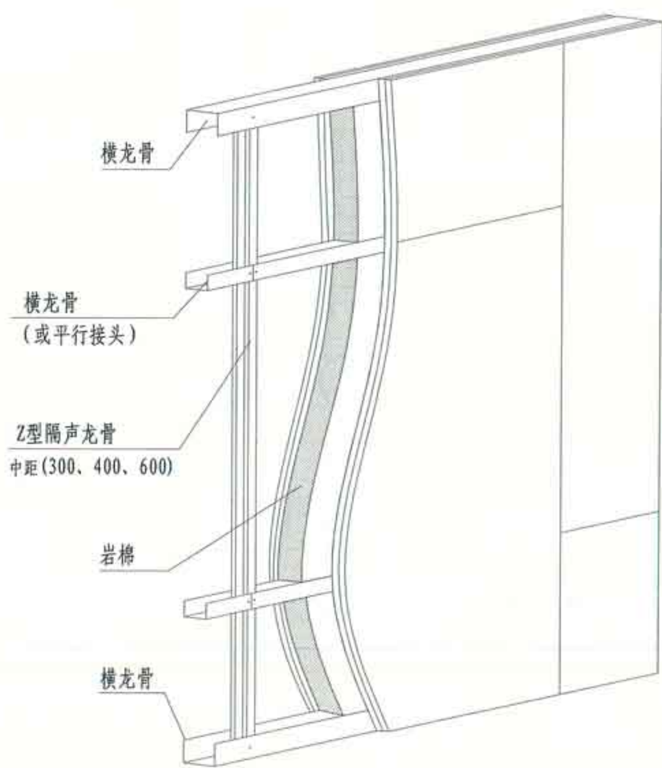
① Z型隔声龙骨体系
