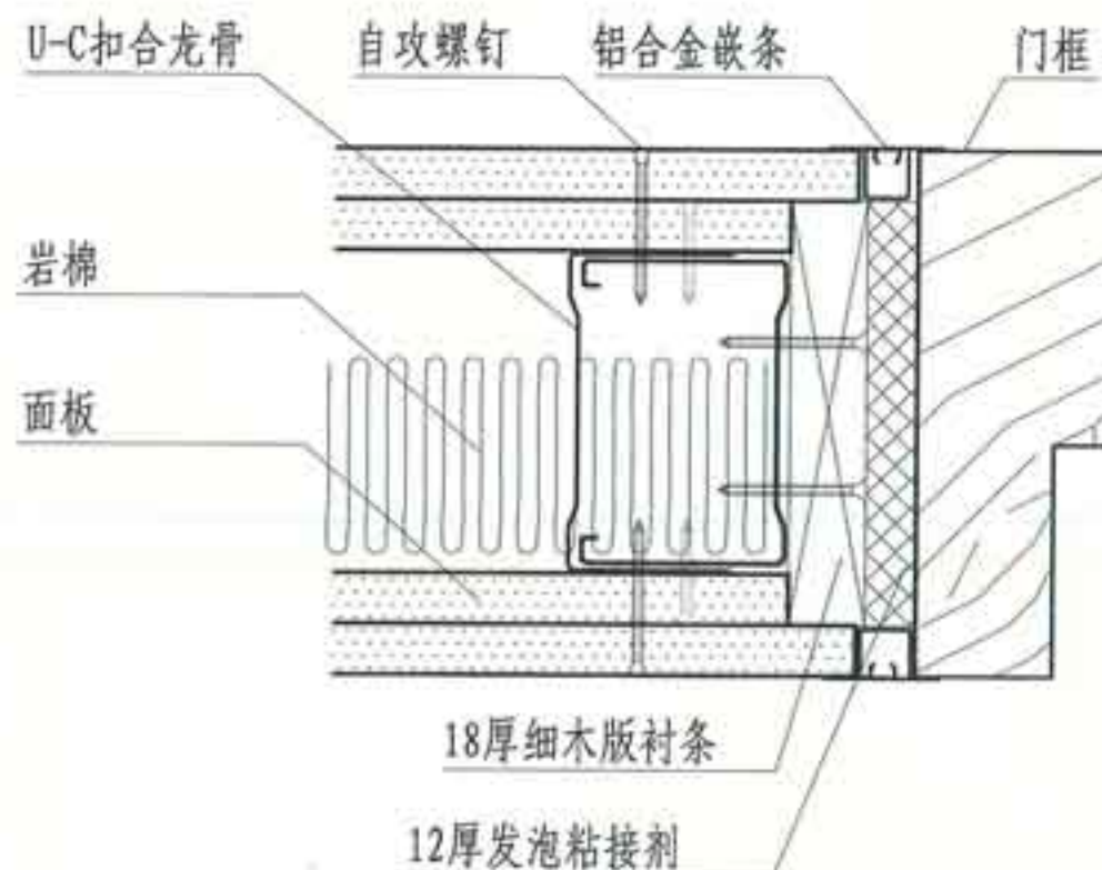
④ U-C扣合组合3
