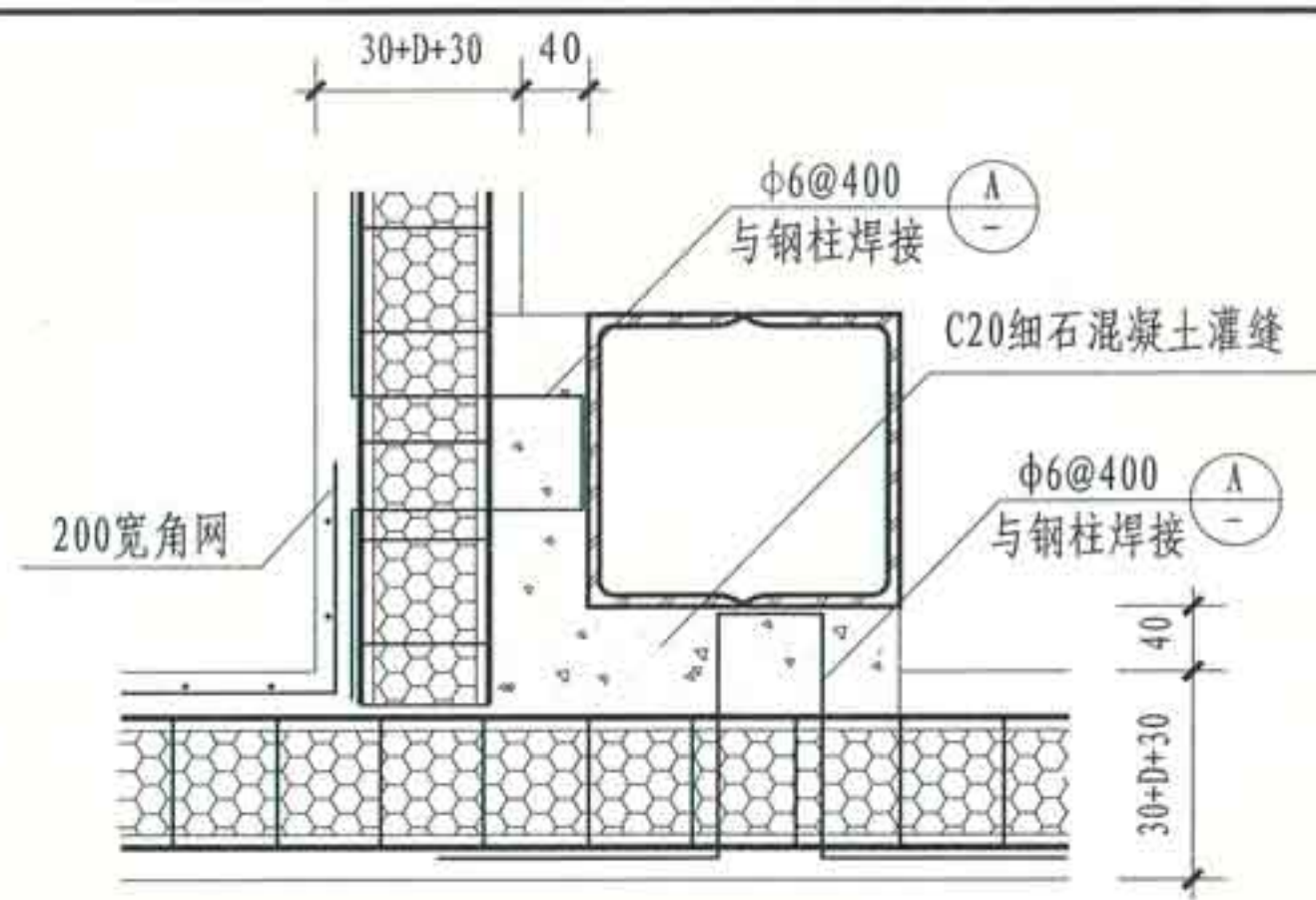
① 丁字墙连接构造(一)
