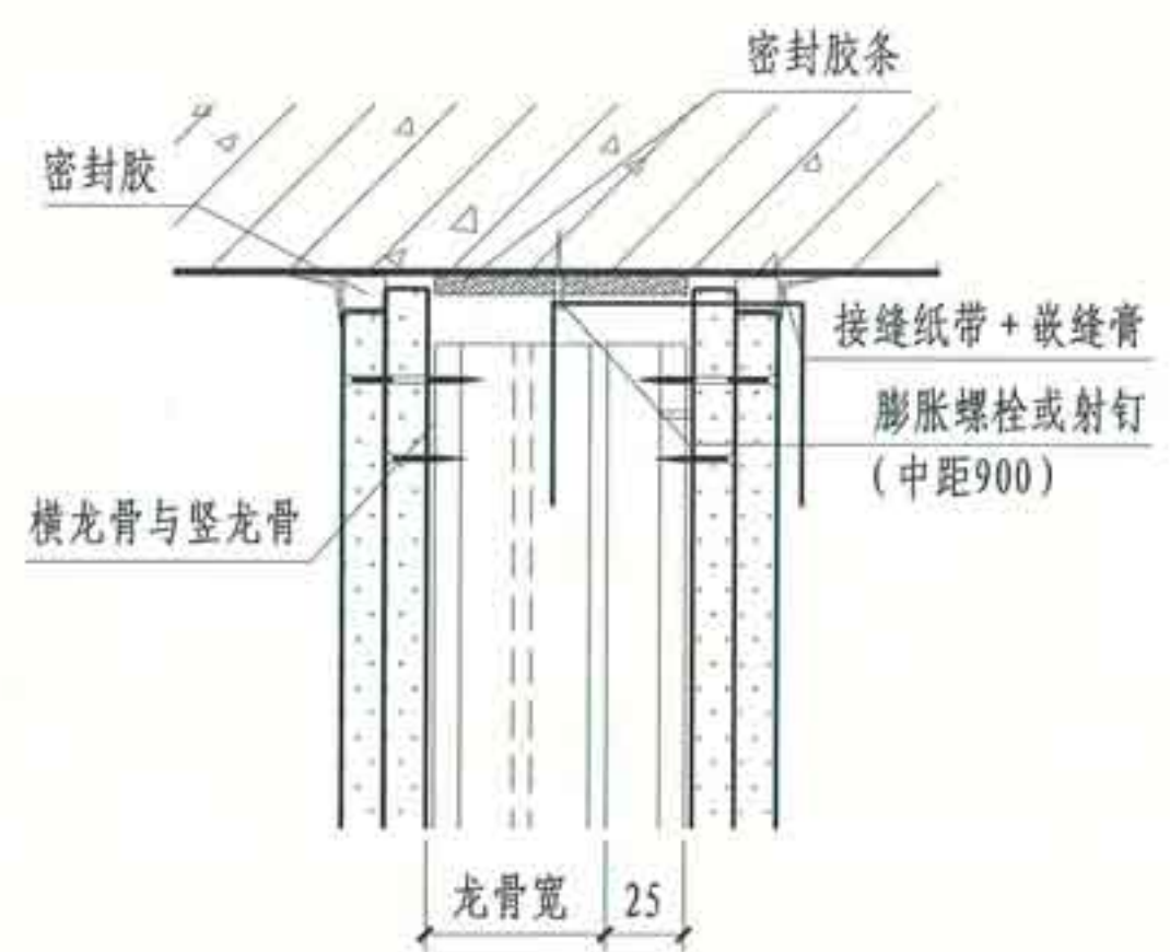
① 竖向龙骨错位排列
