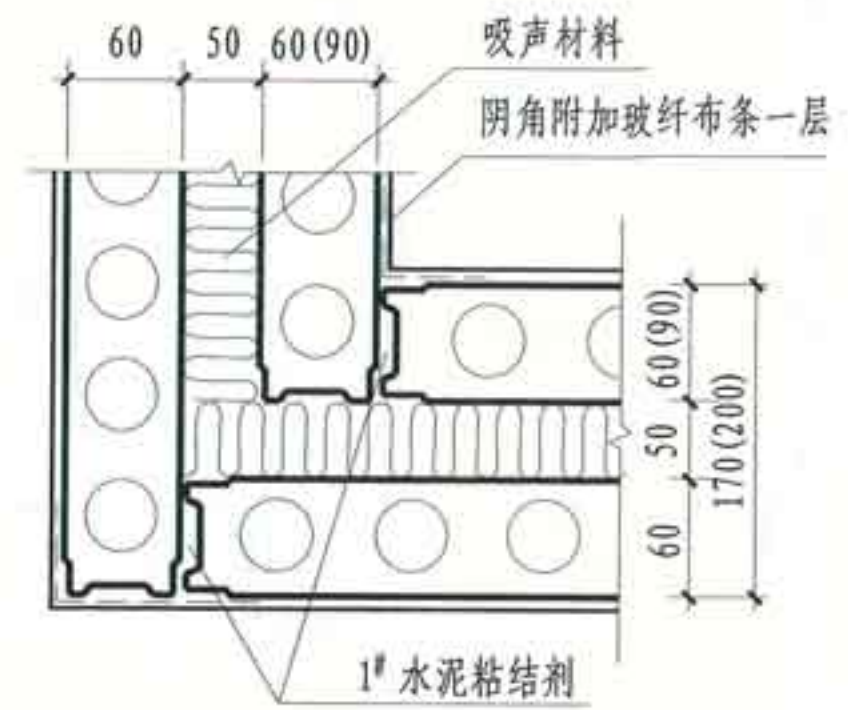
③ 条板隔声墙直角连接
