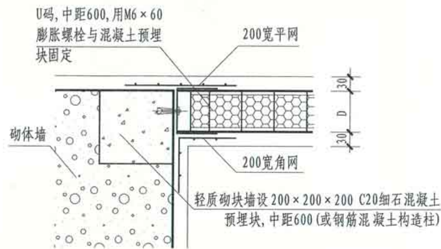
② 板墙与砌体墙连接构造 (一)
