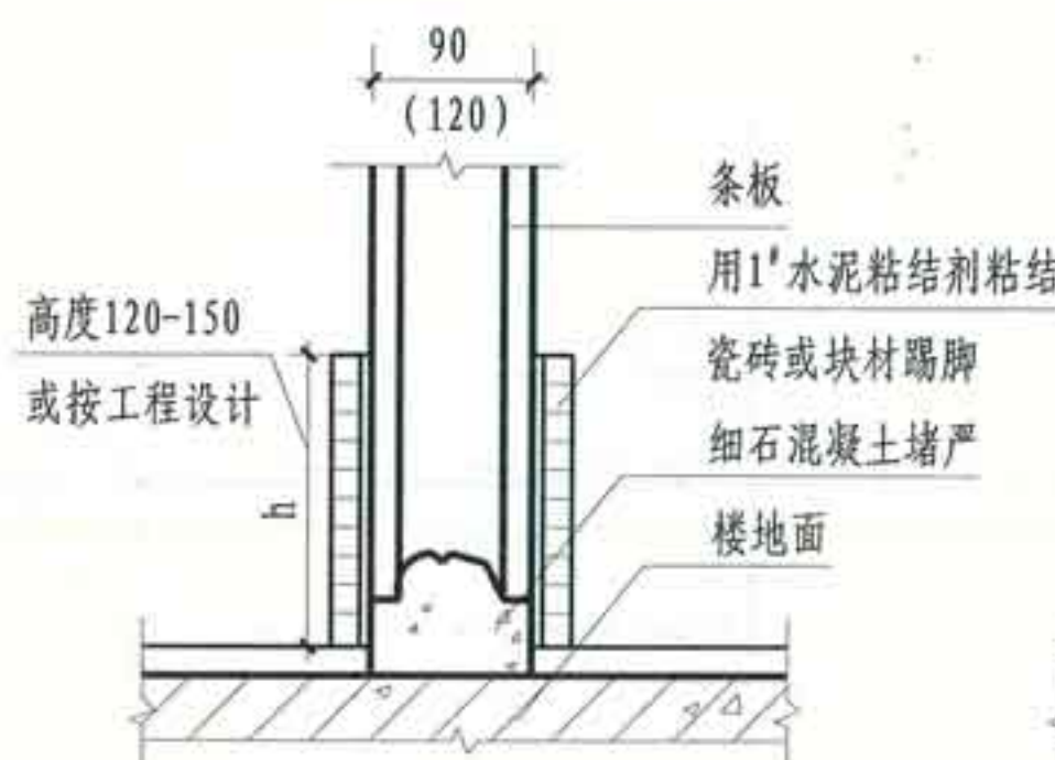
④ 瓷砖或块材踢脚
