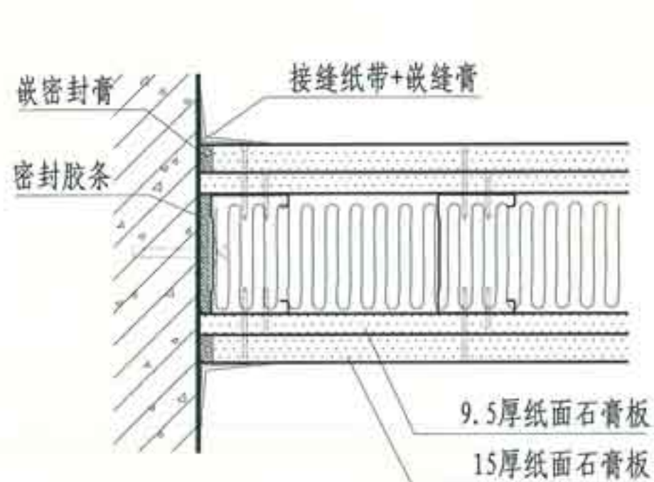
③ 调整石膏板厚度做法
