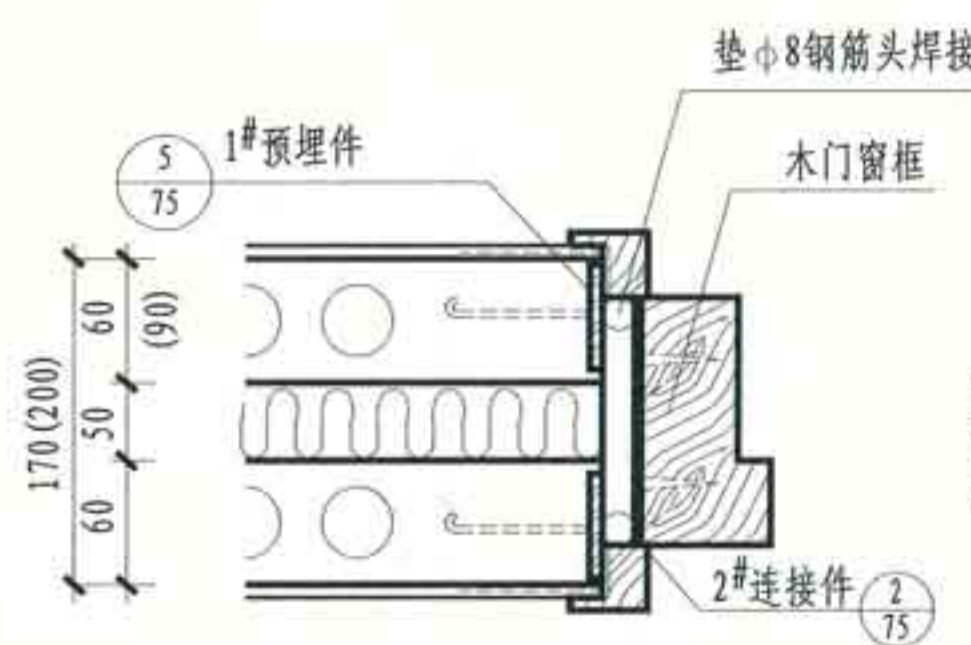
① 双层条板与木门窗框连接
