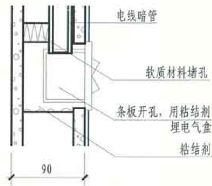
③ 暗线开关
