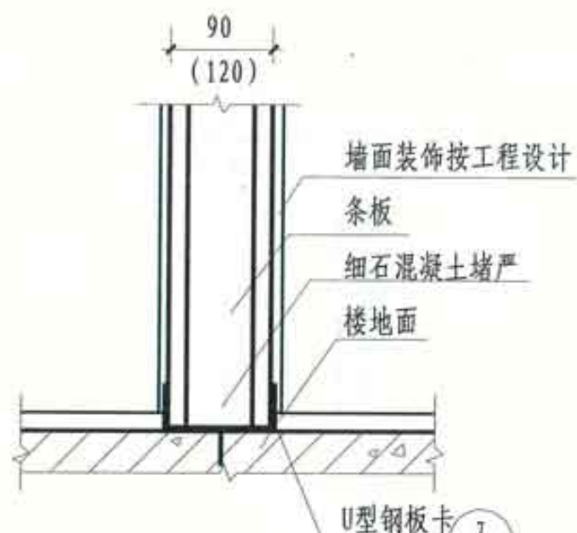
② 条板与楼地面连接
