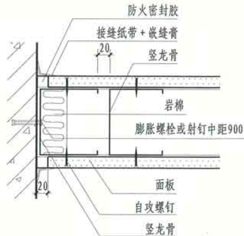
⑤ 防火节点连接
