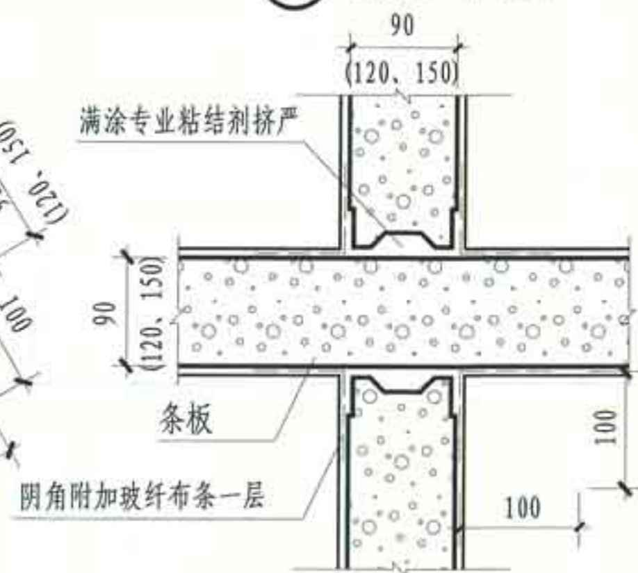
③ 条板丁字连接
