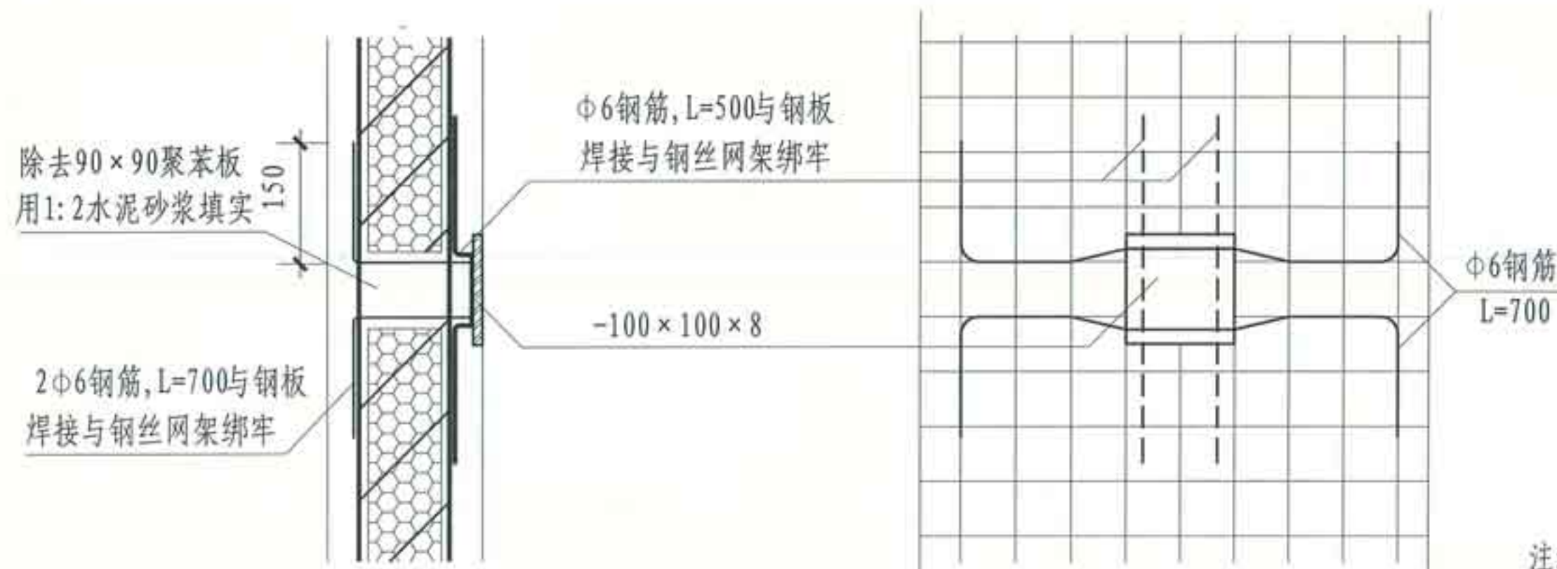
③ 预埋钢板构造
