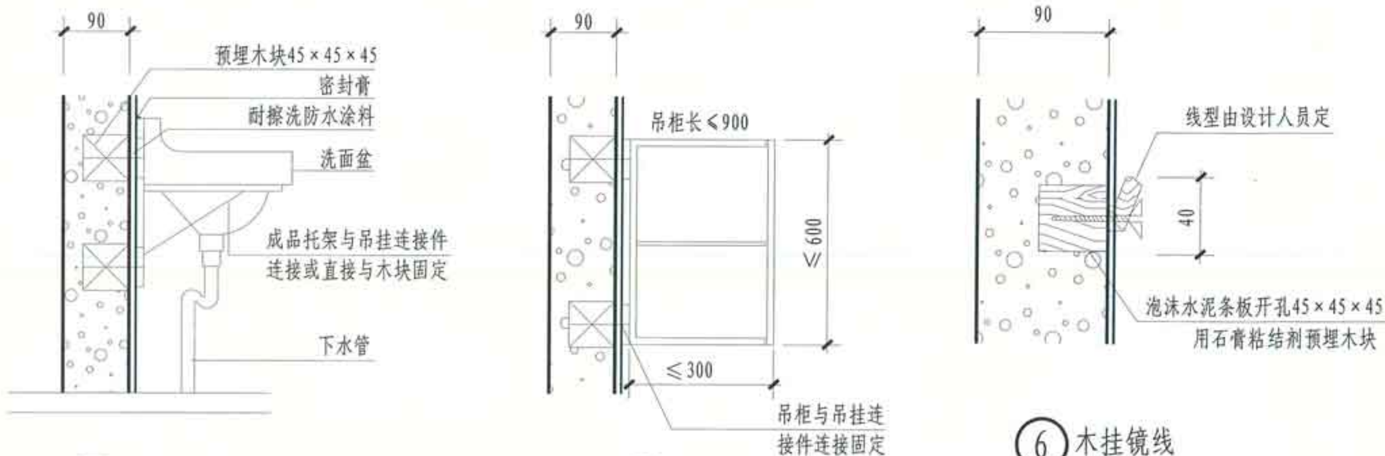
④ 洗面盆 ⑤ 吊柜 ⑥ 木挂镜线
