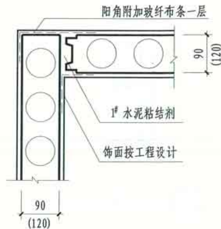
⑥ 条板直角连接
