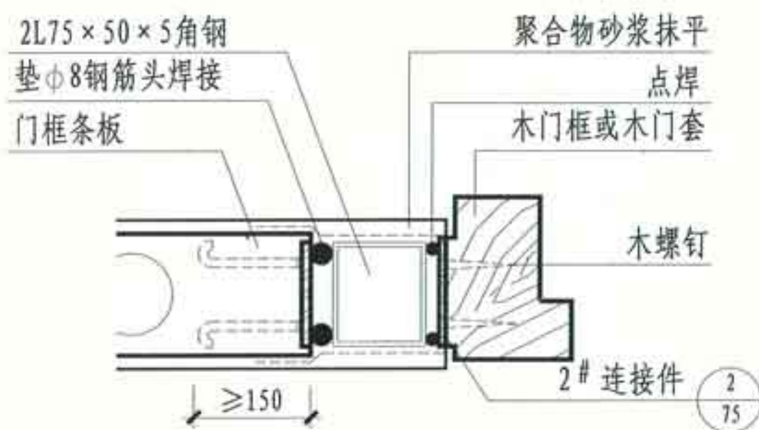
① 条板与钢抱框、木门框连接
