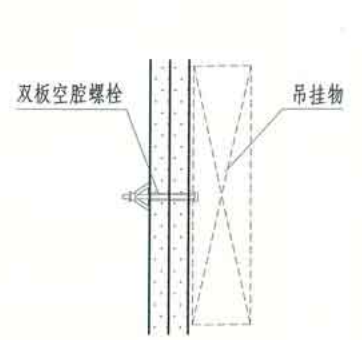
④ 双板空腔螺栓吊挂
