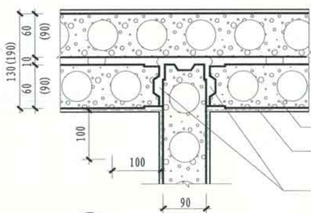
④ 双层条板与单层板丁字连接
