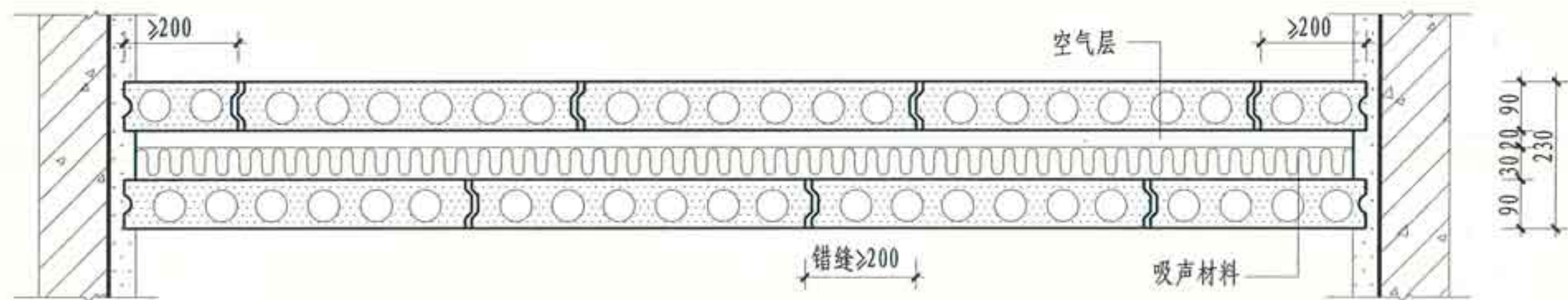
双层水泥、石膏、轻集料混凝土条板隔声墙平面二
