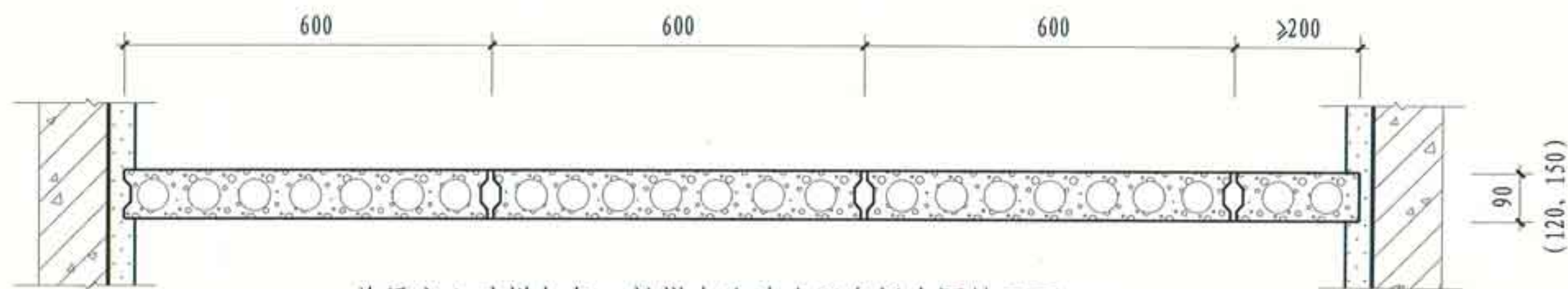
单层空心硅镁加气、粉煤灰泡沫水泥条板内隔墙平面
