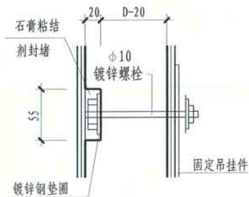
② 吊柜挂件
