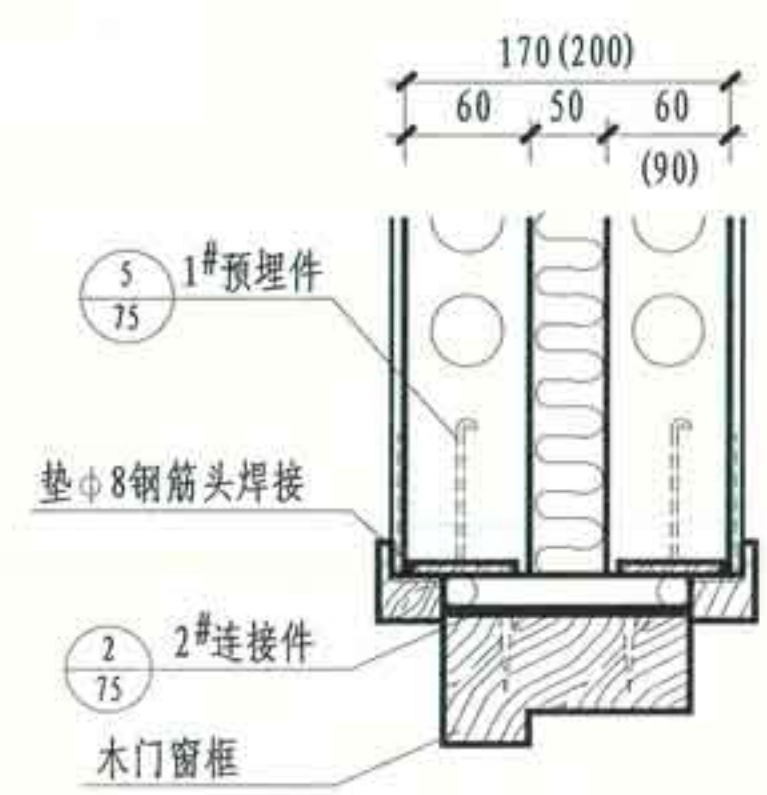
④ 门窗上板与木门窗框连接
