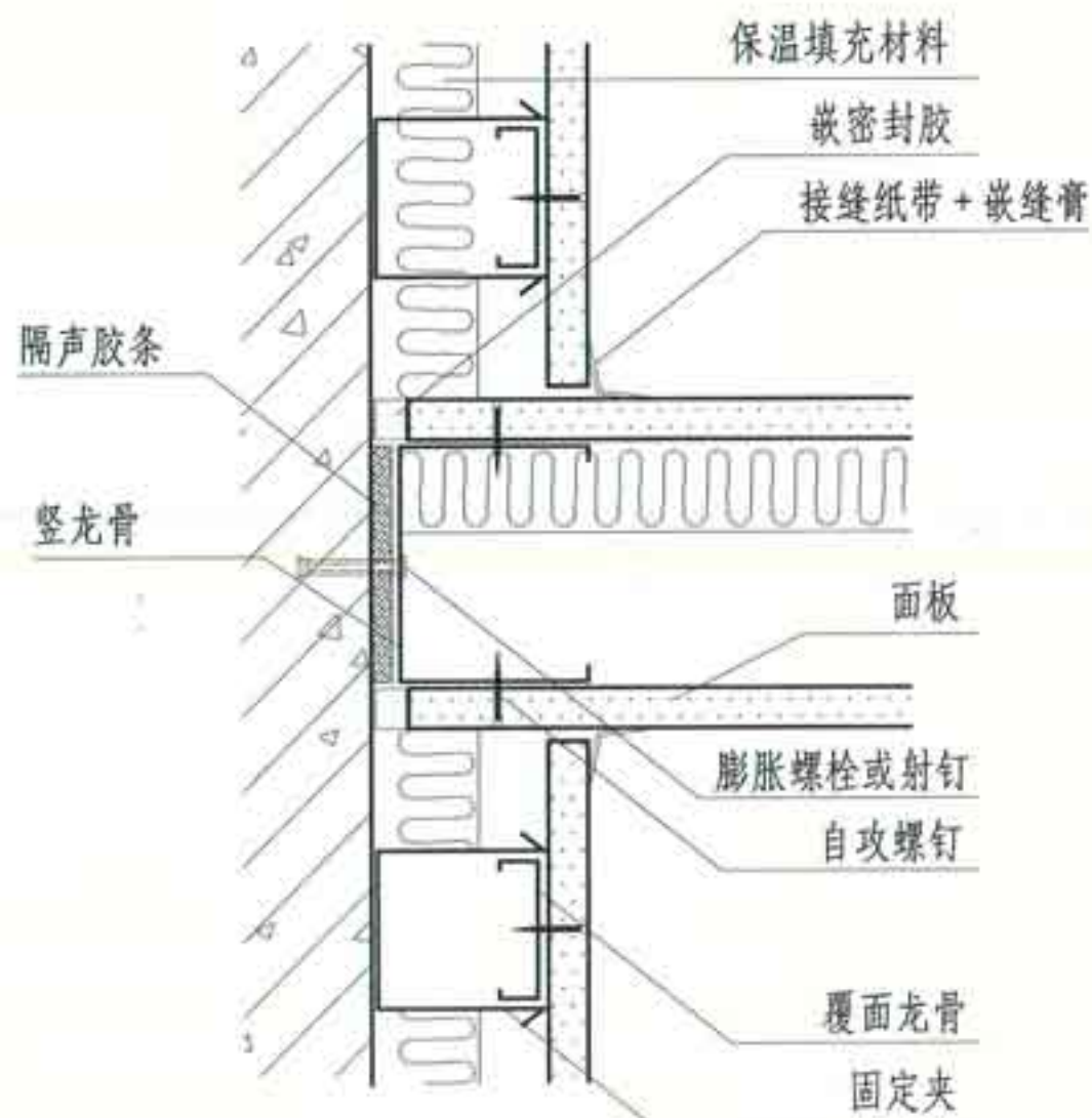
① 隔声墙伸缩缝
