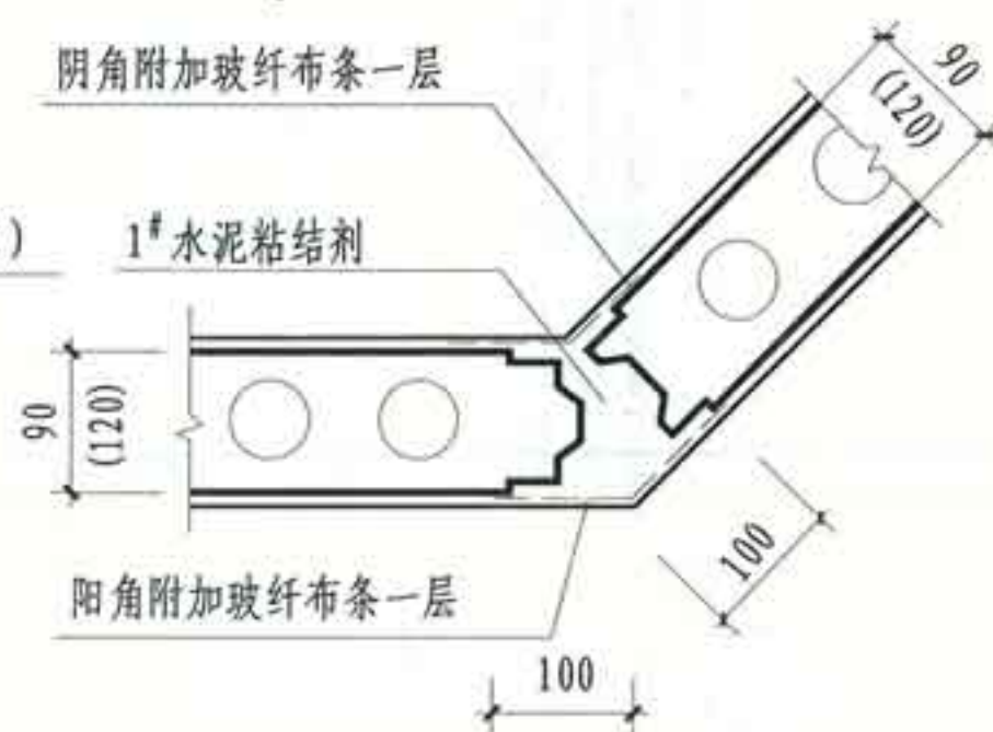
⑤ 条板任意角连接
