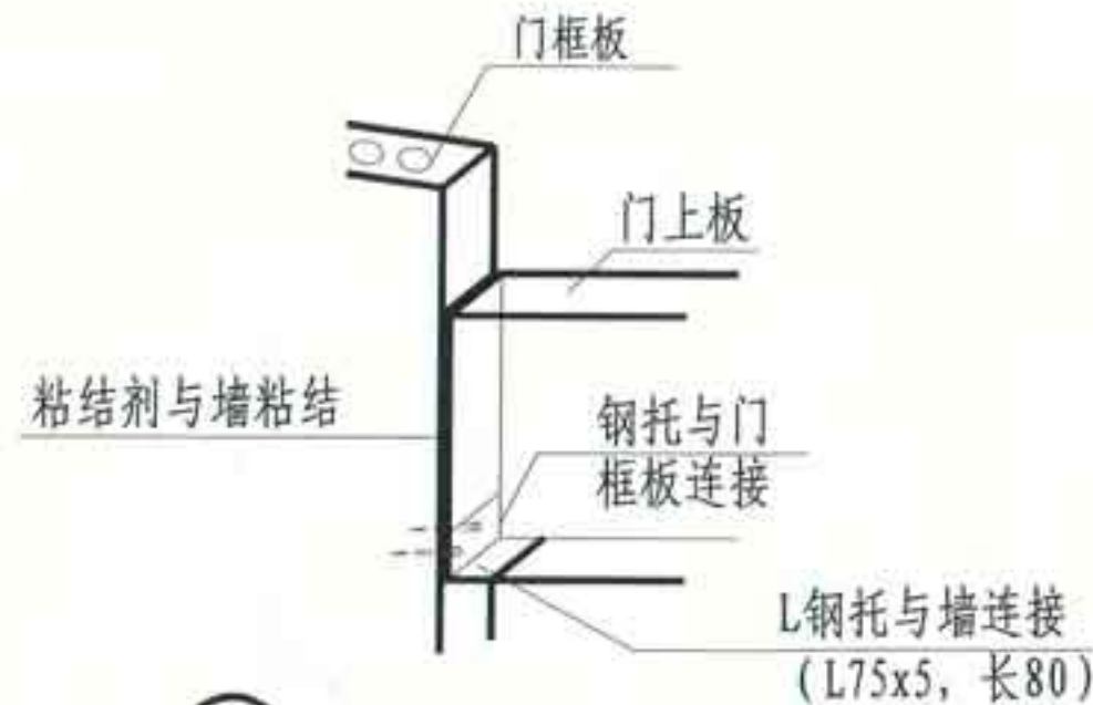
③ 门上板与门框板连接
