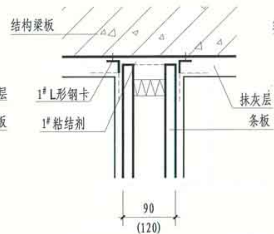
② 条板与结构梁、板连接
