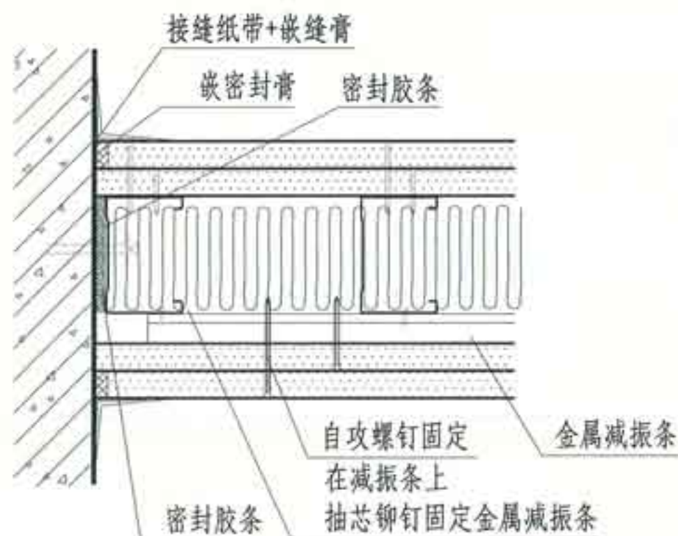
④ 加金属减振条做法
