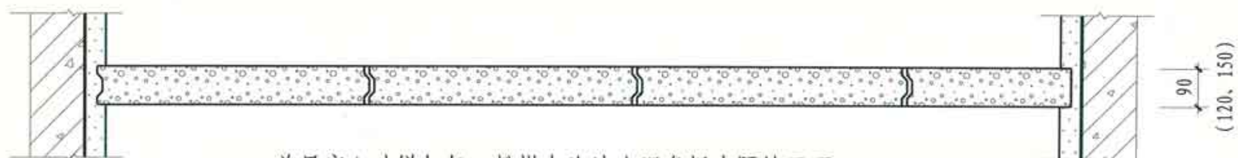
单层实心硅镁加气、粉煤灰泡沫水泥条板内隔墙平面
