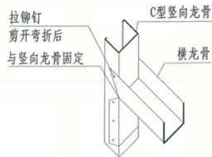
⑤ 门眉做法
