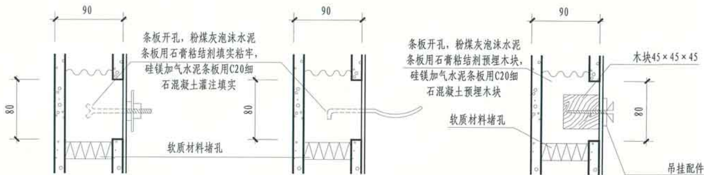
① 钢吊挂件 ② 暖气片挂钩 ③ 木吊挂件
