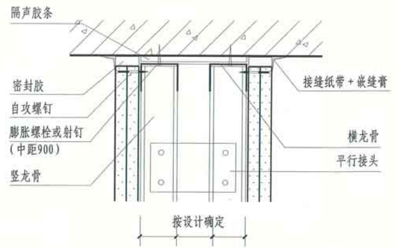
② 双排竖向龙骨并列
