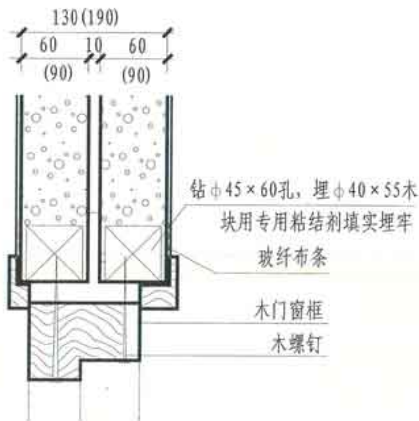
⑤ 门窗上板与木门窗框连接
