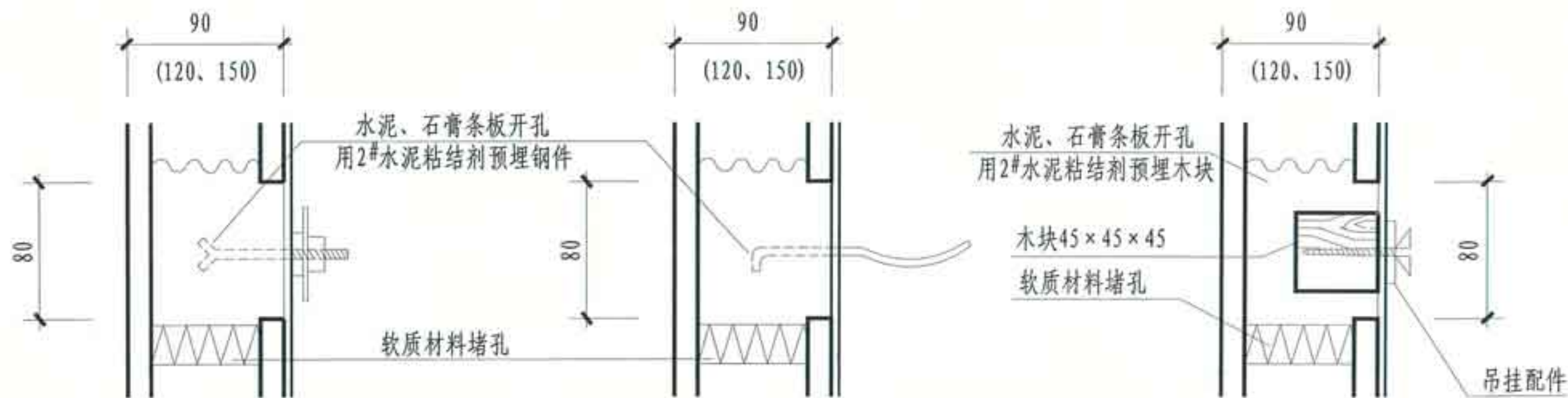
① 水泥、石膏条板钢吊挂件
