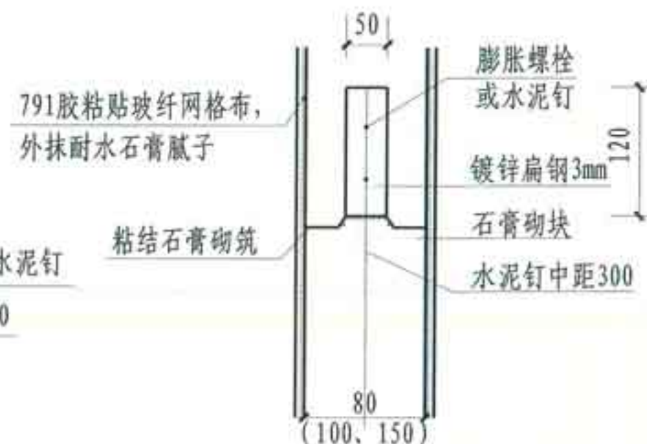
I-I剖面
