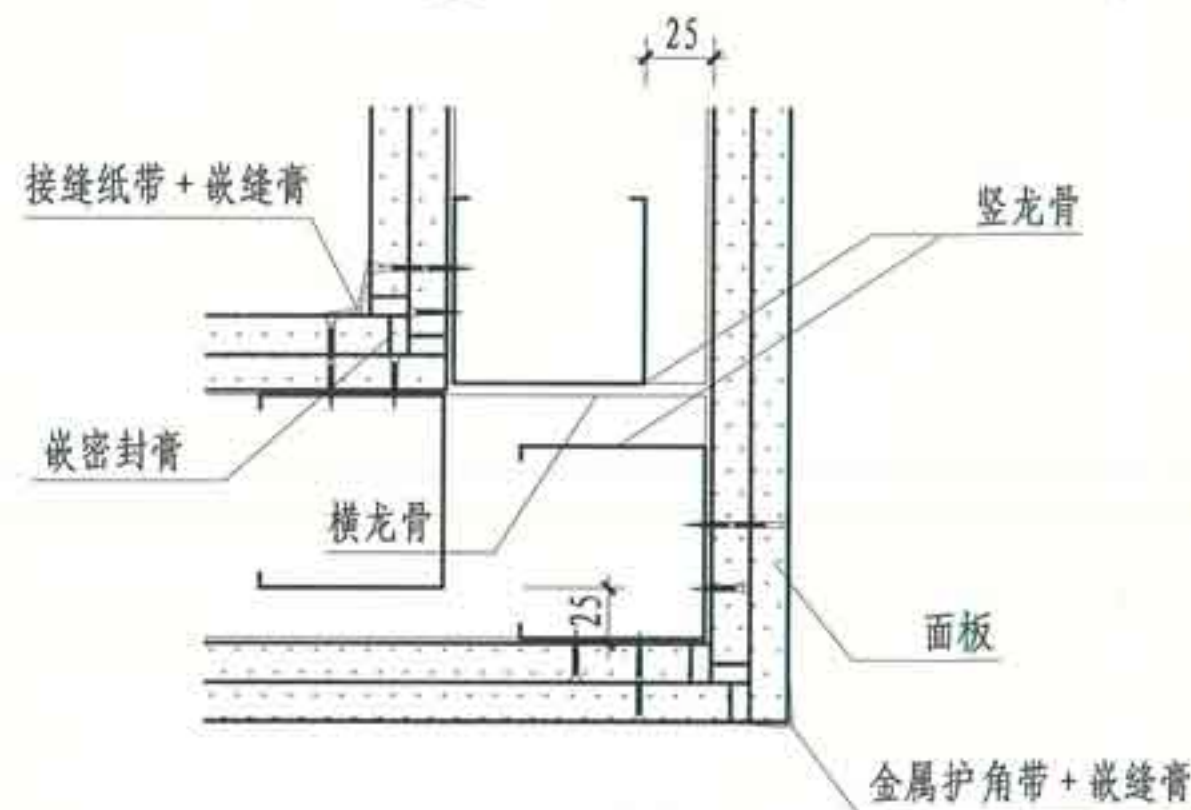
④ L形 (二)
