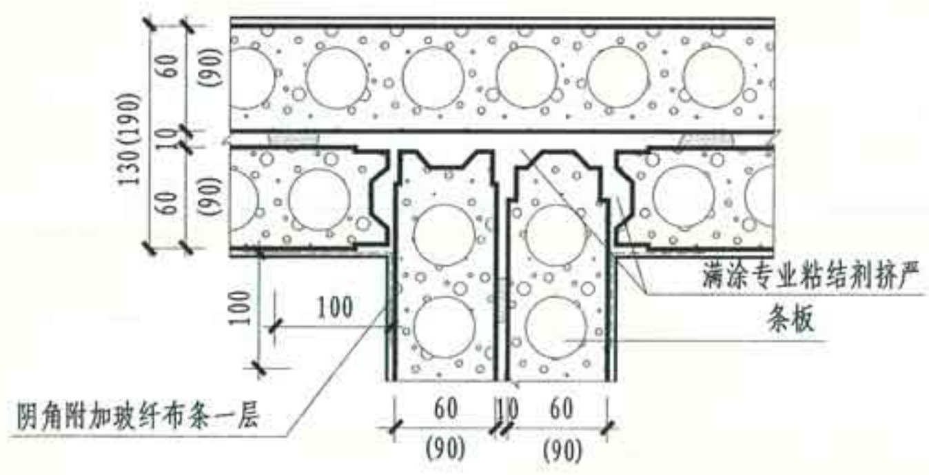
③ 双层条板丁字连接
