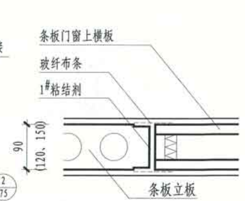
③ 条板门窗上横板与立板连接
