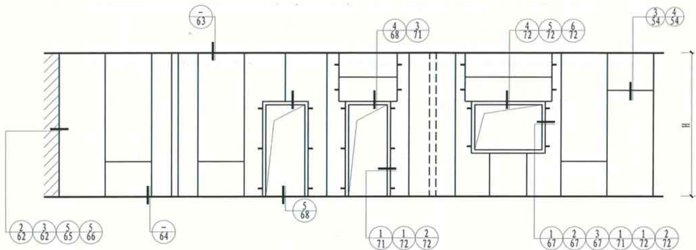
门洞口隔墙立面索引图
