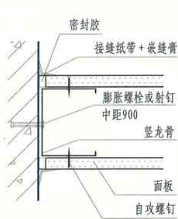
① 与结构墙（柱）连接
