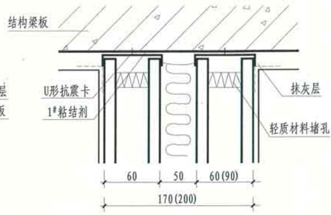
③ 双层条板与结构梁、板连接
