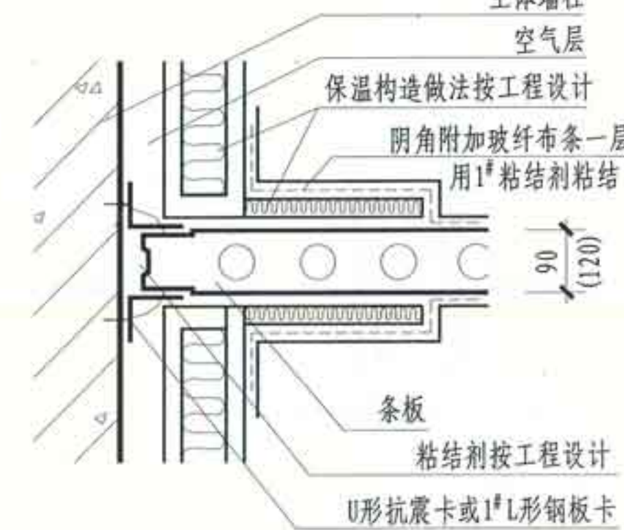
⑤ 条板与保温墙连接
