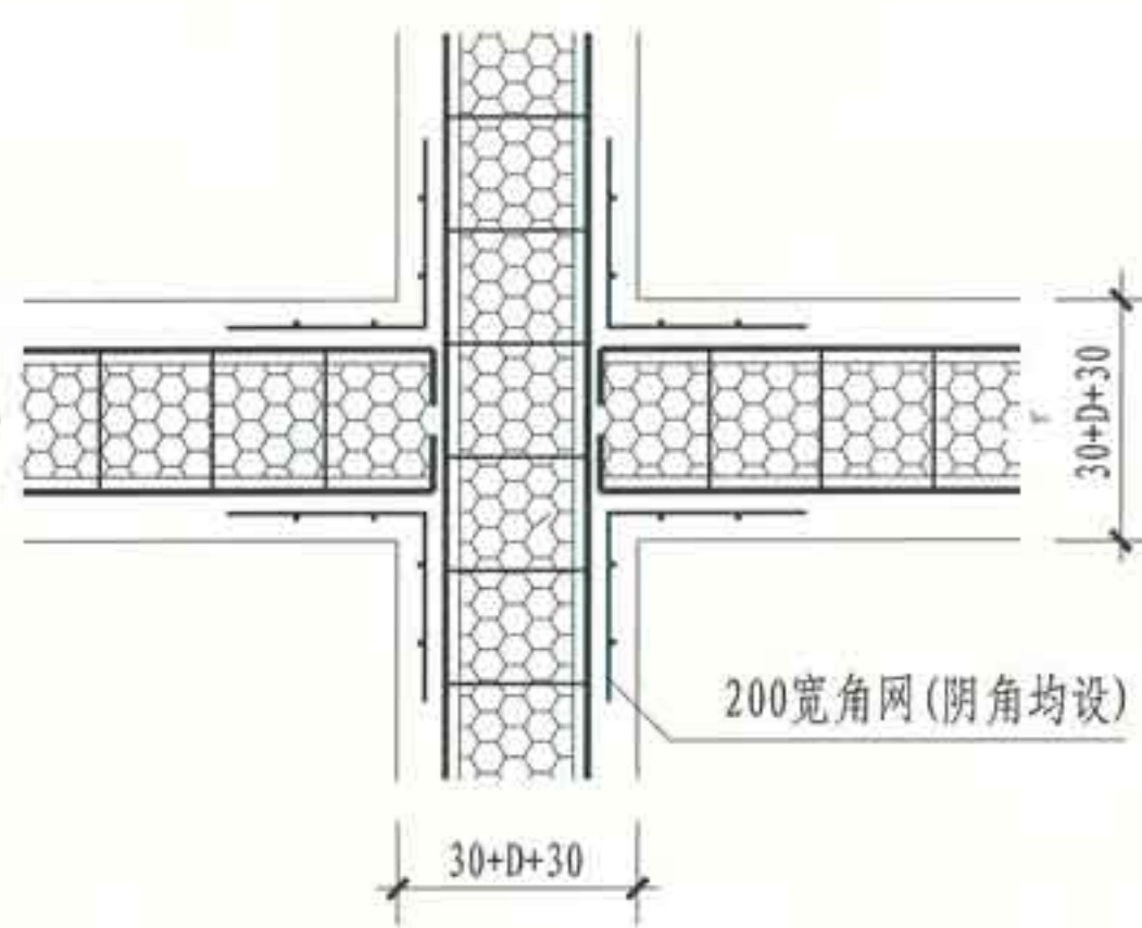
② 板墙与板墙十字连接构造
