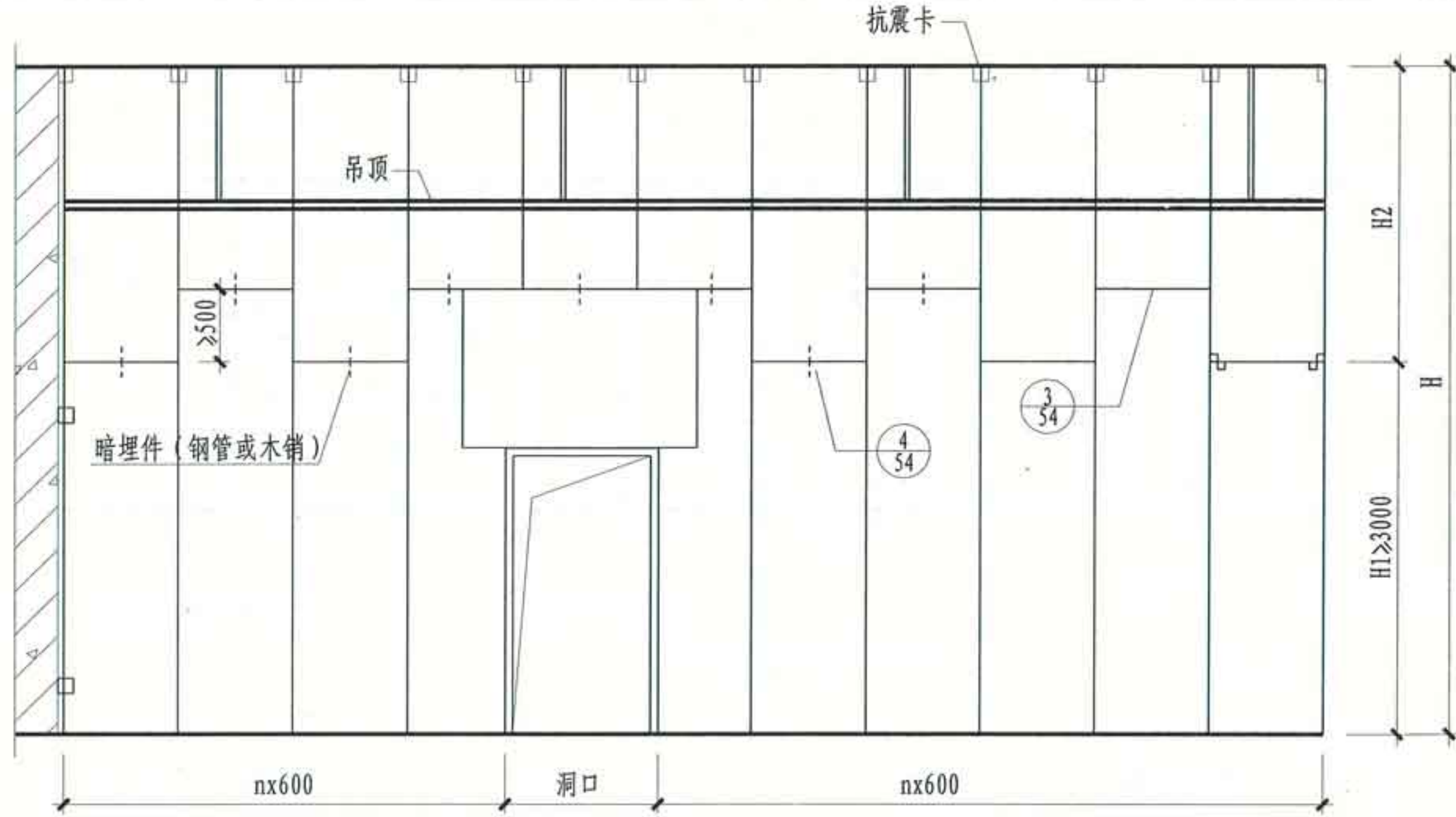
竖向接板立面索引图
