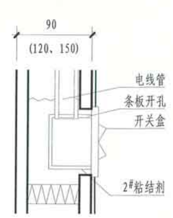
③ 暗线开关
