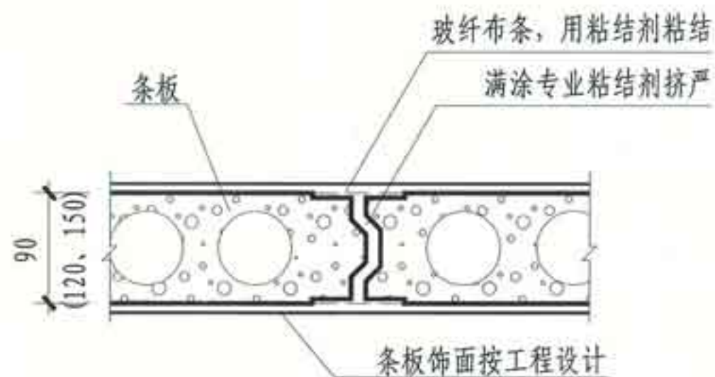
① 条板一字连接
