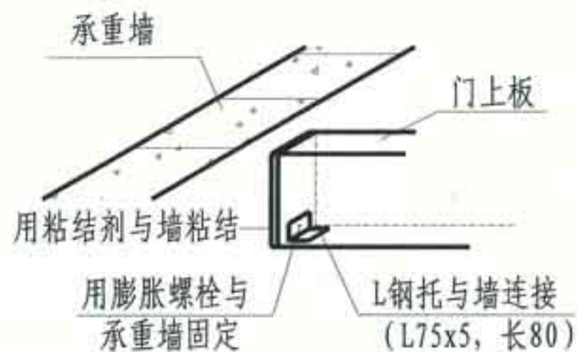
① 门上板与承重墙连接
