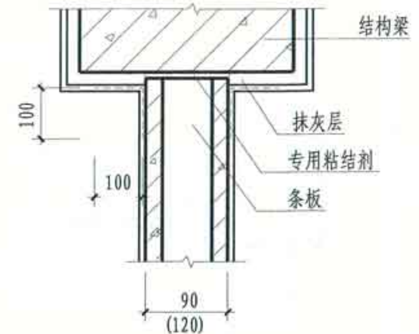
③ 条板与梁底连接
