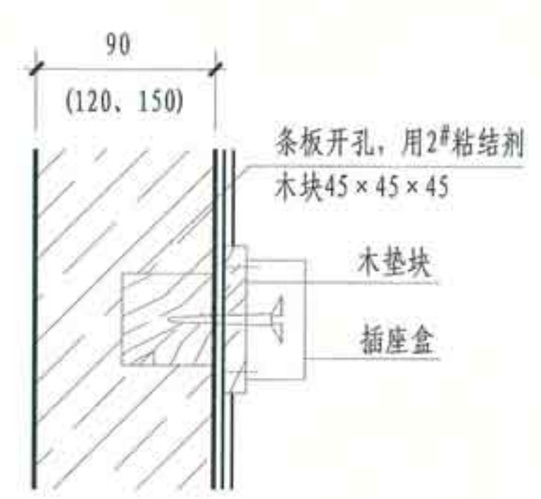
② 明线插座
