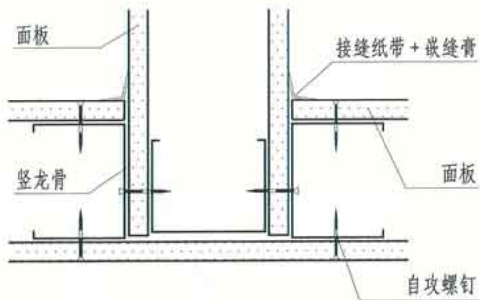
① T形 (一)
