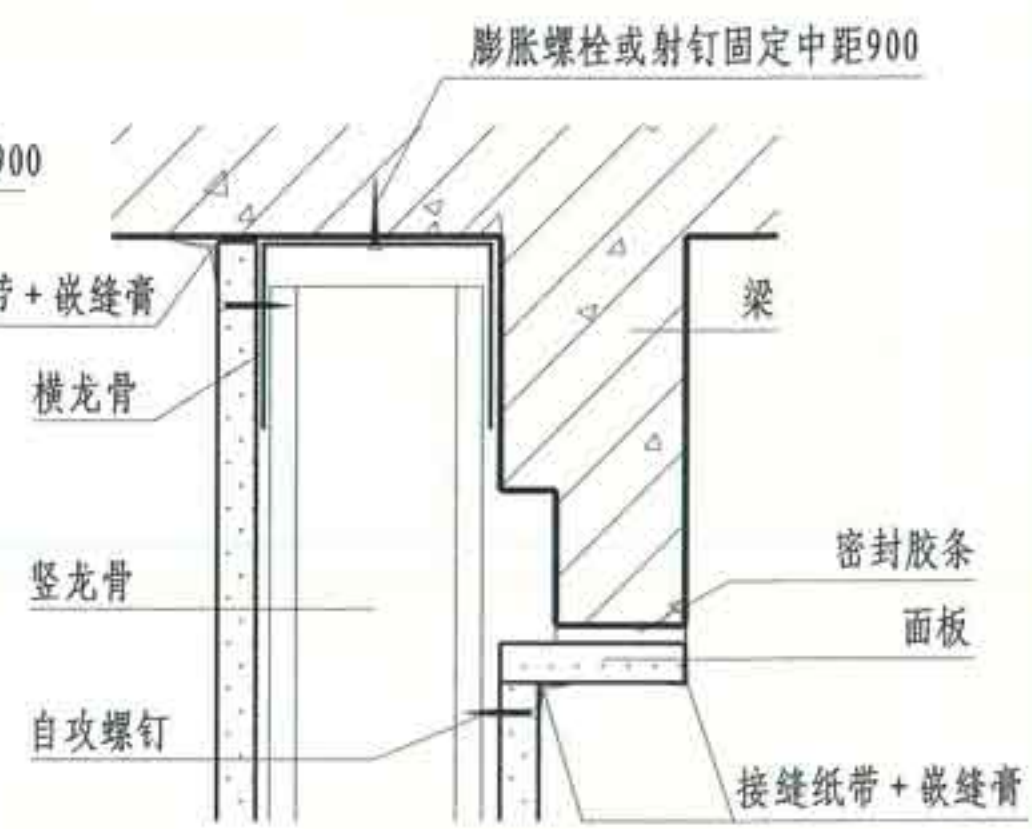
⑥ 梁侧面平齐连接
