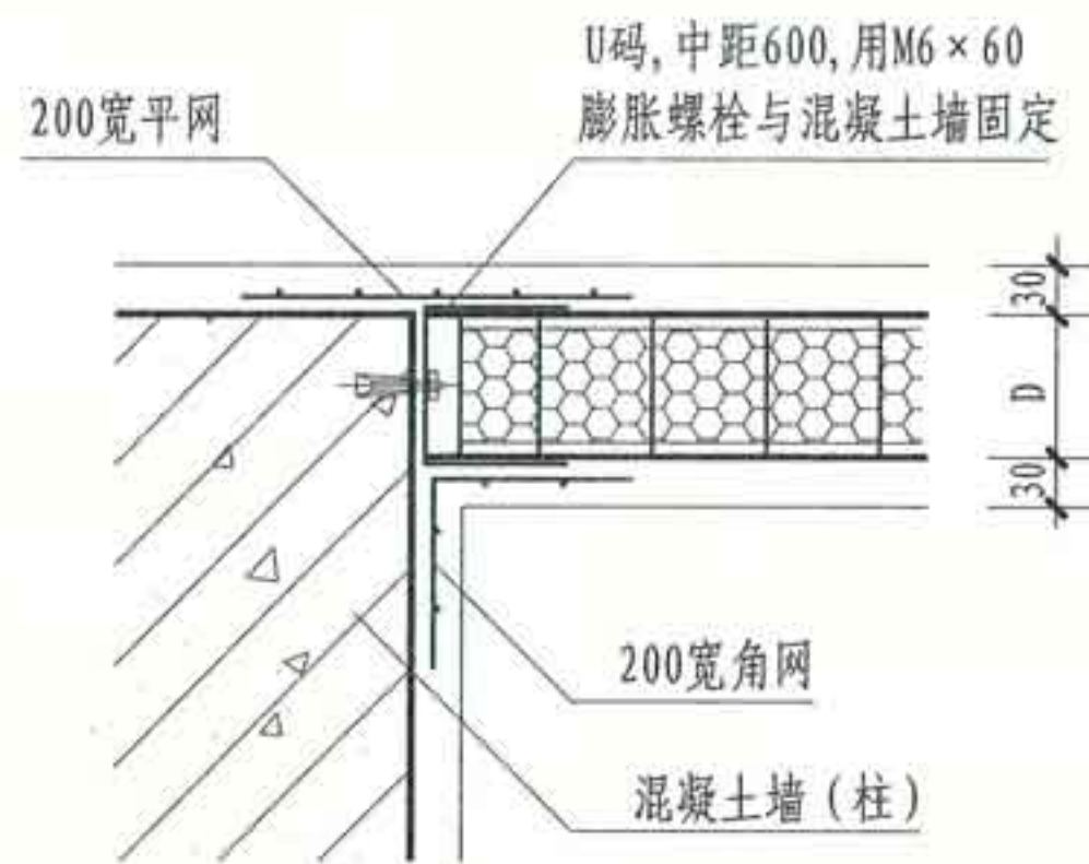
① 板墙与混凝土墙 (柱) 连接构造 (一)
