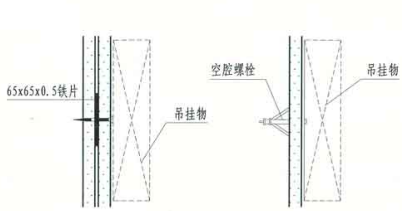
① 自攻螺钉吊挂
