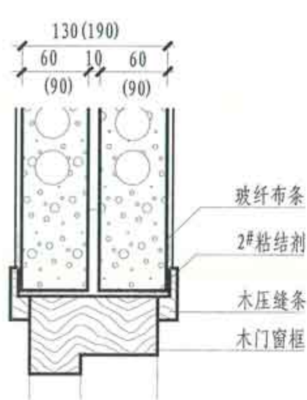
④ 门窗上板与木门窗框连接
