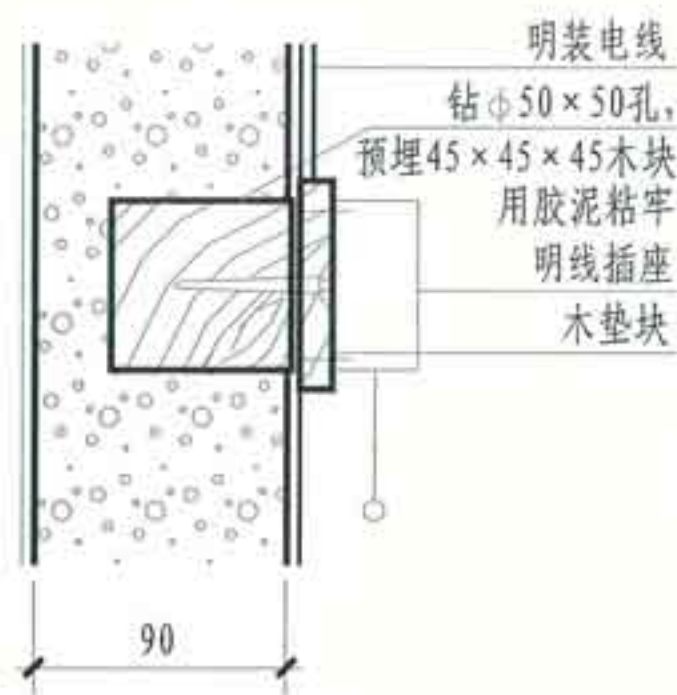
② 明线插座
