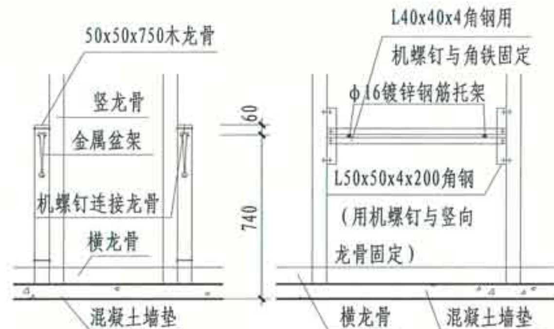
金属盆架支撑龙骨立面
