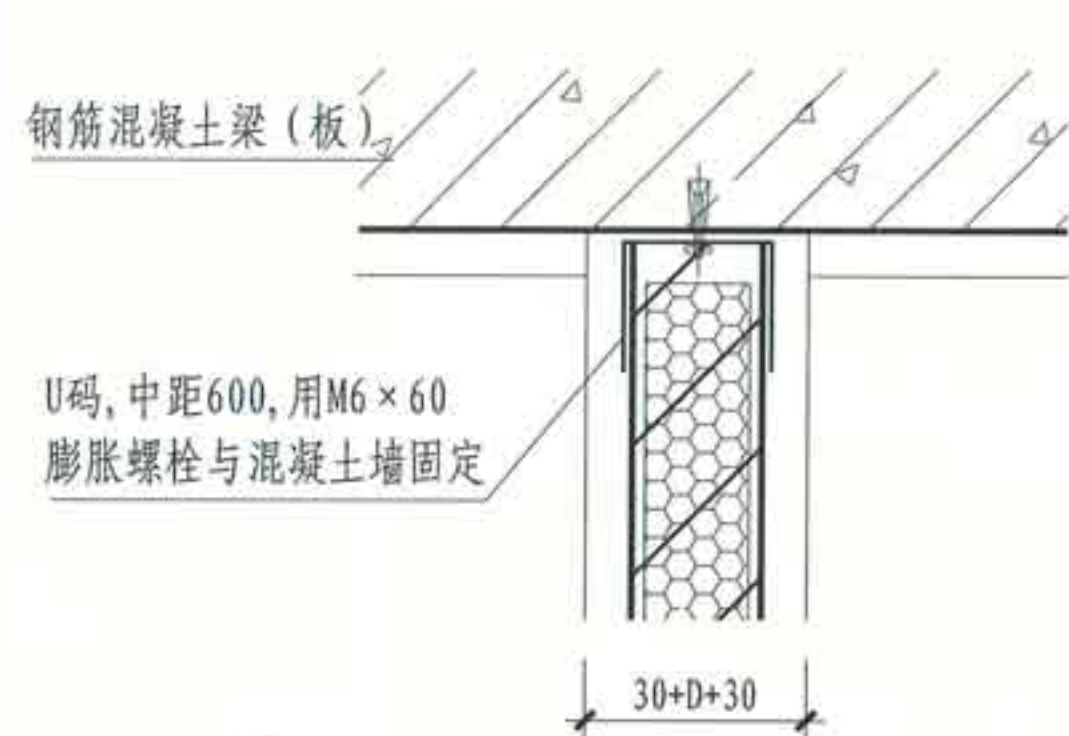
① 板墙与混凝土梁 (板) 连接构造 (一)
