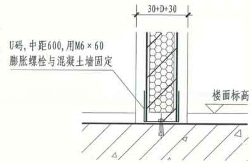
④ 板墙与楼面连接构造
