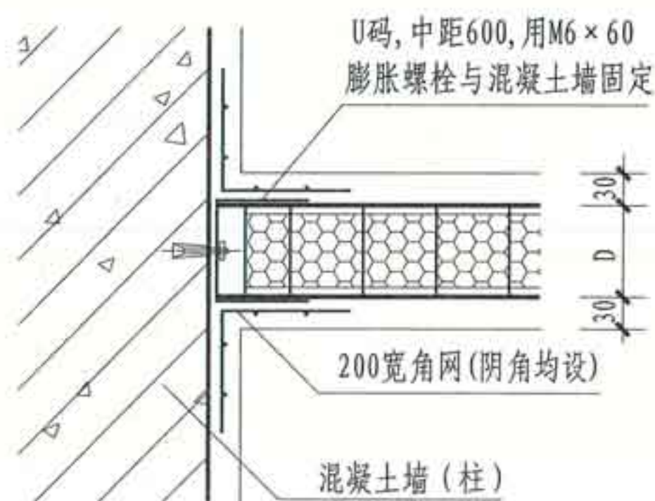
③ 板墙与混凝土墙 (柱) 连接构造 (二)
