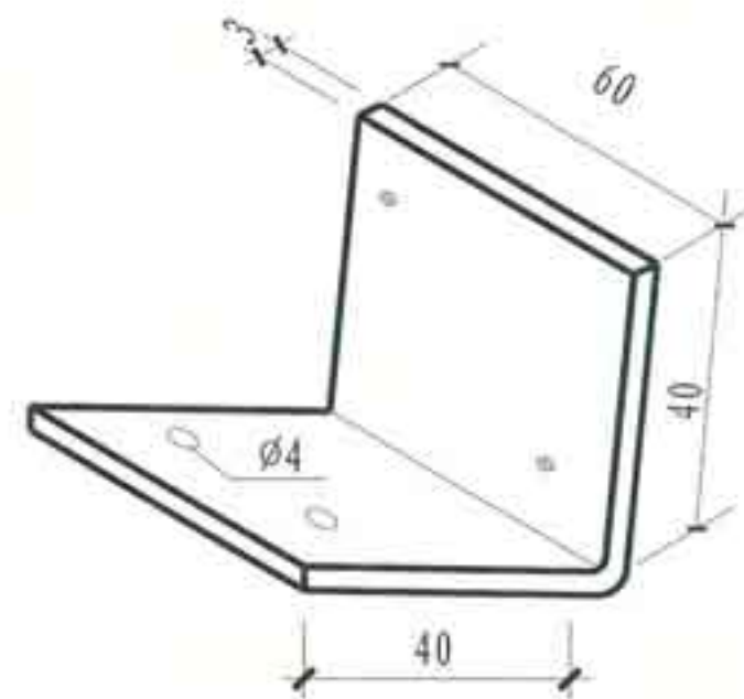
③ 1#L型钢板卡
