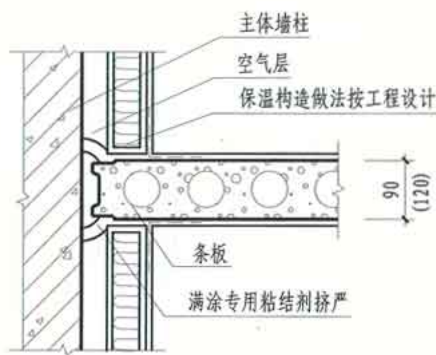
② 条板与保温墙连接
