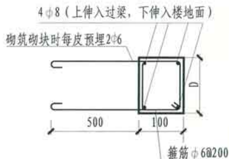
① 木门框与砌块隔墙连接 ② 抱框(C20混凝土门柱) ③ 门洞上部过梁构造 ④ 木门框与钢筋混凝土过梁连接
