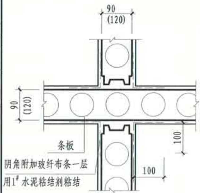
① 条板丁字连接
