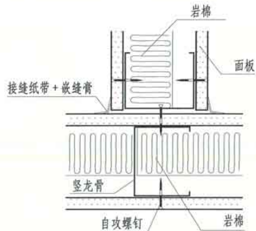
④ T形 (四)
