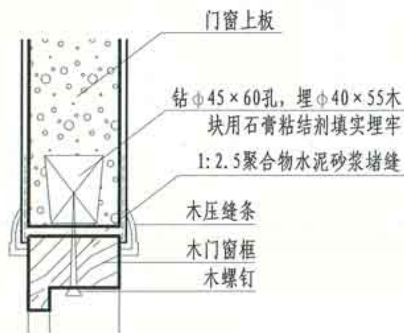
③ 门窗上板与木门窗框连接
