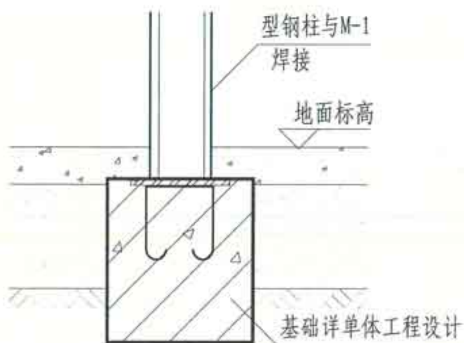
② 加劲柱与地面连接构造
