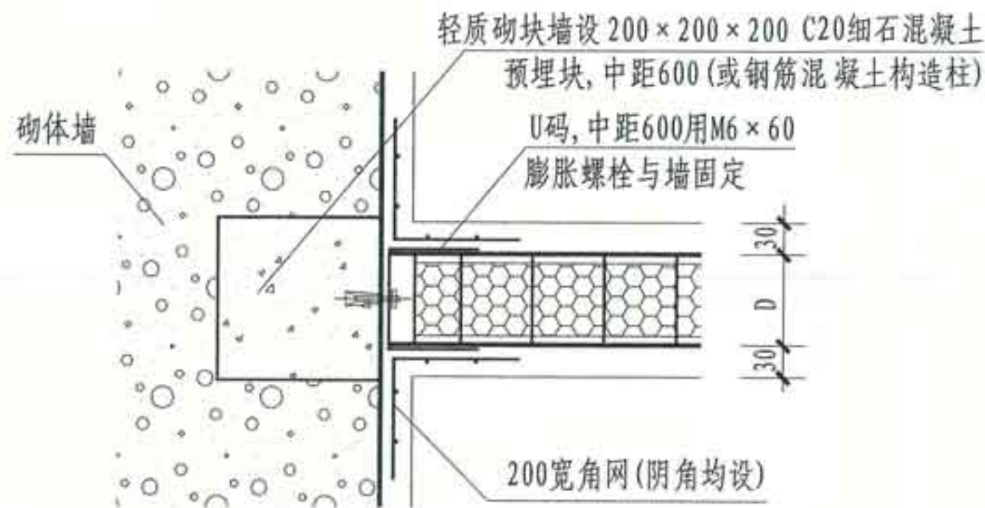
④ 板墙与砌体墙连接构造 (二)
