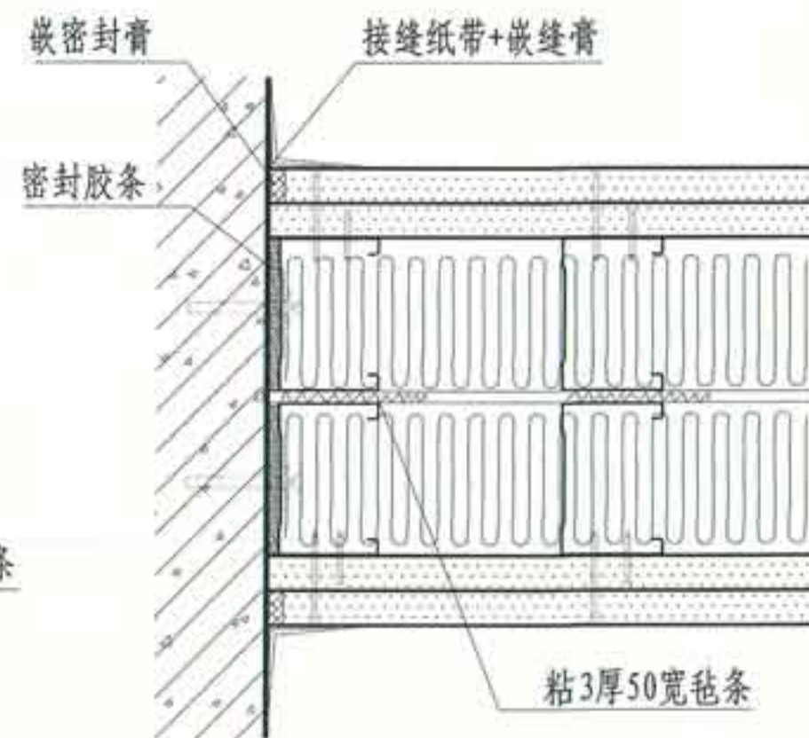
⑤ 双排龙骨做法
