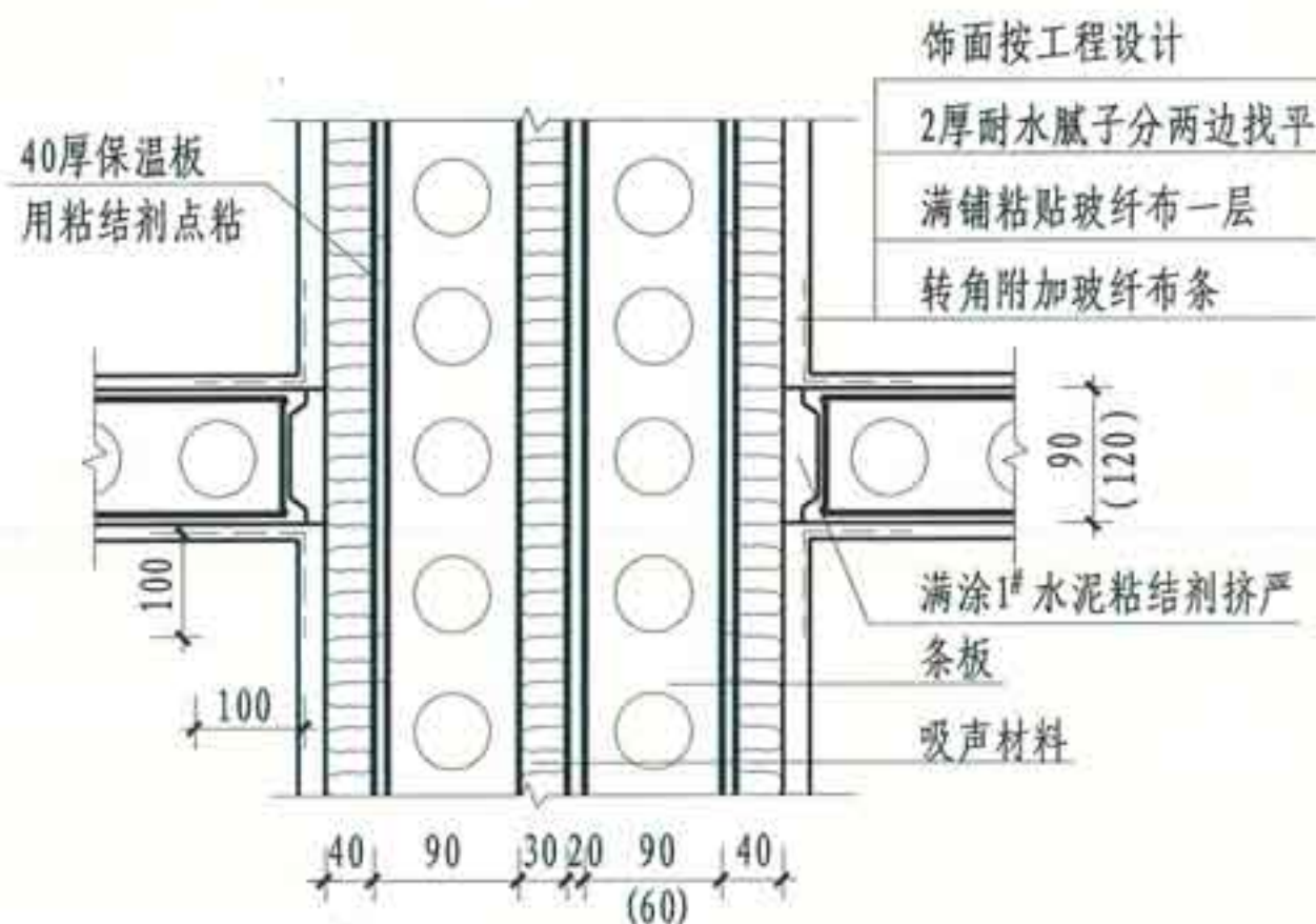
③ 双层条板隔墙 (分户墙保温)
