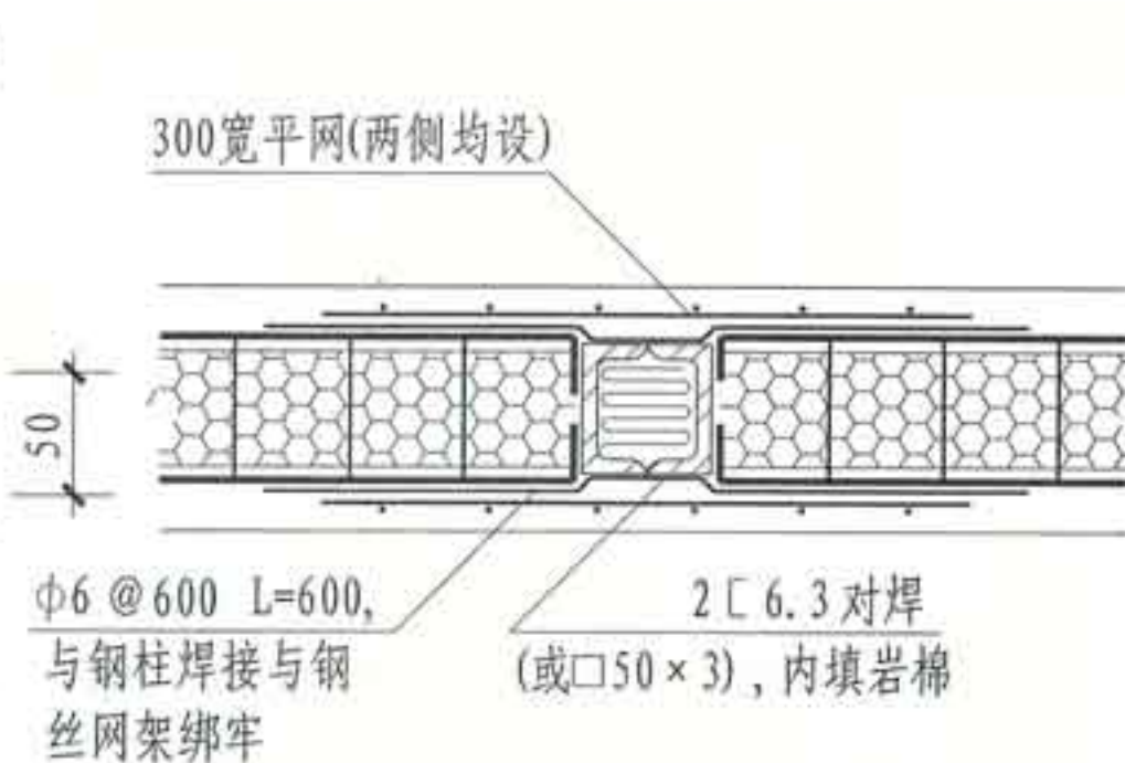
③ 板墙加劲柱构造(一)
