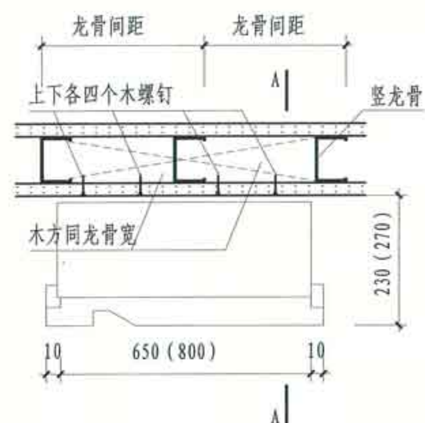
① 明装消火栓
