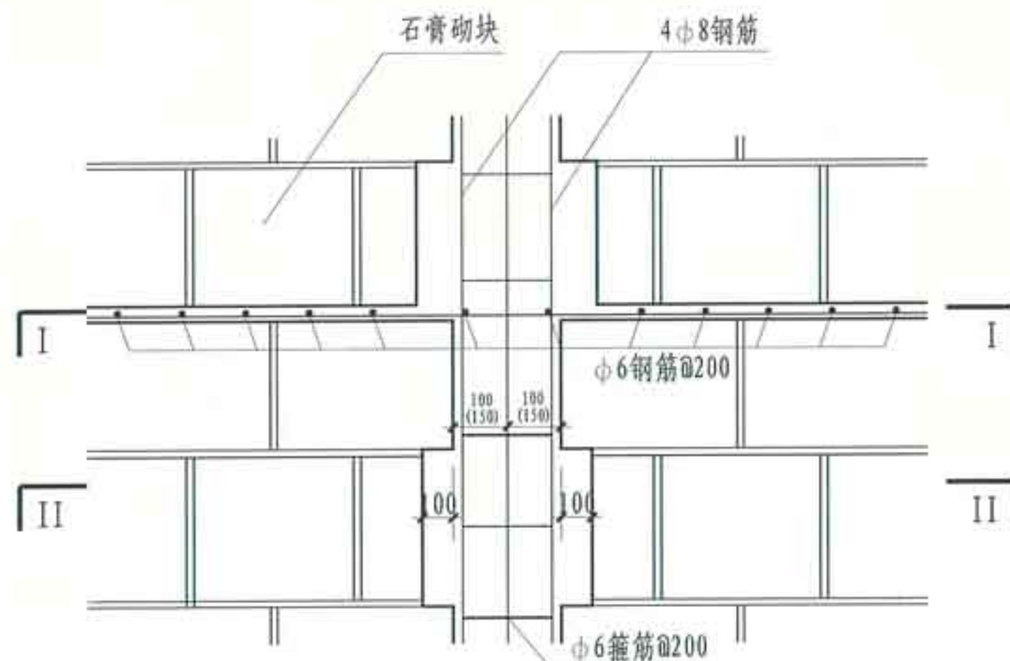
① 构造柱立面
