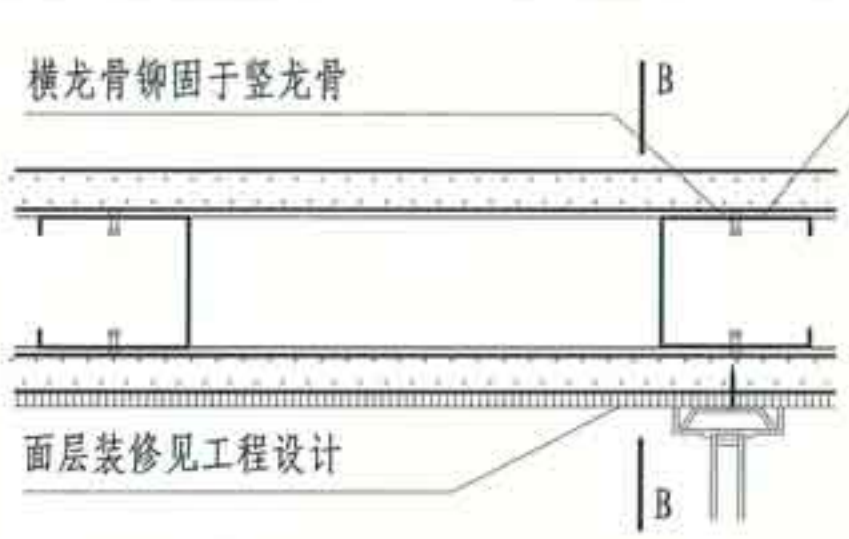
② 固定吊挂件之二
