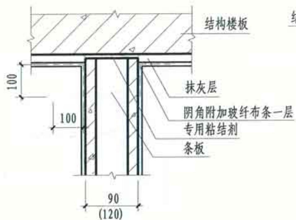
① 条板与楼板底面连接
