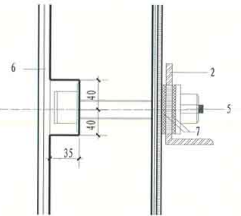
④ 固定各种金属支架详图
