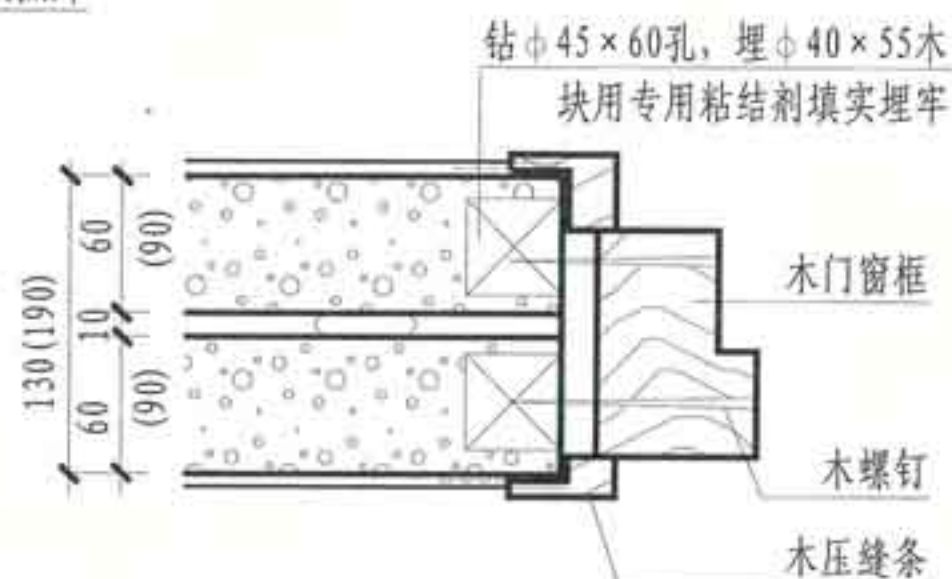
② 双层条板与木门窗框连接
