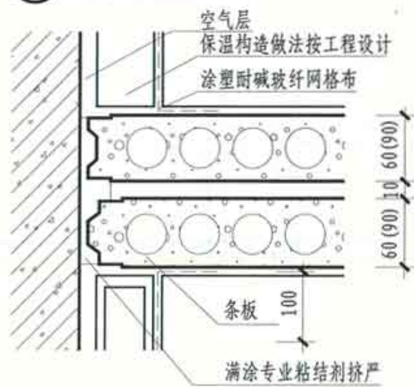
② 条板与保温墙连接
