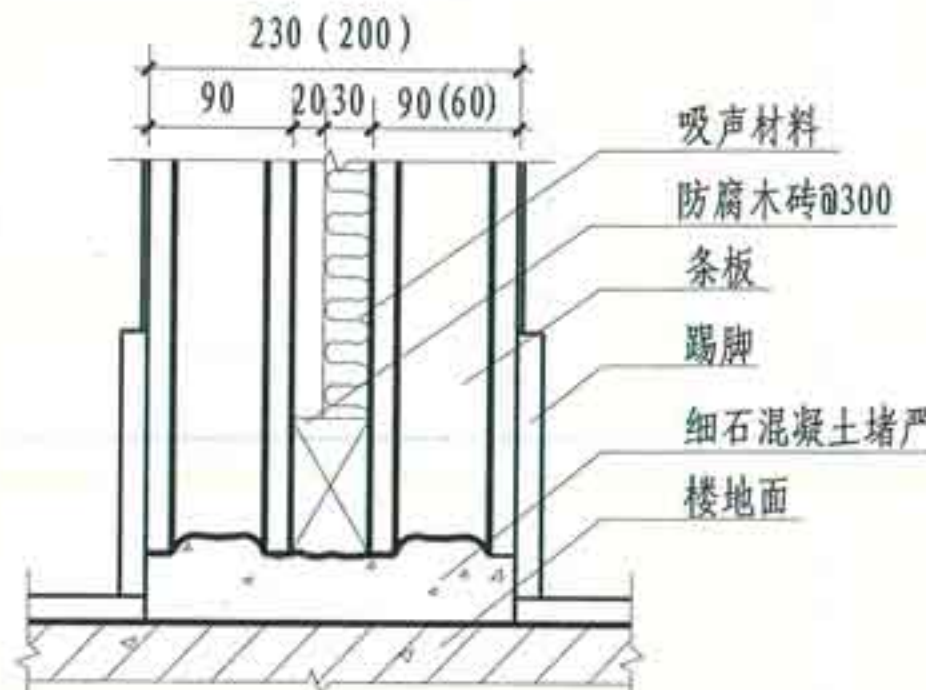
⑥ 双层条板隔声墙与楼地面连接
