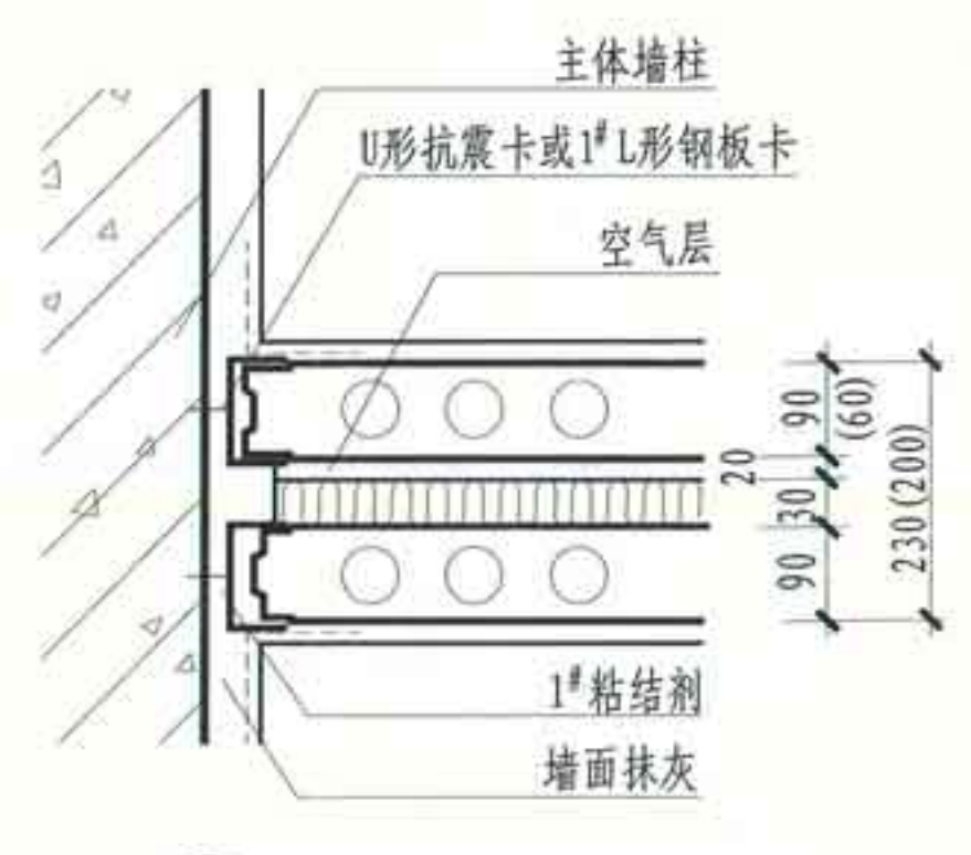
⑥ 双层条板与结构墙、柱连接
