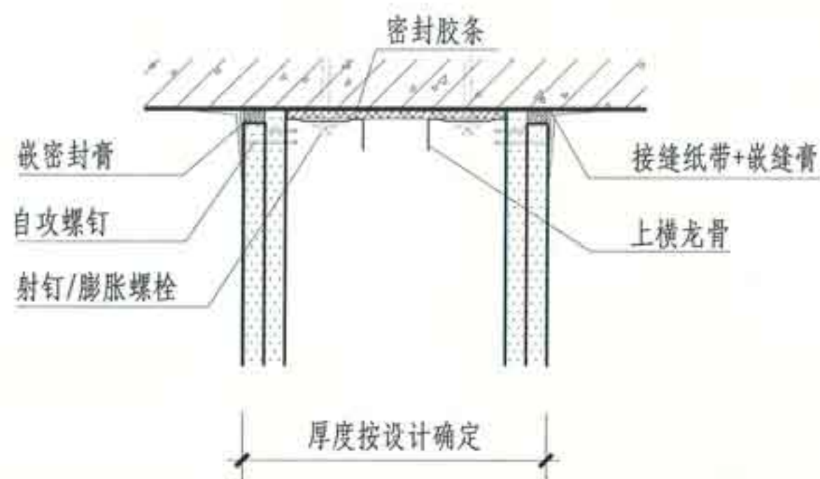
① 双排龙骨并列
