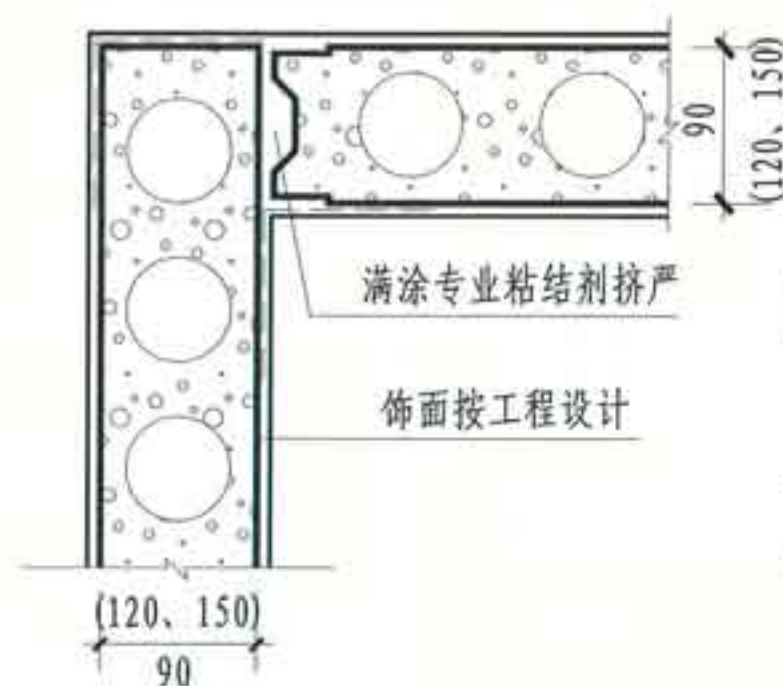
② 条板直角连接
