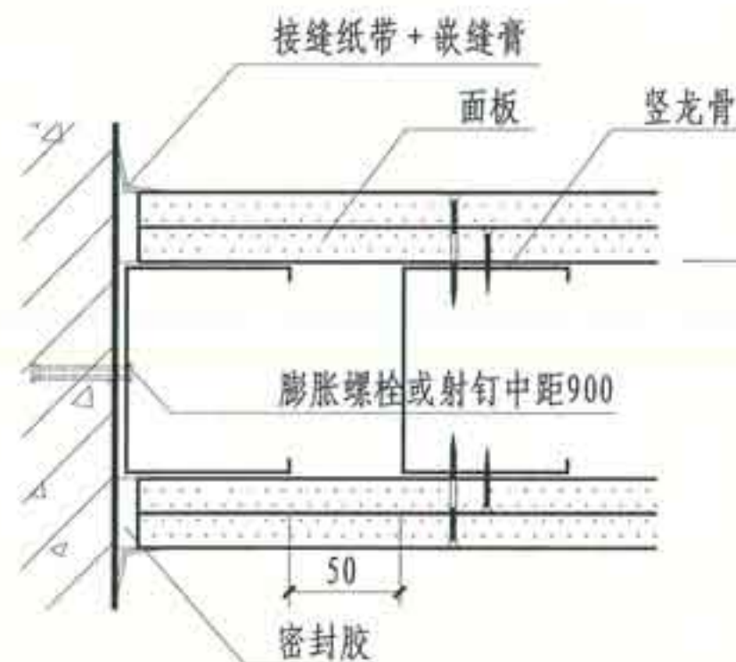
④ 与结构墙（柱）连接
