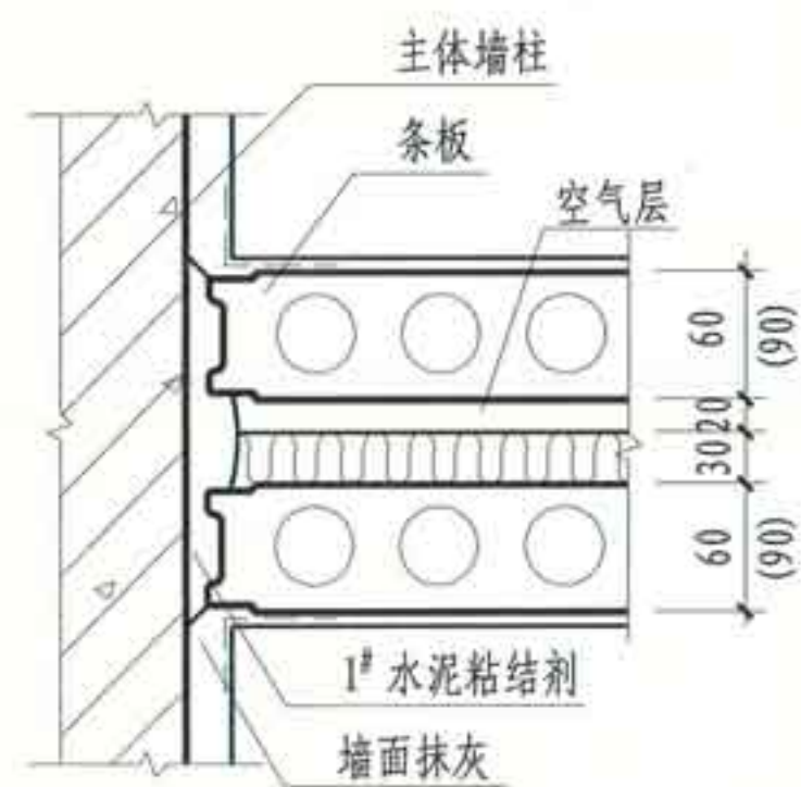
④ 双层条板与墙柱连接
