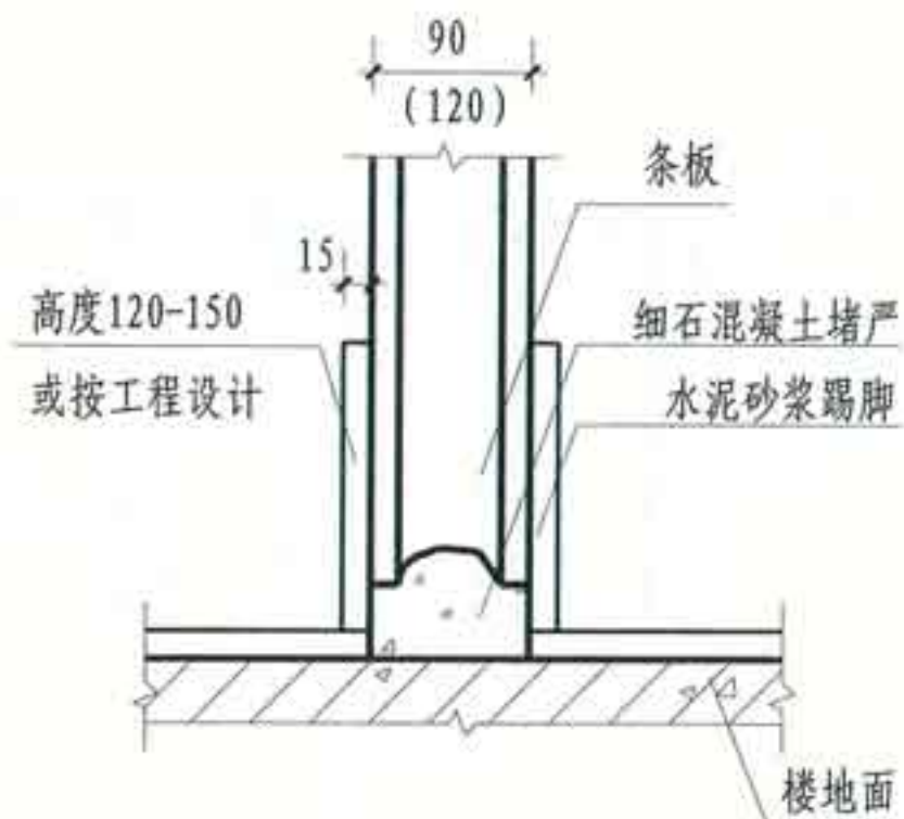
① 水泥砂浆踢脚
