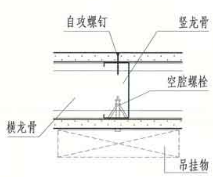
⑥ 竖向龙骨吊挂
