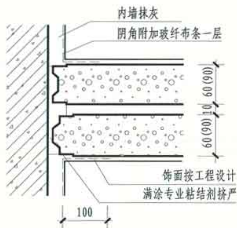
④ 双层条板与墙连接
