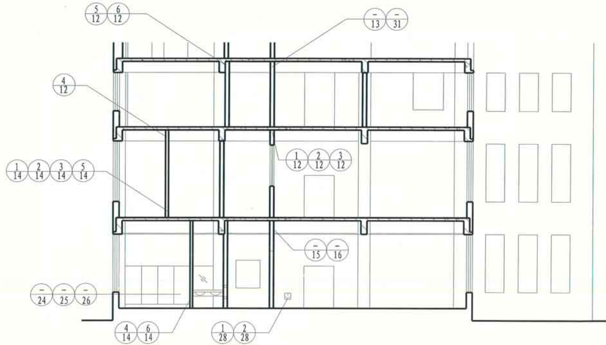
1-1剖面索引图
