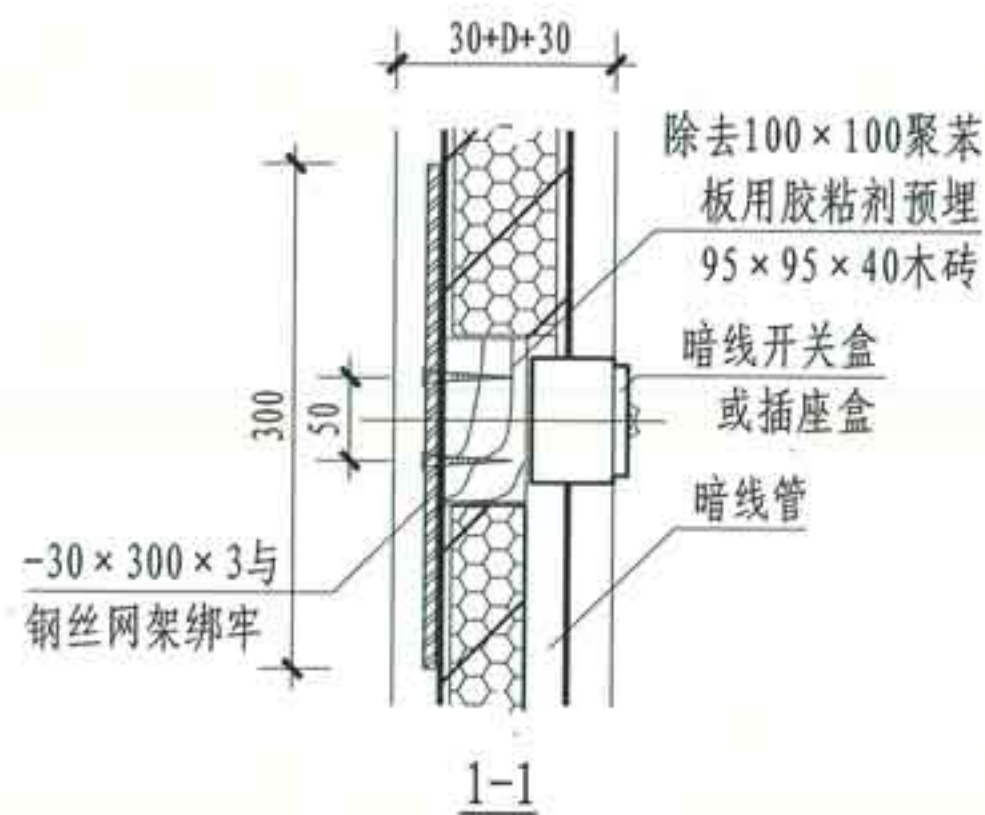
② 暗线开关、插座
