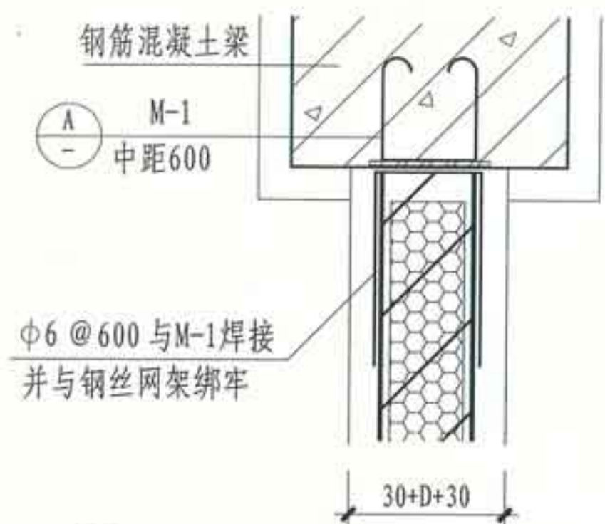
② 板墙与混凝土梁连接构造 (二)
