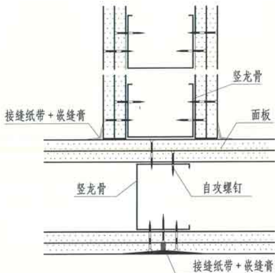
③ T形 (三)
