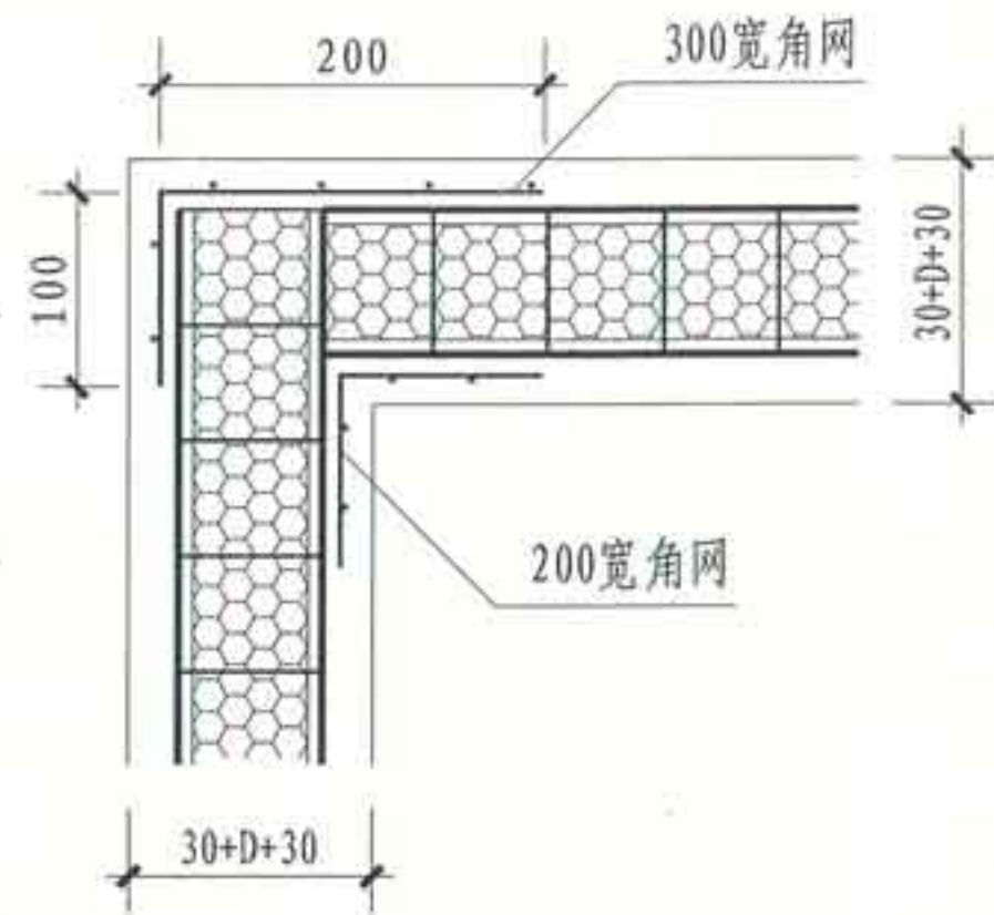
③ 板墙与板墙转角连接构造
