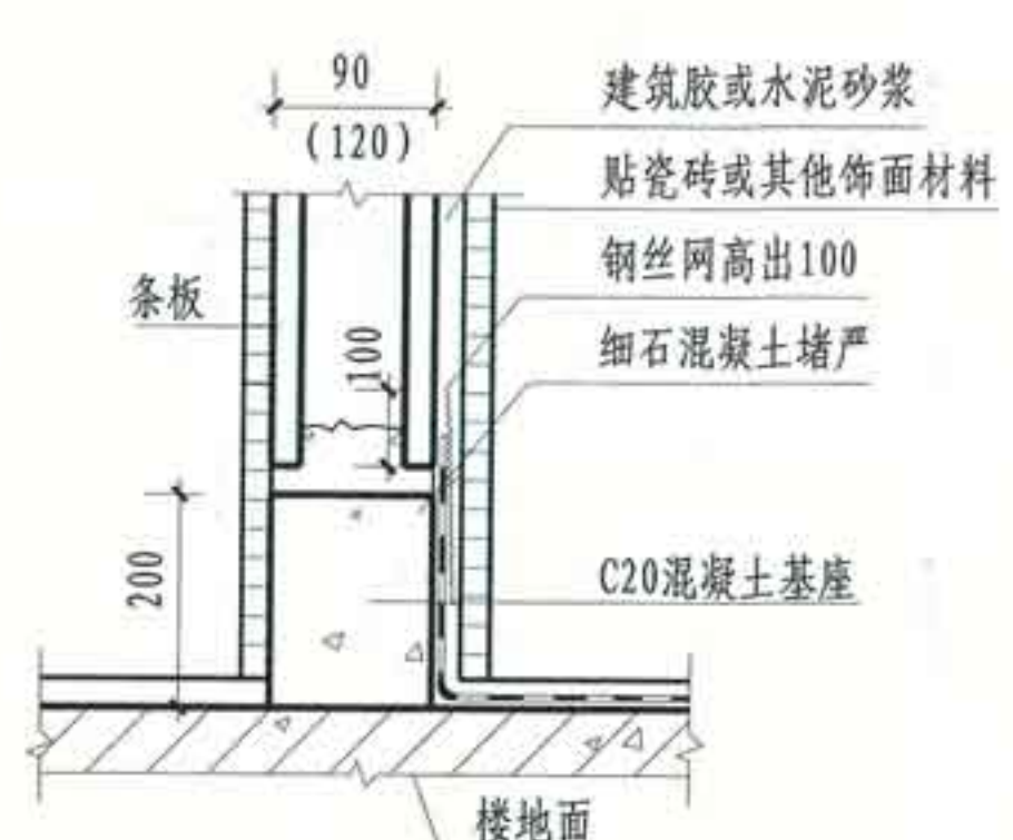
③ 条板与卫生间楼地面连接
