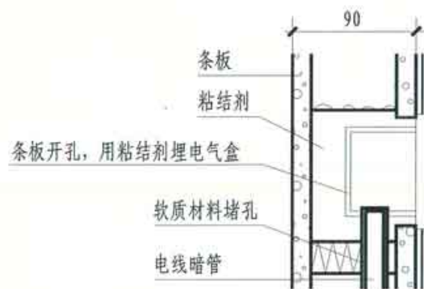
④ 暗线插座
