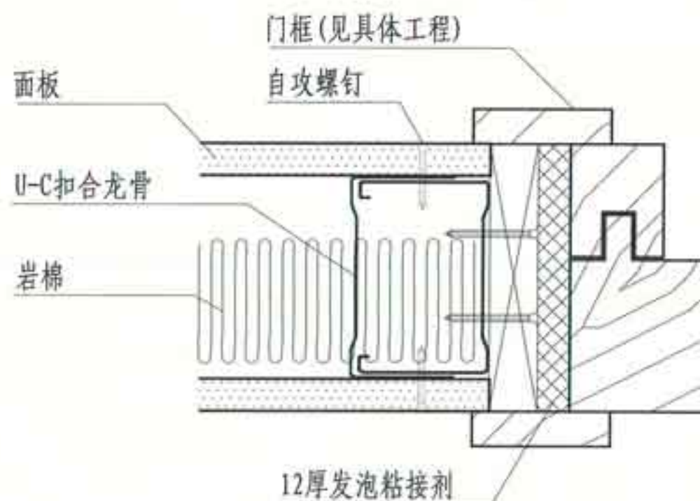
③ U-C扣合组合2
