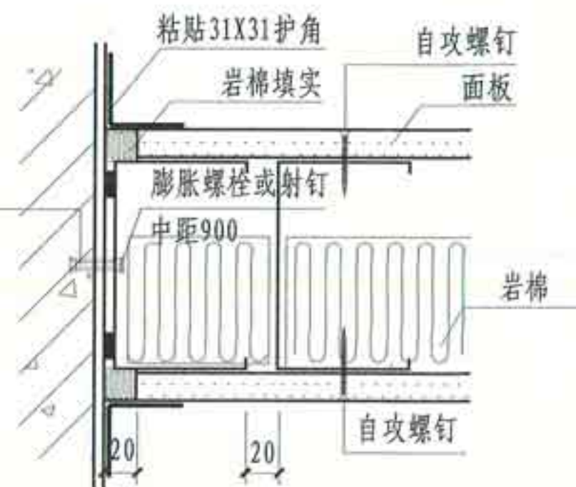
⑥ 滑动连接
