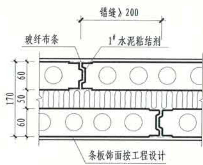
② 双层条板一字连接
