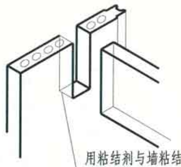
② 门上板与轻隔墙连接
