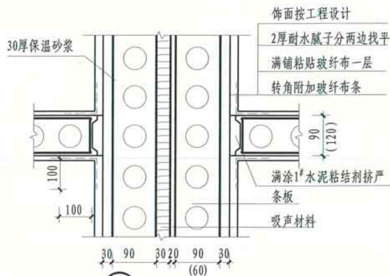
④ 双层条板隔墙 (分户墙保温)
