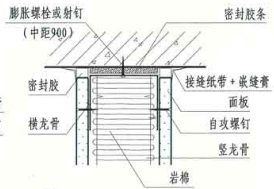
② 单层板、有隔音、带密封胶条
