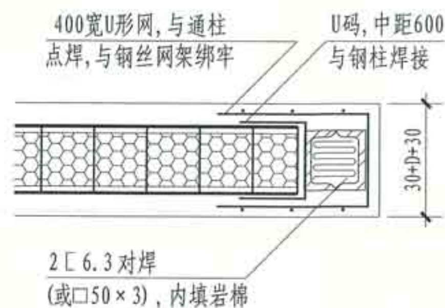
⑥ 板墙水平端构造
