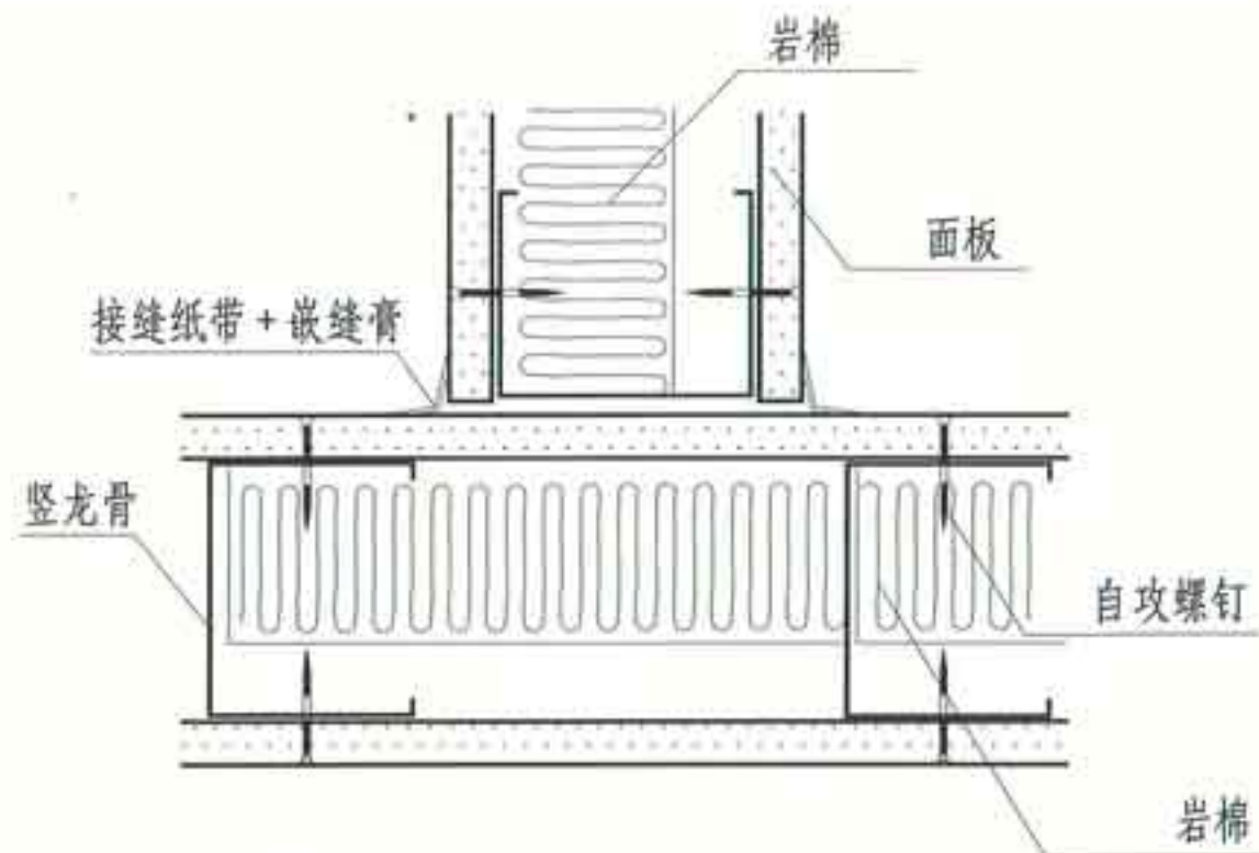
② T形 (二)
