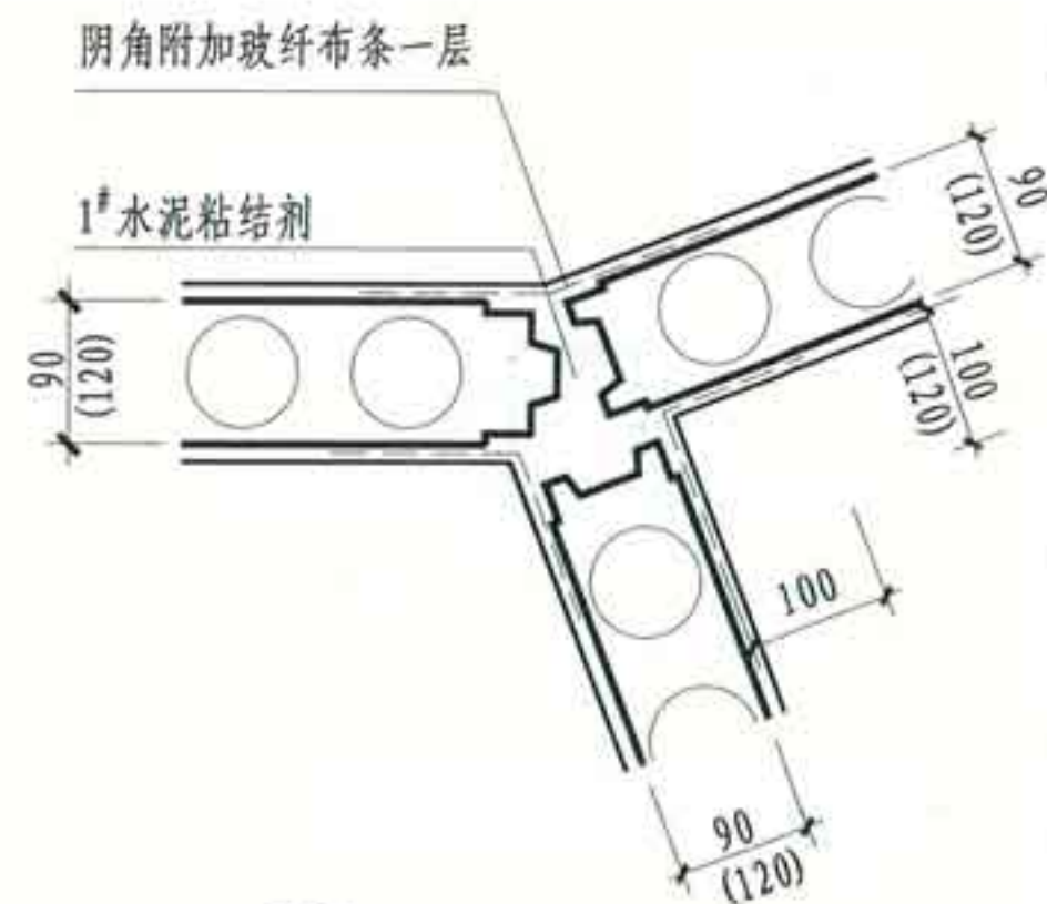
③ 条板Y字连接
