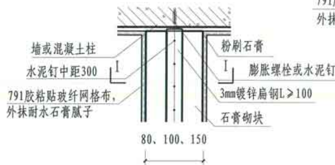
⑤ 木门框与钢筋混凝土柱连接 ⑥ 石膏砌块与墙(柱)连接构造
