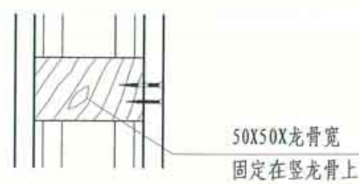
⑥ 吊挂件节点 (三)
