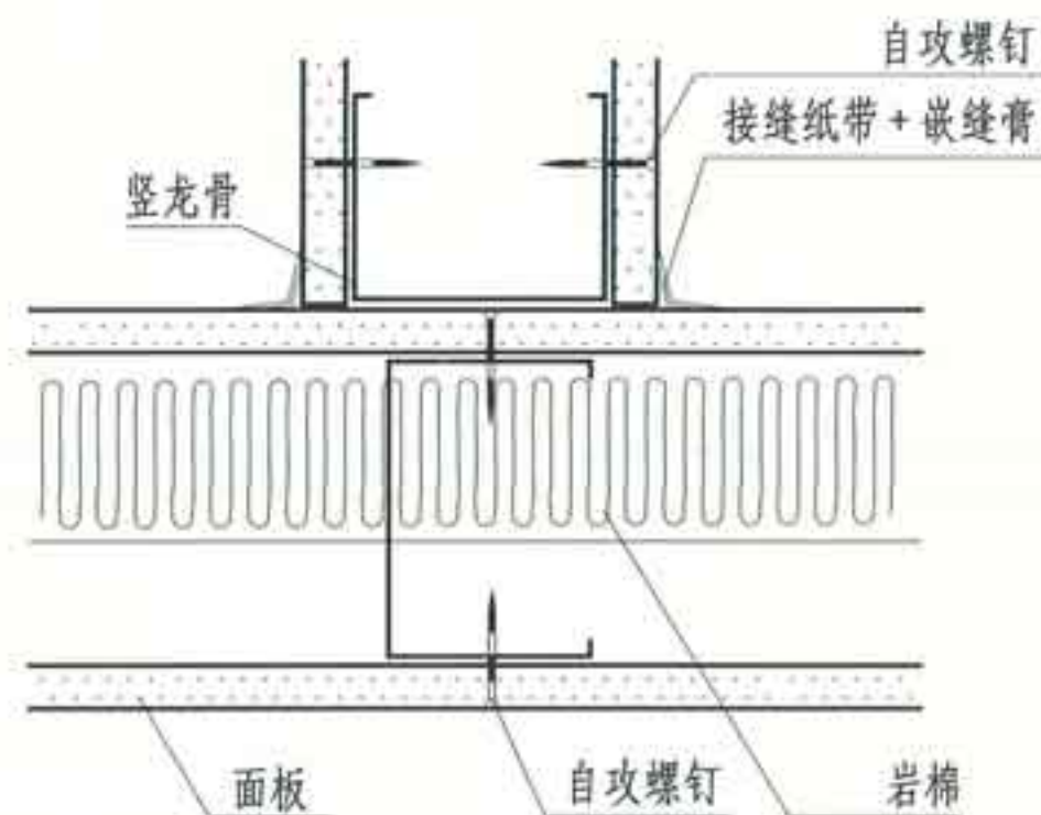
③ T形 (六)
