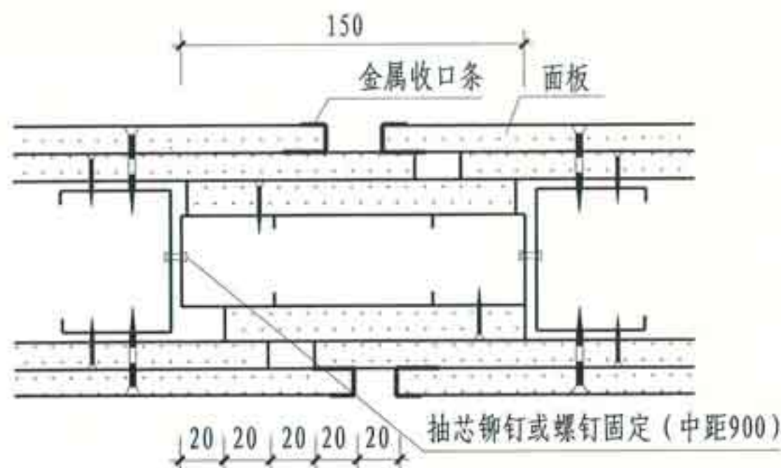
① 隔声墙伸缩缝
