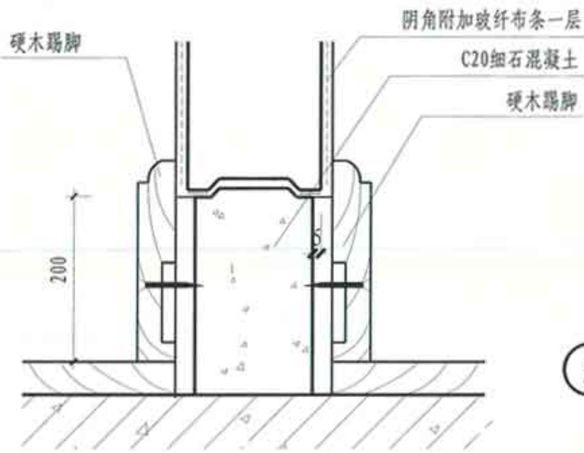
④ 砌块隔墙与楼、地面连接
