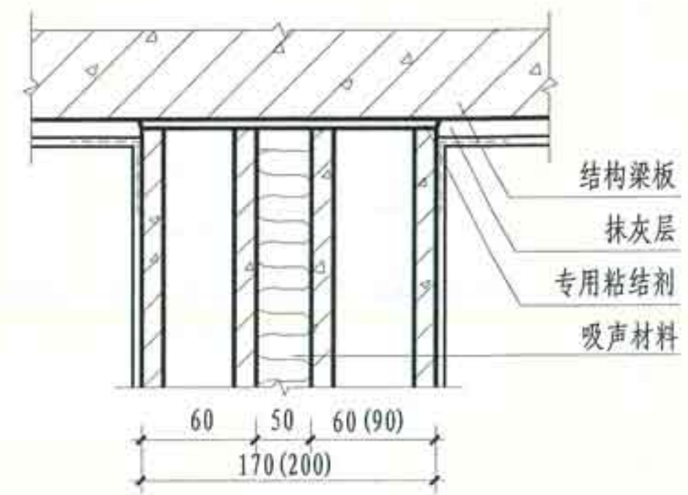
⑥ 双层条板与梁板连接
