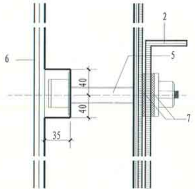
② 固定卫生洁具座桶水箱详图
