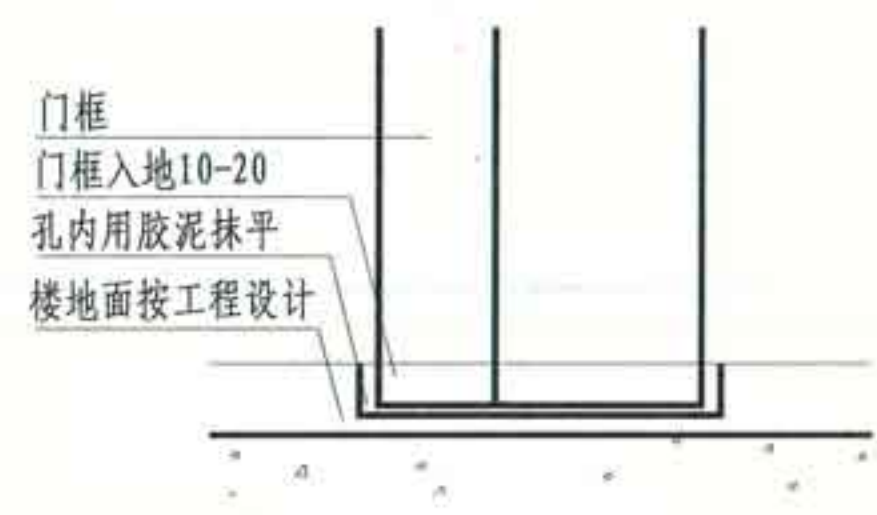
⑤ 门框入地连接
