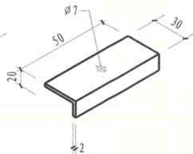
⑧ L型钢板卡
