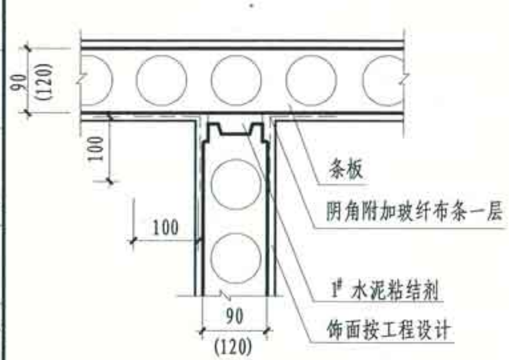
① 条板丁字连接
