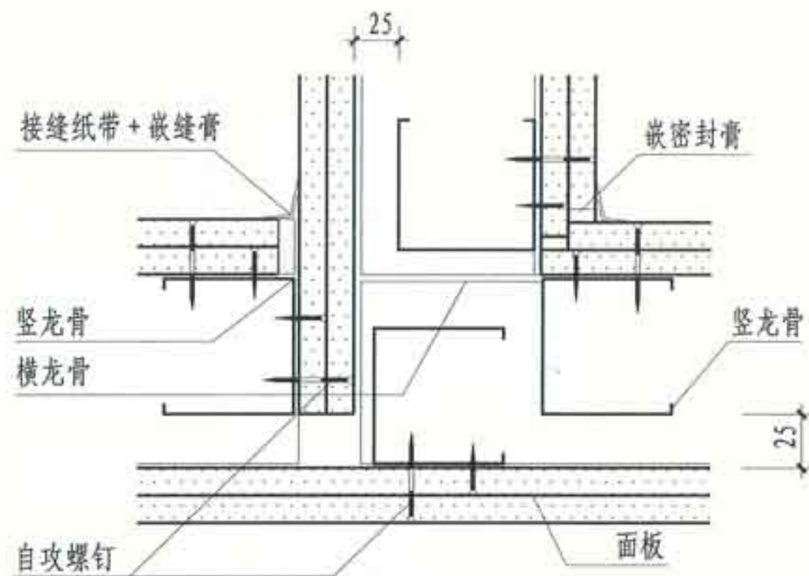
① T形 (五)
