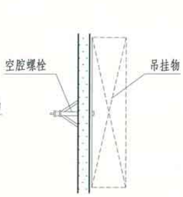
② 单板空腔螺栓吊挂
