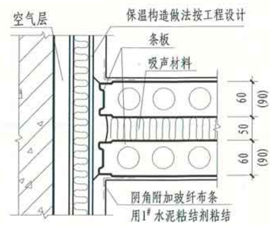
⑥ 双层条板与保温墙连接
