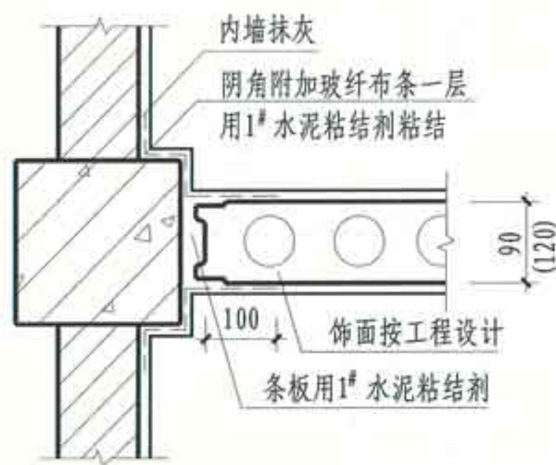
① 条板与墙、柱连接
