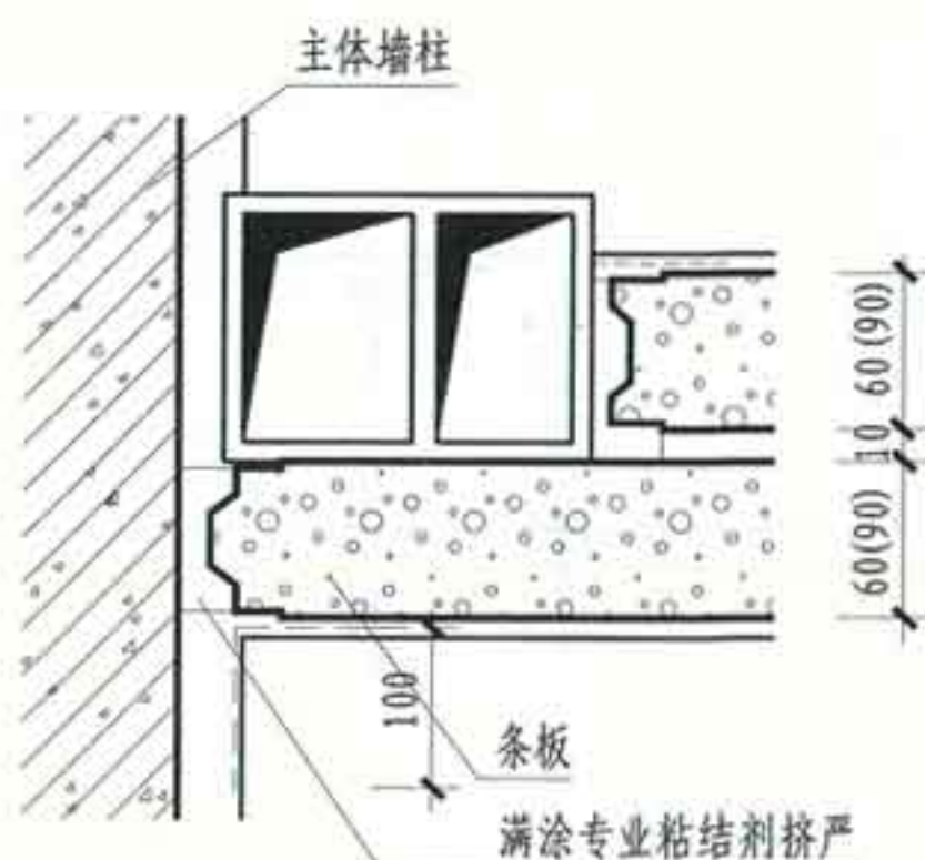
⑥ 双层条板与风道连接
