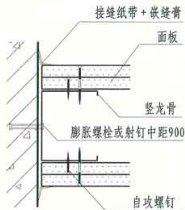
② 与结构墙（柱）连接
