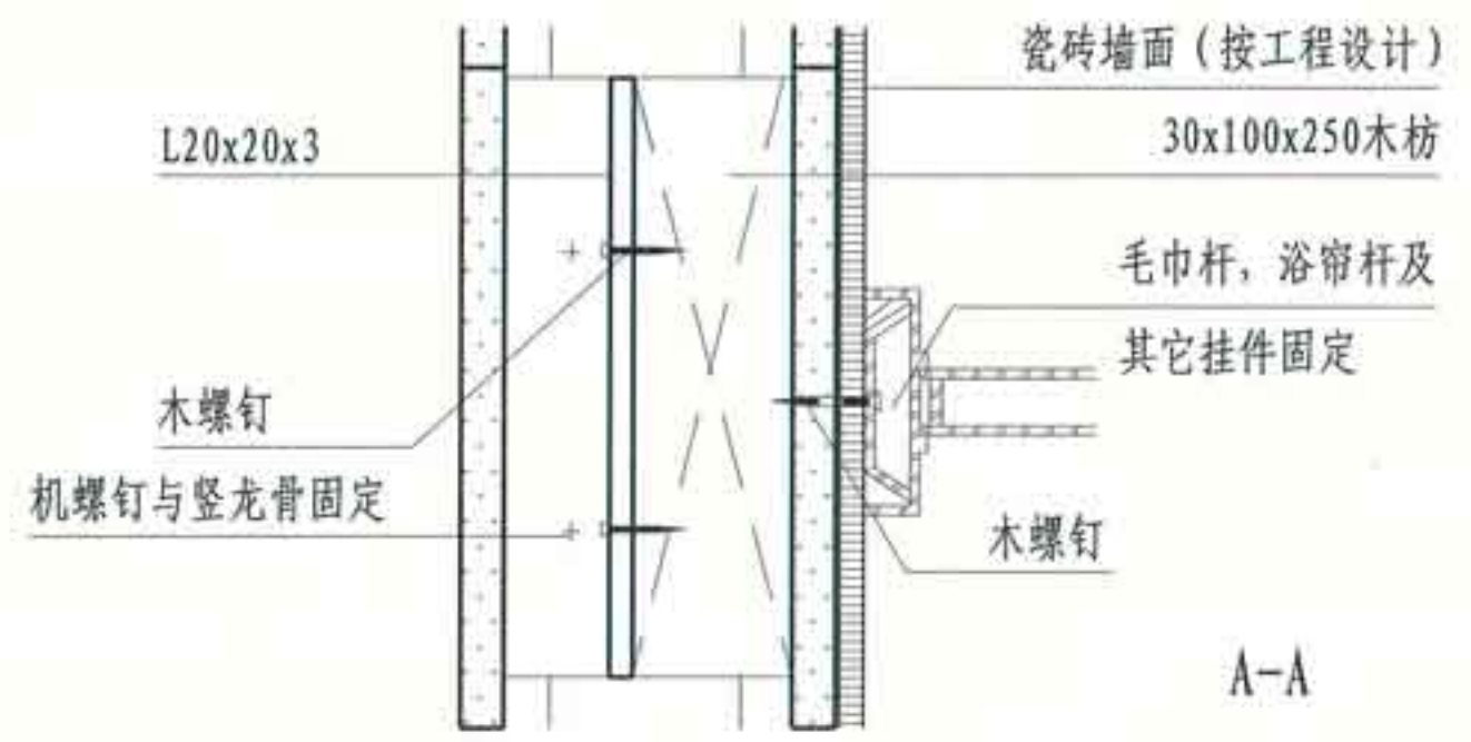
① 固定吊挂件之一
