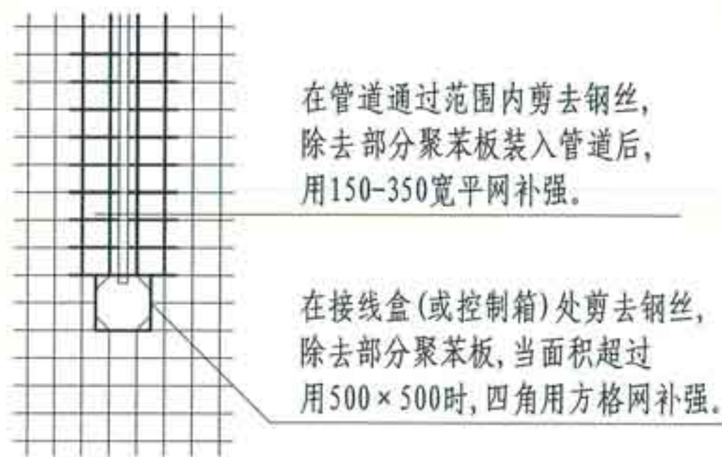
③ 预埋管线做法
