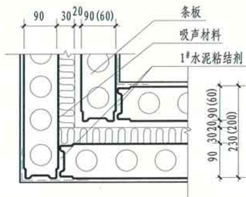
① 条板隔声墙直角连接
