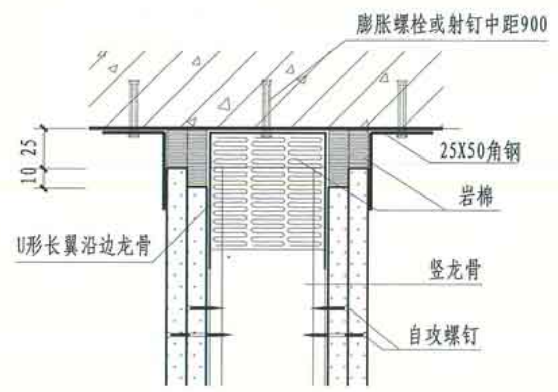
③ 滑动连接
