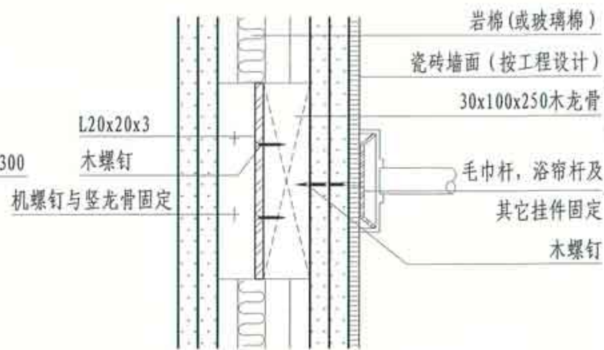
③ 与杆件连接
