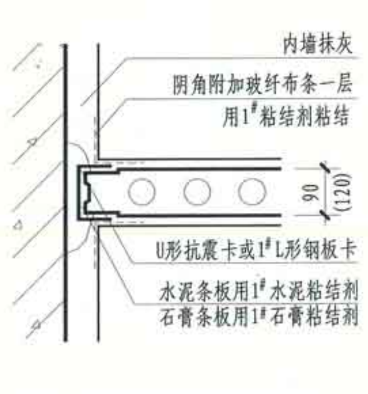
④ 条板与结构墙、柱连接
