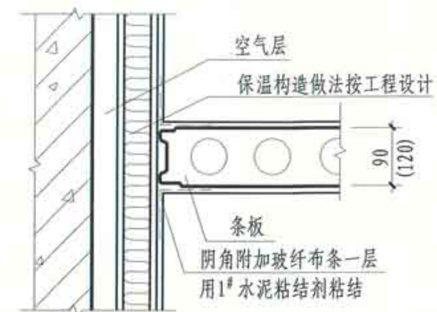
③ 条板与保温墙连接
