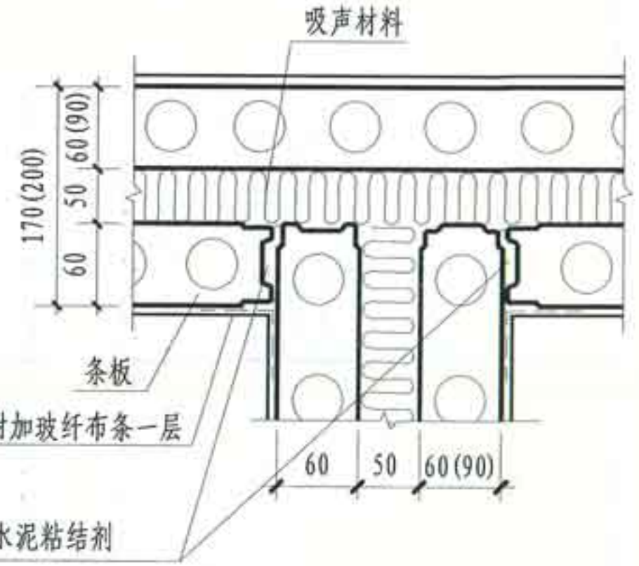
③ 条板隔声墙直角连接
