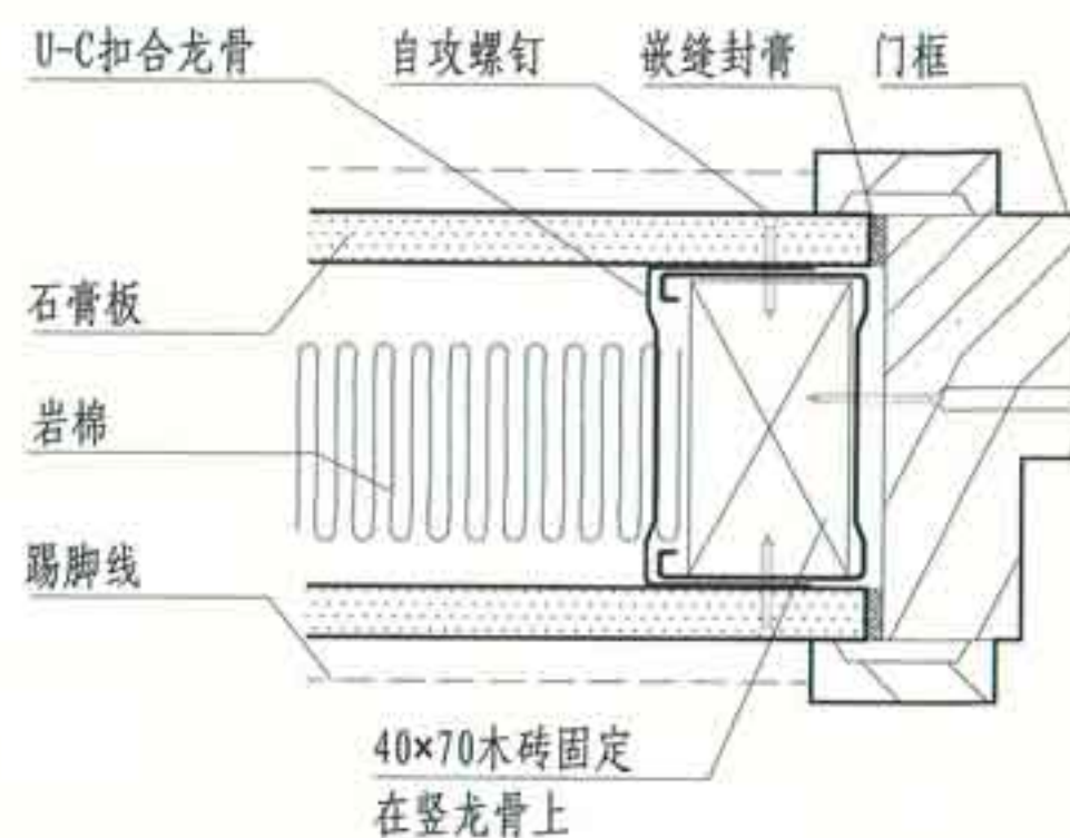
② U-C扣合组合1
