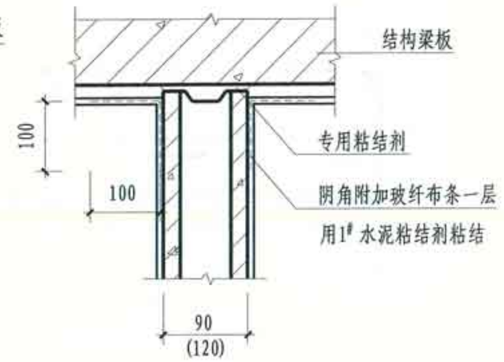
⑤ 条板门窗上横板与梁板连接
