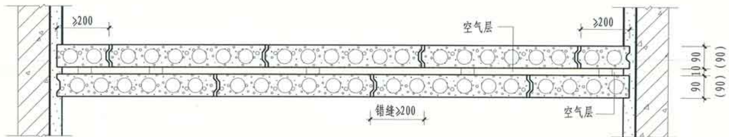
双层空心硅镁加气、粉煤灰泡沫水泥条板内隔墙平面
