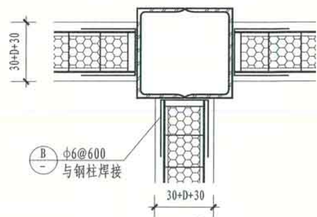
④ 丁字墙连接构造(四)
