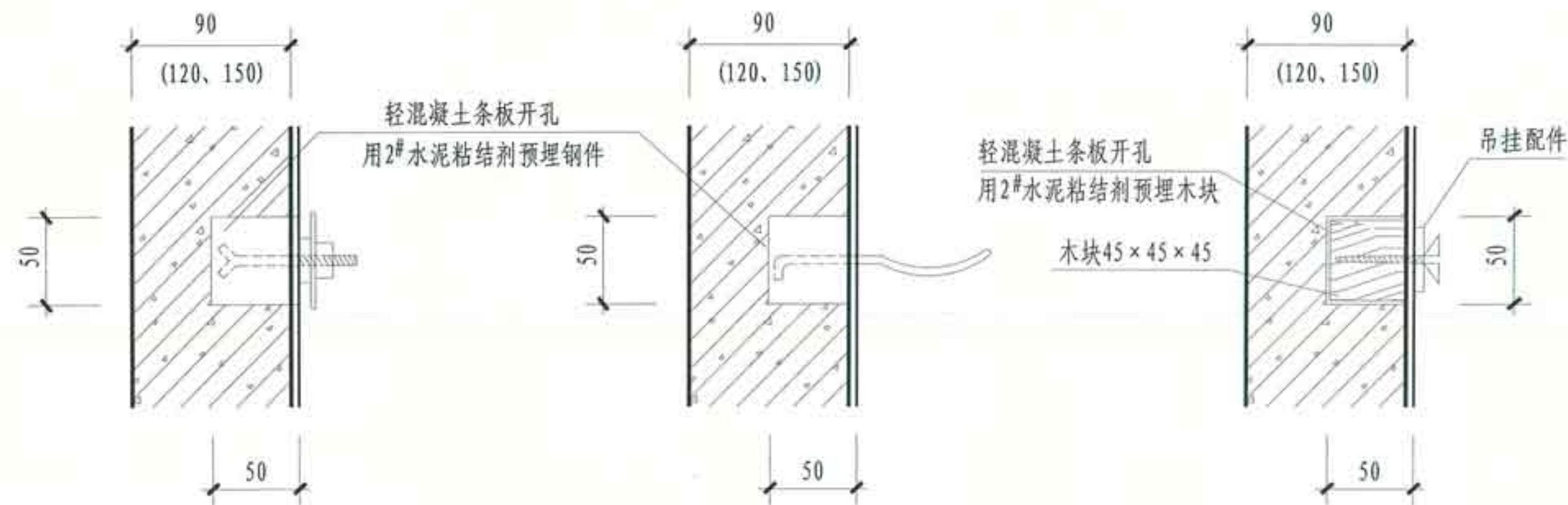
④ 轻集料混凝土条板钢吊挂件
