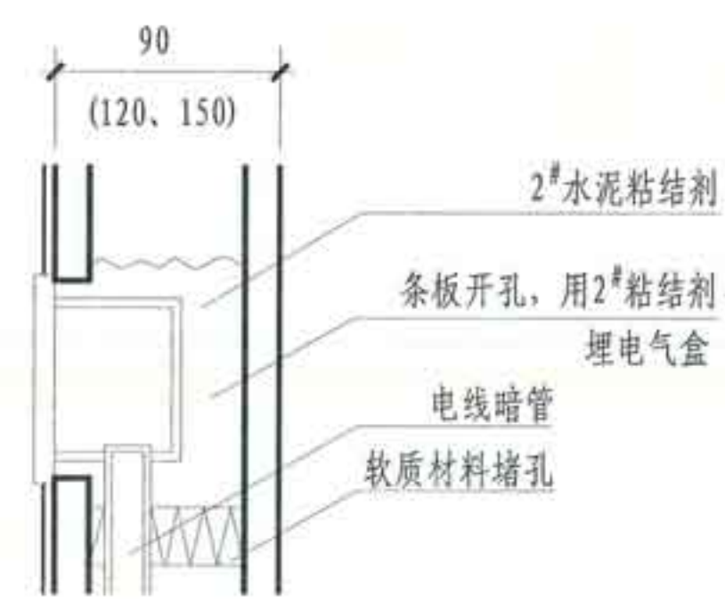
④ 暗线插座
