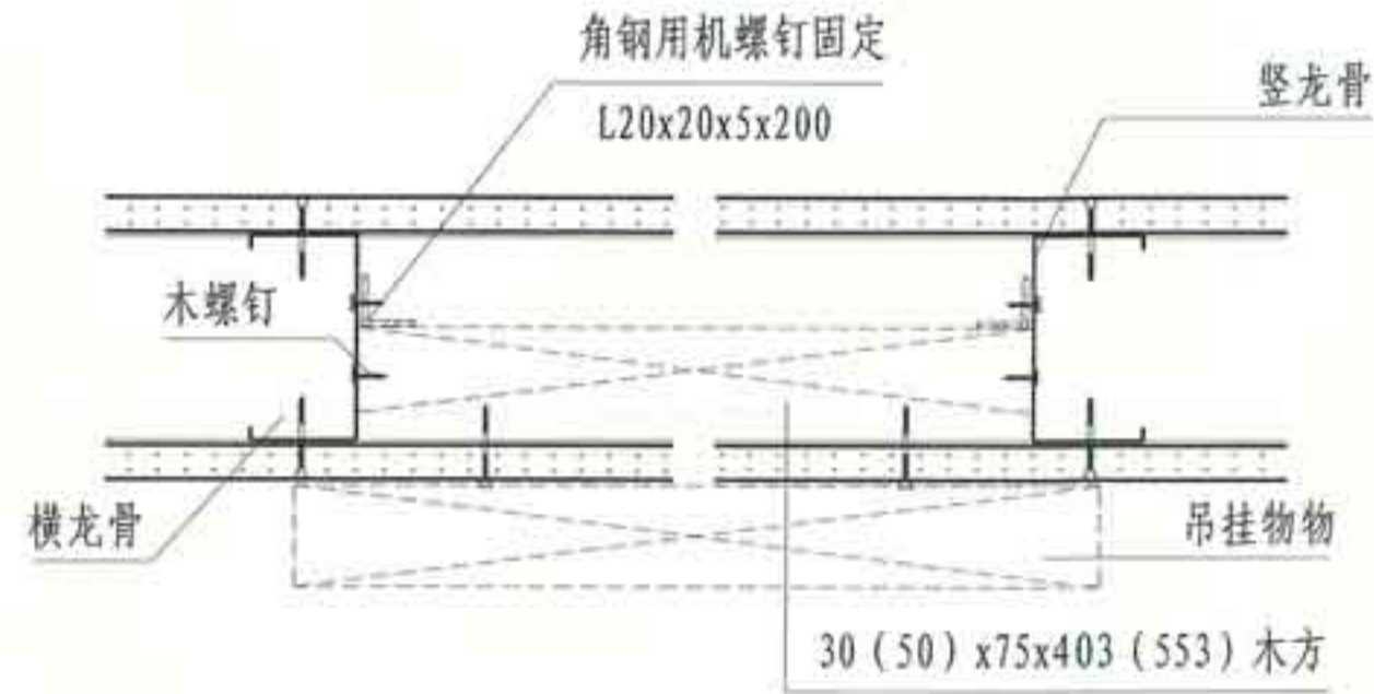
⑦ 木方吊挂 (吊挂重量35-50kg)
