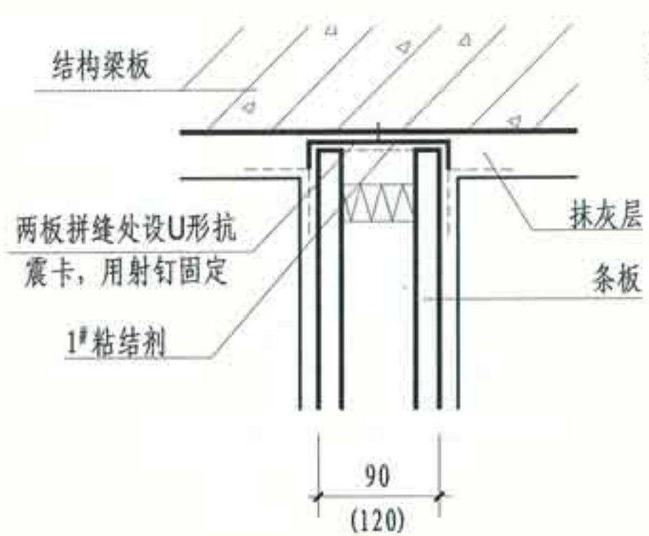
① 条板与结构梁、板连接
