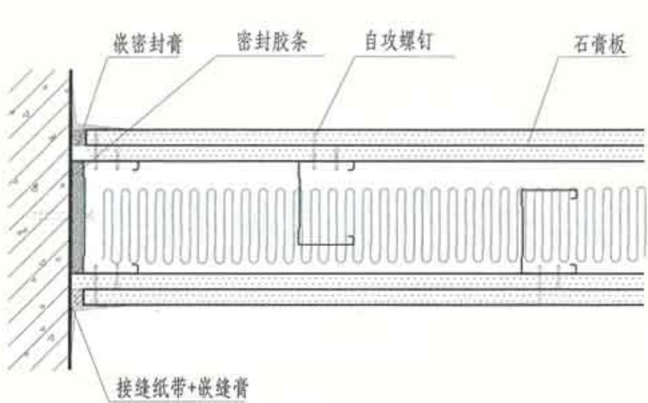
① 双排错位龙骨隔墙（有较高隔声要求）
