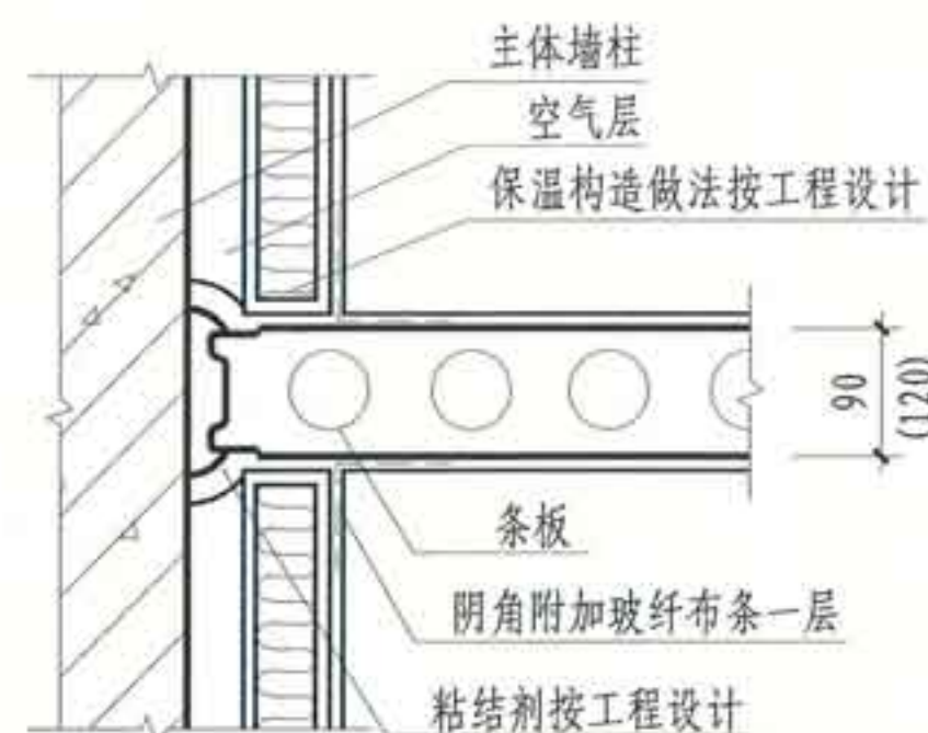
② 条板与保温墙连接
