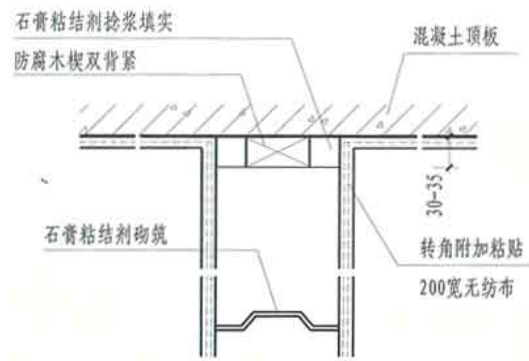
① 砌块隔墙与混凝土顶板连接
