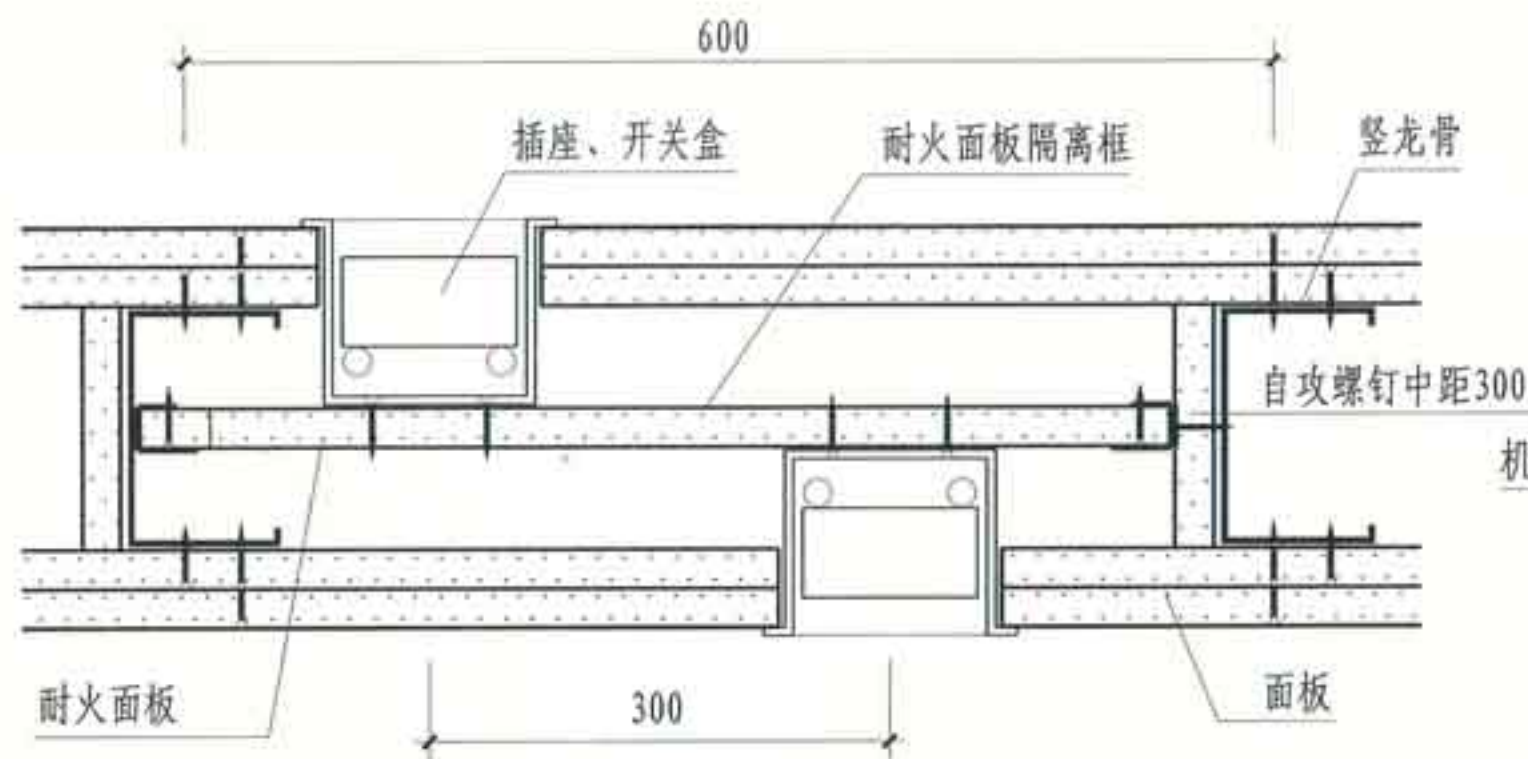
① 插座、开关盒（有防火要求）
