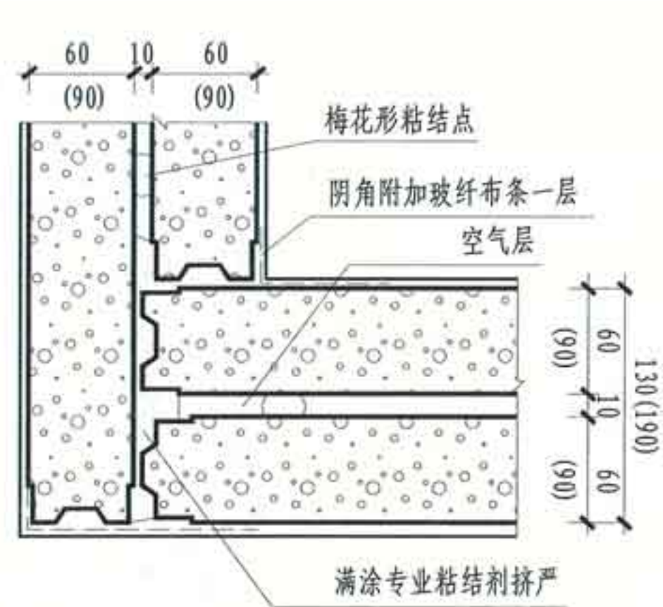
② 双层条板直角连接
