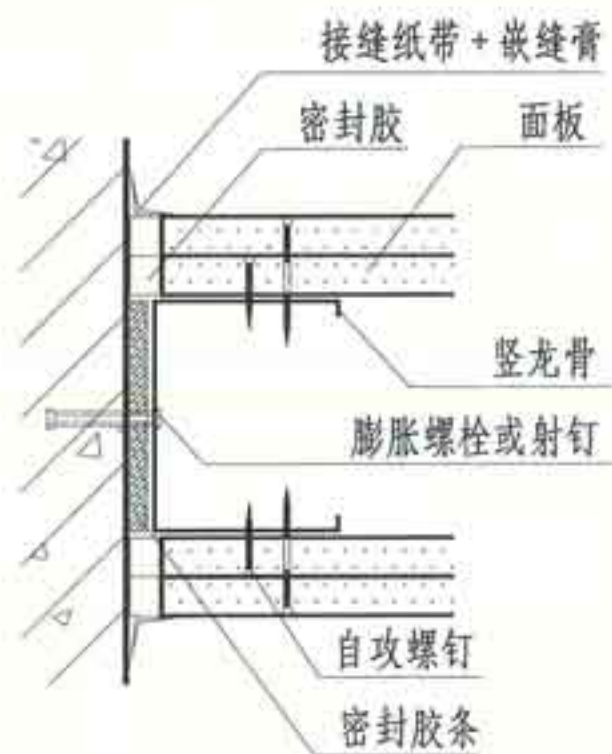
③ 与结构墙（柱）连接
