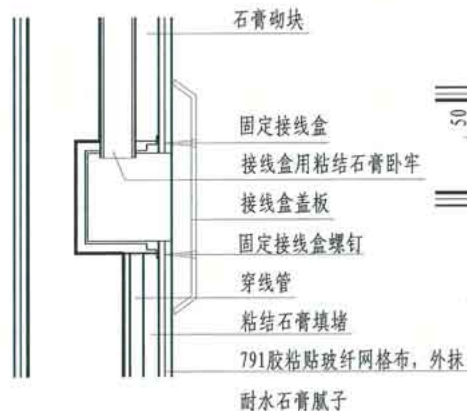
① 接线盒、开关盒安装
