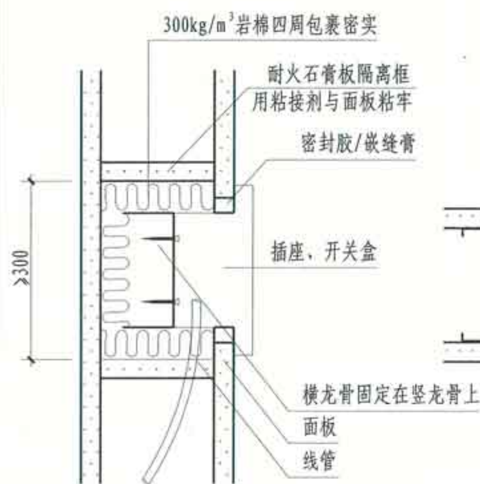
① 与插座、开关连接
