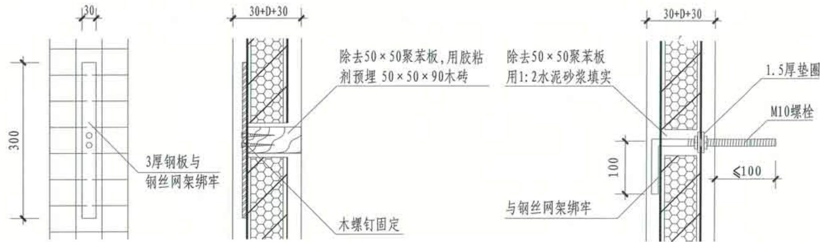
② 预埋螺栓构造
