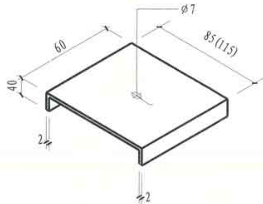
⑦ U型钢板卡
