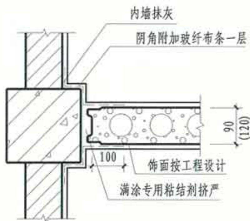
① 条板与墙柱连接
