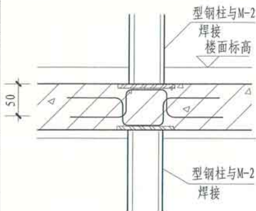
① 加劲柱与楼板(梁)连接构造
