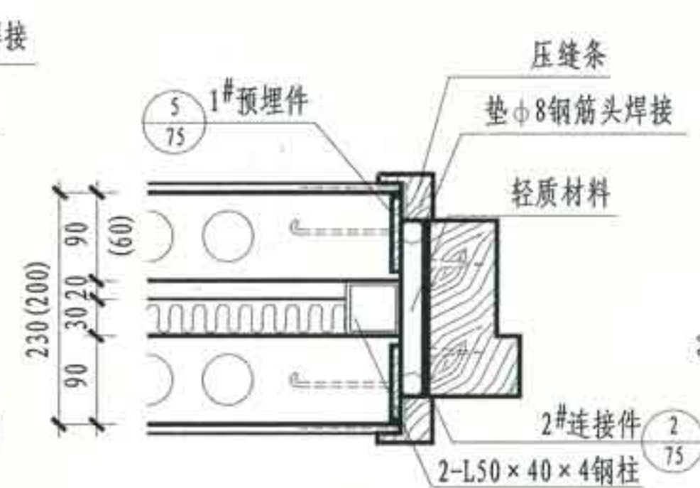
② 双层条板与钢柱、木门窗框连接
