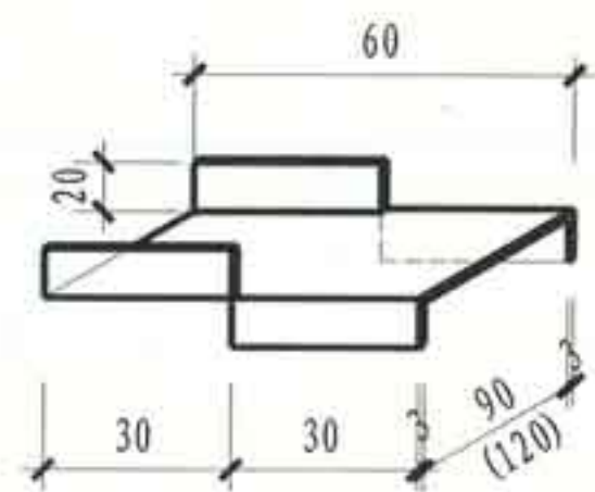
A 万字形铁固件
