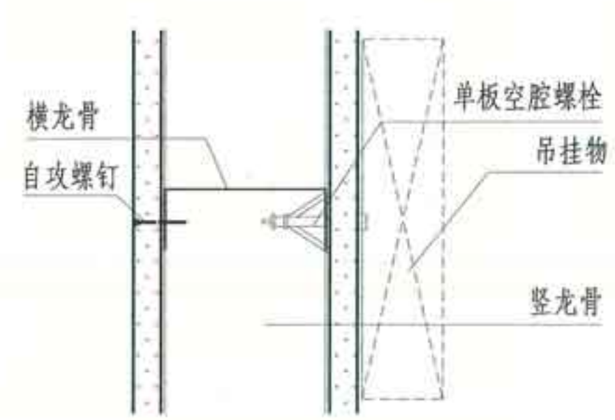
⑤ 横龙骨吊挂
