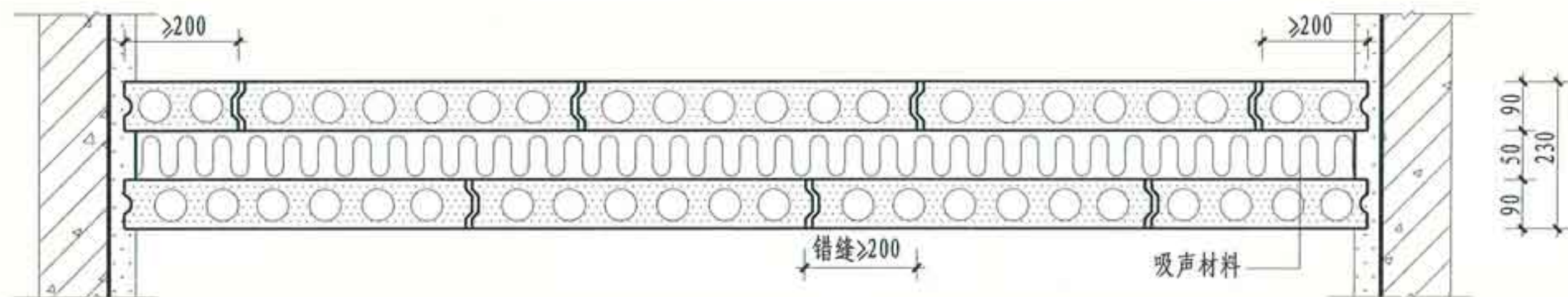
双层水泥、石膏、轻集料混凝土条板隔声墙平面一
