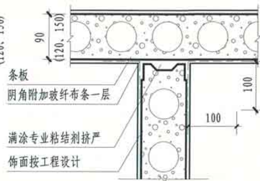
③ 条板丁字连接
