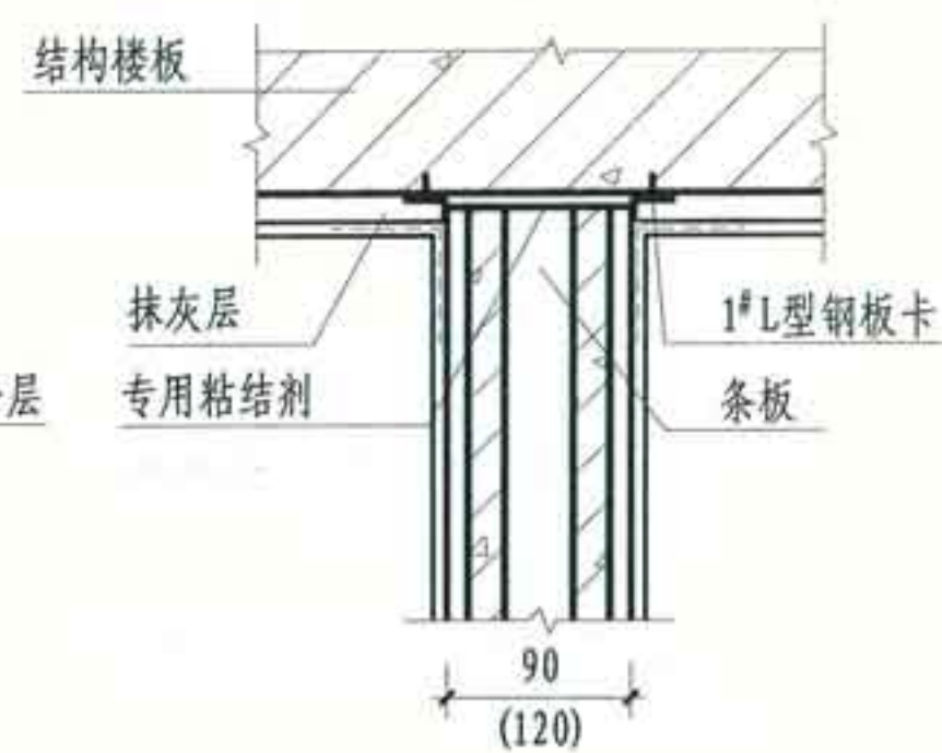
② 条板与楼板底面连接
