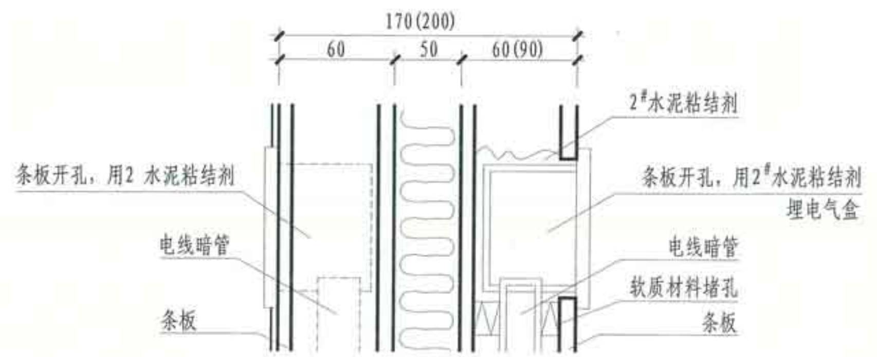
⑤ 暗线插座
