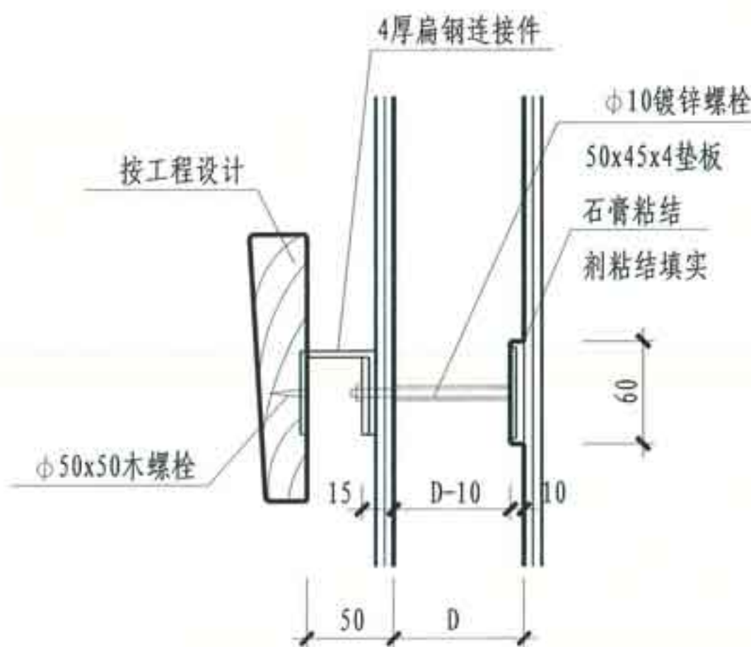
④ 靠墙扶手安装
