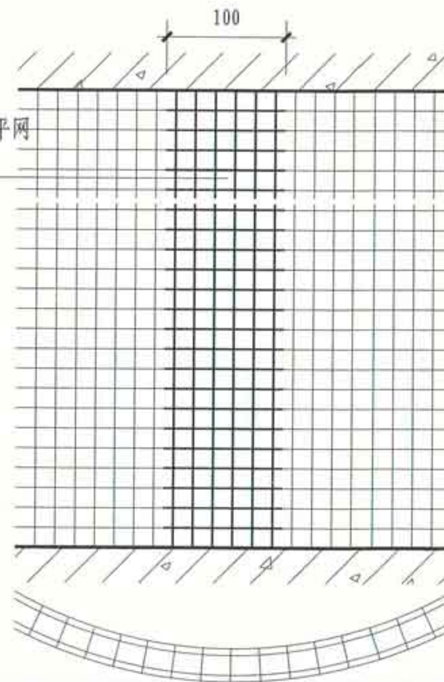
R > 500\text{cm} 弧面墙补强 (双面)
