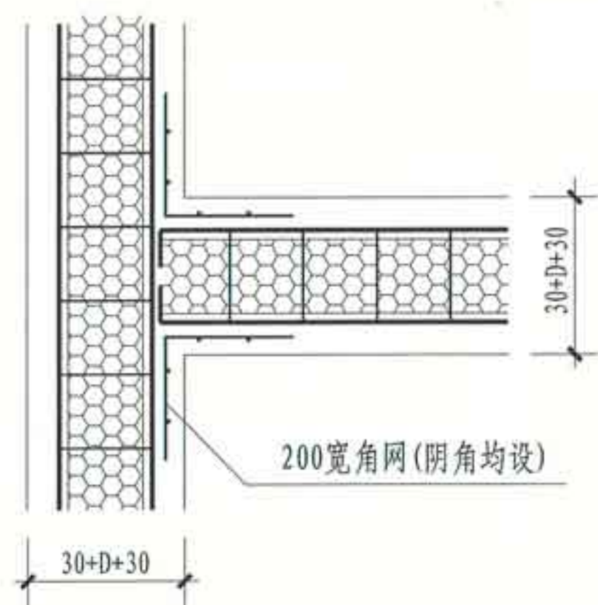
① 板墙与板墙丁字连接构造
