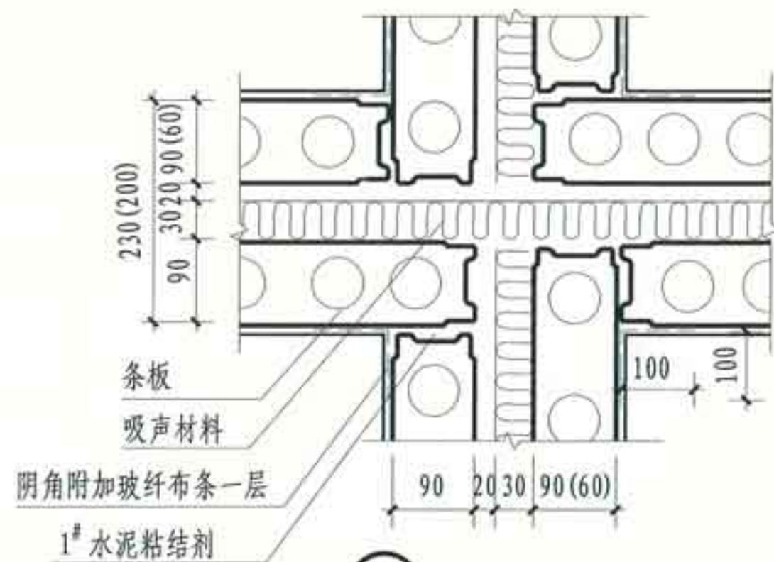
② 条板隔声墙十字连接
