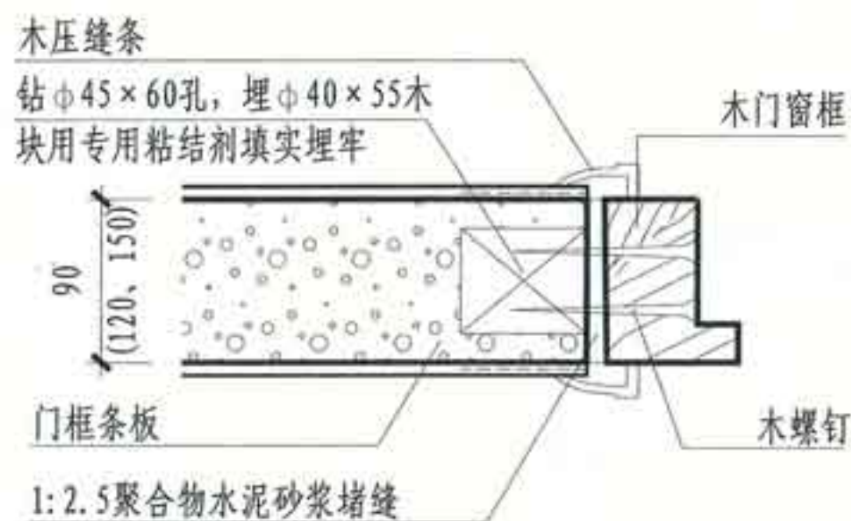
① 条板与木门窗框连接
