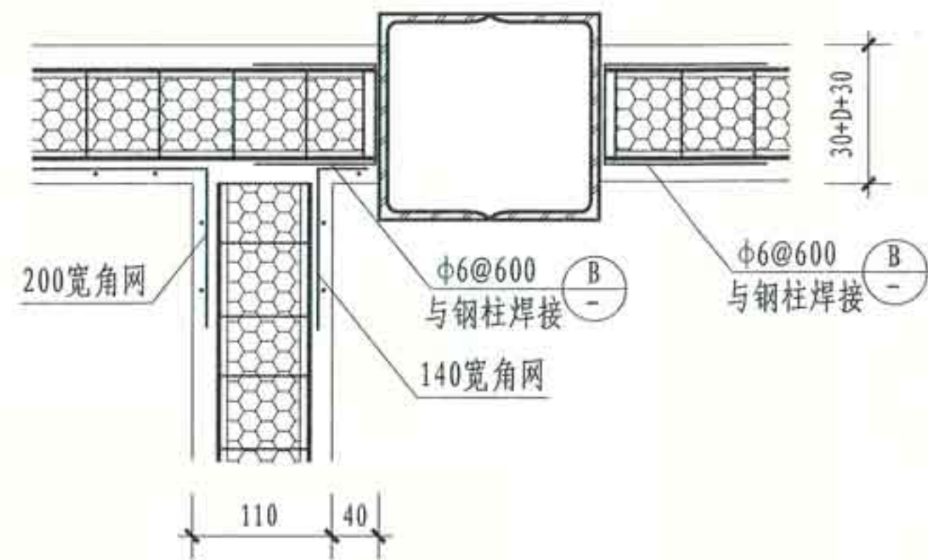
② 丁字墙连接构造(二)
