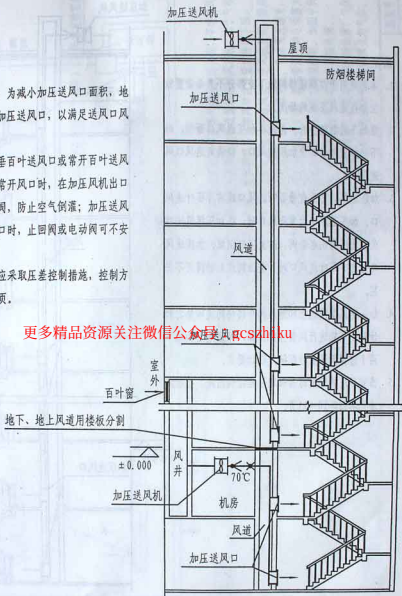
剖面示意图
