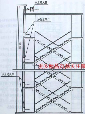
剖面示意图
