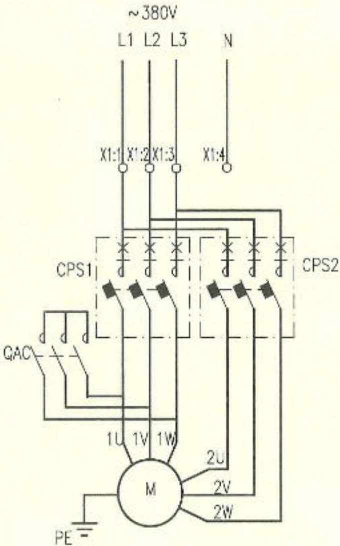
主回路
