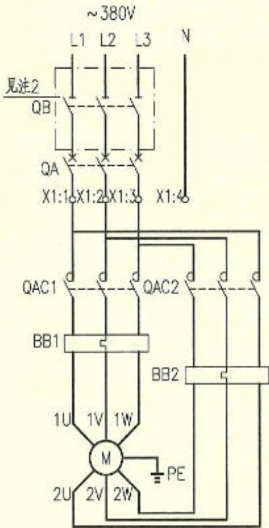
主回路
