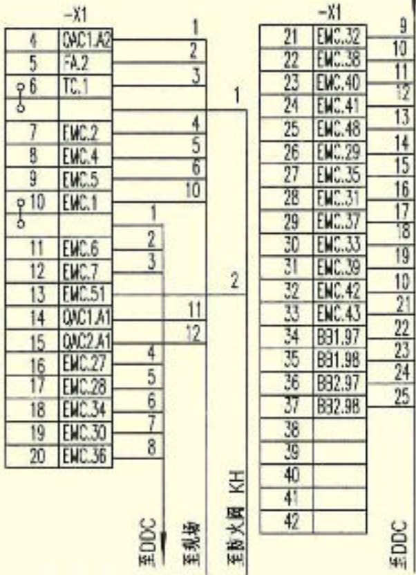
外部接线端子图
