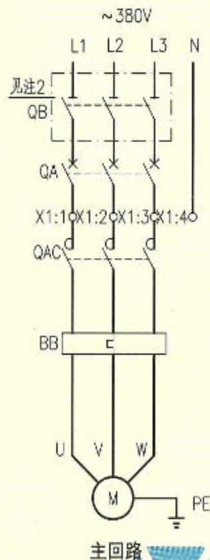
外部接线端子图
