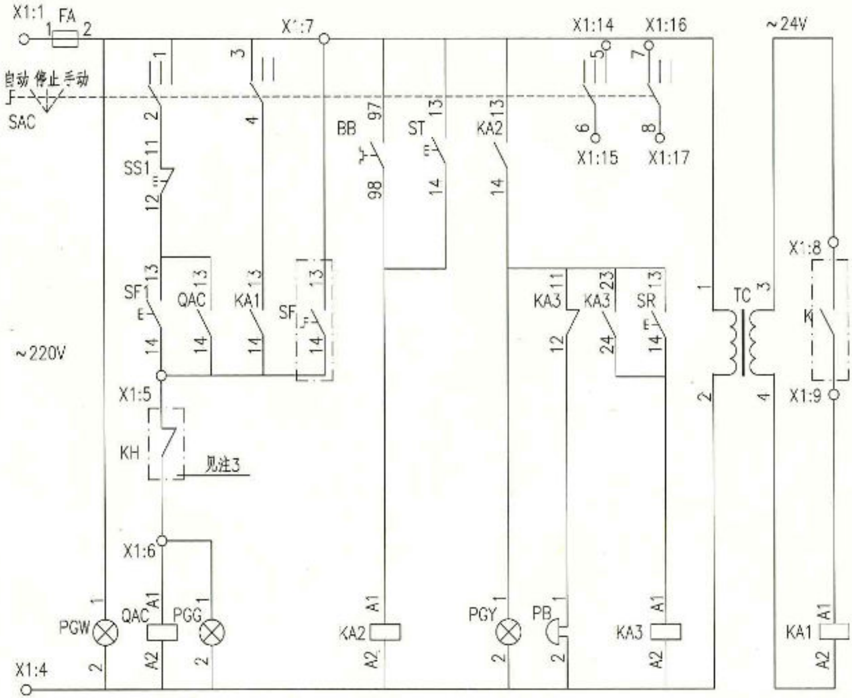
控制原理图
