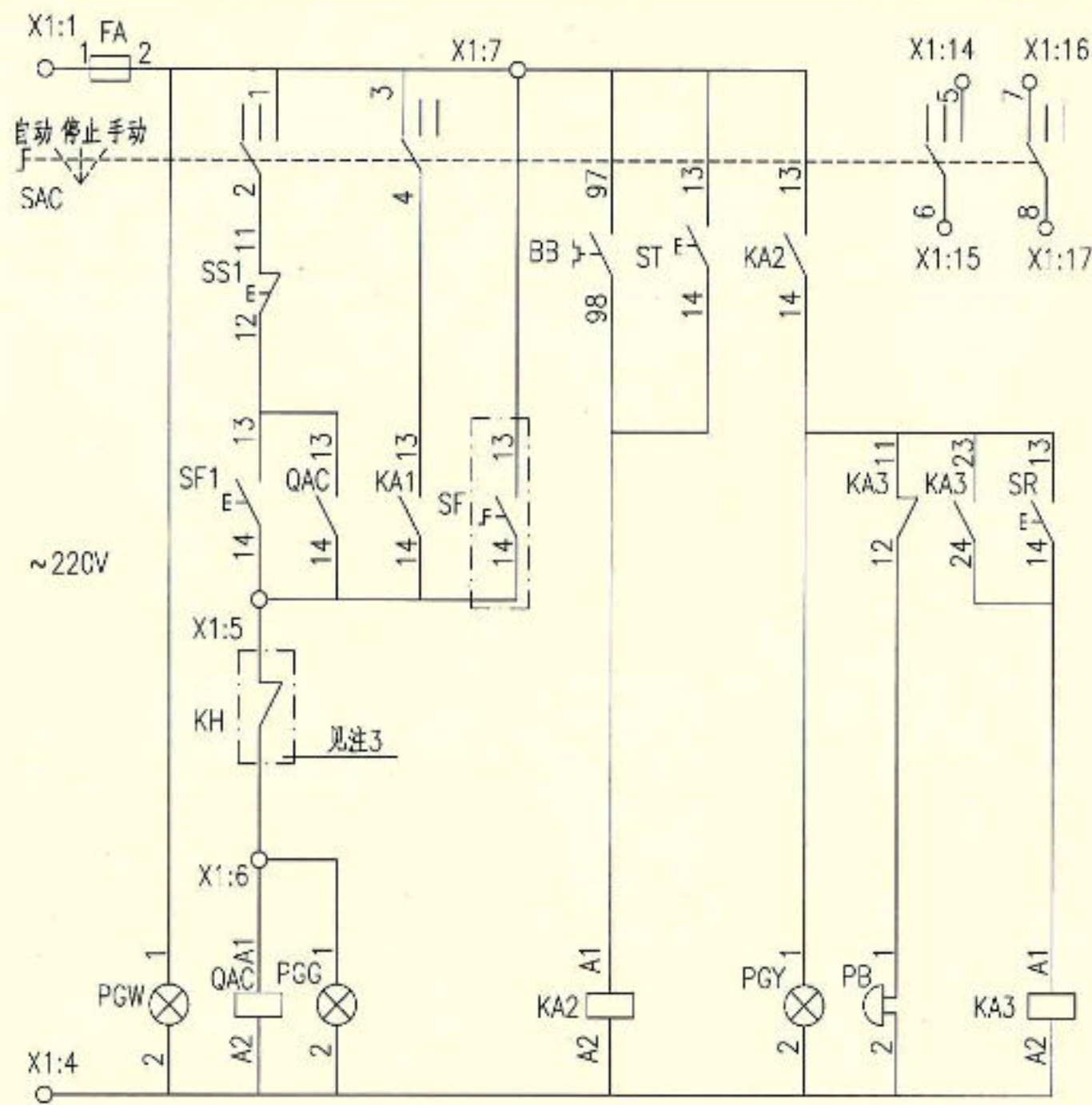
控制原理图
