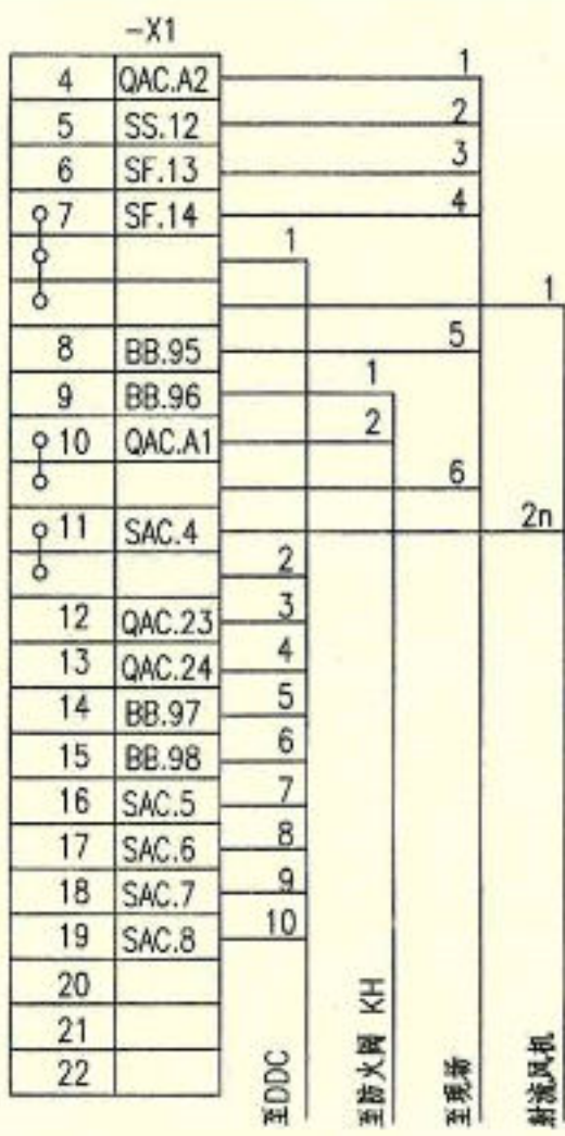
外部接线端子图
