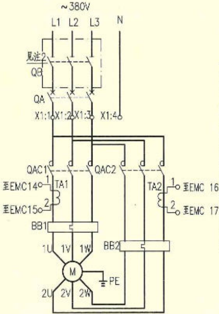
主回路
