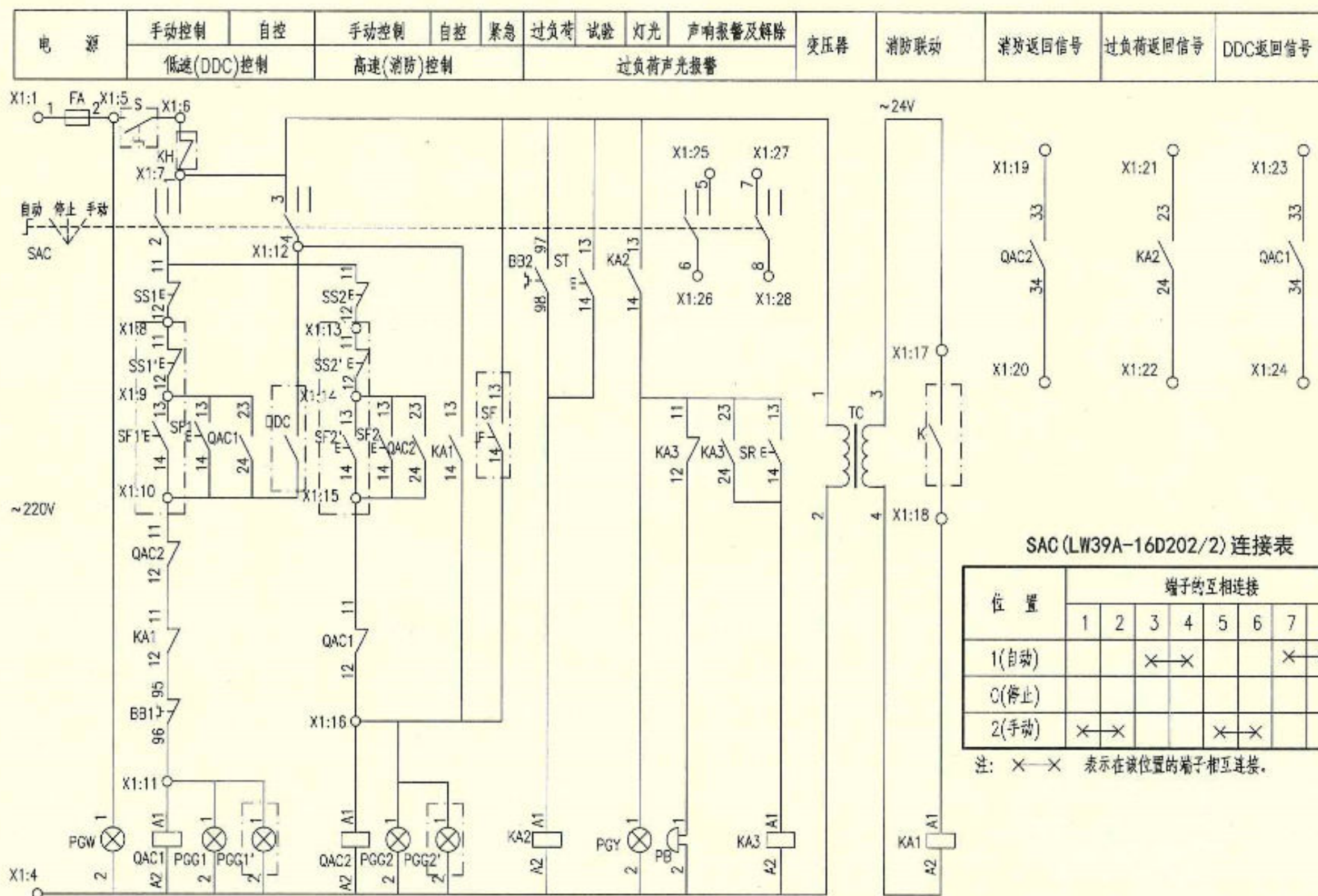
控制原理图
