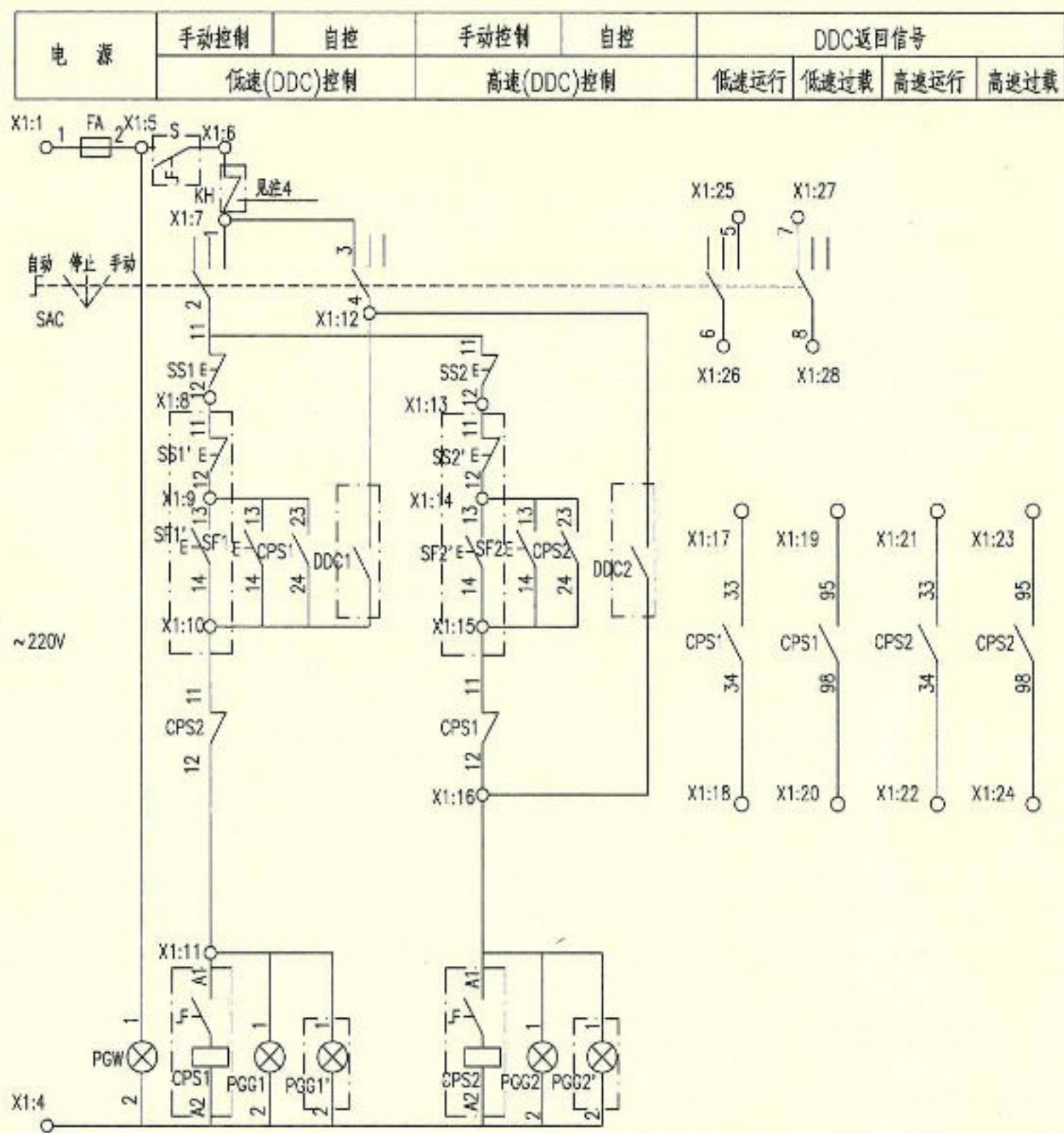
控制原理图
