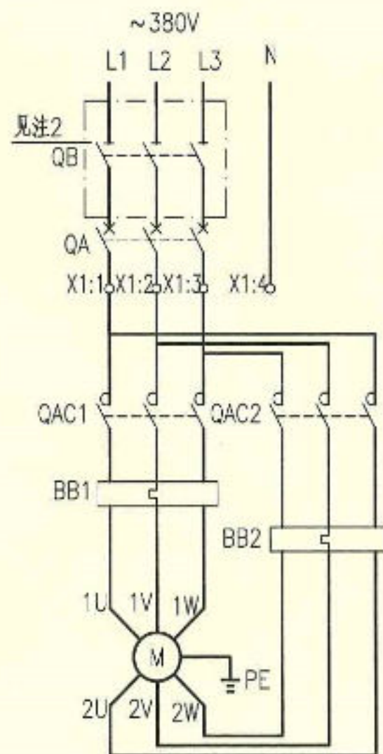
主回路
