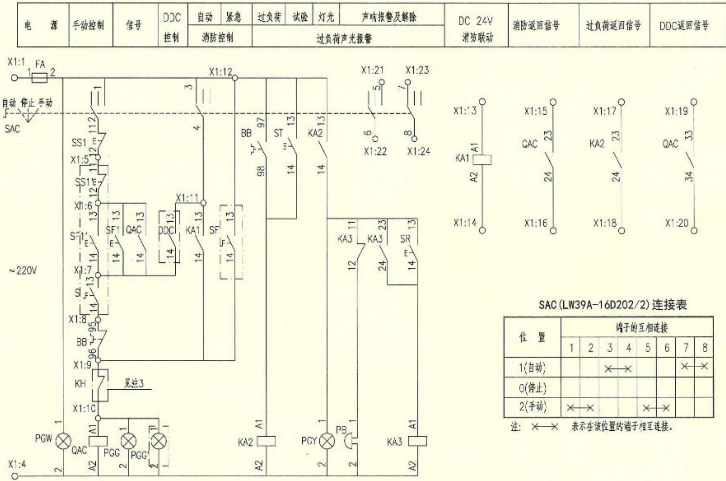
控制原理图
