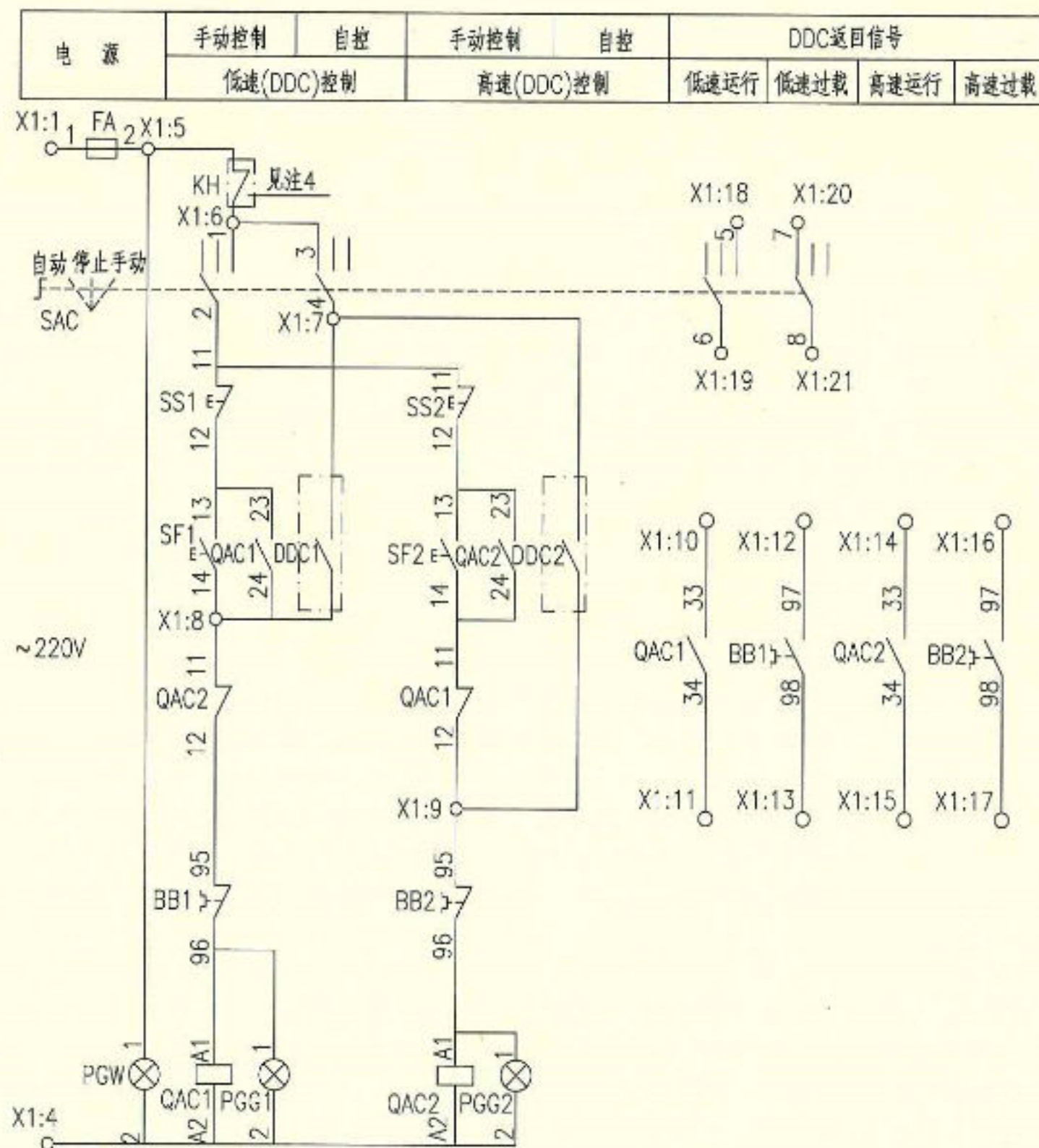
控制原理图
