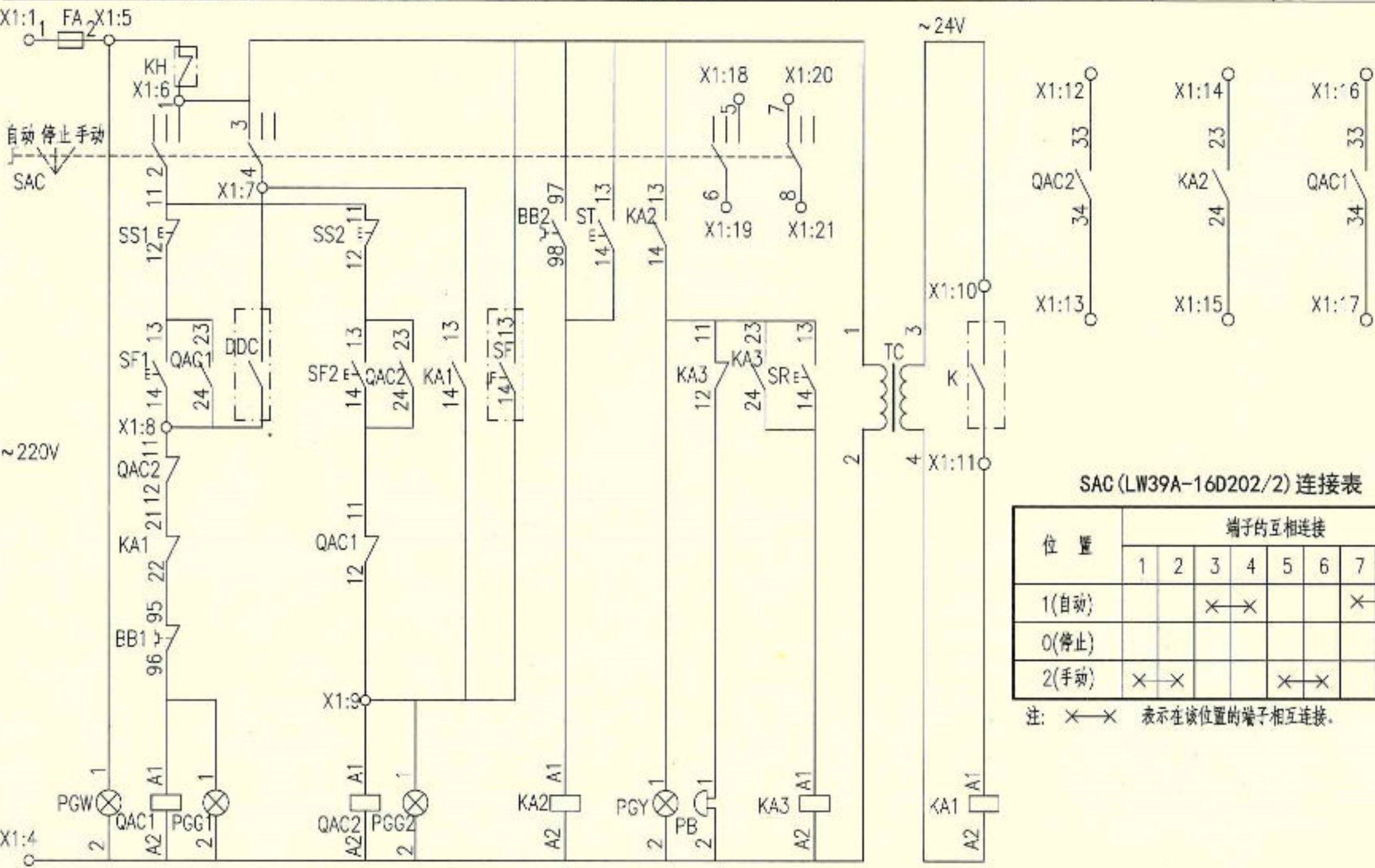
控制原理图
