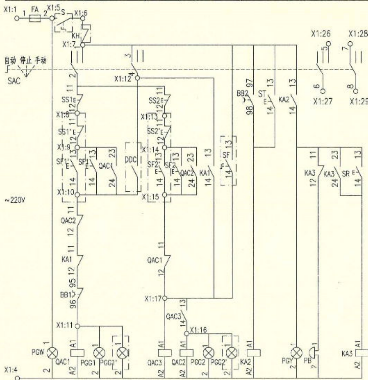
控制原理图
