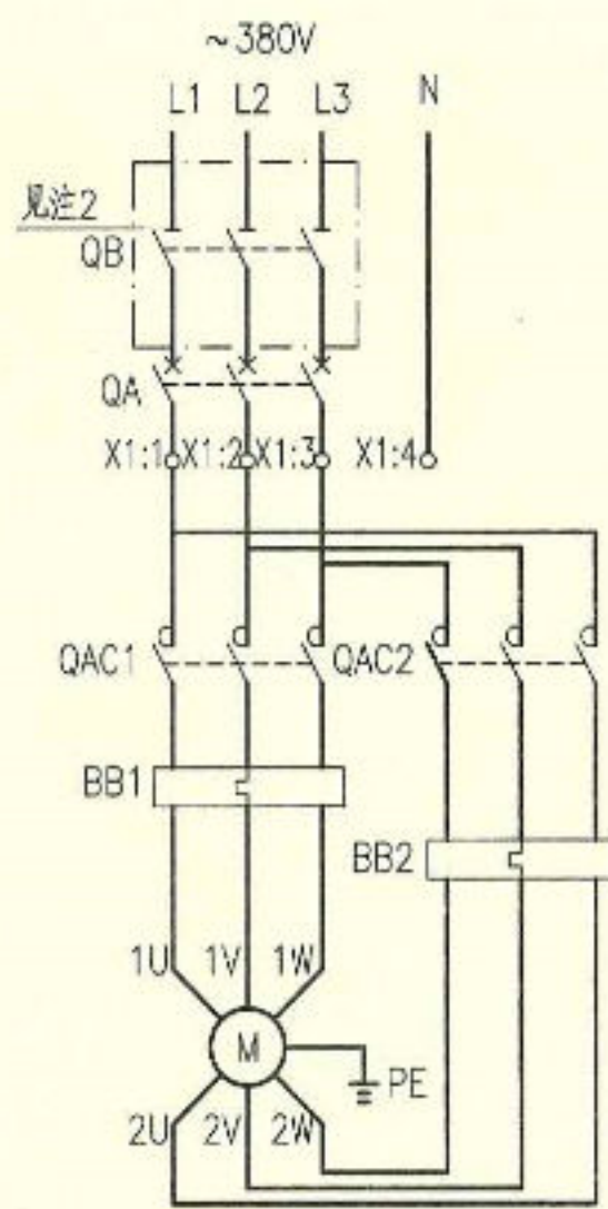
主回路
