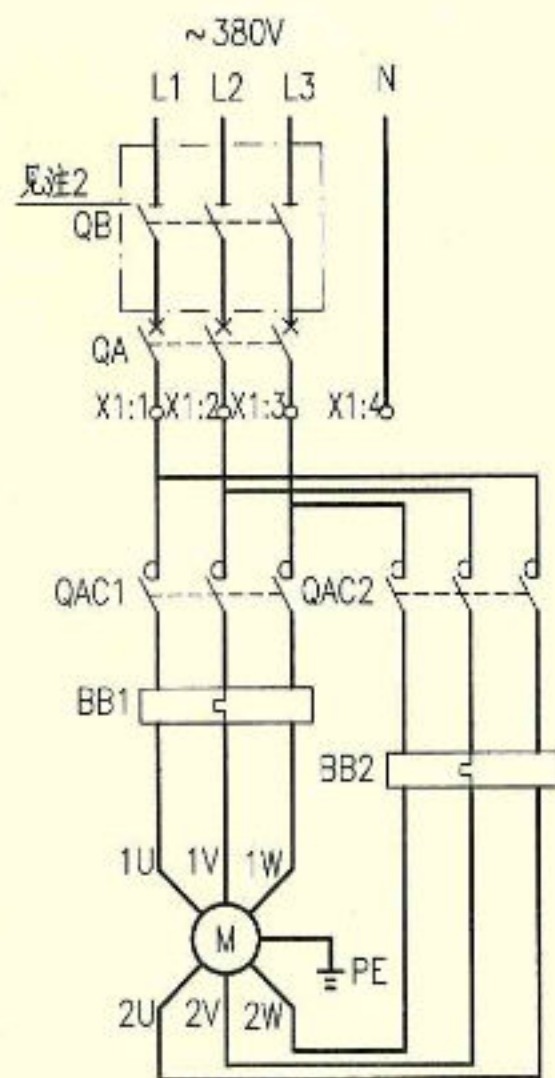
主回路
