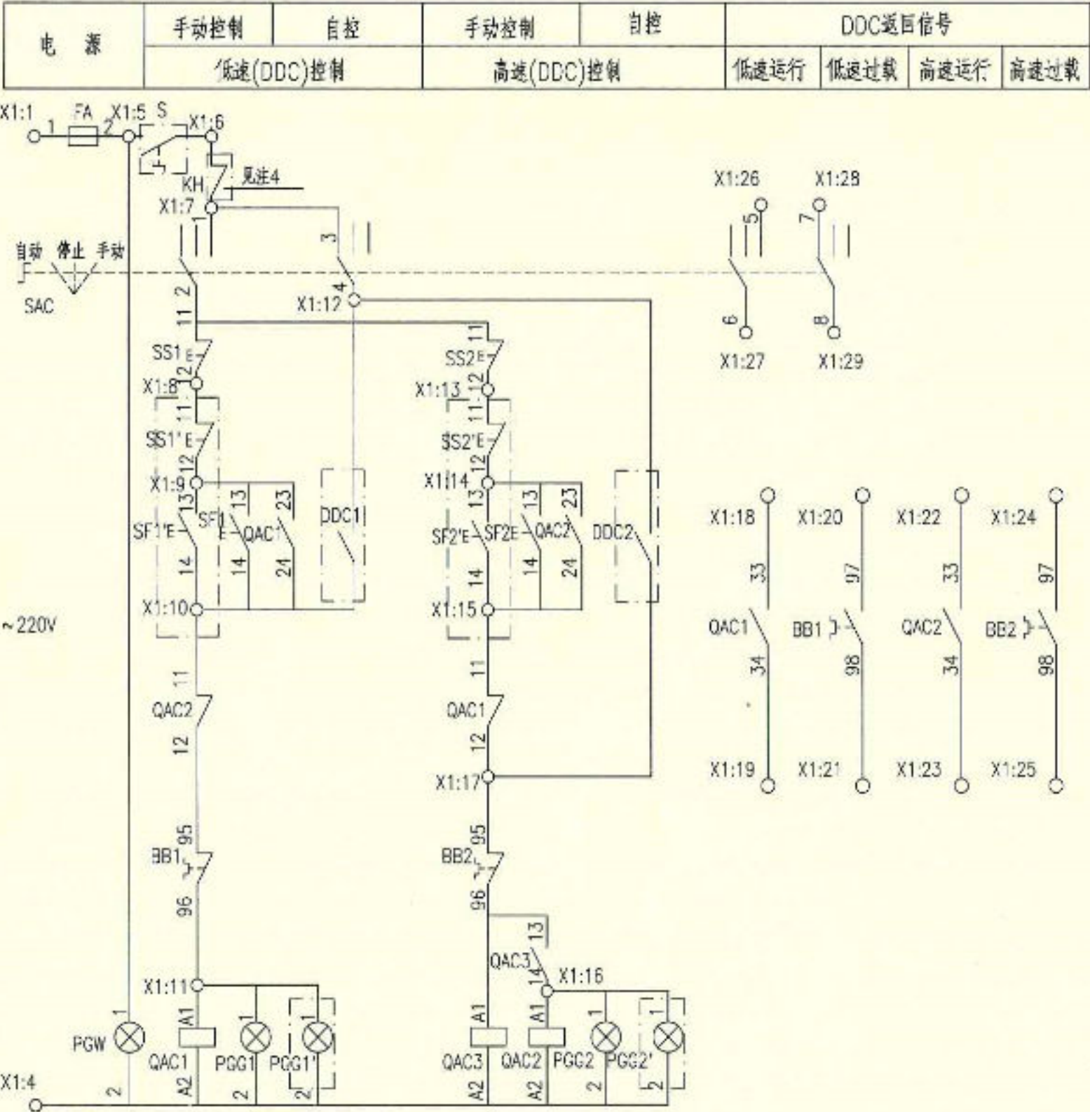
平时用双速风机电路图 XKSF-2
