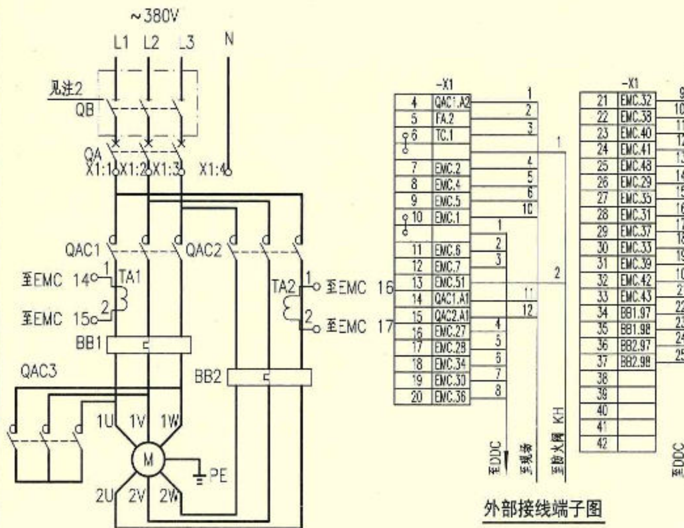
主回路
