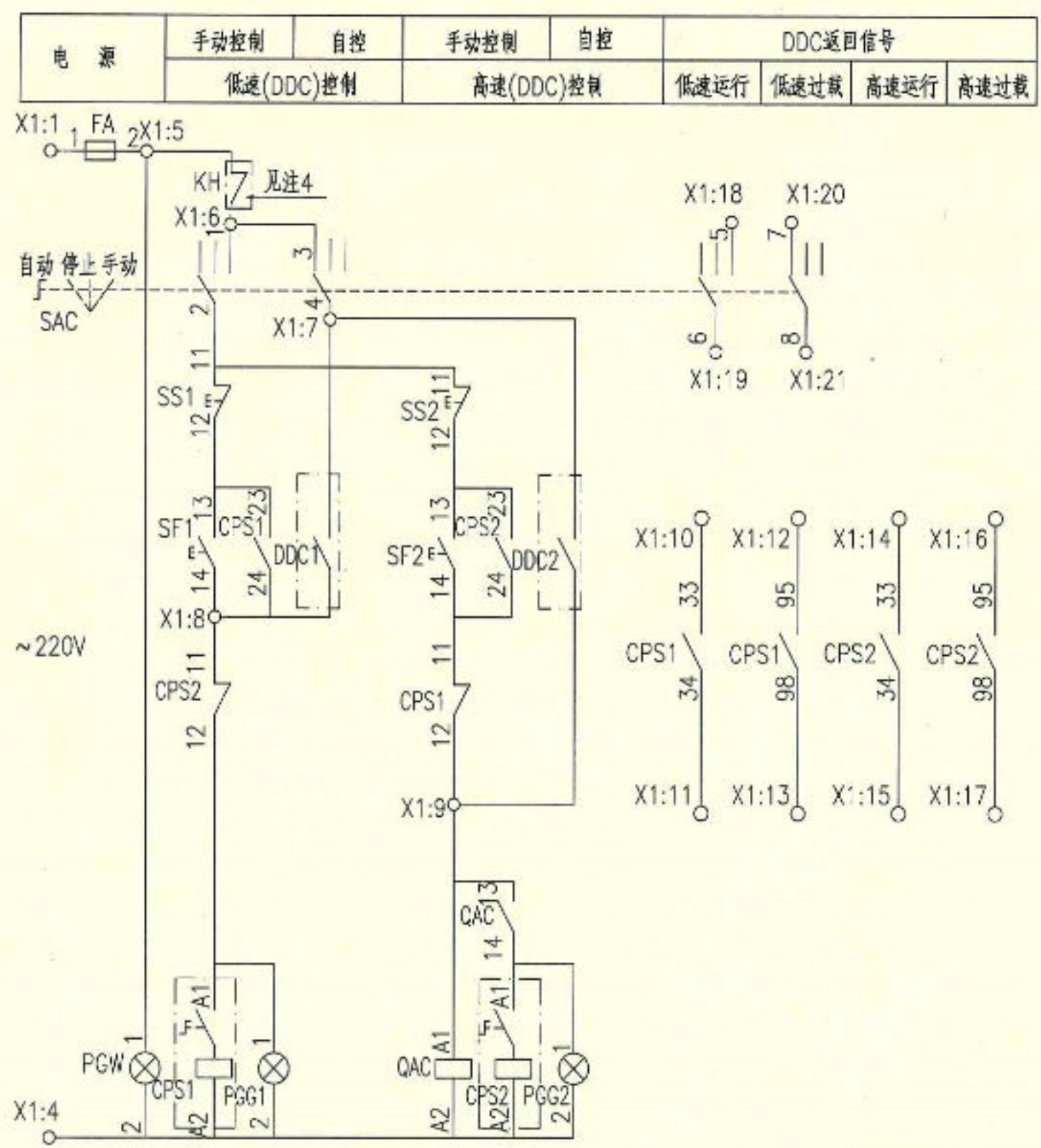
控制原理图
