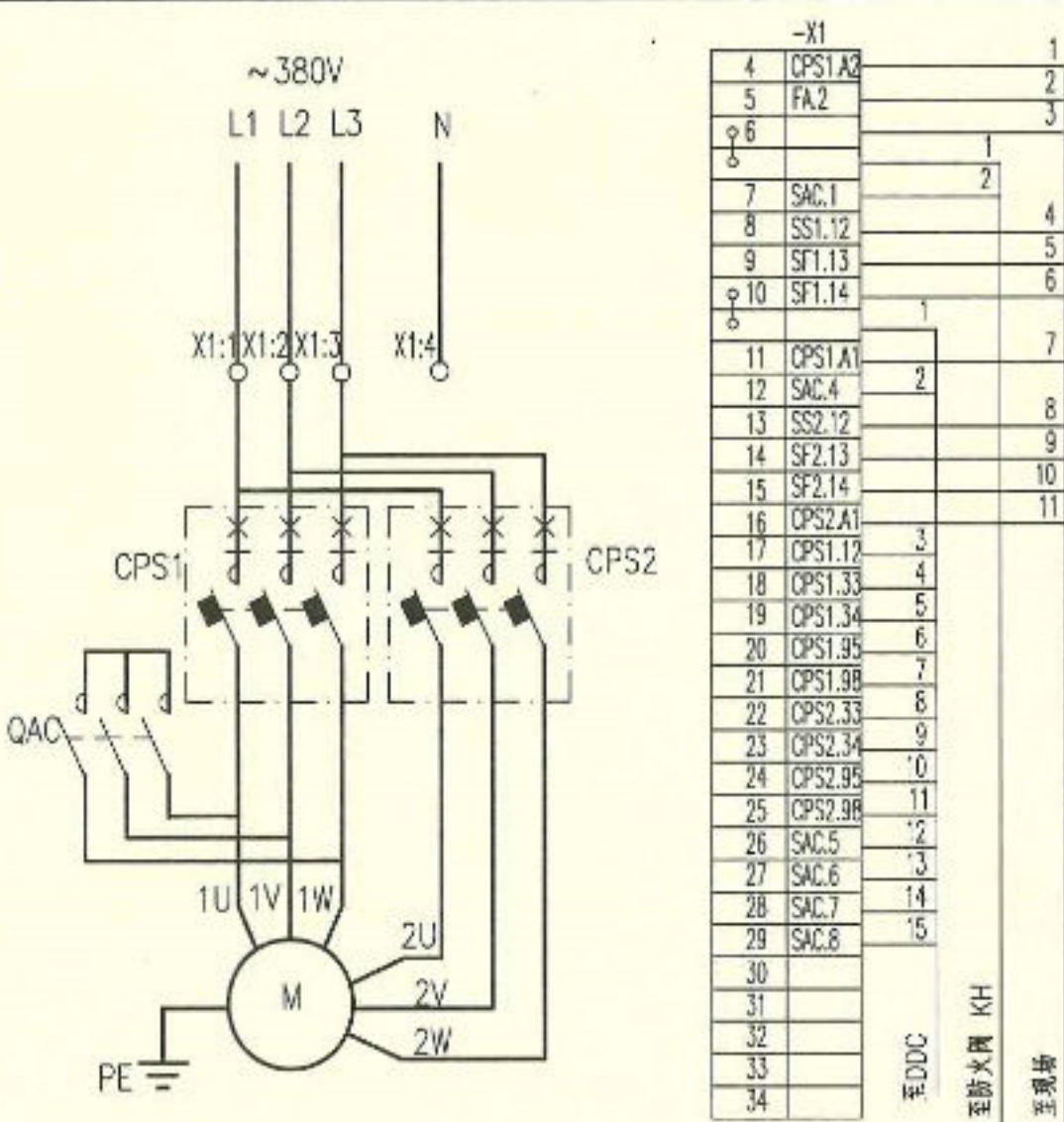
主回路
