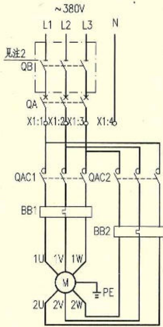
主回路
