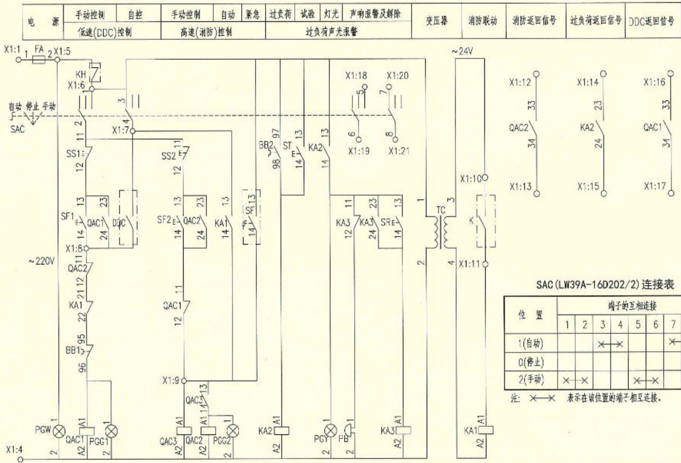
消防兼平时两用双速风机电路图XKXF-1
