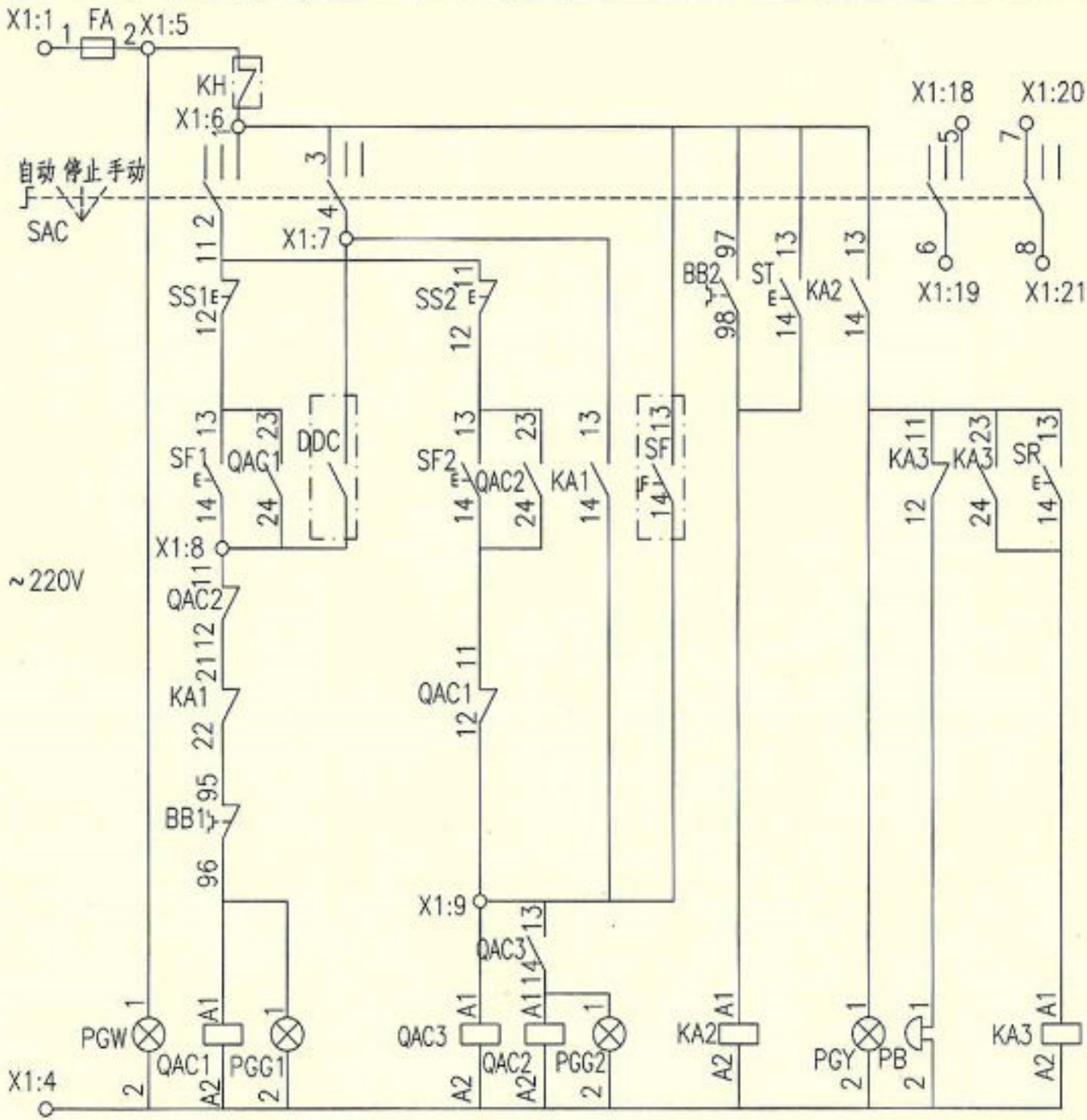
控制原理图
