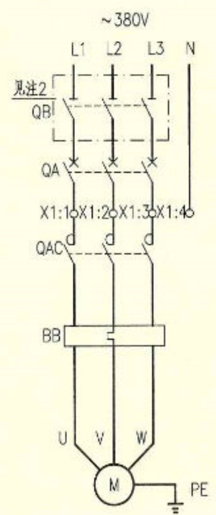
主回路
