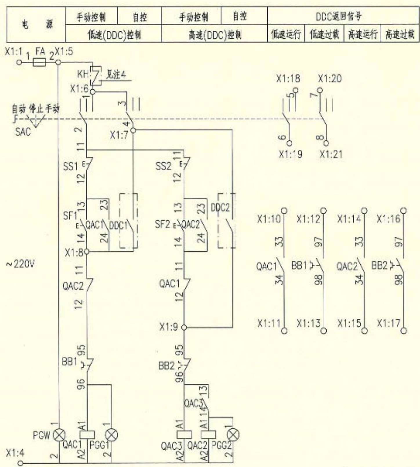
控制原理图
