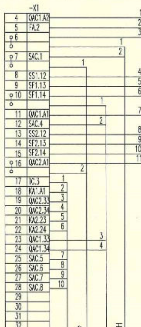
外部接线端子图
