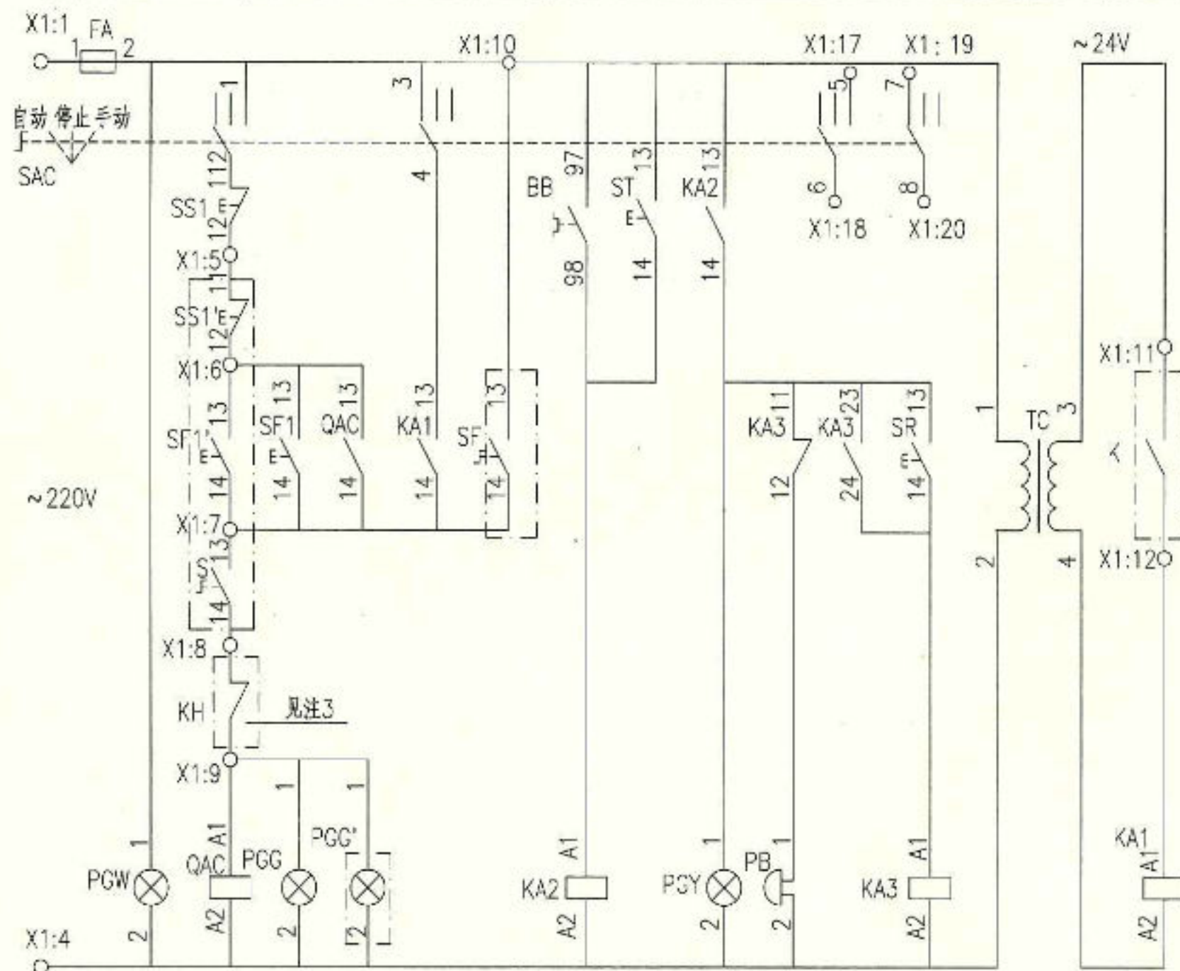
控制原理图
