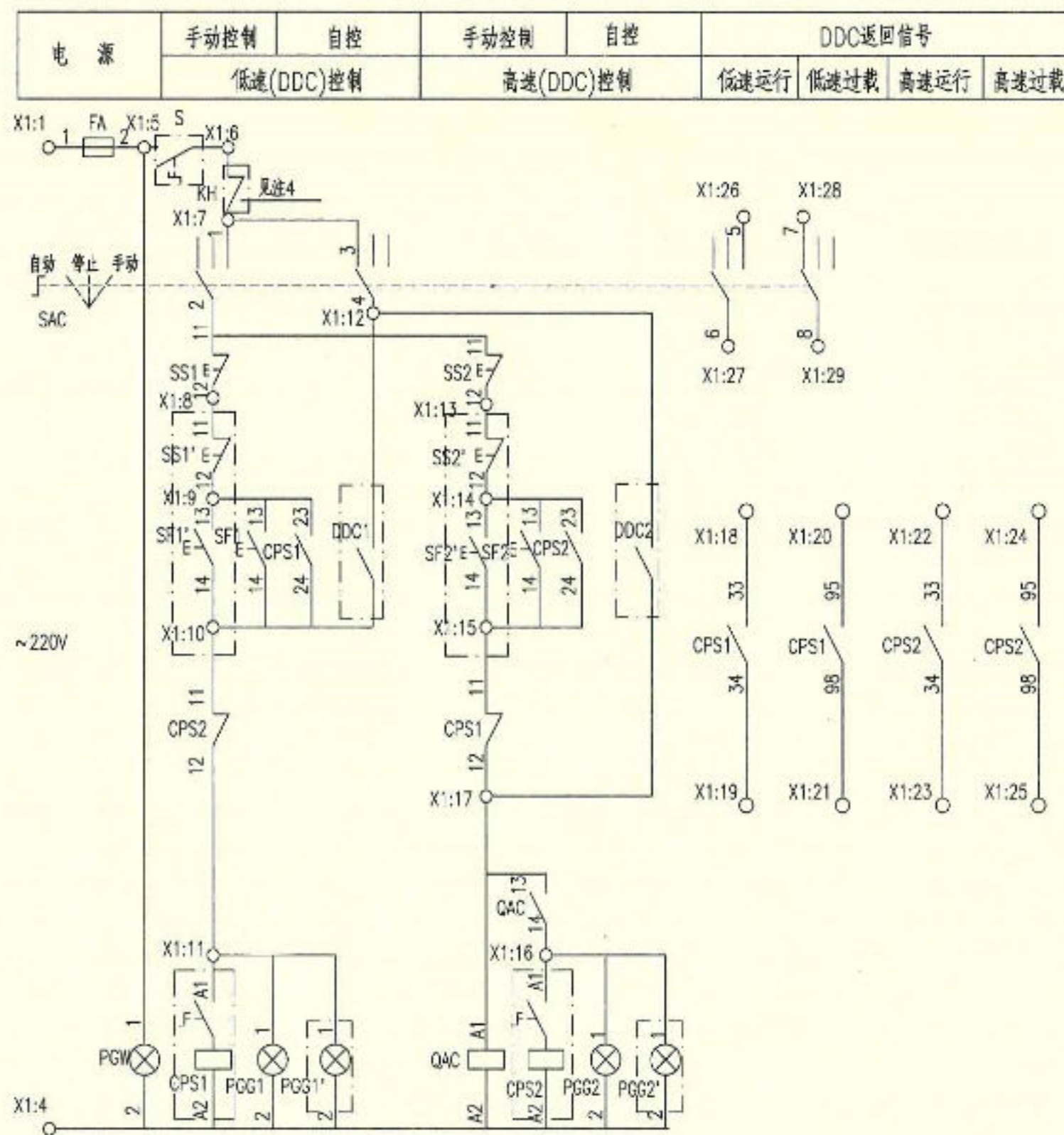
控制原理图
