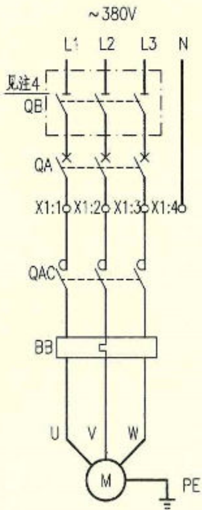
主回路
