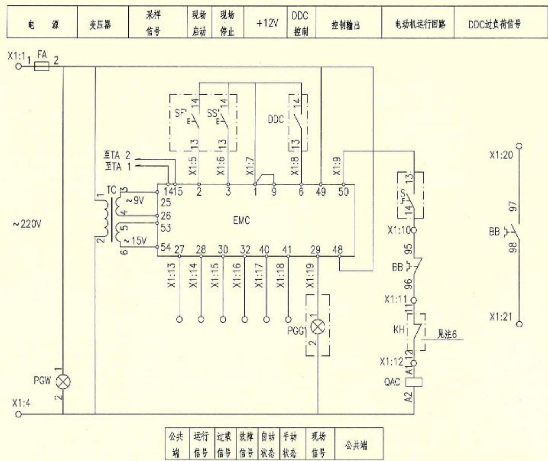
控制原理图
