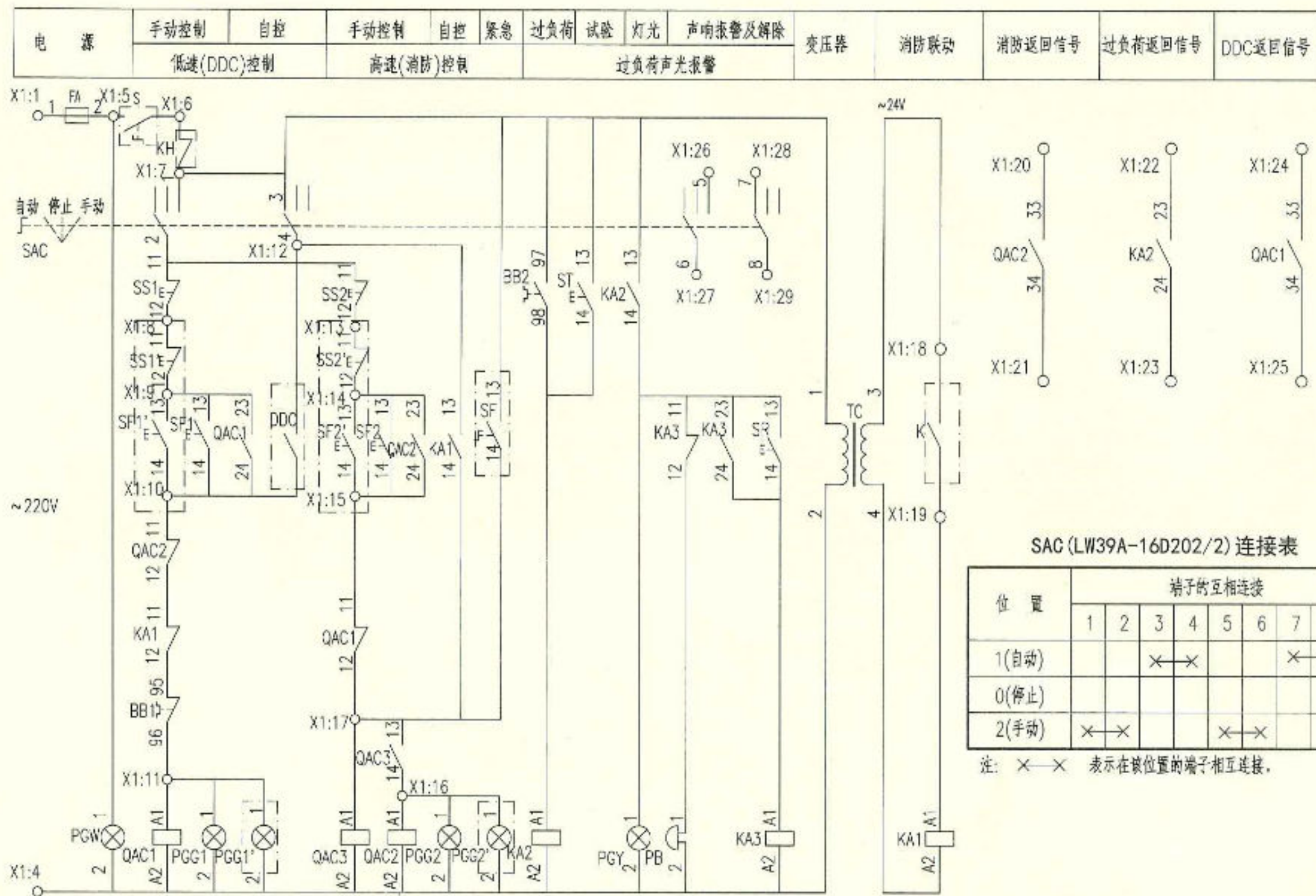
控制原理图
