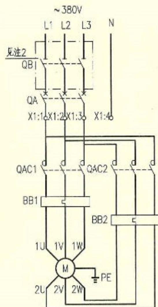
主回路
