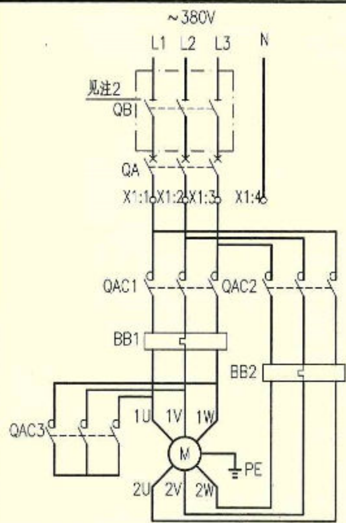
主回路
