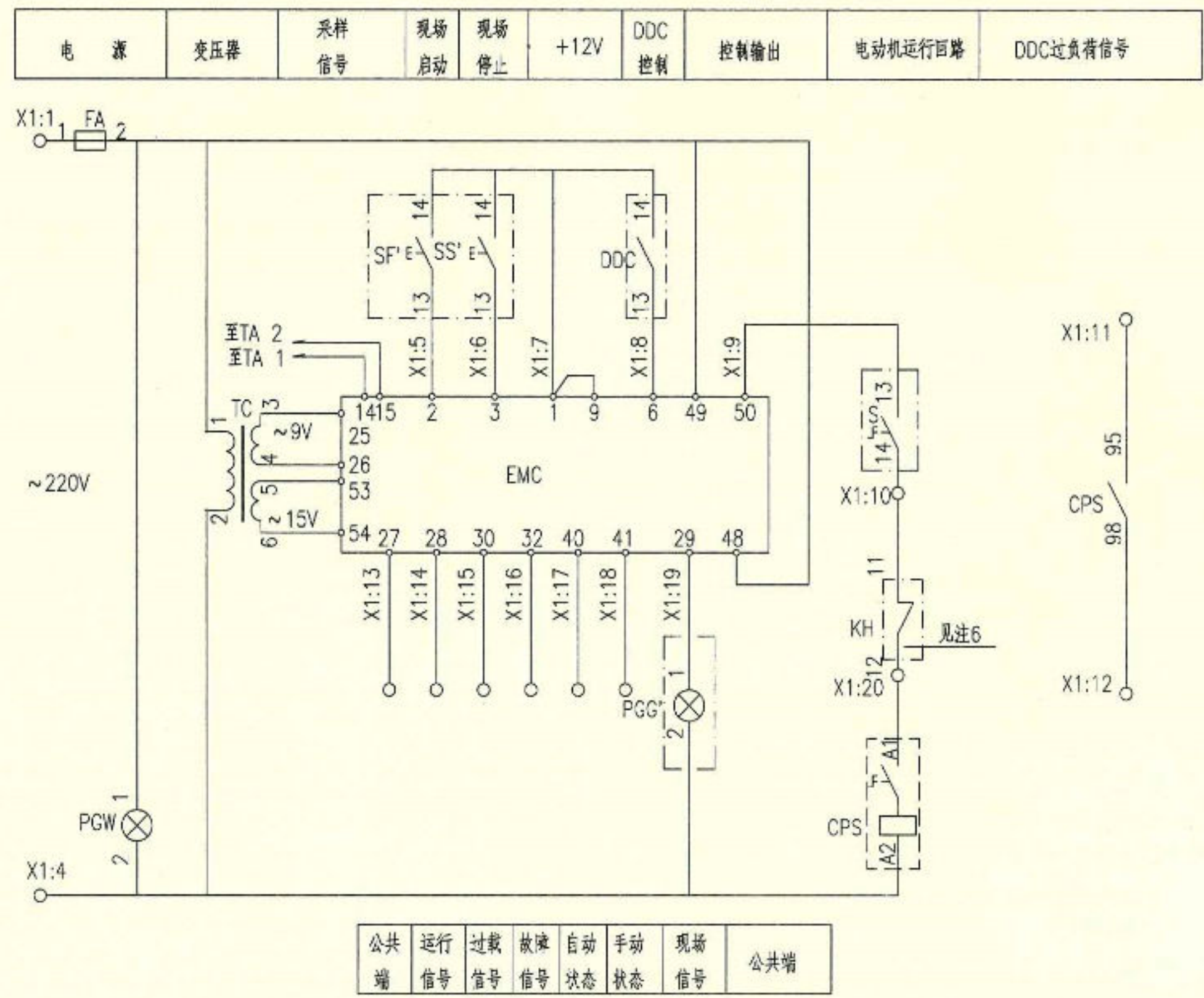
控制原理图
