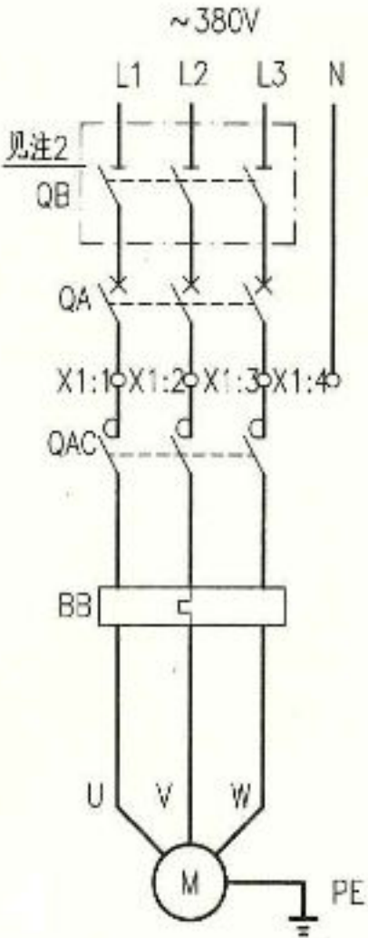
主回路
