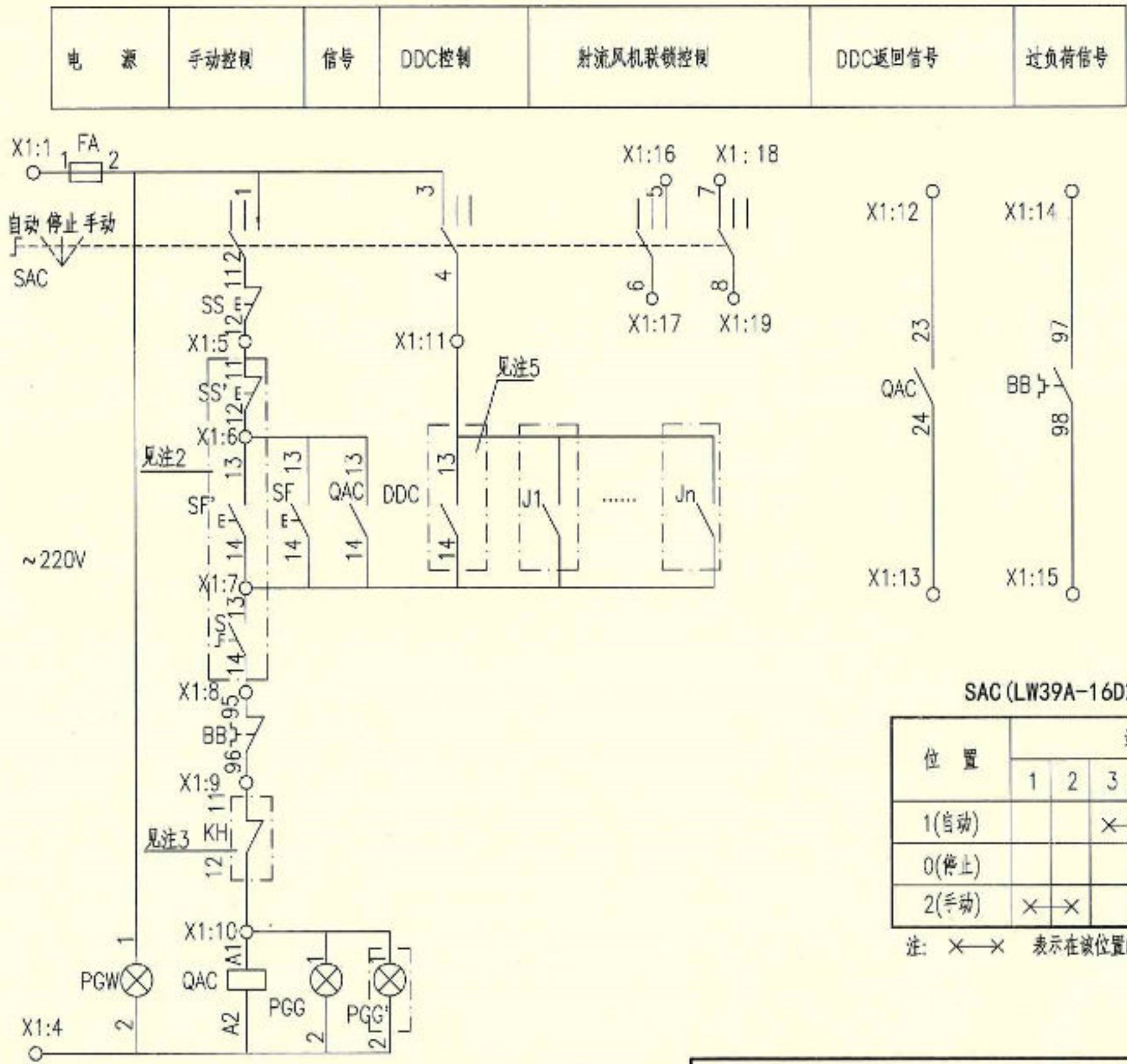
射流风机联锁排风机电路图 XKLF-1
