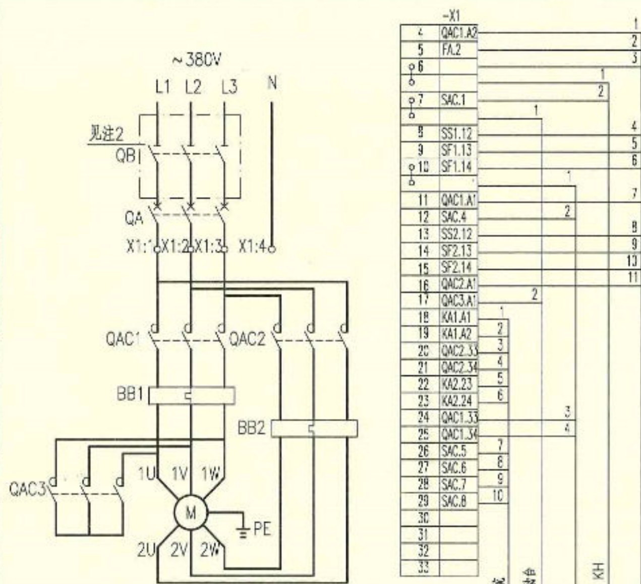
外部接线端子图
