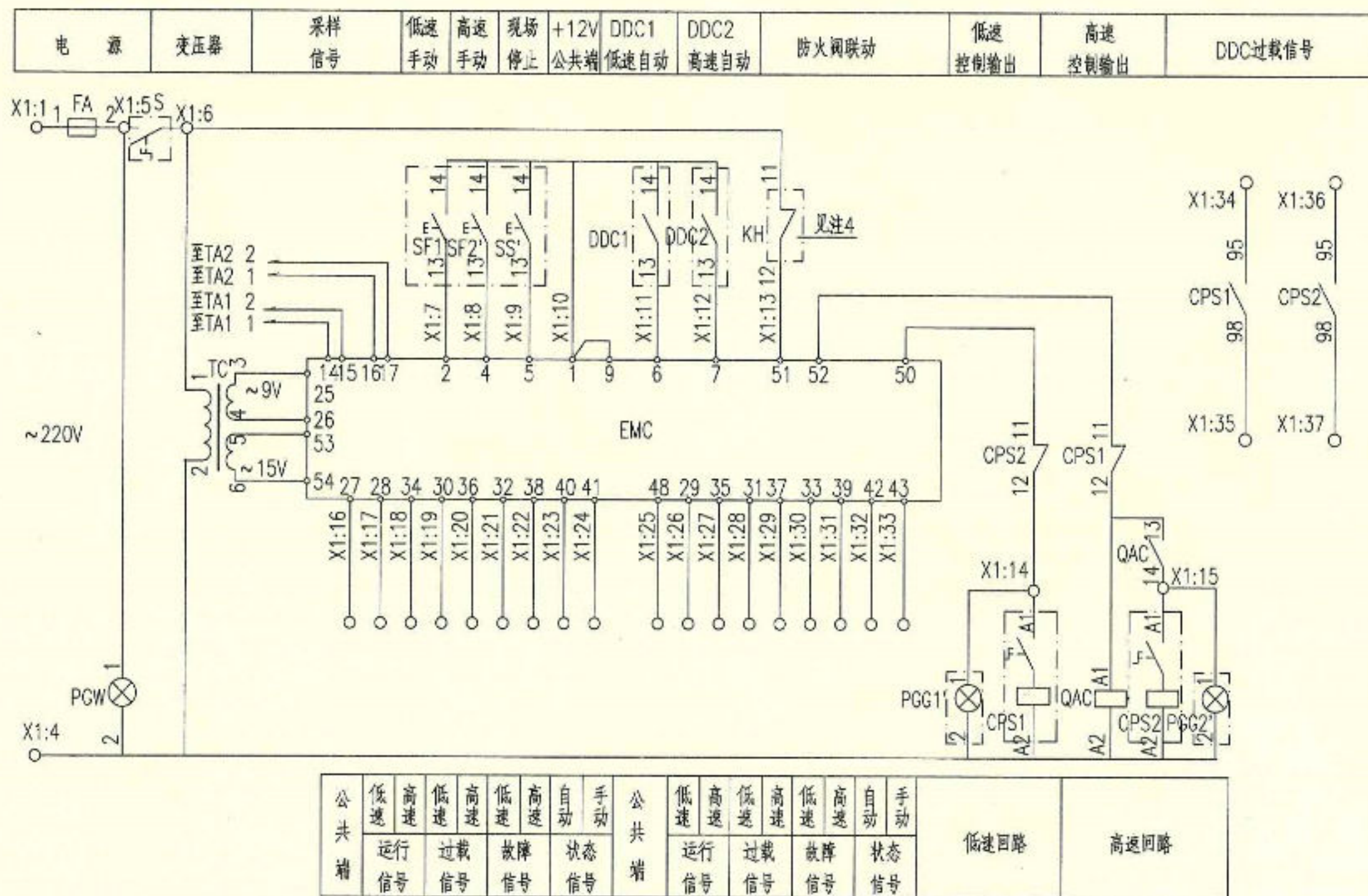
控制原理图
