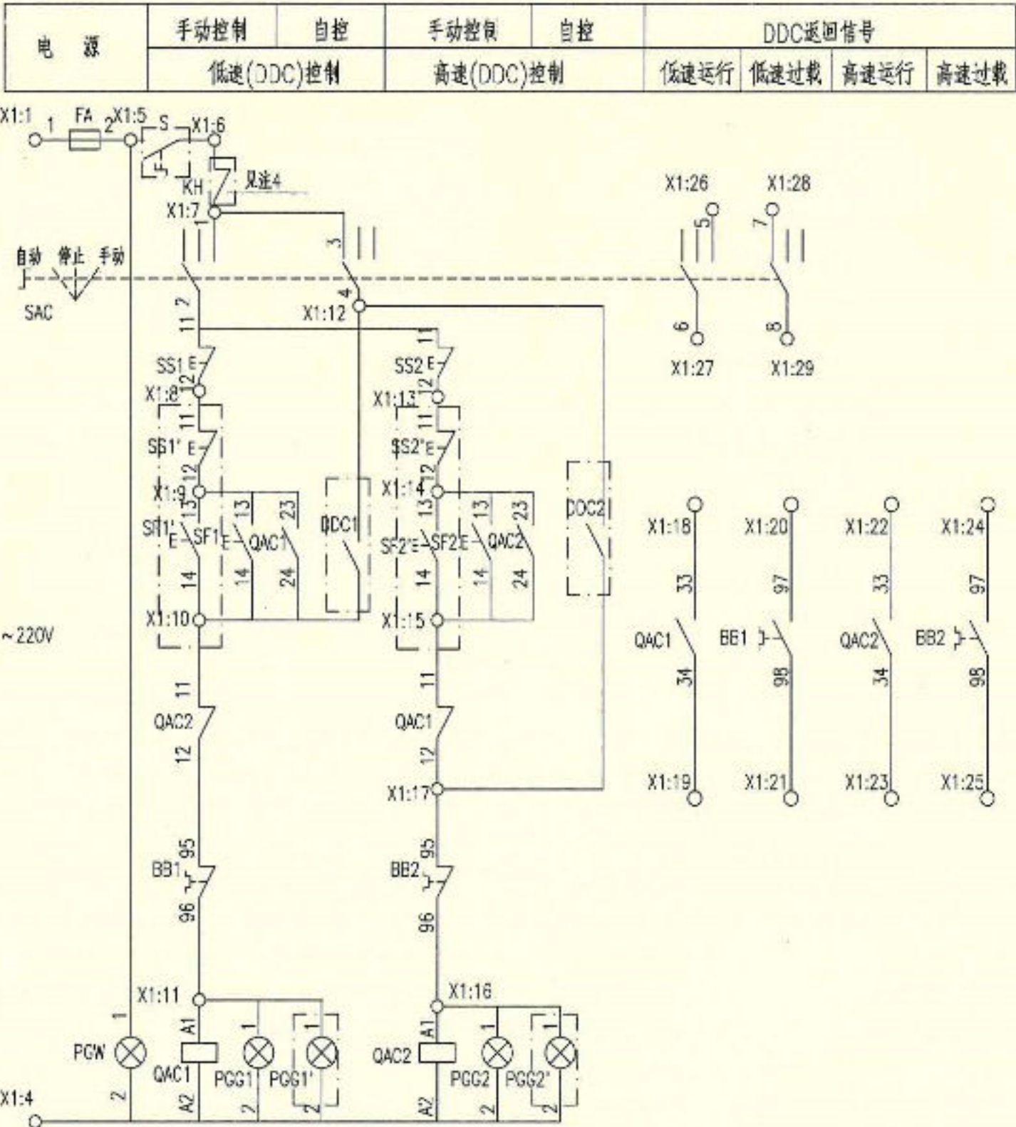
控制原理图
