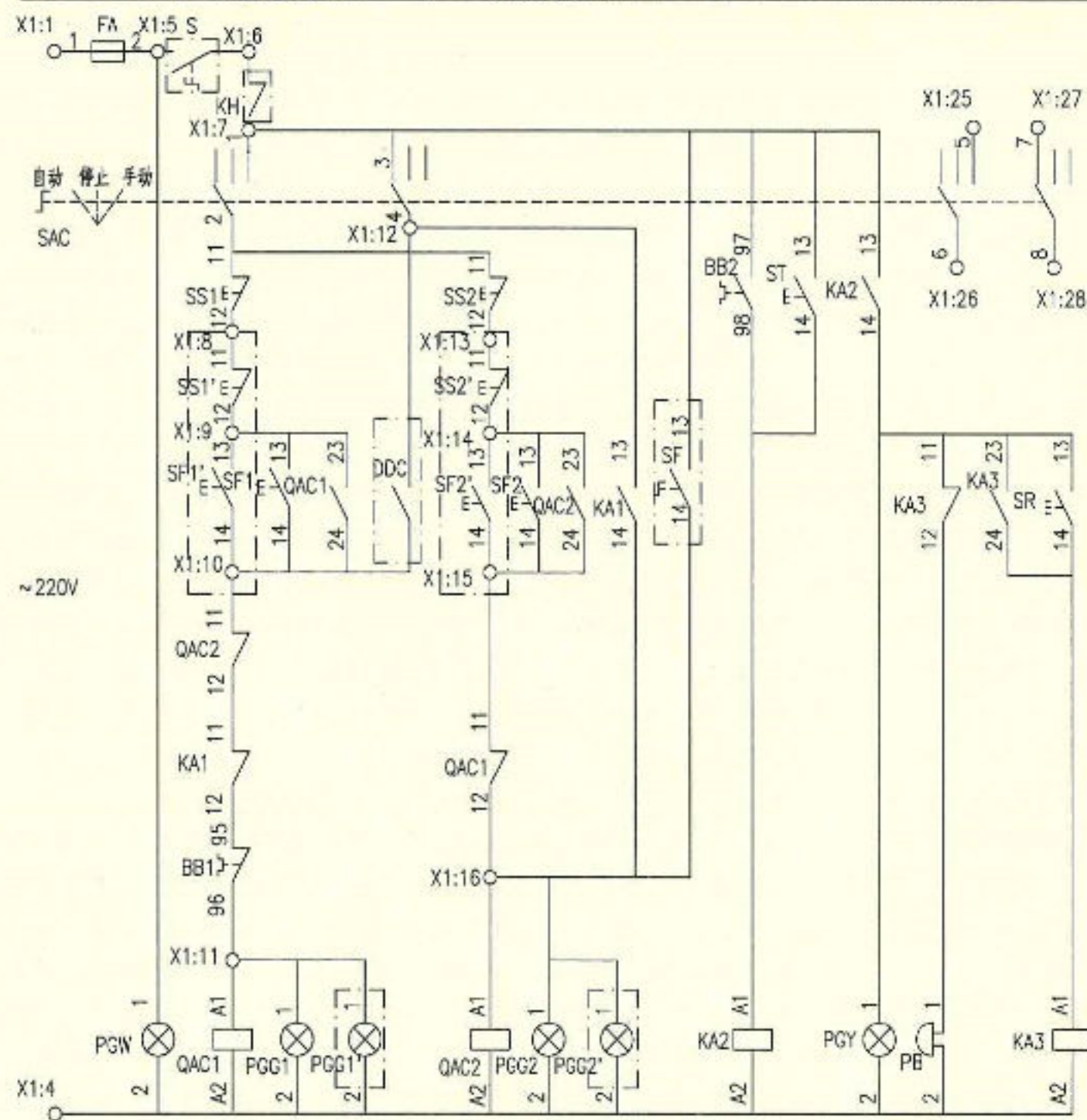
控制原理图
