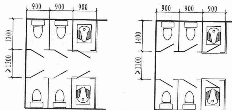
单侧隔间至对面墙之间的净距
