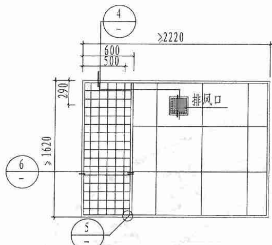
1 顶棚平面 排风口 排气扇 位置按工程设计
