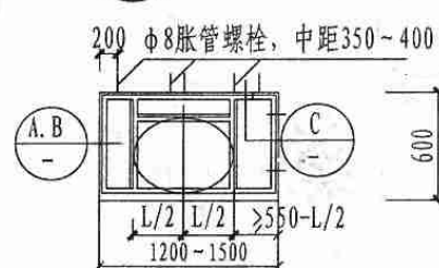
3 平面
