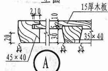
立面
