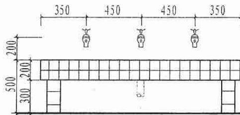
立面
