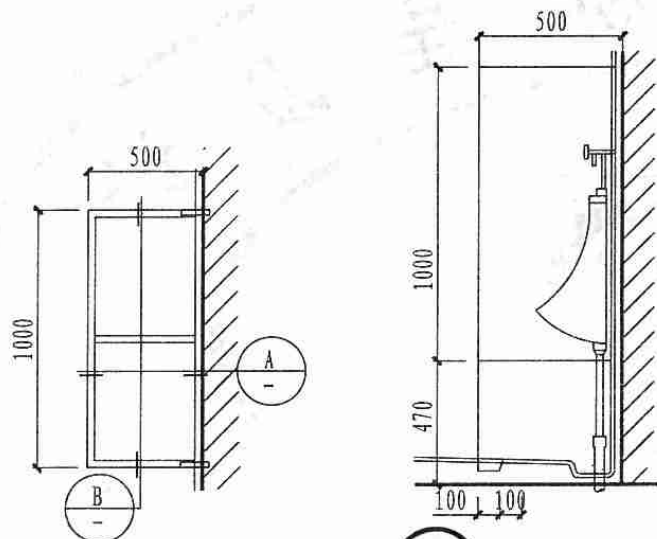
1 成品塑料板隔断
