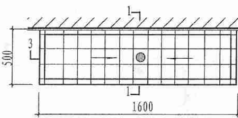
② 平面
