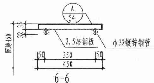
淋浴坐凳 (一)
