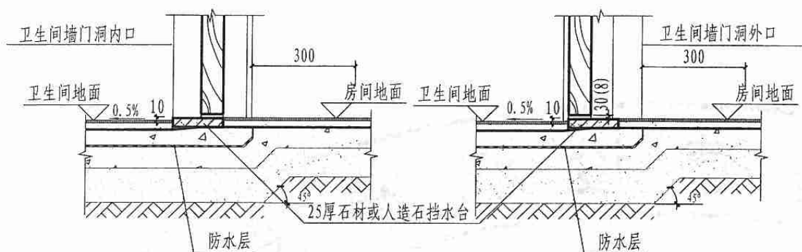
① a 门框立于墙外平 (括号内尺寸为百页门)
