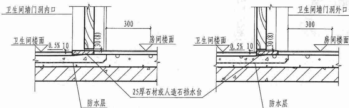
② a 门框立于墙外平 (括号内尺寸为百页门)
