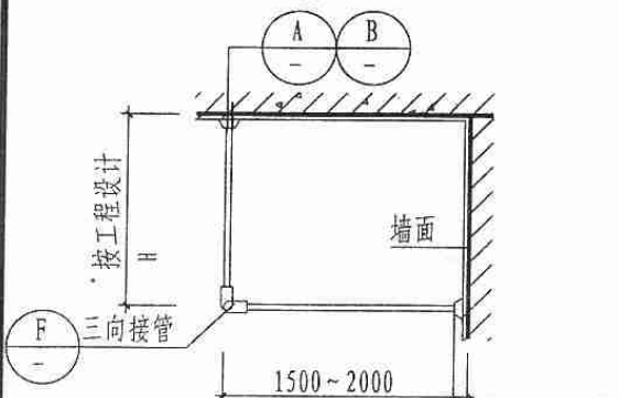
3 平面
