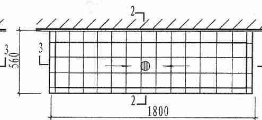
④ 平面
