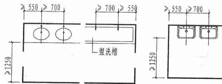
单侧并列盥洗台、槽或洗手盆盥洗间距至对面墙面的净距
