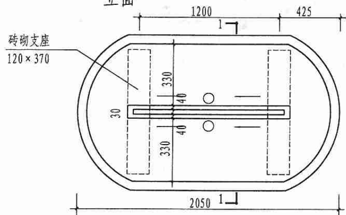
平面
