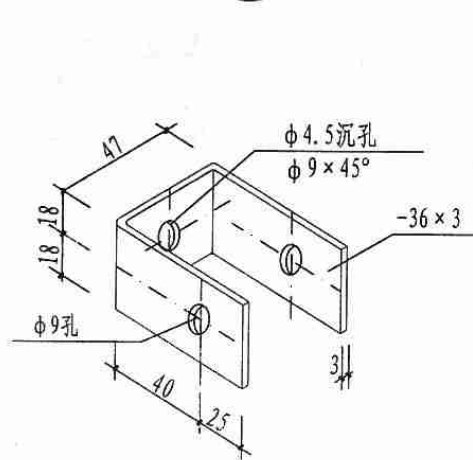
铁件6
