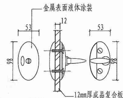
5 门锁大样
