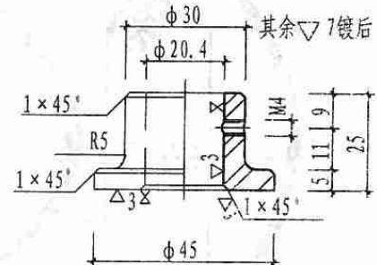
H 法兰压盖
