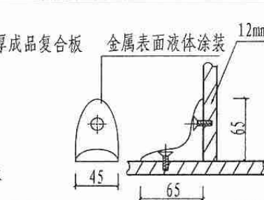
3 L型固定片大样
