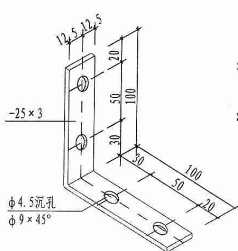
铁件4
