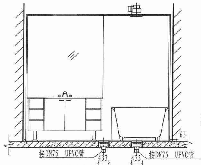
2-2 地漏直排
