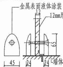
2 U型固定料大样
