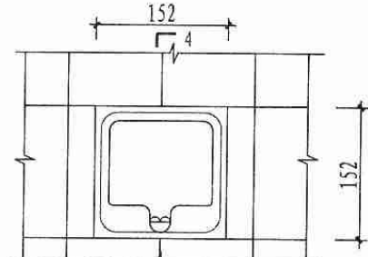
立面
