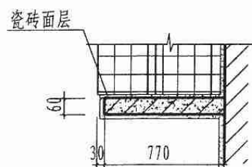
1 混凝土隔断
