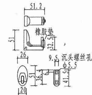
9 挂衣钩大样
