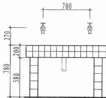
立面
