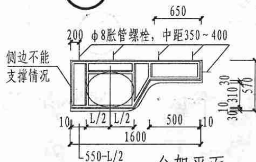
台架平面
