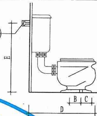
侧立面
