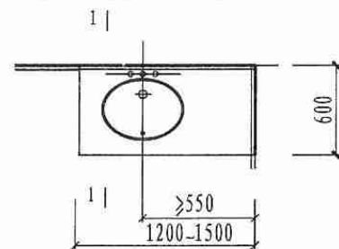
3 平面
