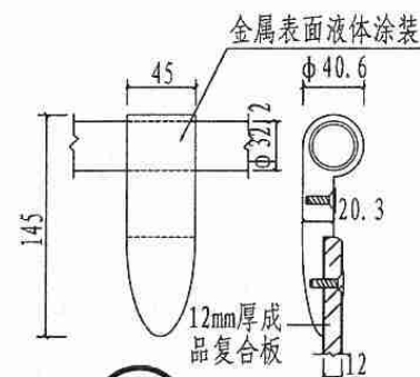
6 拉杆大样
