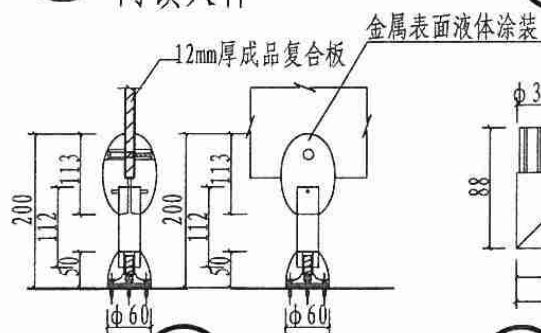
7 脚座大样
