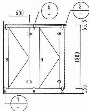
厕所隔间(内、外开)正立面图 厕所隔间侧立面图 小便斗隔屏侧立面图
