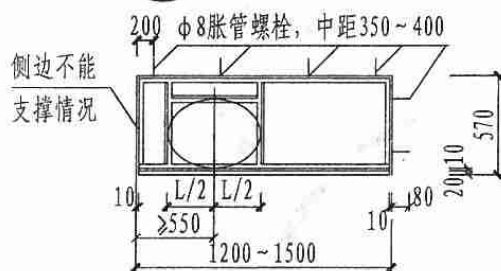
台架平面
