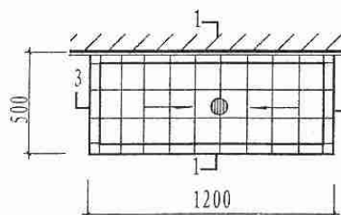
① 平面
