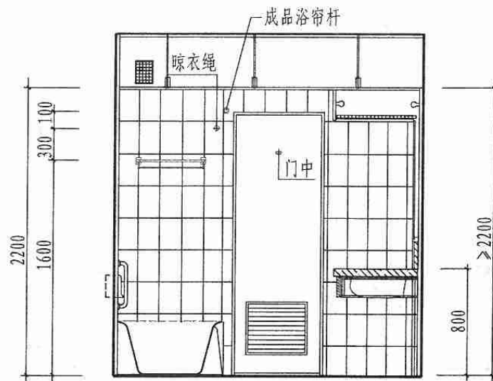
2-2 剖面
