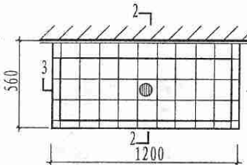
③ 平面
