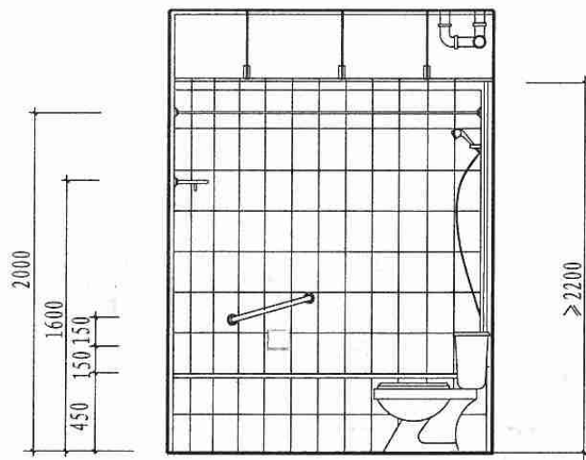
2-2 剖面
