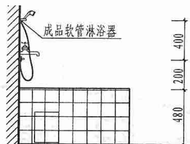
立面
