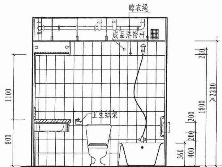
1-1 剖面
