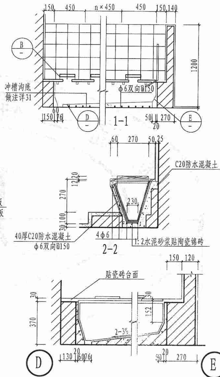
幼儿园厕所详图(二)
