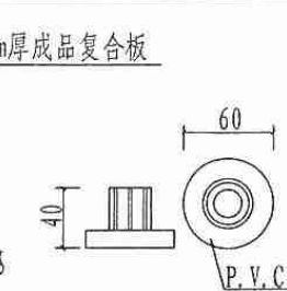
4 拉杆固定座大样
