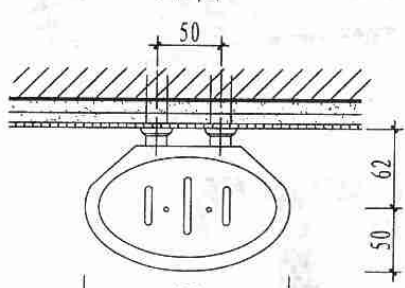
平面
