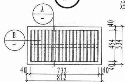
木踏板
