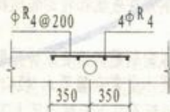
附图 9.4.11 板内管线做法
