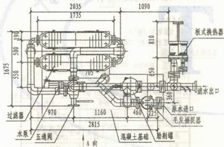
PA100-210型可逆式硅藻土泳池过滤机组大样图
