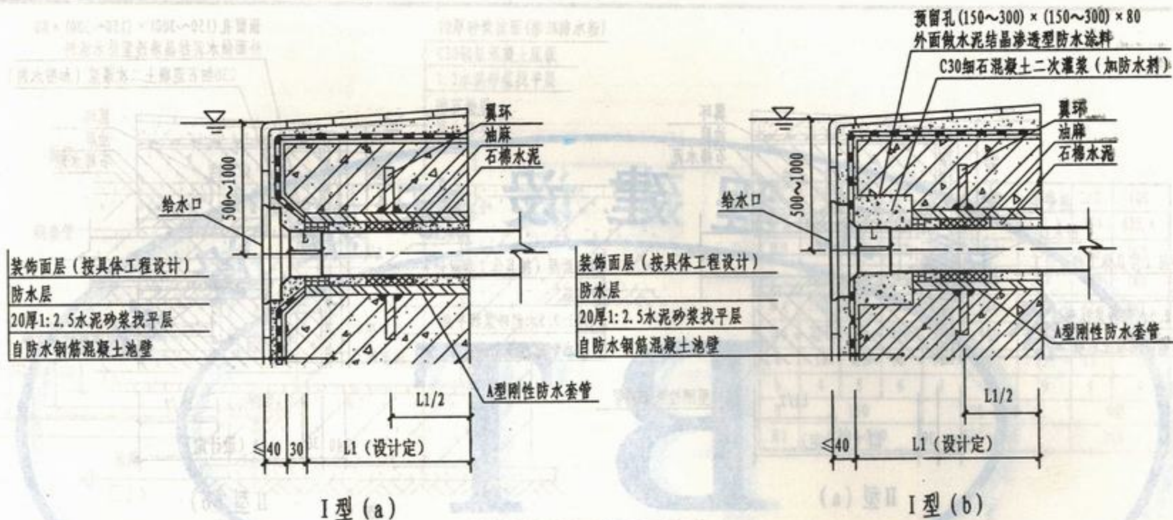
给水口配水管穿池壁安装图
