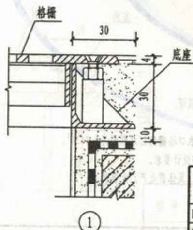
HSK-360 HSK-450 回水口安装图
