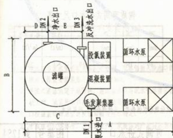
平面图
