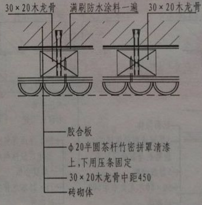
木装修内墙面 (二)
