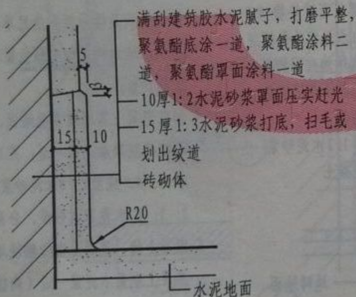
⑤ 聚氨酯涂料水泥踢脚
