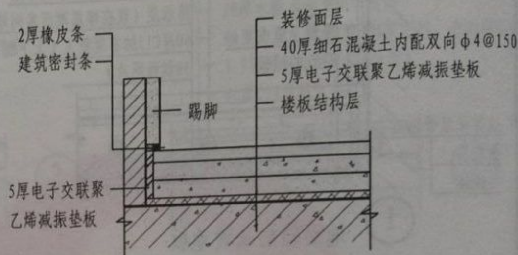
① 减振垫板隔声楼板
