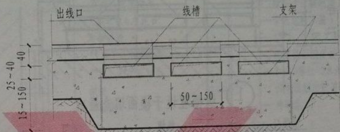
① 线槽埋设于地面垫层内
