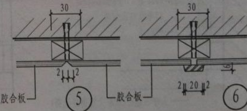
木墙裙 (一)
