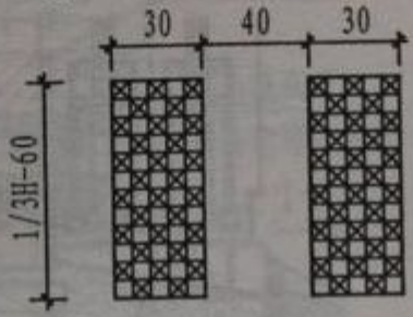
③ 孔洞大样
