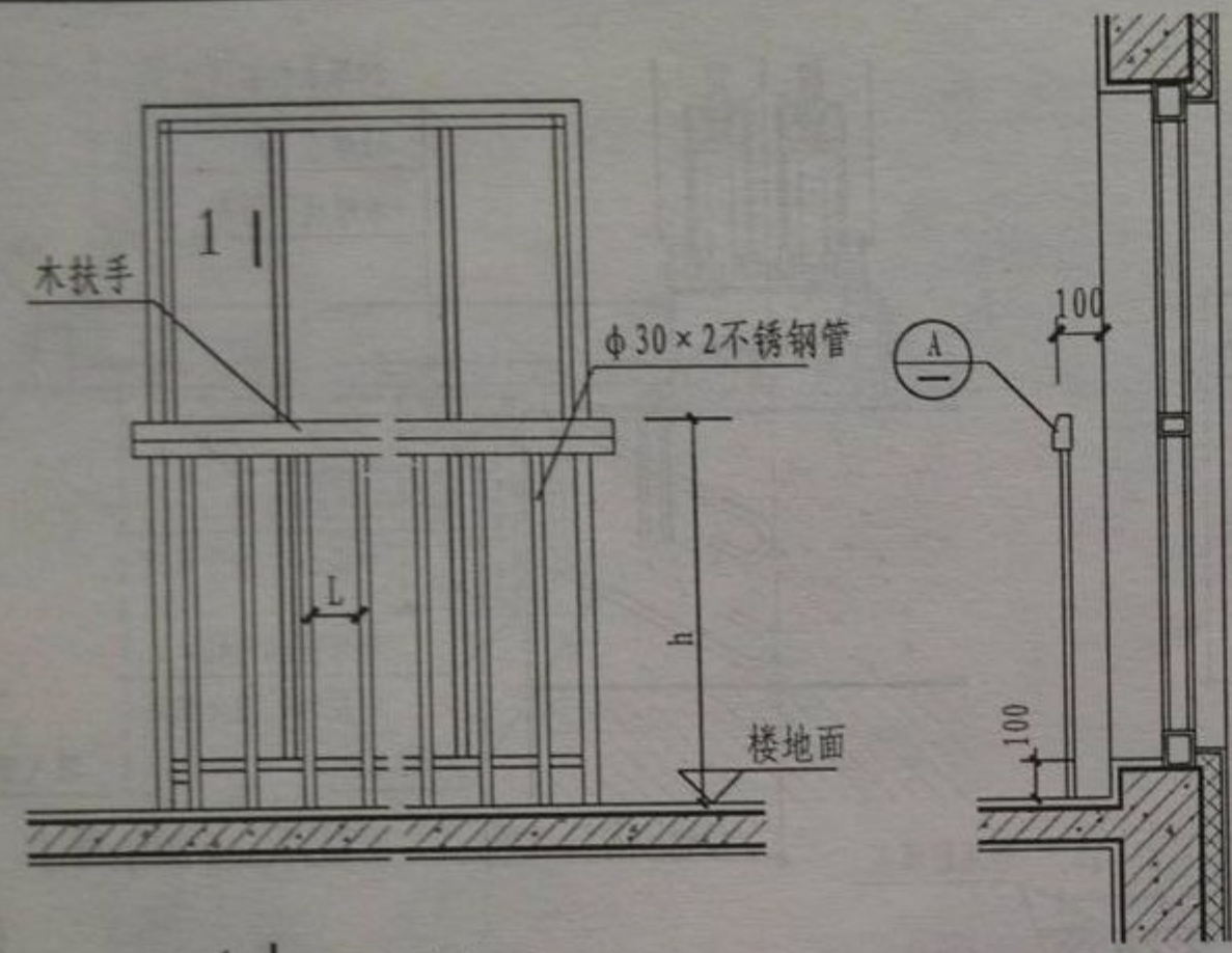
1-1 室内立面
