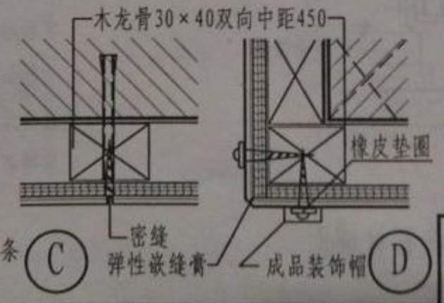
墙、柱贴面-玻璃面料 (一)
