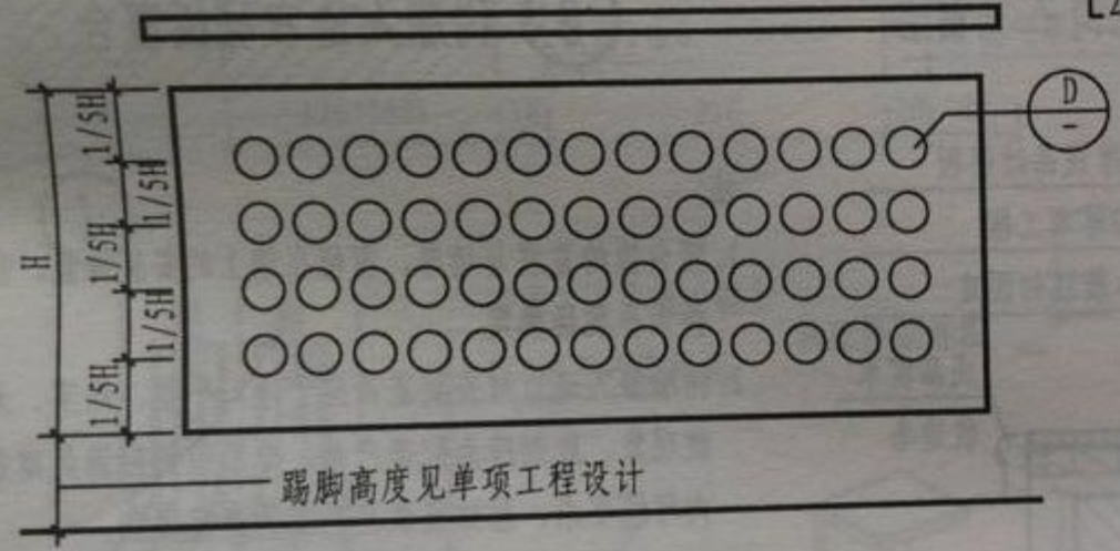
暖气罩立面示意 ②
