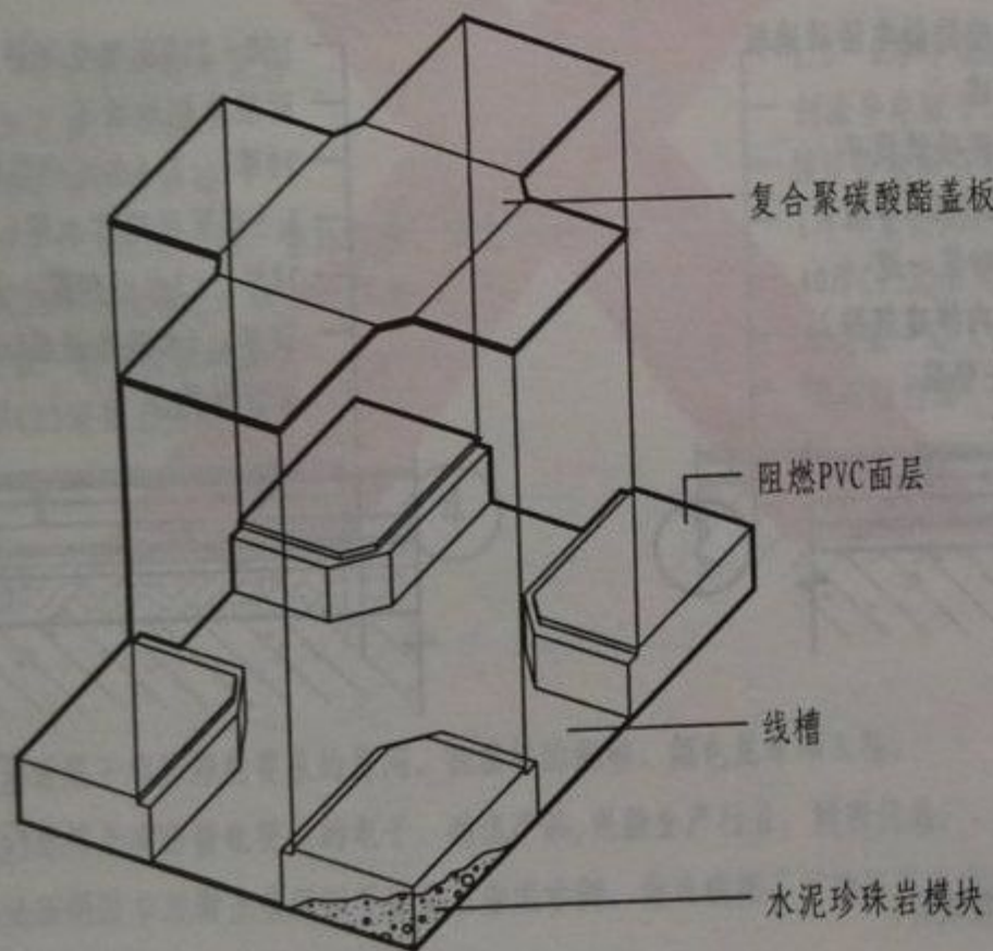
平铺型网络地板结构示意图
