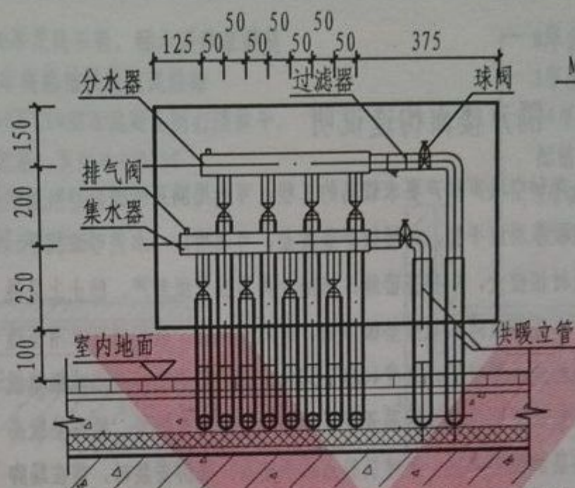
低温热水辐射分、集水器安装示意图
