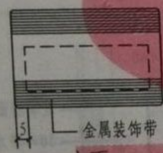
立面
