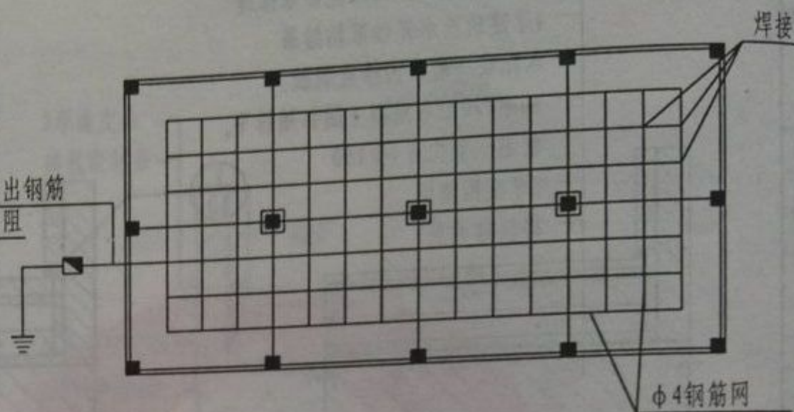
方格形导静电接地网示意图
