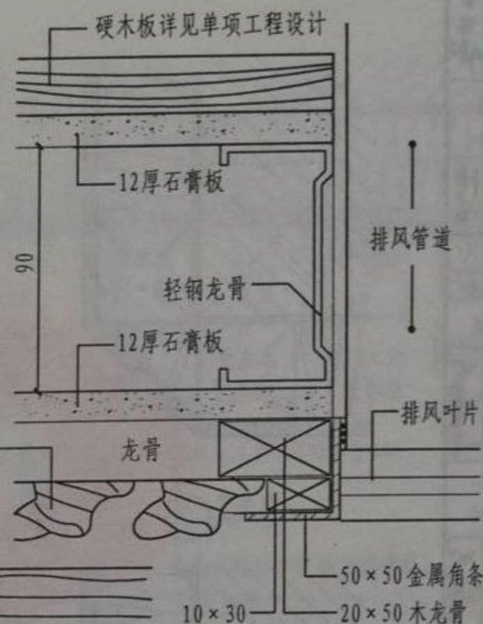
1-1 剖面
