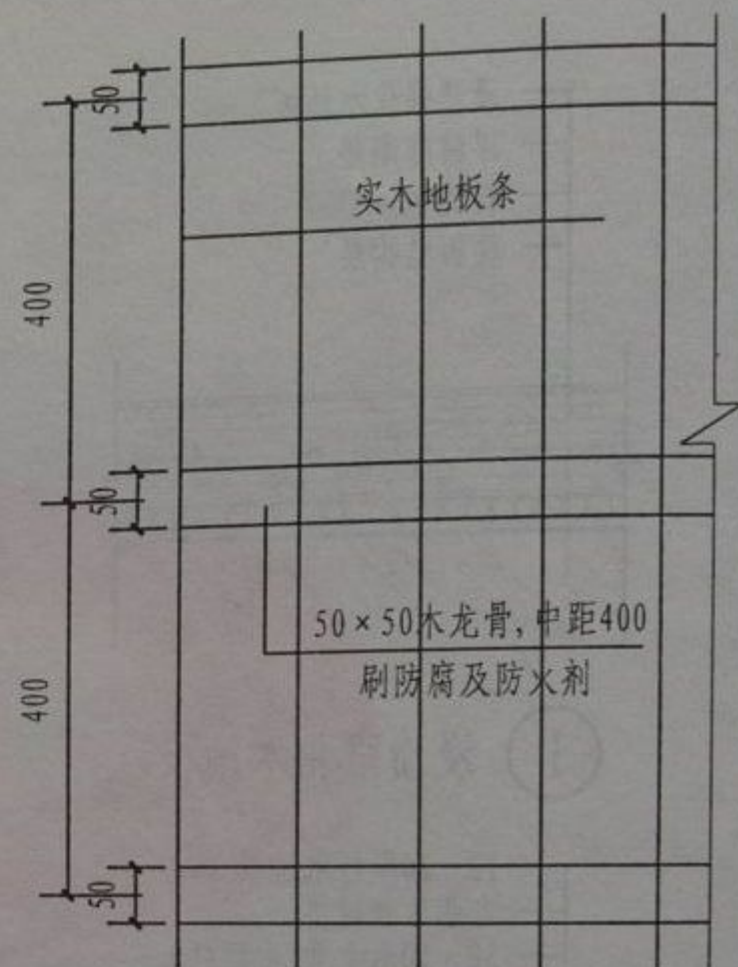
实木地板示意图
