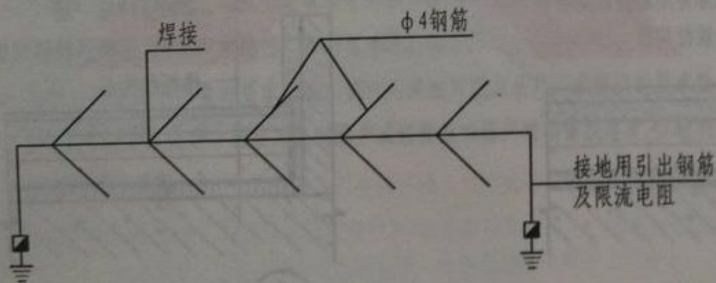
鱼骨形导静电接地网示意图
