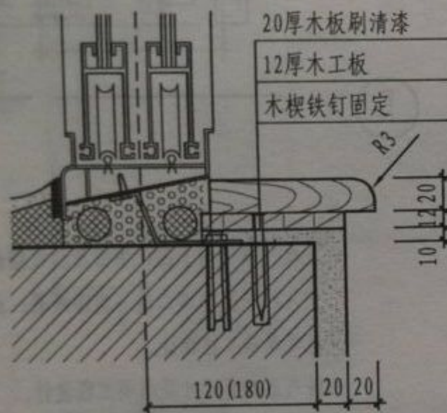
④ 木窗台
