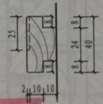
剖面
