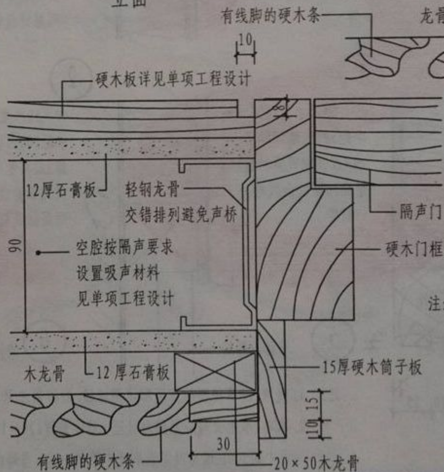
2-2 剖面
