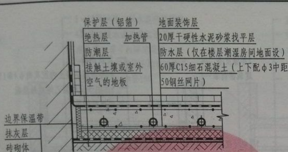
1 地面辐射采暖地板
