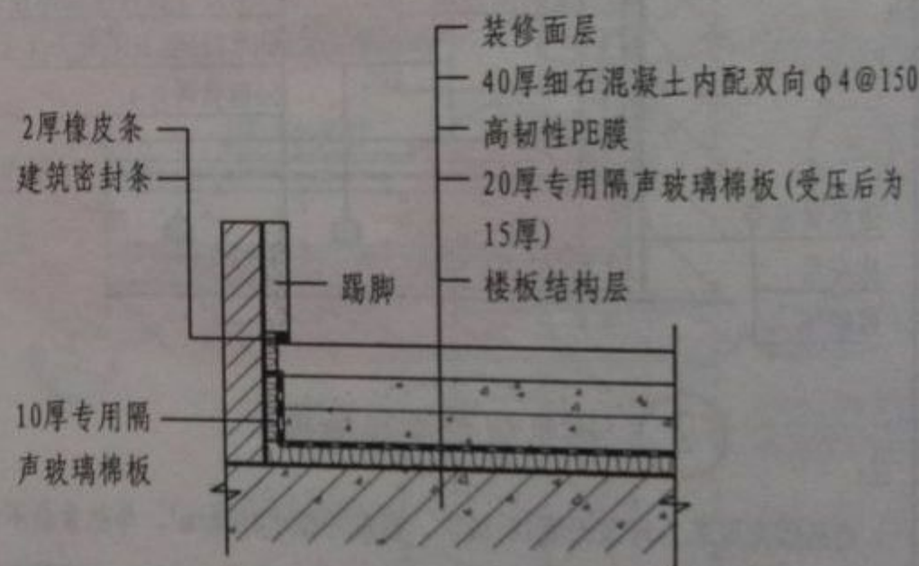
② 隔声玻璃棉板隔声楼板
