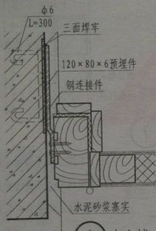
1 中立樘
