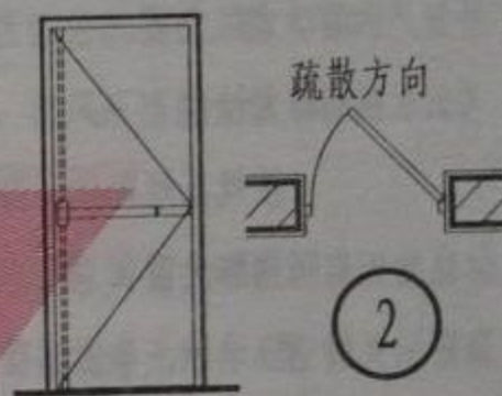
b. 暗装插销式
