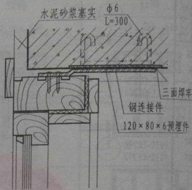
2a 边立樑
