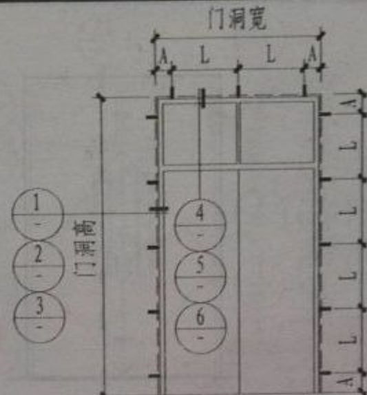
带亮门立樘缝隙及 钢连接件位置立面
