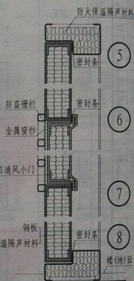
双扇门框与墙体连接位置图
