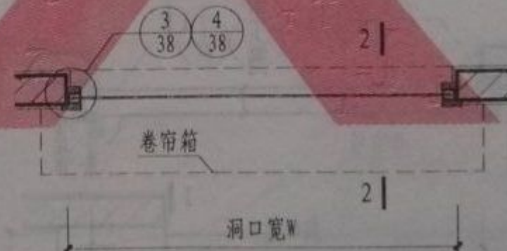
④ WFJ (中装) 平面图
