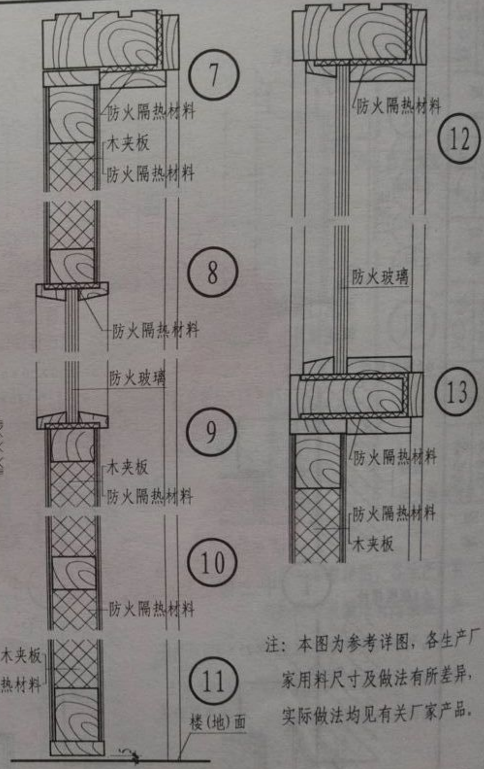
木夹板防火门详图
