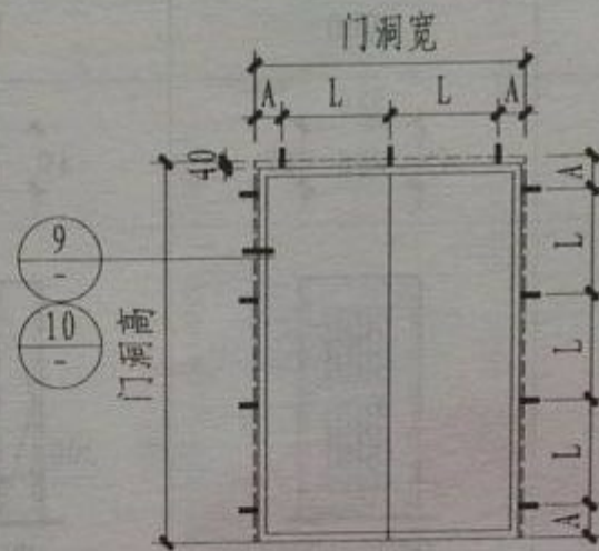
双扇门框与墙体连接位置图
