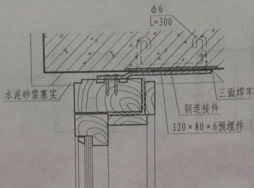
2 中立樑
