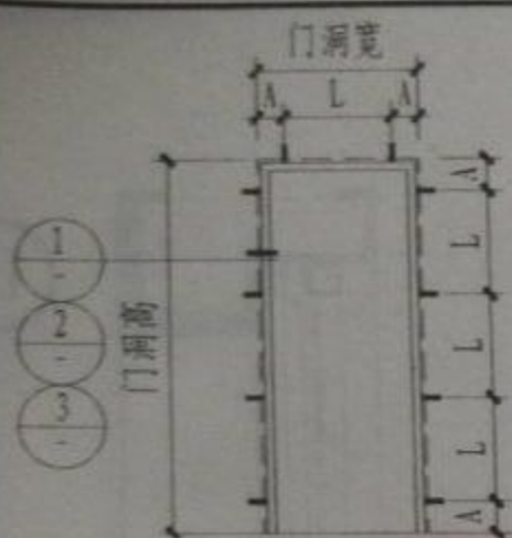
单扇门立樘缝隙及 钢连接件位置立面
