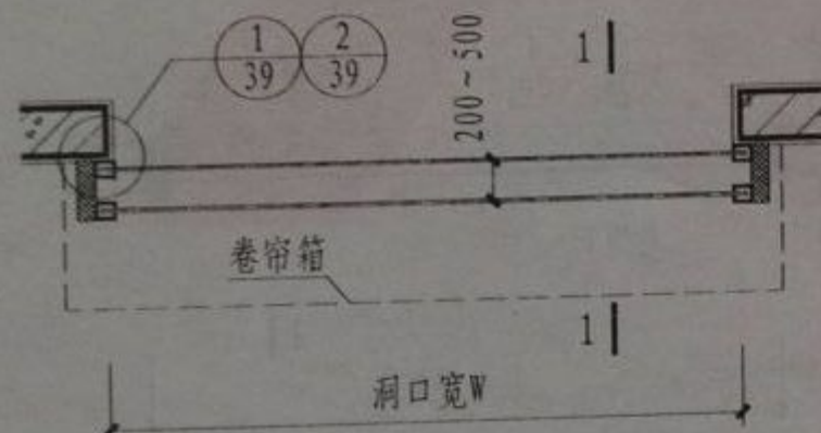
② TFJ(侧装)平面图
