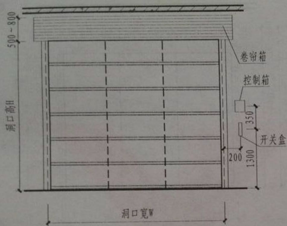
① TFJ立面图
