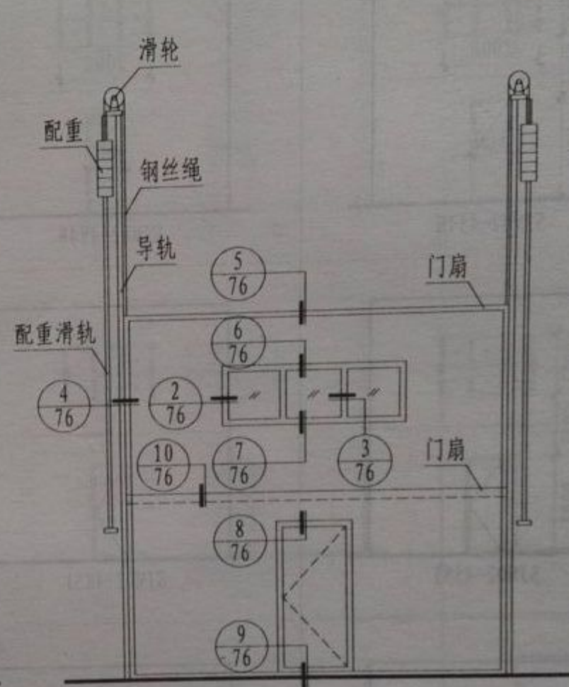
SJM02内立面图
