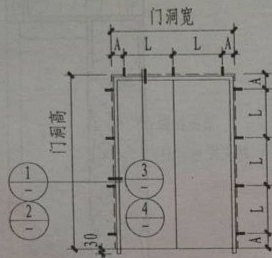
双扇门立樘缝隙及 钢连接件位置立面
