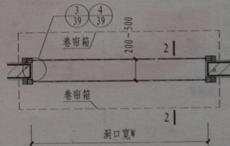
③ TFJ(中装)平面图
