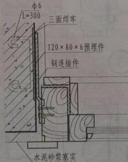
1a 边立樑
