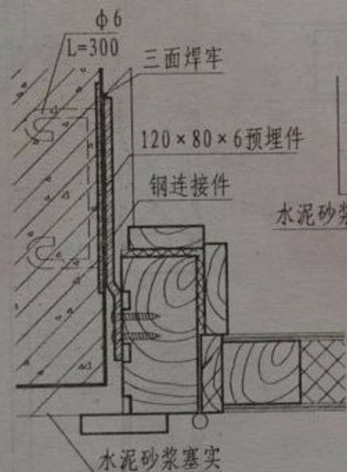
2 边立樘
