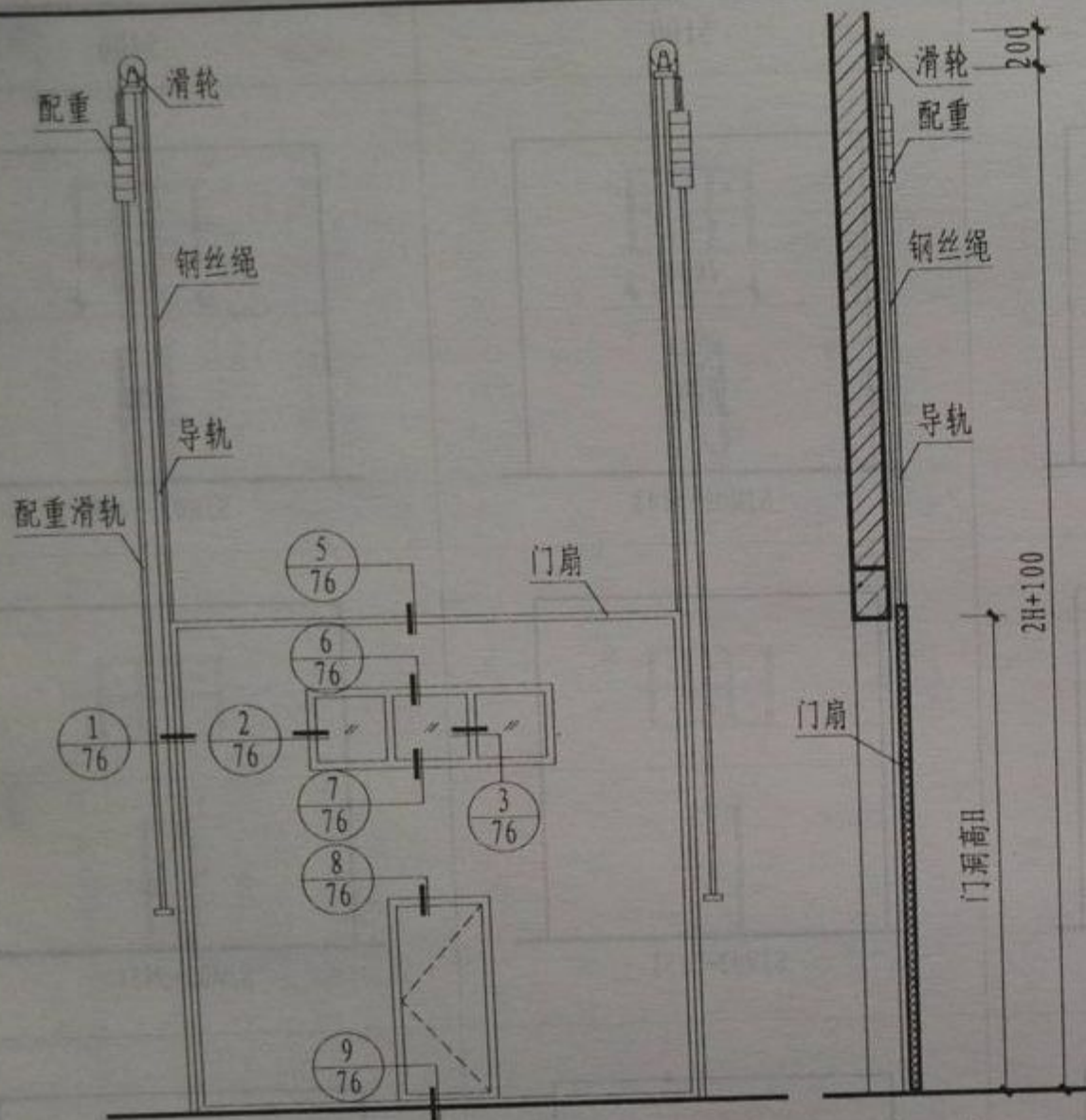
SJM01内立面图
