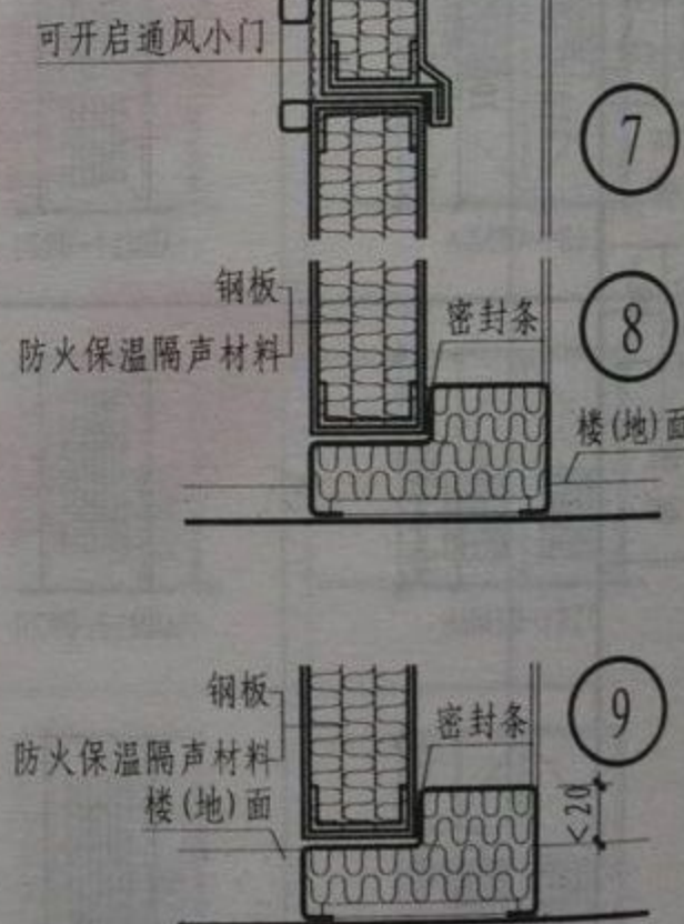
无障碍入口做法
