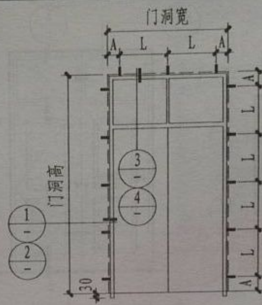
带亮门立樘缝隙及 钢连接件位置立面
