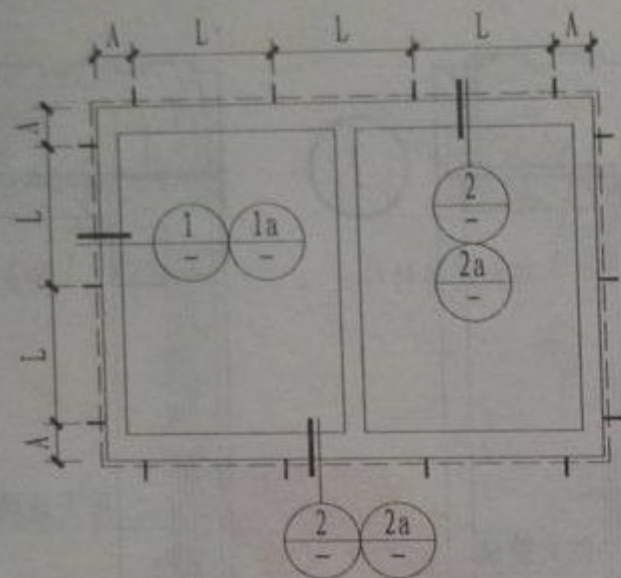
钢连接件位置立面图
