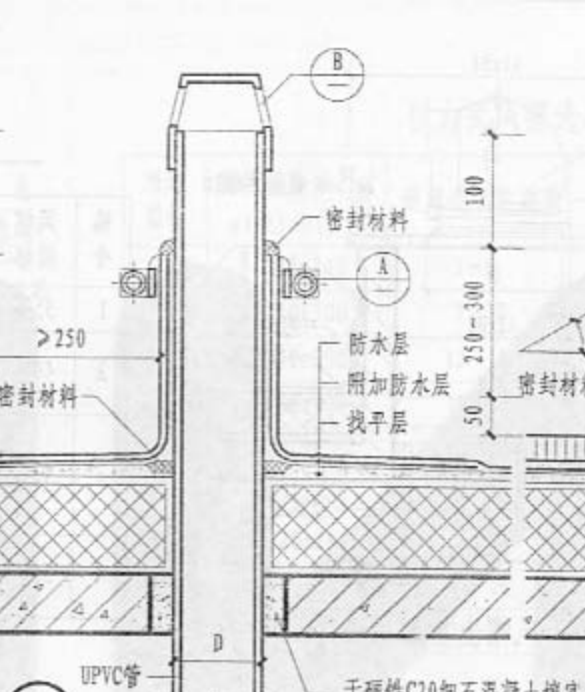
2 UPVC管出屋面(一)
