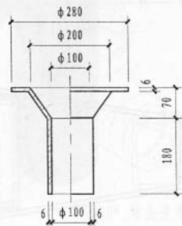
铸铁雨水口底座
