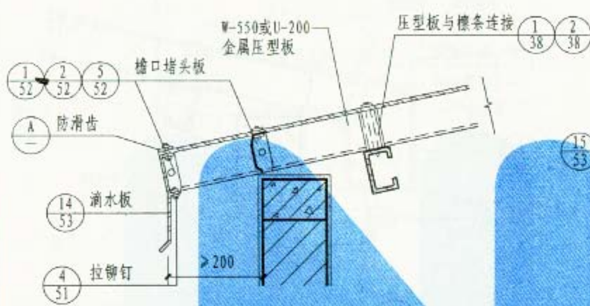
① 自由排水檐口 (用于W-550及U-200)
