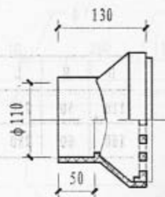
⑥ UPVC外雨水口
