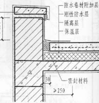
⑥ 有保温女儿墙处泛水
