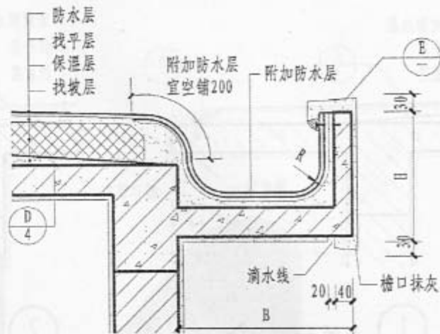
② 下沉式檐沟
