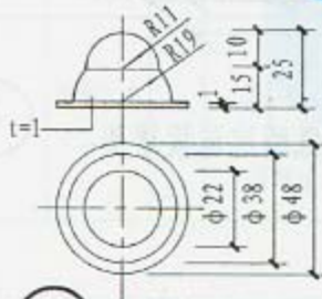
⑩ 密封条
