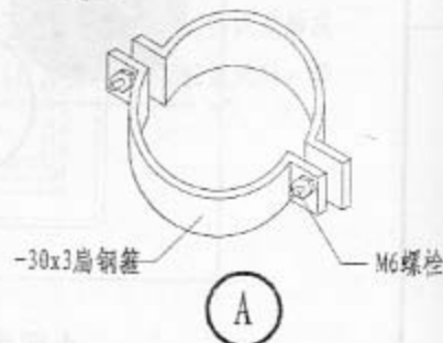
3 UPVC管出屋面(二)
