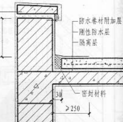
③ 无保温女儿墙处泛水
