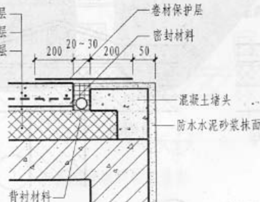
14 有保温屋面变形缝
