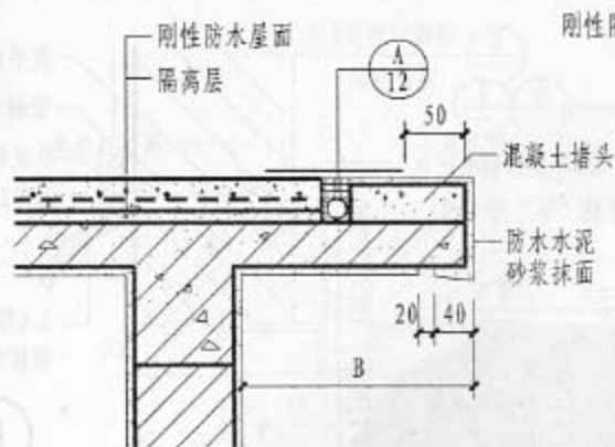
① 无保温自由排水屋面
