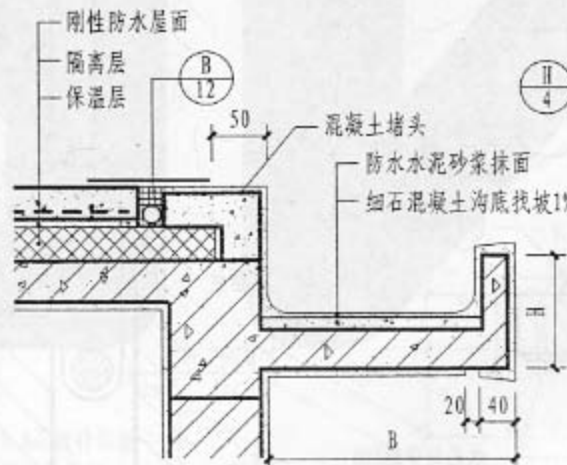
⑤ 有保温有组织排水屋面
