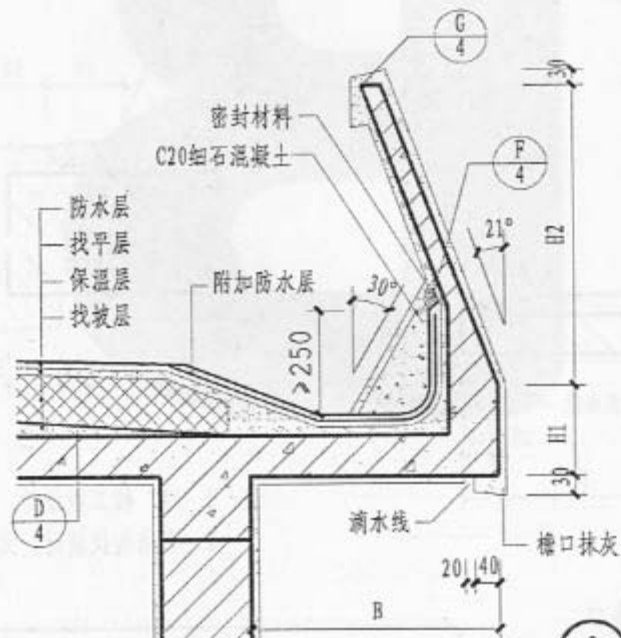
① 平出式檐沟
