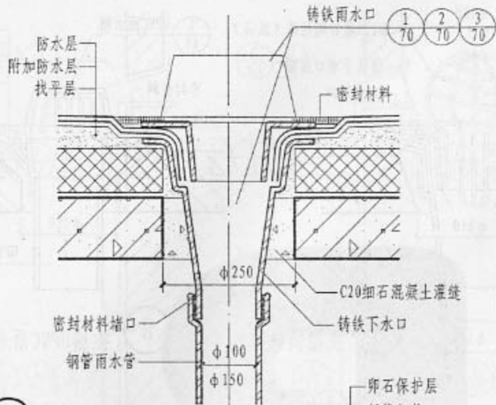
E 内排水铸铁雨水口
