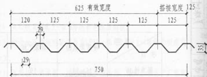
③ V-125压型板断面 金属压型板重量
