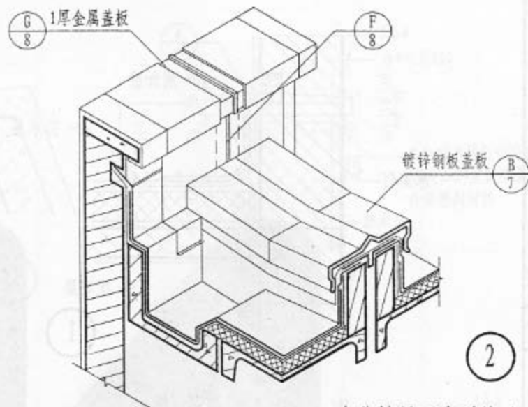
女儿墙屋面变形缝 (一)
