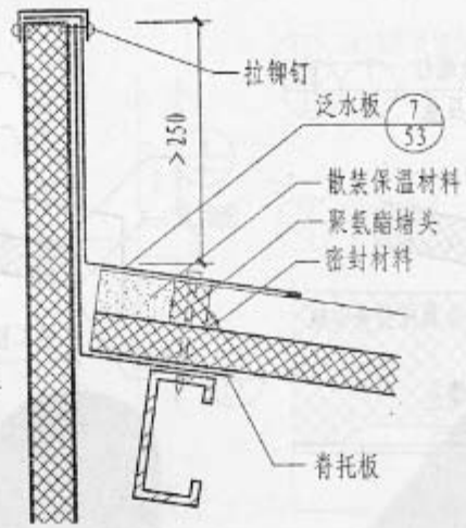
5 单坡屋脊 (一)
