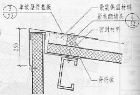
6 单坡屋脊 (二)
