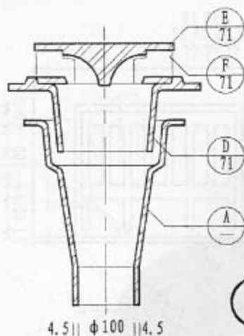
铸铁内雨水口组装
