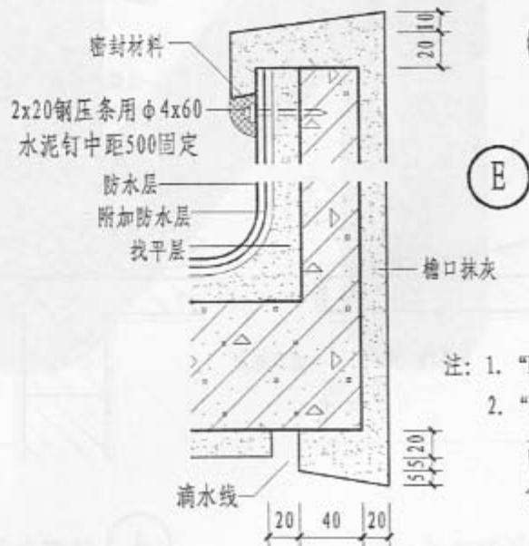
③ 斜坡式檐沟
