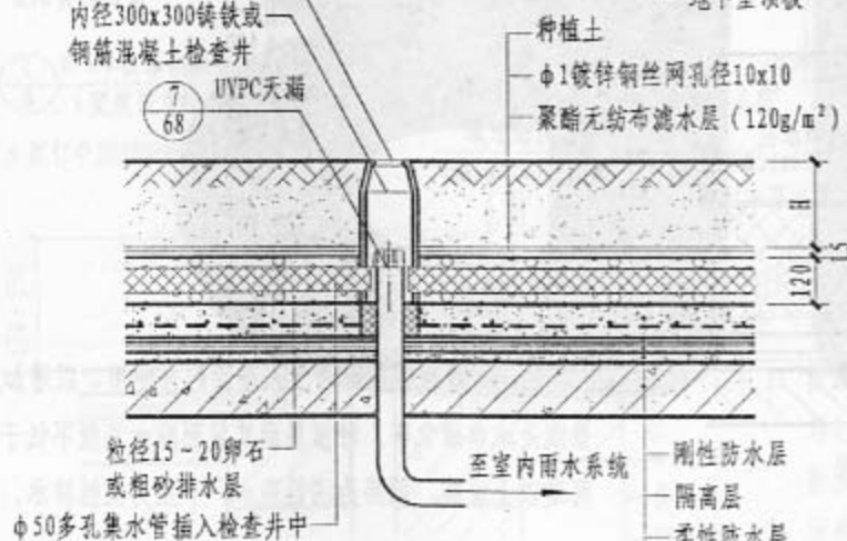
③ 室内地下室上种植屋面
