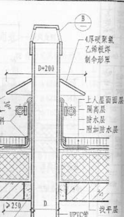
3 UPVC管出屋面(二)
