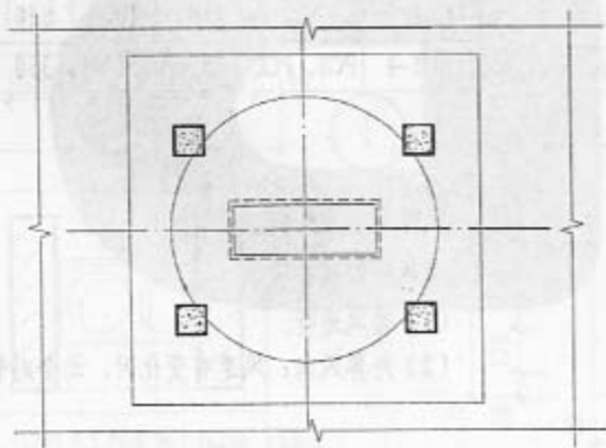
自力式风帽平面图
