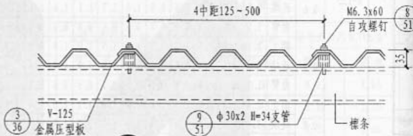
3 V-125金属压型板固定
