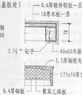
上人孔盖尺寸
