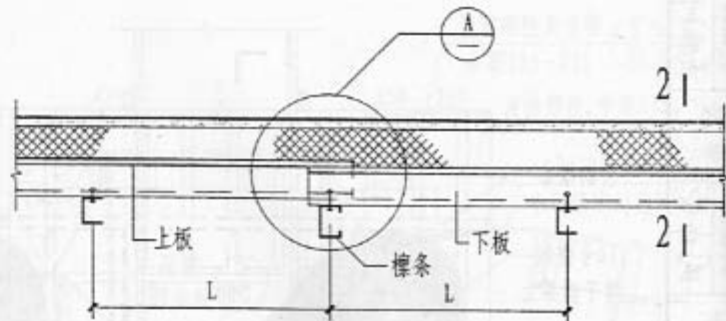
1-1 压型屋面板长向搭接
