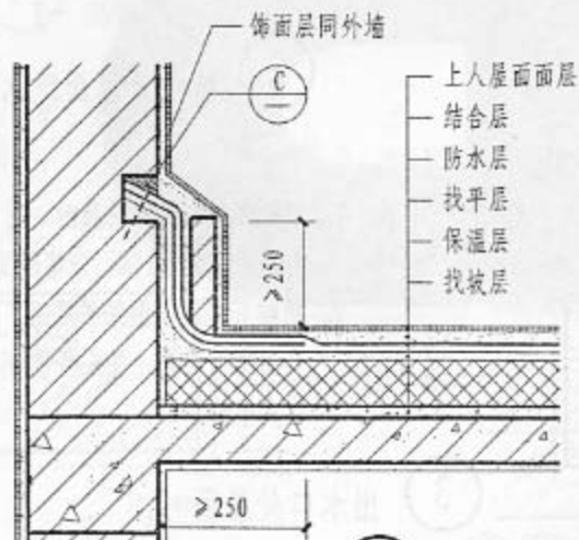
5 有饰面层处泛水
