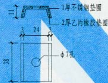
⑦ 压盖
