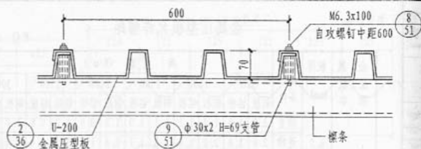
2 U-200金属压型板固定
