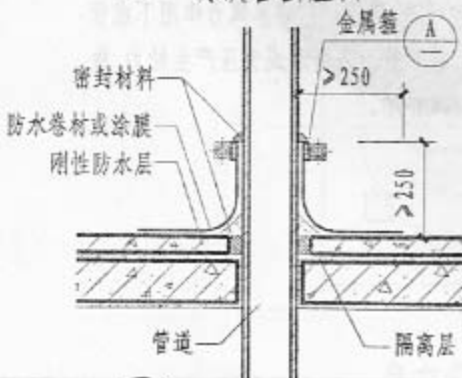
4 铸铁管出屋面
