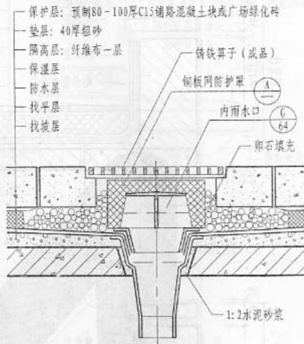
5 块材保护层及内排水口 (1-1)
