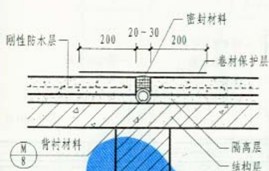
7 无保温屋面分格缝构造(一)
