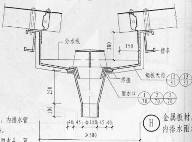
F 内排水UPVC雨水口
