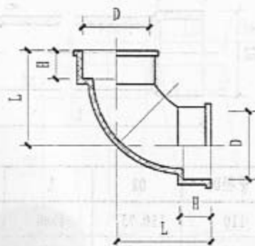
⑧ UPVC90° 弯头
