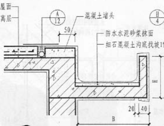
② 无保温有组织排水屋面
