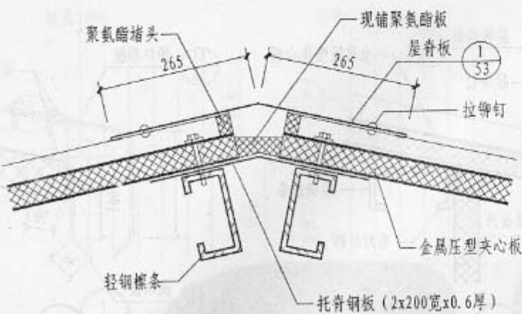
4 双坡屋脊
