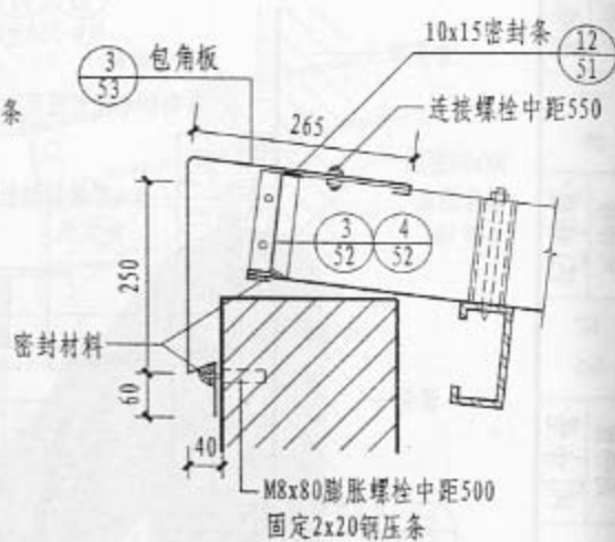
⑦ 单坡屋脊
