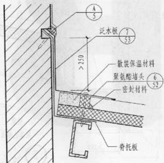
7 高低跨外
