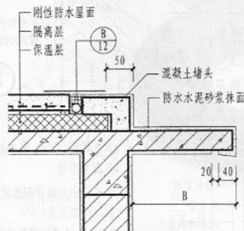
④ 有保温自由排水屋面
