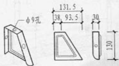
① W-550屋面板 端部檐口堵头板
