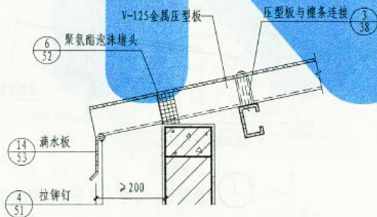
③ 自由排水檐口 (用于V-125)
