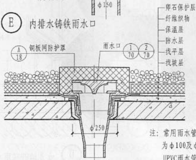
G 倒置式屋面内排水雨水口
