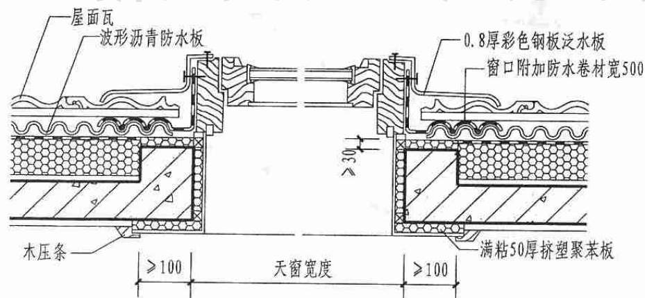
2-2剖面
