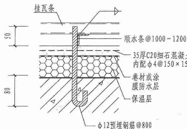
1 预埋钢筋角钢顺水条
