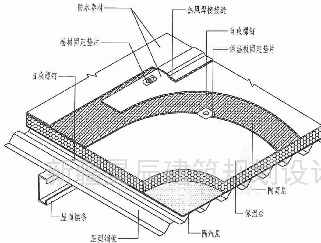
压型钢板复合保温卷材防水屋面(机械固定1)构造示意
