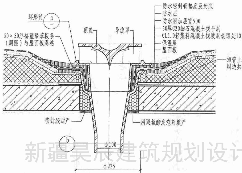
65型雨水斗屋面（天沟）安装图
