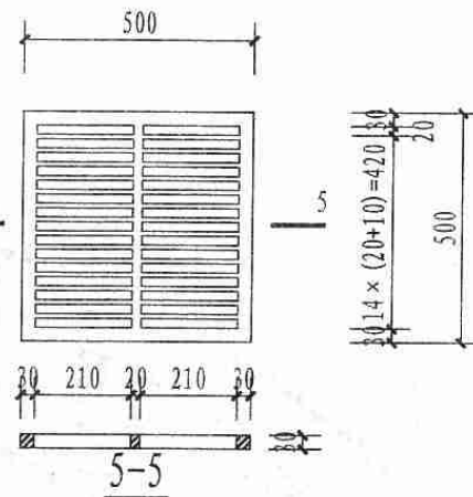
铸铁算子
