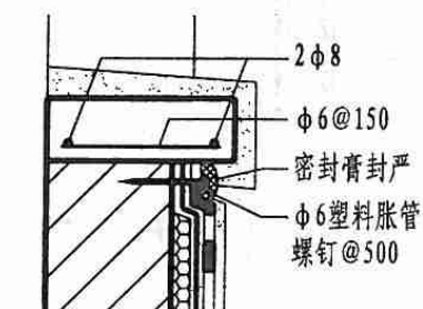
A 泛水
