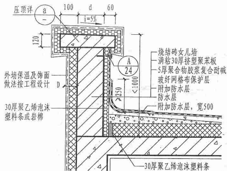
1 烧砖女儿墙构造详图
