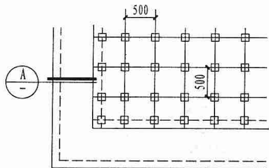
1 挑檐屋顶平面示例
