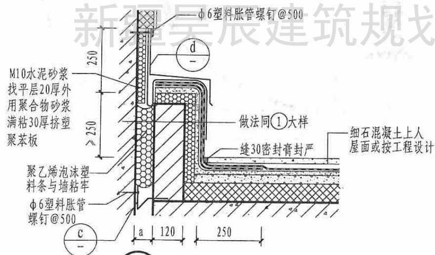
2 高低跨上人屋面
