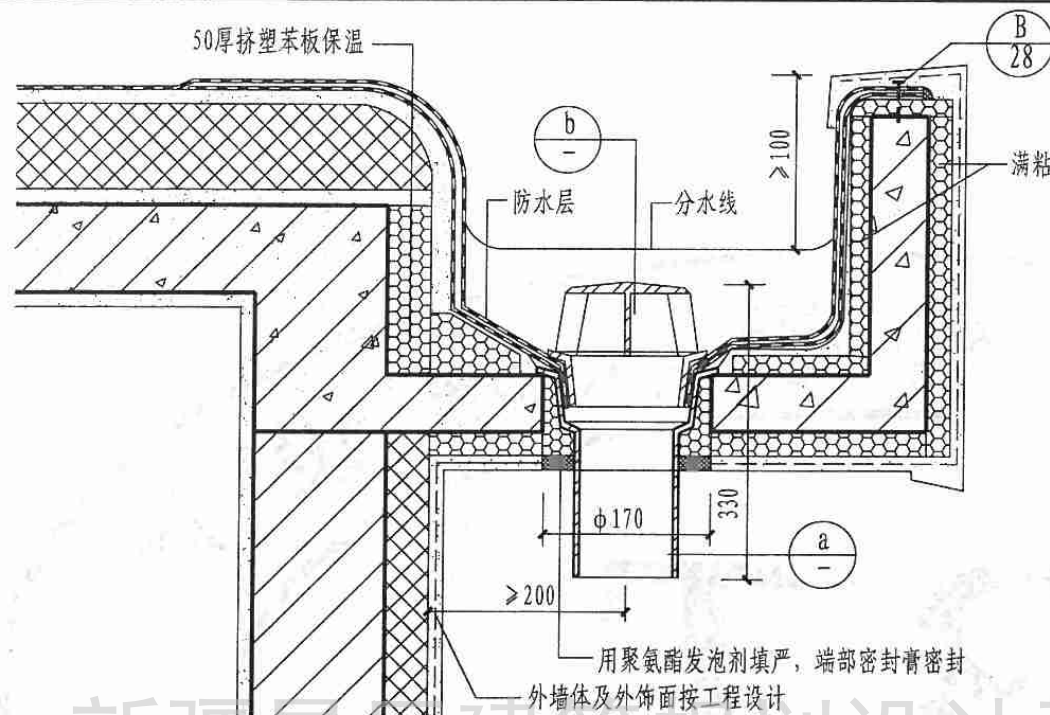
挑檐水落口
