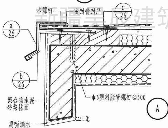
1 自由落水挑檐详图
