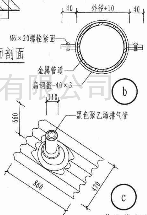
成品排气瓦
