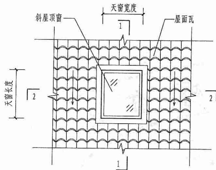
天窗平面
