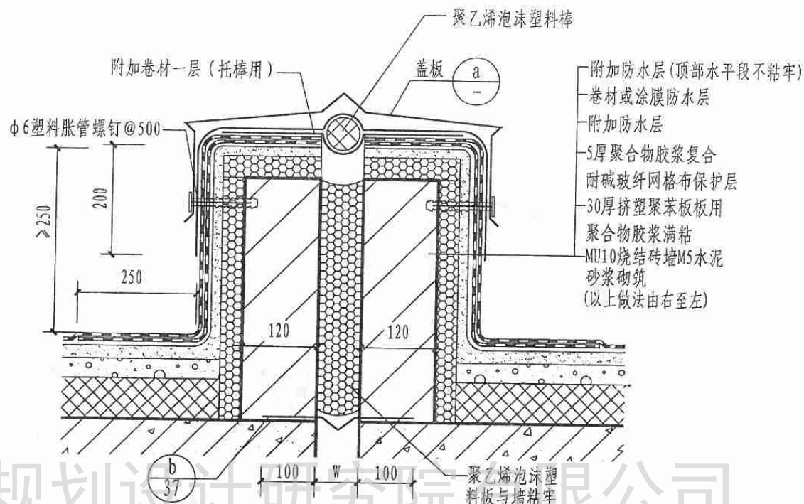
A 卷材防水屋面变形缝
