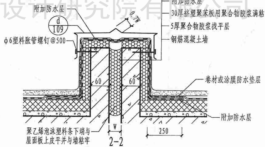
块瓦坡屋面构造 变形缝详图(二)
