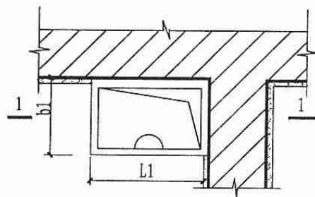
1 排气道平面位置图
