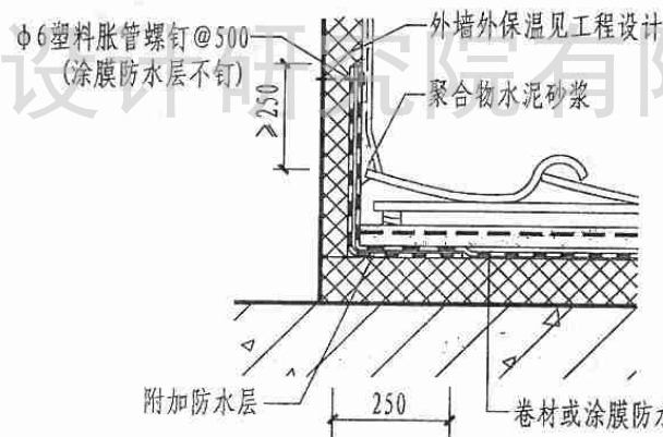
4 泛水
