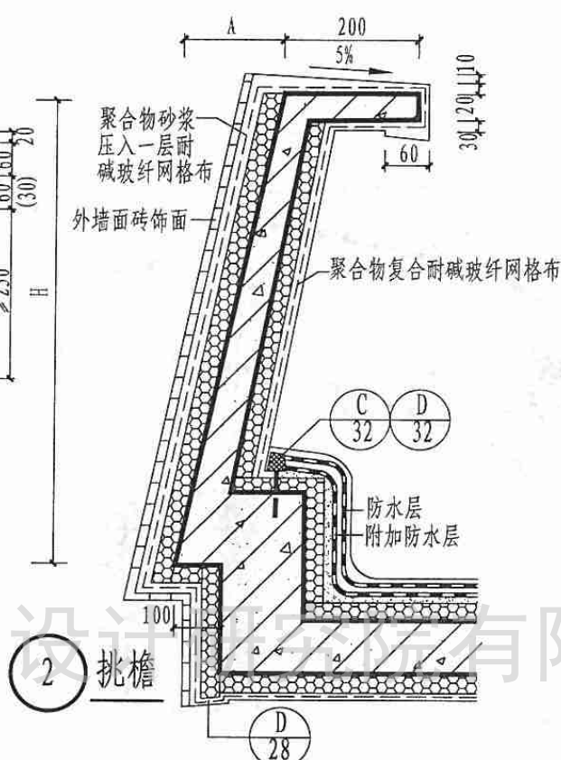
A 用于卷材防水层
