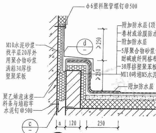
1 高低跨不上人屋面
