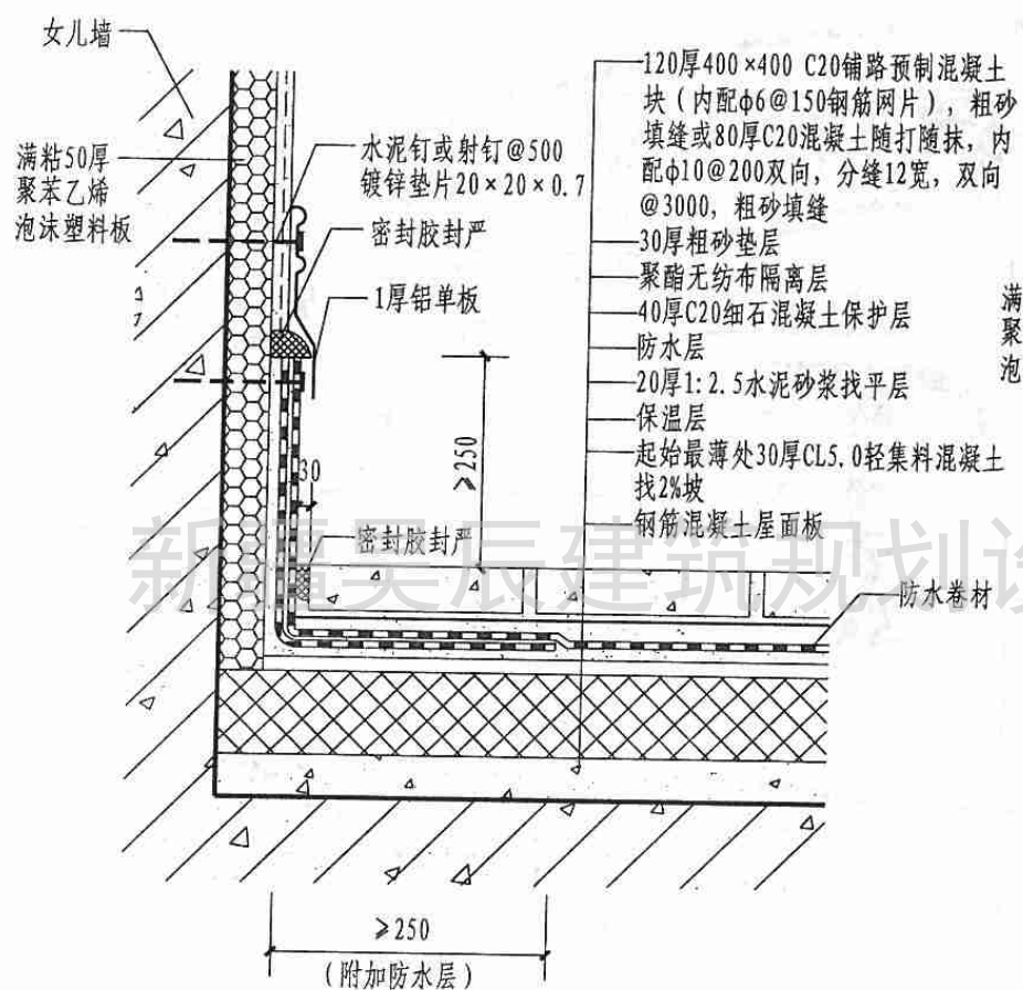
2 女儿墙泛水
