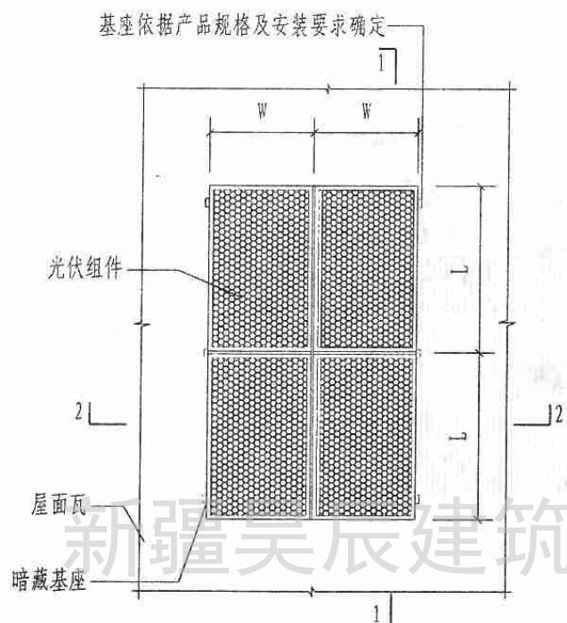
嵌入式光伏组件安装平面图
