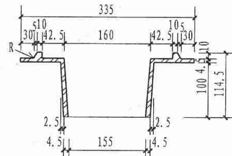
a 环形筒剖面图
