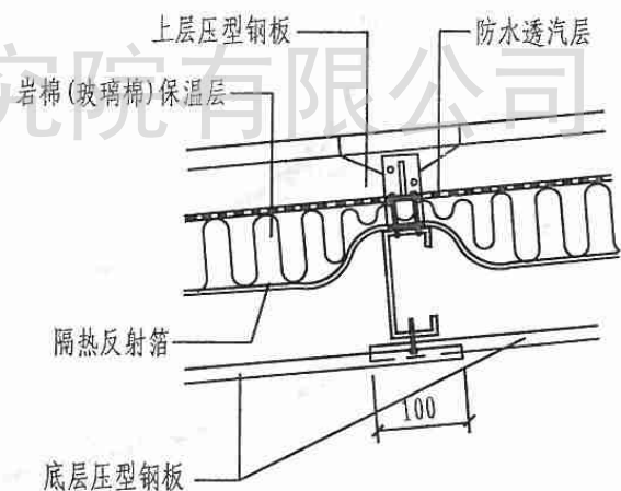
屋面底层板纵向搭接
