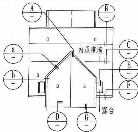
双坡顶平面示例
