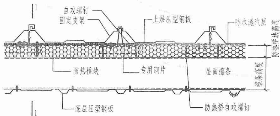
屋面横向连接
