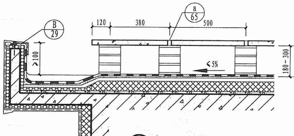
A 架空屋面剖面示例
