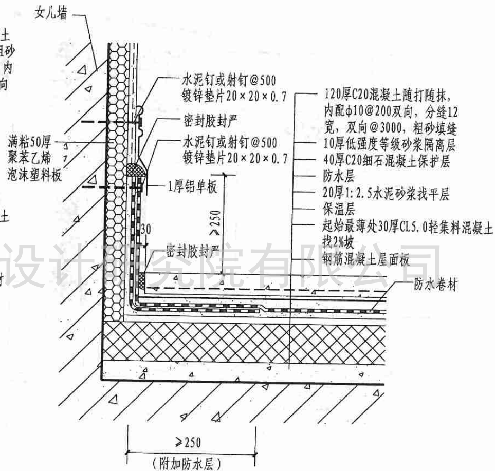
3 女儿墙泛水
