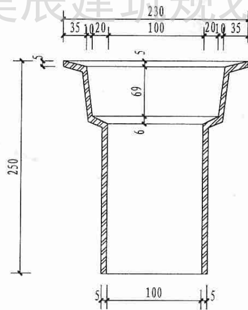
挑檐水落口
