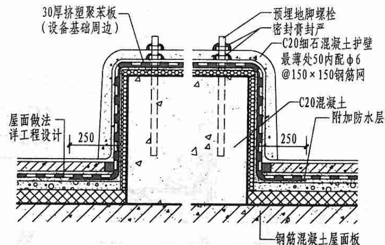
2 设备基座
