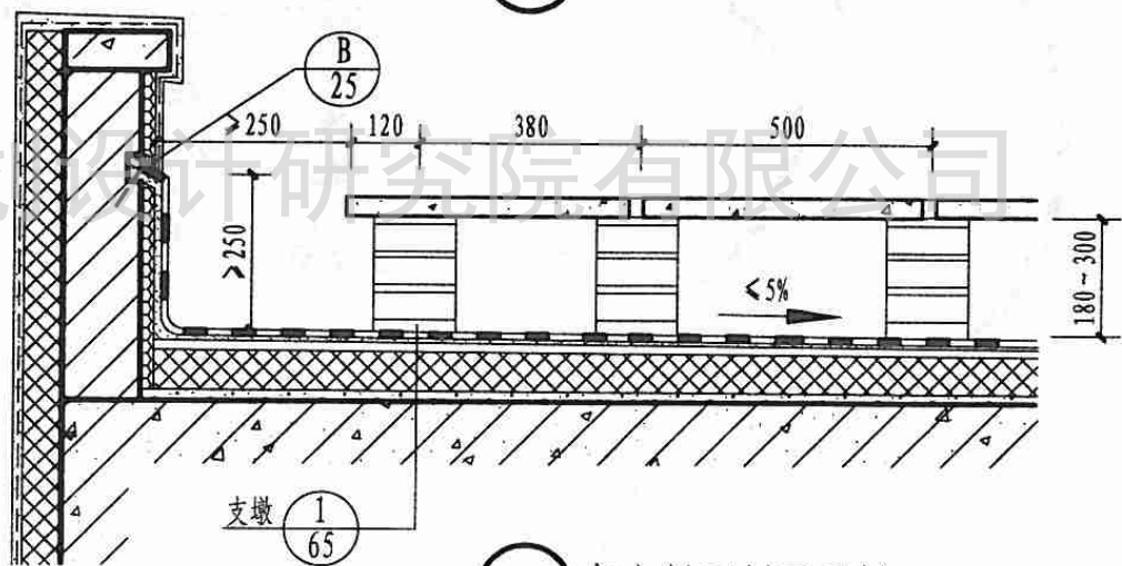
B 架空屋面剖面示例
