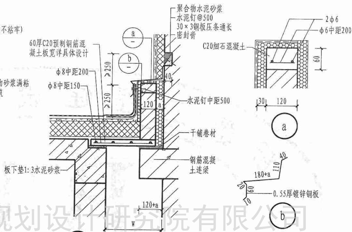
3 高低跨不上人屋面
