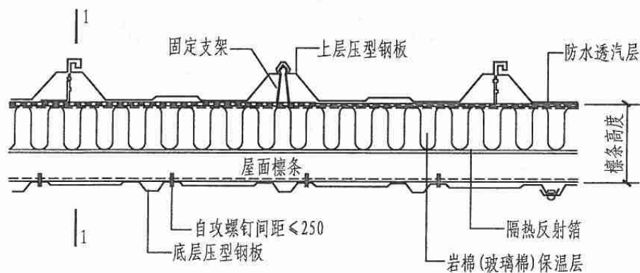
屋面横向连接
