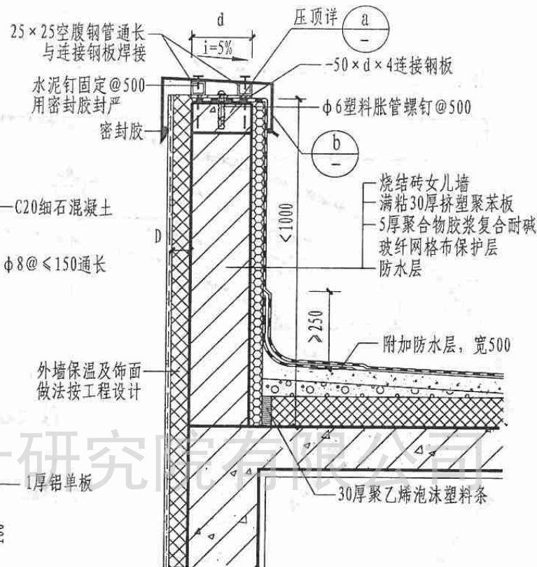
3 烧砖女儿墙构造详图
