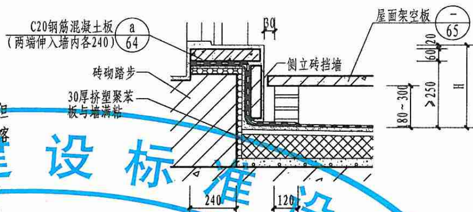
1 门槛做法
