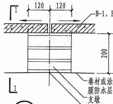
2 屋脊支墩
