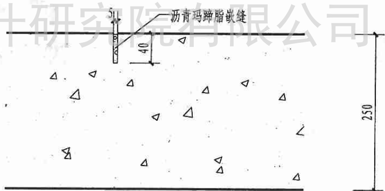
B 路面缩缝
