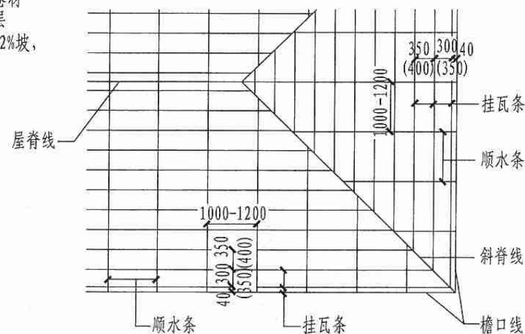
顺水条、挂瓦条平面布置
