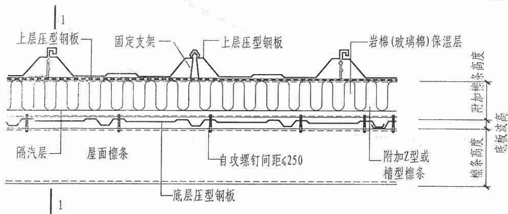
屋面横向连接
