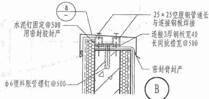
钢筋混凝土檐沟构造详图(二)
