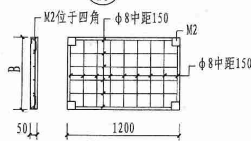
C 预制斜板
