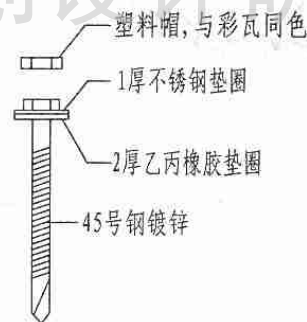
自攻螺丝
