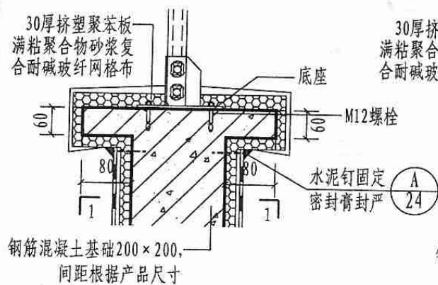
A 混凝土支墩
