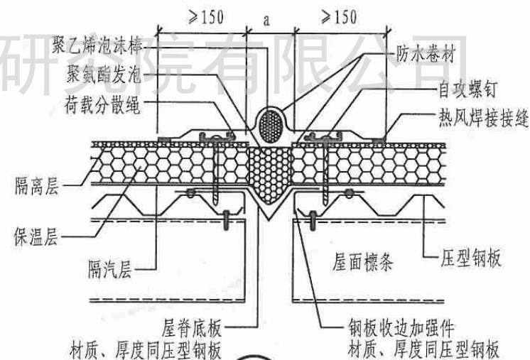
2 水平变形缝
