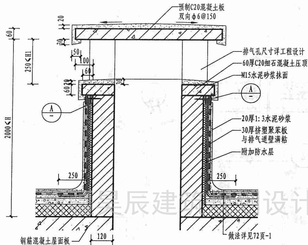
烧结砖砌排气道
