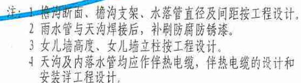
压型钢板复合保温屋面 女儿墙内檐沟
