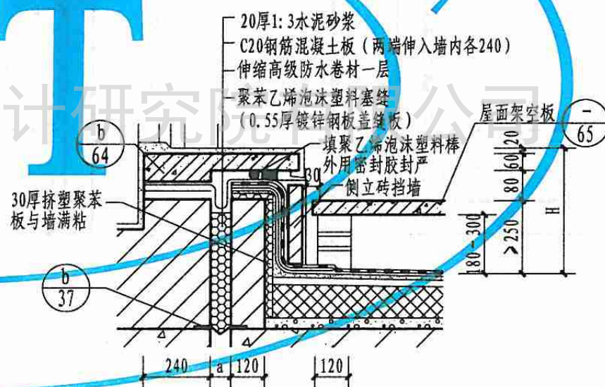
2 变形缝处门槛做法
