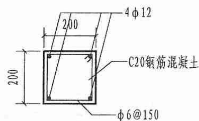
2-2 (混凝土墩配筋)
