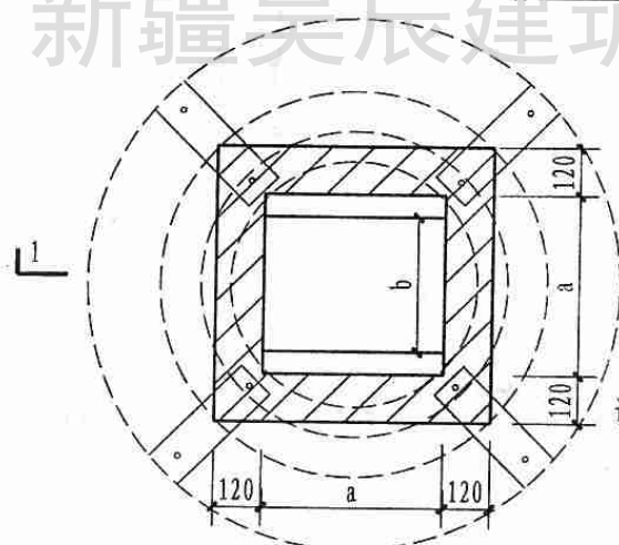
1 排气道出屋面图
