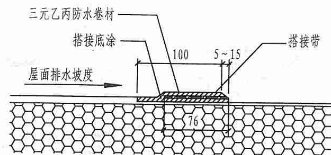
2 三元乙丙防水卷材标准搭接做法
