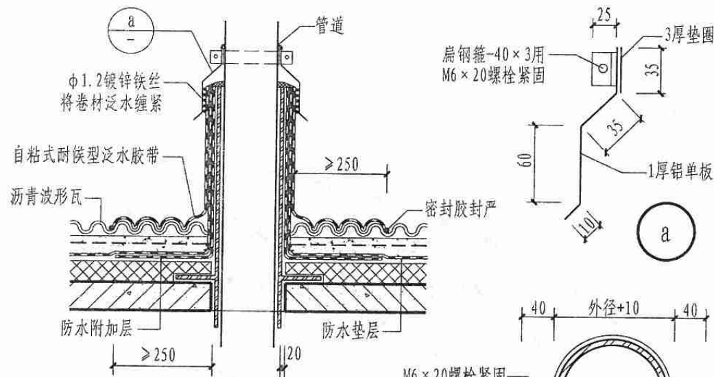
2 管道出屋面剖面
