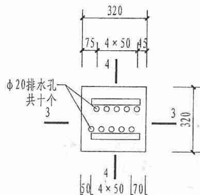
排水板PB-1
