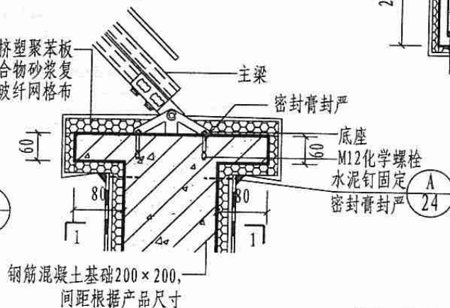
B 混凝土支墩
