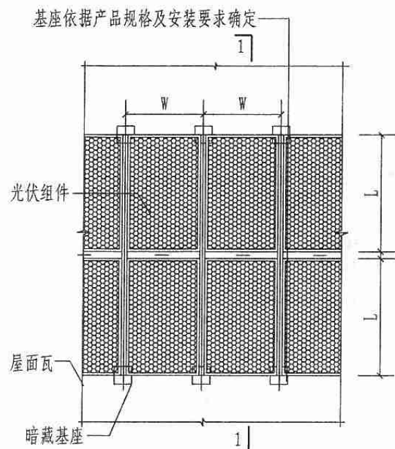
架空式光伏组件安装平面图
