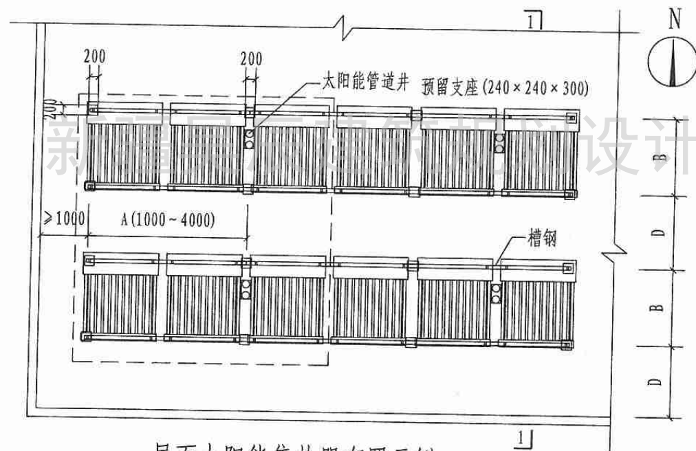
屋面太阳能集热器布置示例
