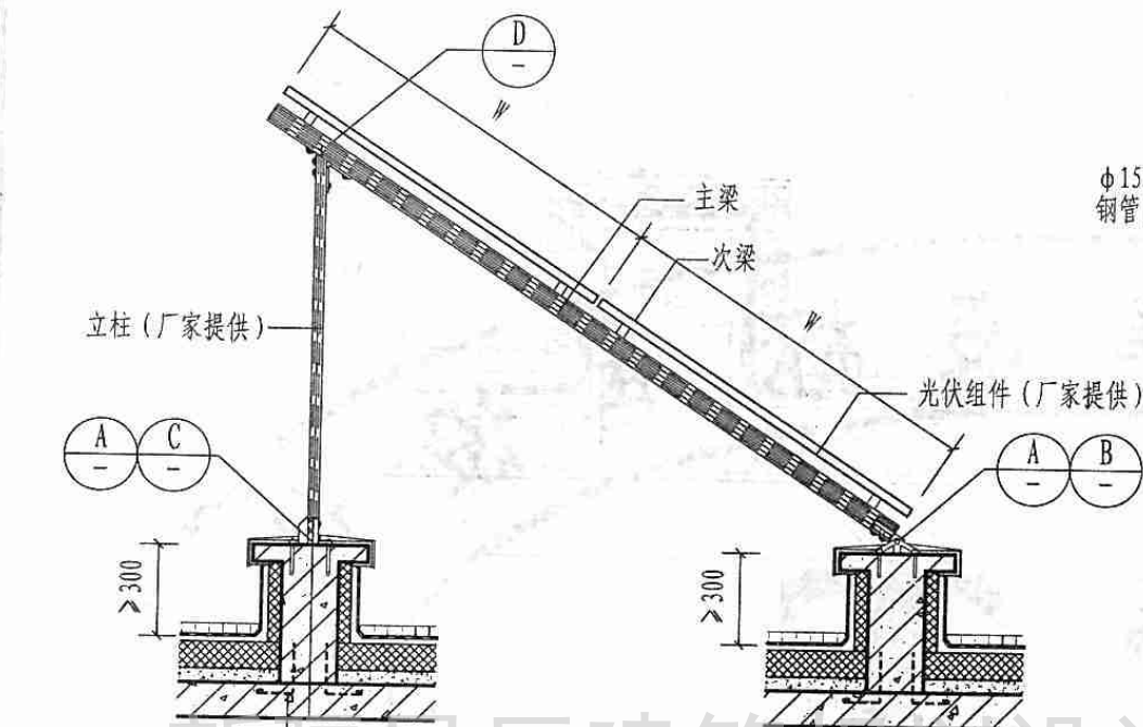
2-2剖面图
