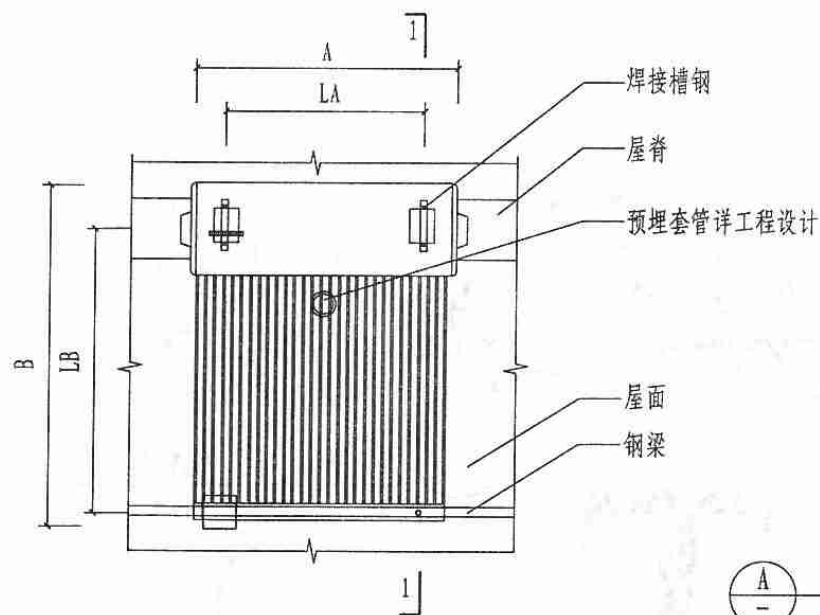
整体式太阳能集热器安装平面图
