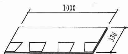
图二 双层沥青瓦
