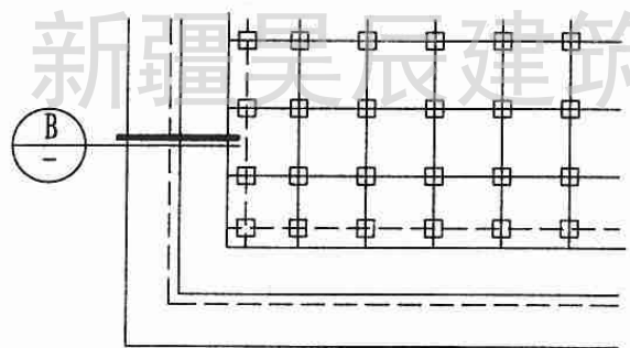
2 女儿墙屋顶平面示例
