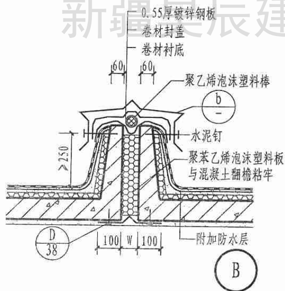
屋面变形缝示意
