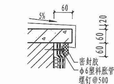
A 用于卷材防水层
