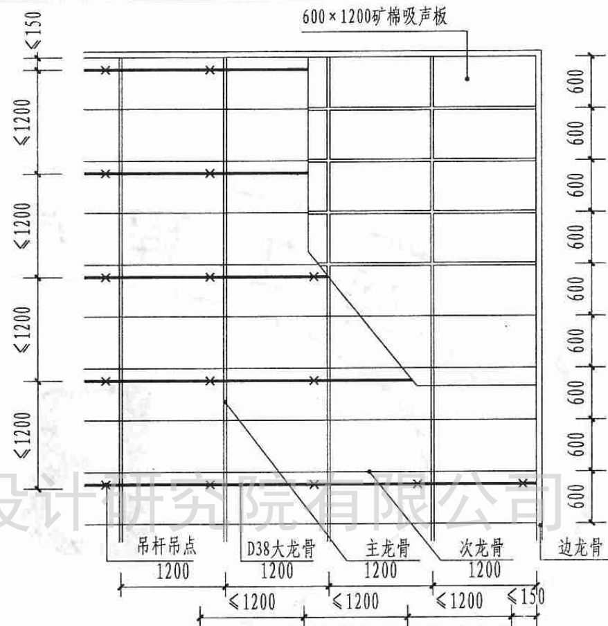
600×1200矿棉吸声板明架吊顶平面
