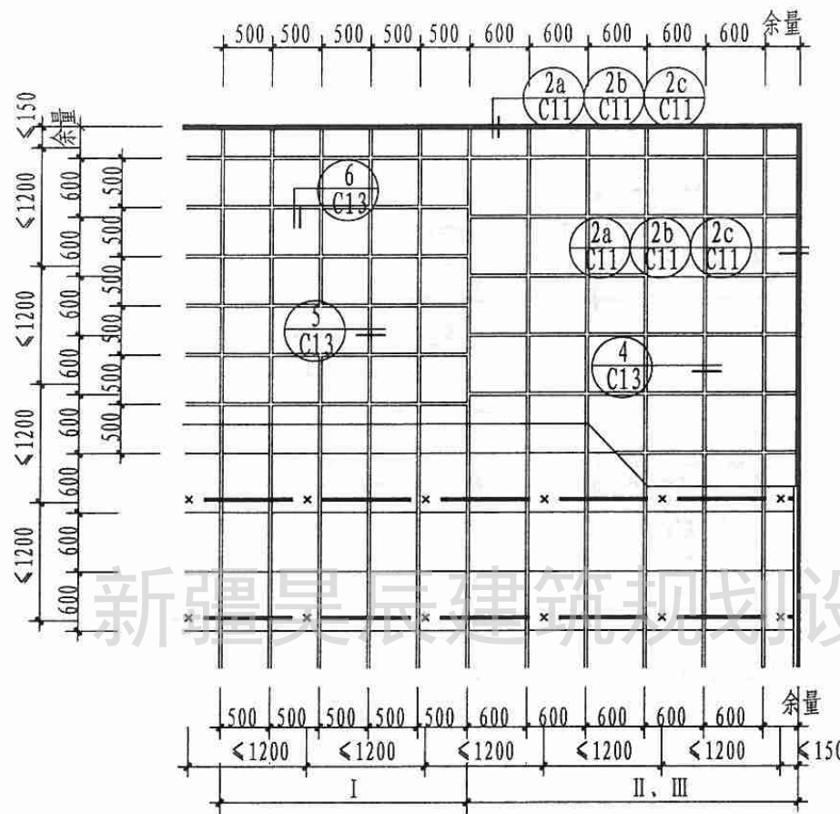
T3 A. B. C明龙骨双层龙骨单层方形板吊顶
